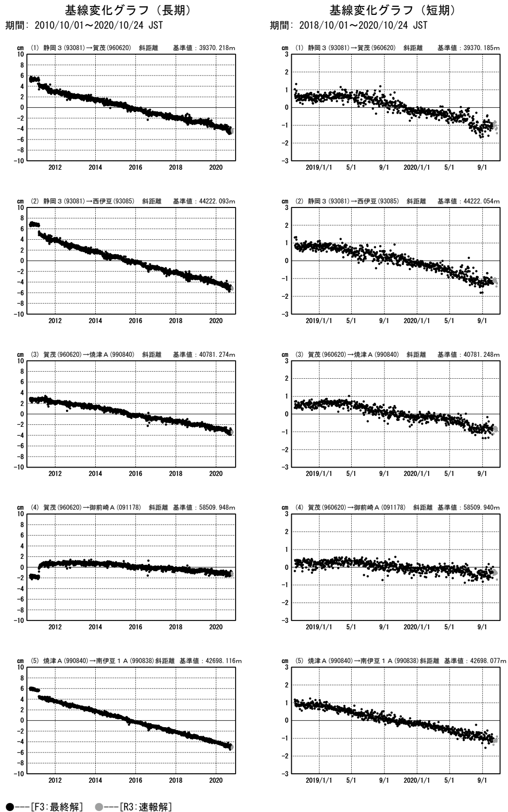
第 19 図 駿河湾周辺 GNSS 連続観測点観測結果 (斜距離) (1)
