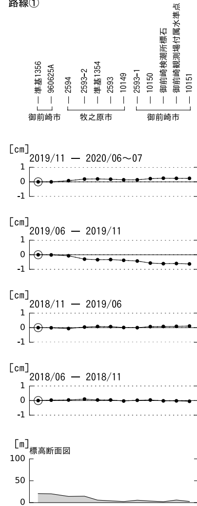
第 11 図 水準測量による御前崎先端部の上下変動 (1)
