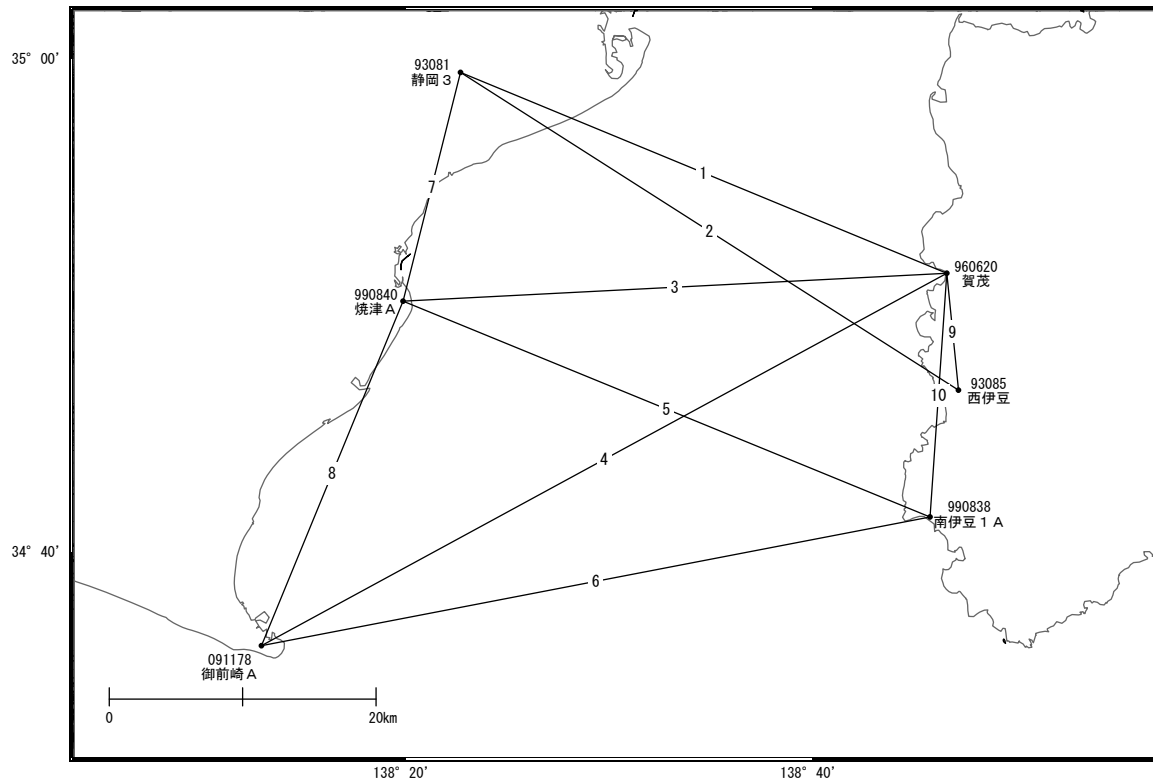
基線図
