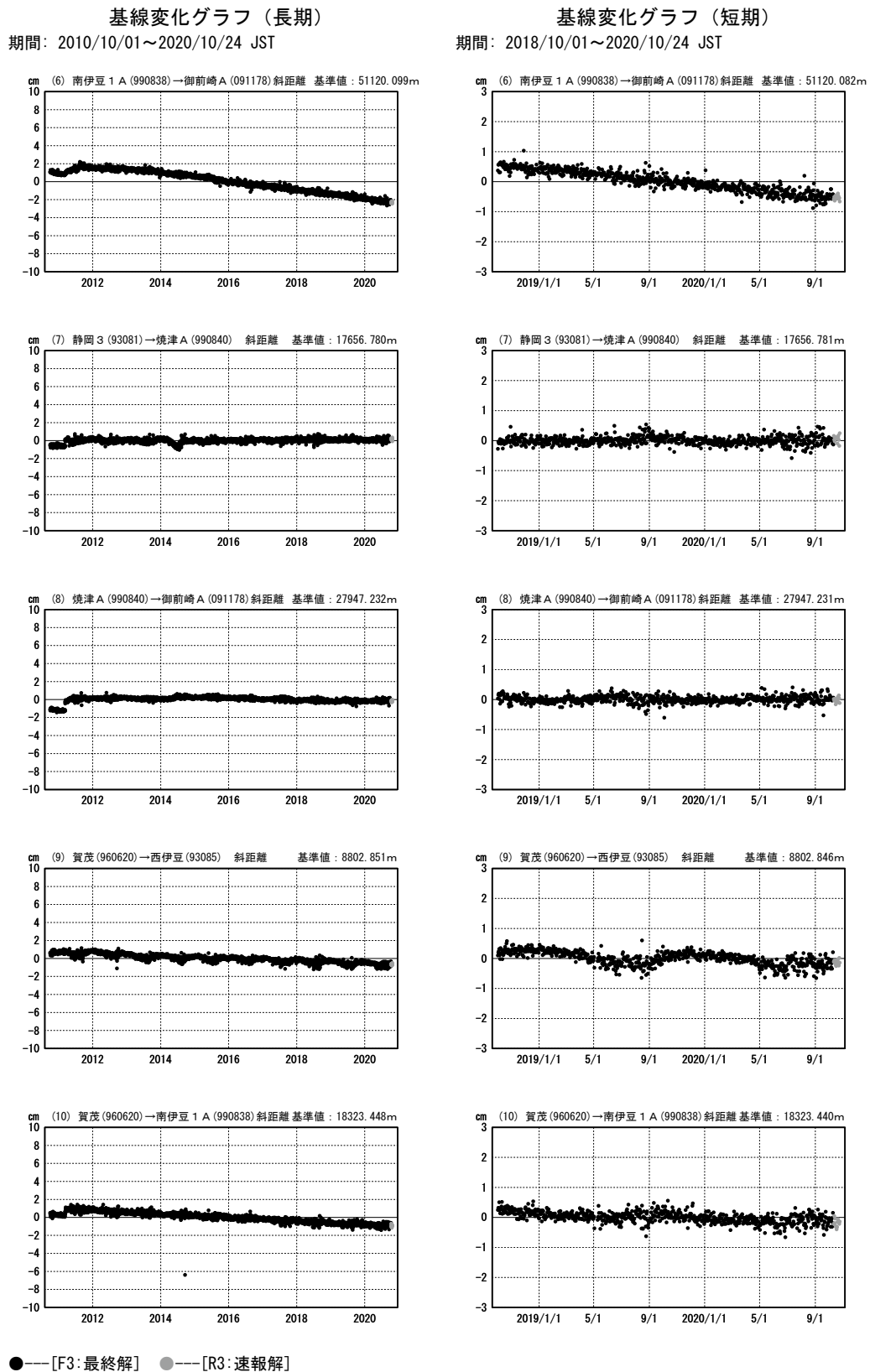
第 20 図 駿河湾周辺 GNSS 連続観測点観測結果 (斜距離) (2)
