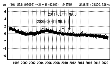
第 15 図 御前崎周辺 GNSS 連続観測点観測結果 (斜距離) (2)
