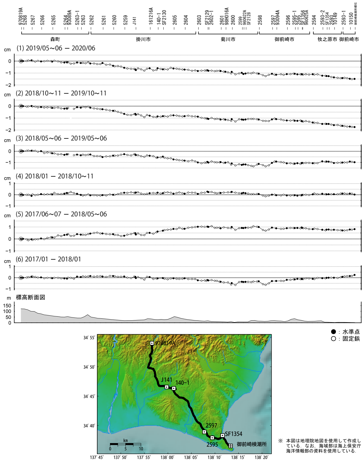
第 6 図 水準測量による森町～掛川市～御前崎市間における上下変動 Fig. 6 Vertical displacements from Mori town to Omaezaki city via Kakegawa city.
