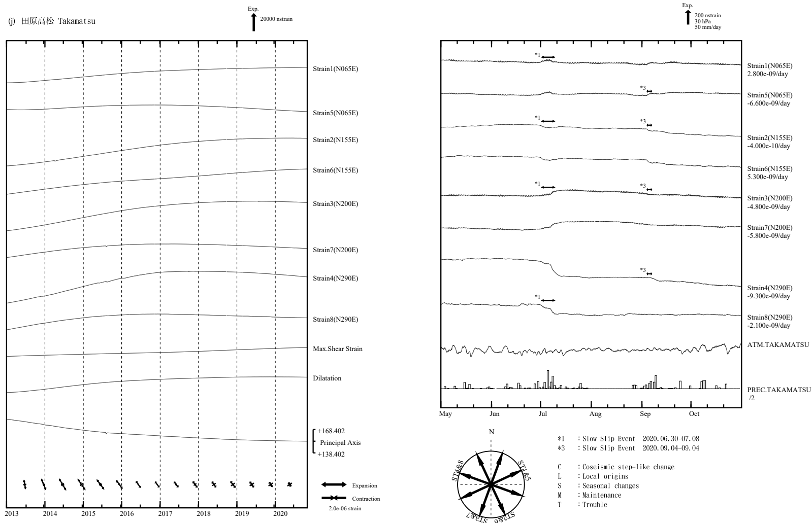
第 4 図 (j) 左：2013 年 1 月以後の多成分ひずみ計変化（日平均値）。主ひずみ・最大せん断ひずみ・面積ひずみは各方向成分から計算されている。
