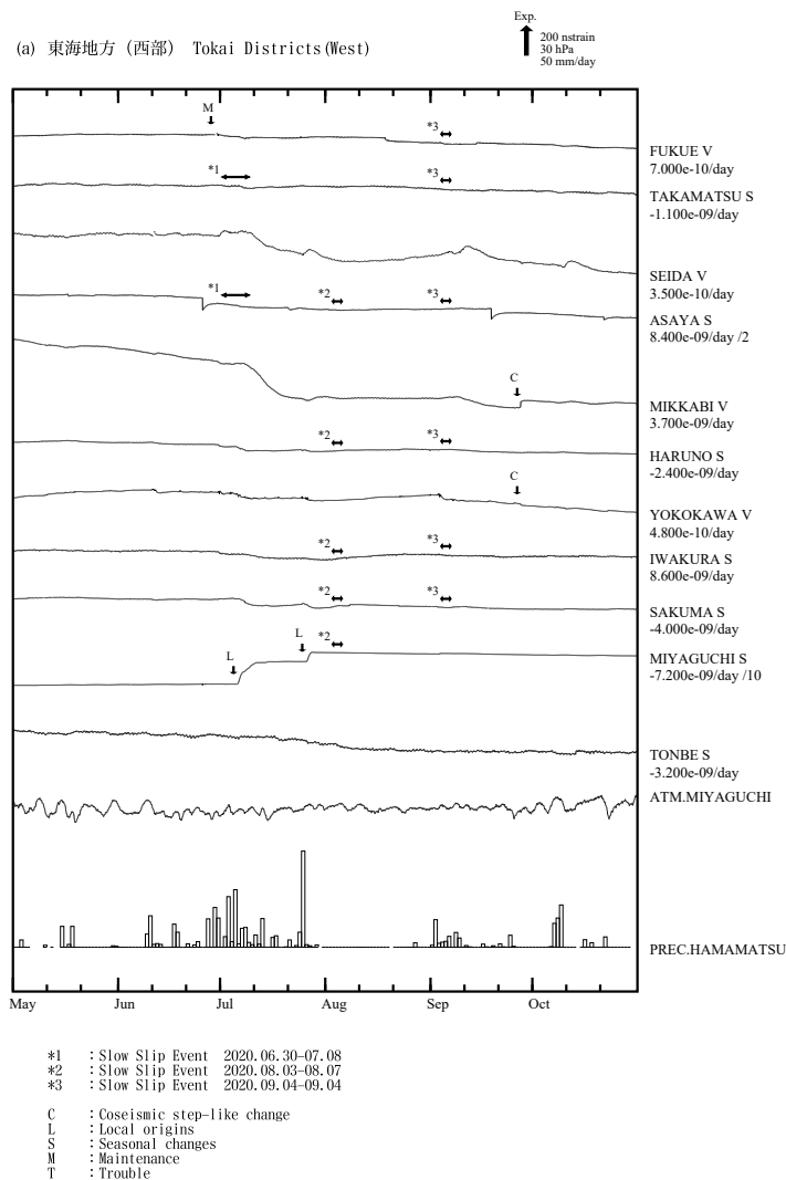
第3図 (a), (b) 2020年5月～10月の東海・伊豆・南関東地域における区域別体積ひずみ (V) 及び面積ひずみ (S) の変化 (時間値: 気圧・潮汐・降水補正した値). 各図下部に区域を代表する気圧変化と降水量を示す. 地点名の下に D strain/day 及び /M はそれぞれ1日あたりのトレンド変化量を D として補正していること及び縮尺を 1/M 倍にして表示していることを示している.
