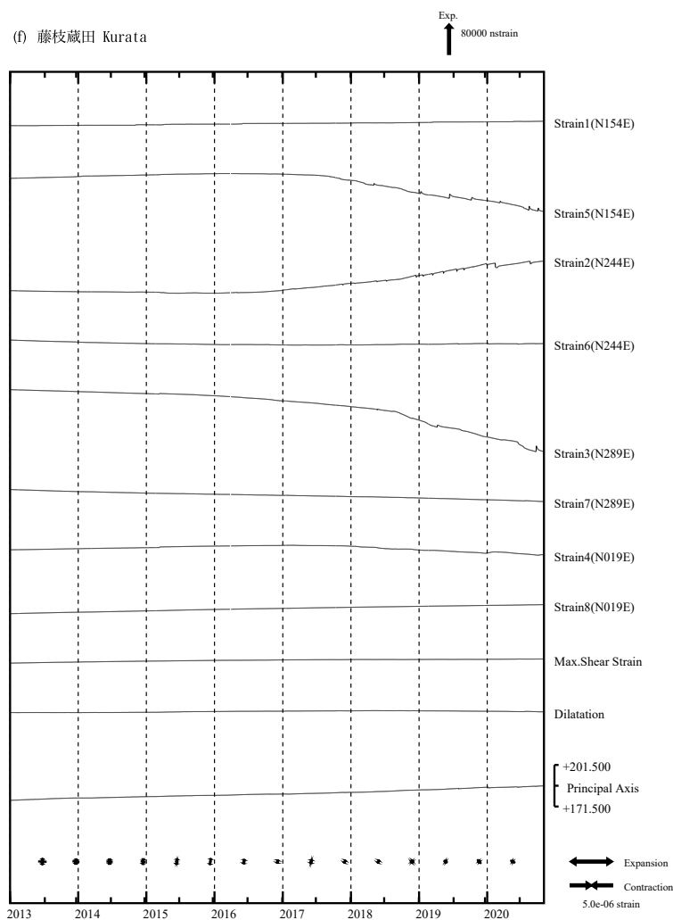
第 4 図 (f) 左 : 2013 年 1 月以後の多成分ひずみ計変化 (日平均値)。主ひずみ・最大せん断ひずみ・面積ひずみは各方向成分から計算されている。
