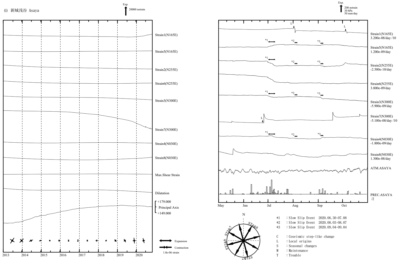
第 4 図 (i) 左 : 2013 年 1 月以後の多成分ひずみ計変化 (日平均値). 主ひずみ・最大せん断ひずみ・面積ひずみは各方向成分から計算されている. 右 : 2020 年 5 月～10 月の多成分ひずみ計変化 (時間値 : 気圧・潮汐・地磁気補正した値). 各図下部に気圧変化と降水量を示す.
