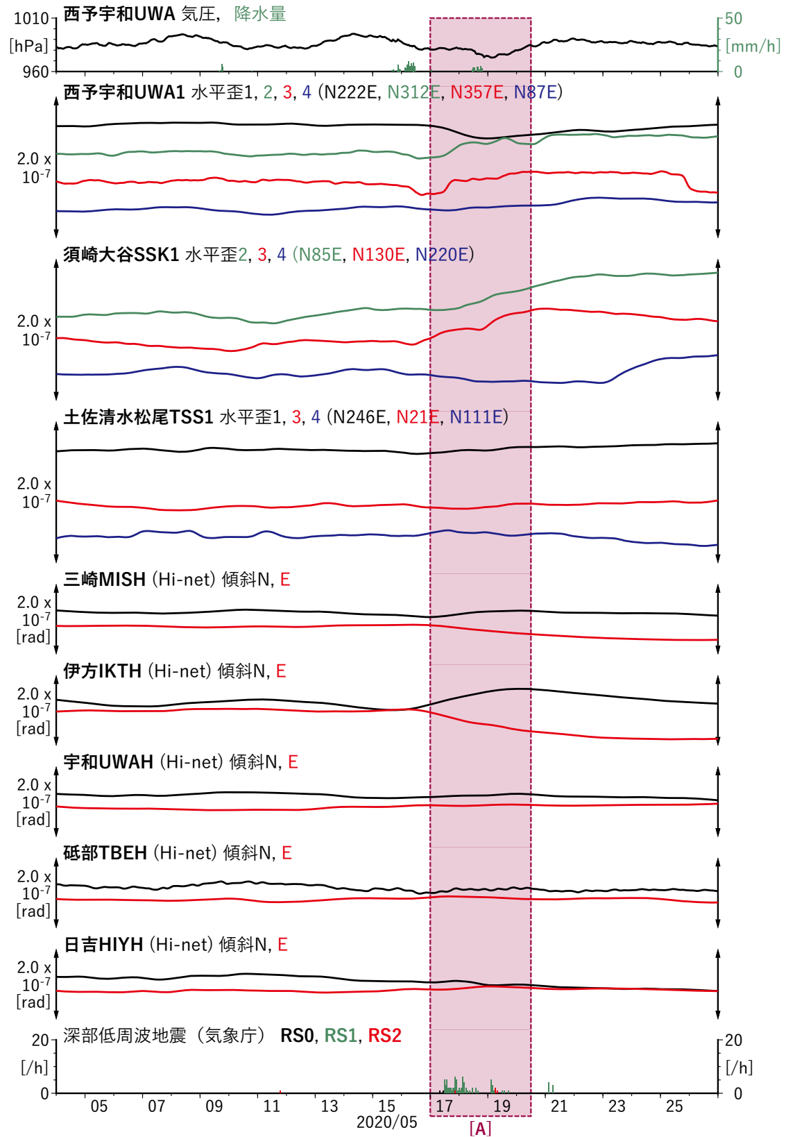
第 5 図 四国地方における歪・傾斜・地下水位の観測結果と深部低周波地震の検出数 (2020/05/04 ~ 2020/05/27)。
