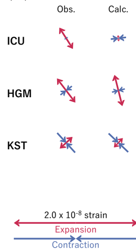
第 3 図 第 2 図 [A] を説明する断層モデル。以下の凡例の説明は以降の同様の図に共通。黒・緑・青の丸印はそれぞれ産総研・気象庁および静岡県・防災科研 Hi-net の観測点、緑の小さな丸印は気象庁の推定した低周波地震。(a) 1 段階目の結果。灰色の濃淡は残差の総和で、赤色矩形が残差の総和が最小となる断層面の位置（大きさは 20x20 km で固定）。(b1) 2 段階目の結果。赤色矩形が残差の総和が最小となる断層面。矢印は傾斜の観測値と計算値の比較。灰色矩形は最近周辺で発生した短期的 SSE の推定断層面（番号との対応は本文参照）。(b2) 主歪の観測値と(b1)に示した断層モデルから求めた計算値との比較。(b3) 体積歪の観測値と(b1)に示した断層モデルから求めた計算値との比較。
