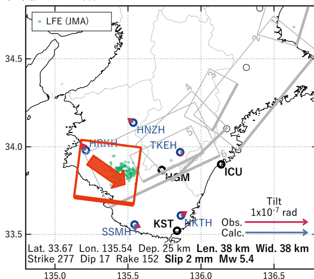
第 3 図 第 2 図 [A] を説明する断層モデル。以下の凡例の説明は以降の同様の図に共通。黒・緑・青の丸印はそれぞれ産総研・気象庁および静岡県・防災科研 Hi-net の観測点、緑の小さな丸印は気象庁の推定した低周波地震。(a) 1 段階目の結果。灰色の濃淡は残差の総和で、赤色矩形が残差の総和が最小となる断層面の位置（大きさは 20x20 km で固定）。(b1) 2 段階目の結果。赤色矩形が残差の総和が最小となる断層面。矢印は傾斜の観測値と計算値の比較。灰色矩形は最近周辺で発生した短期的 SSE の推定断層面（番号との対応は本文参照）。(b2) 主歪の観測値と(b1)に示した断層モデルから求めた計算値との比較。(b3) 体積歪の観測値と(b1)に示した断層モデルから求めた計算値との比較。
