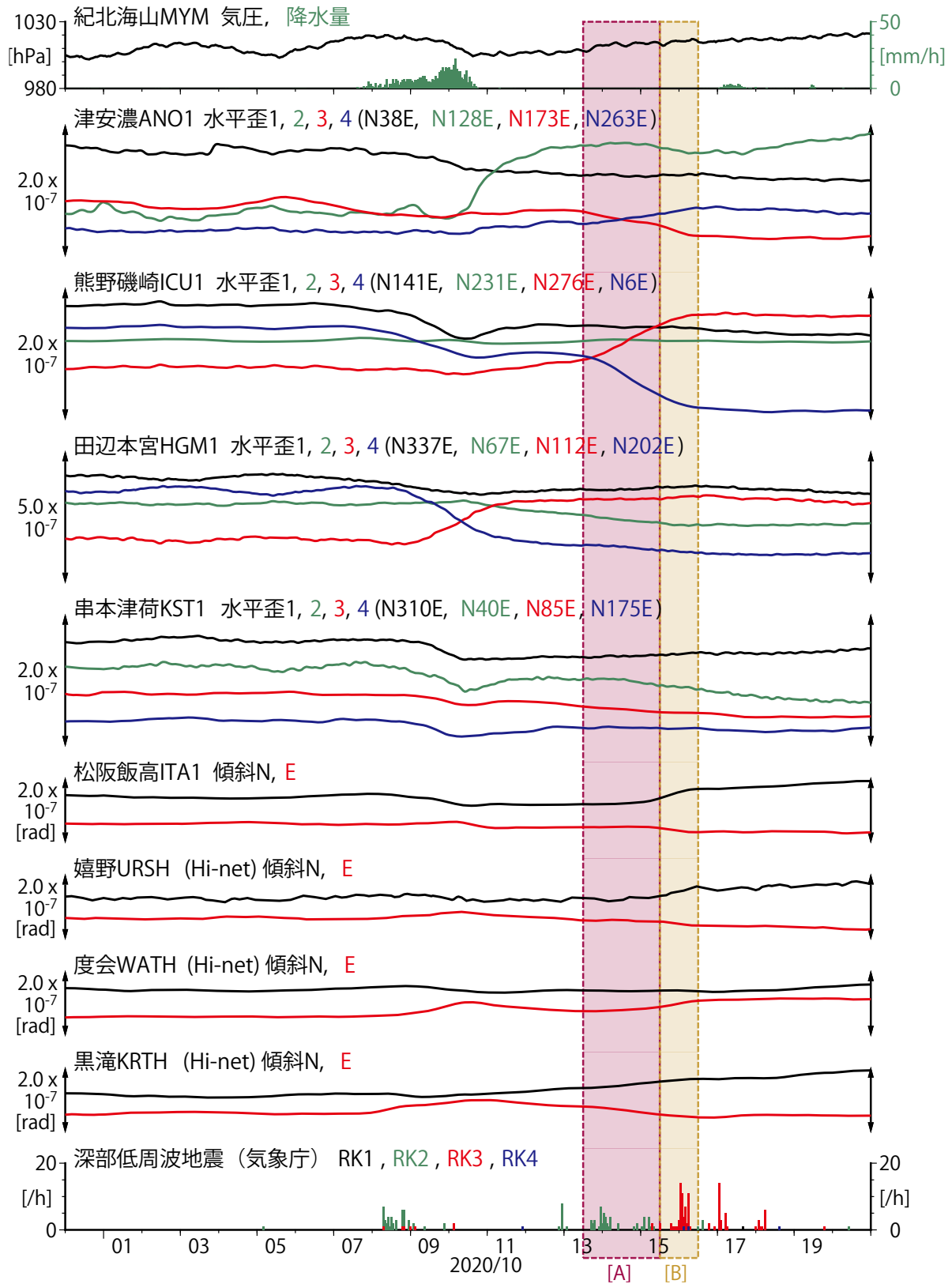
第 39 図 紀伊半島における歪・傾斜の観測結果と深部低周波地震の検出数 (2020/09/30 ~ 2020/10/21).
