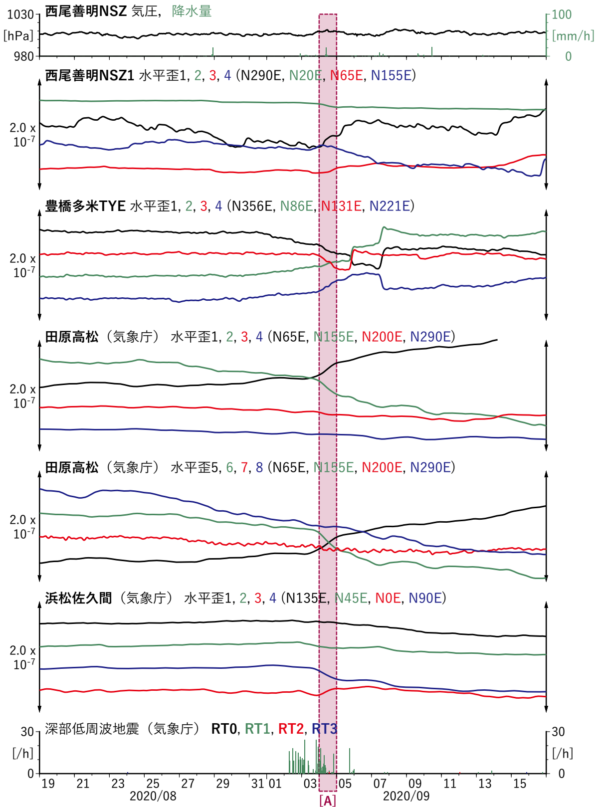
第 32 図 東海地方における歪・傾斜の観測結果と深部低周波地震の検出数 (1) (2020/08/19 ~ 2020/09/17).
