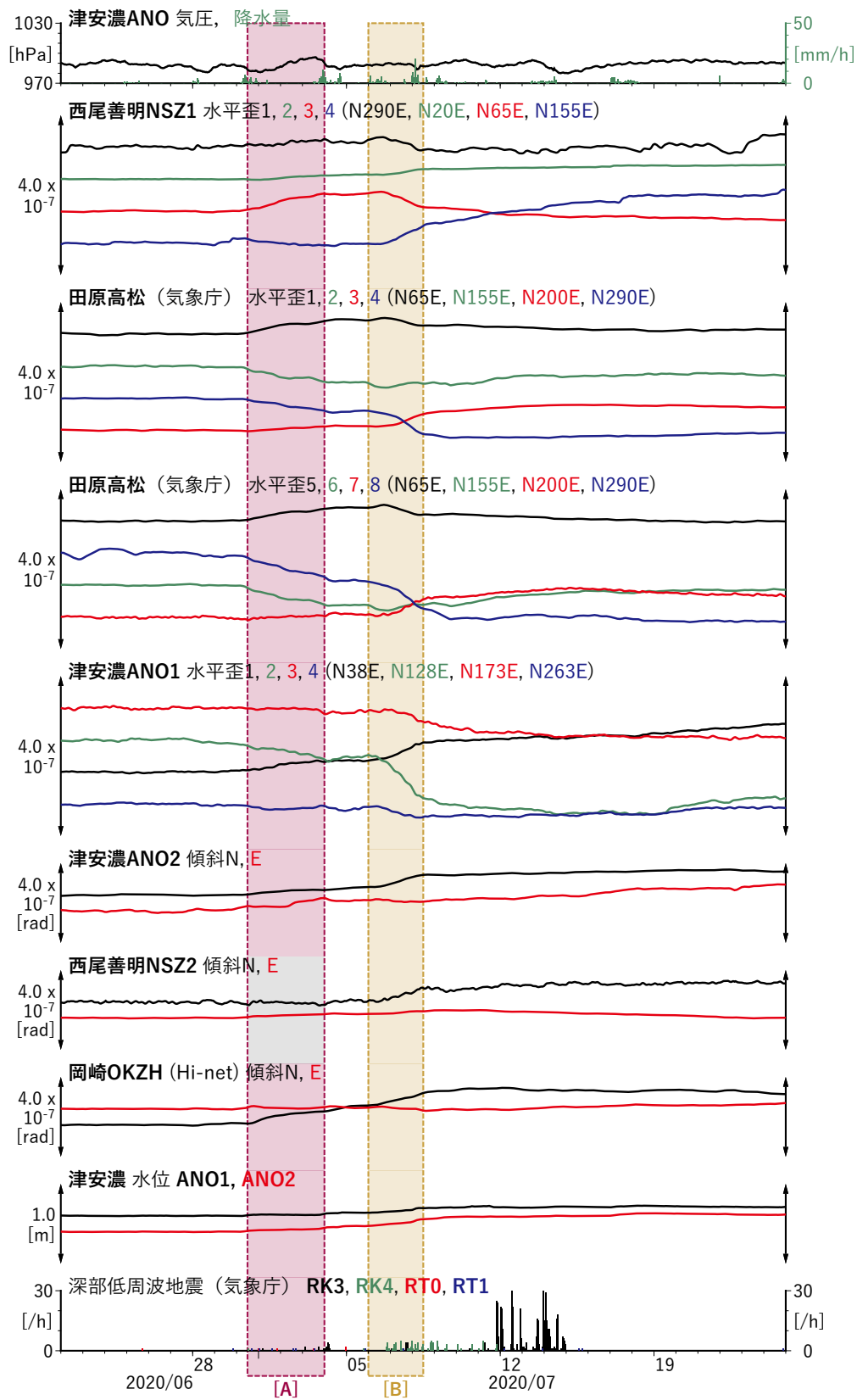
第 11 図 紀伊半島から東海地方における歪・傾斜の観測結果と深部低周波地震の検出数 (2020/06/22 ~ 2020/07/25)。
