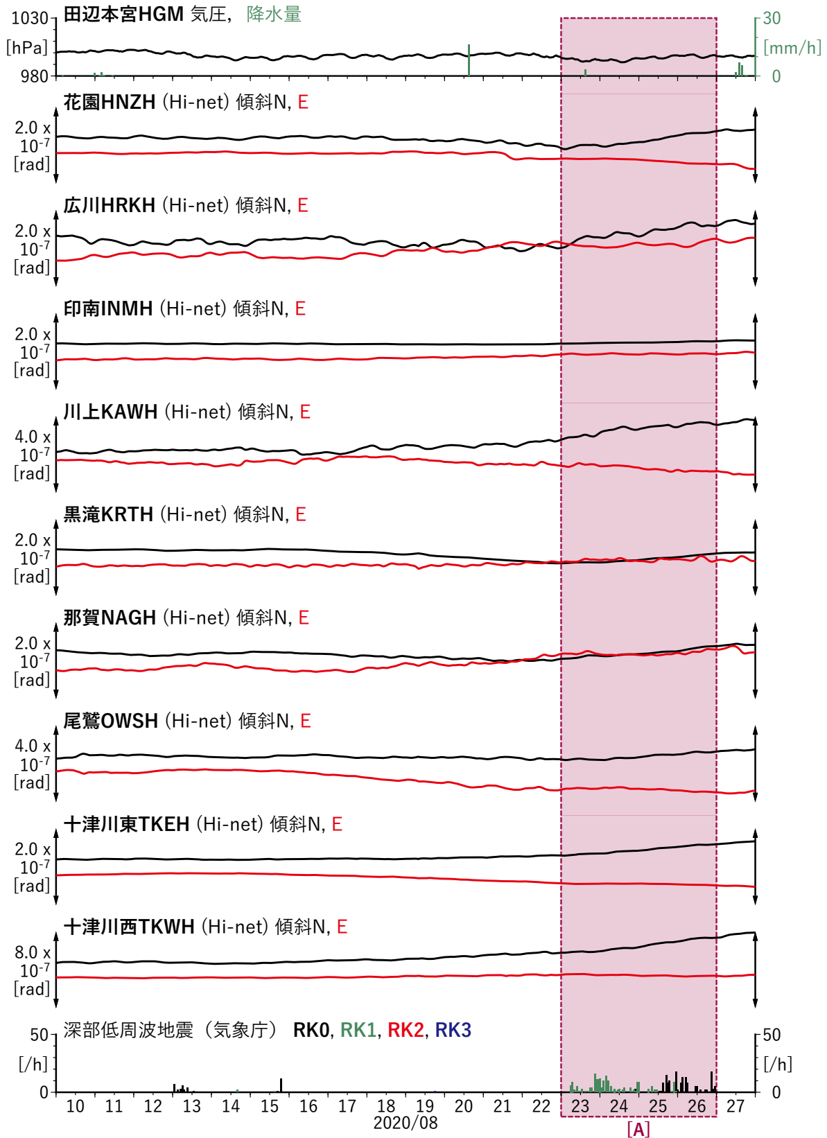
第 29 図 紀伊半島における歪・傾斜の観測結果と深部低周波地震の検出数 (2) (2020/08/10 ~ 2020/08/28).
