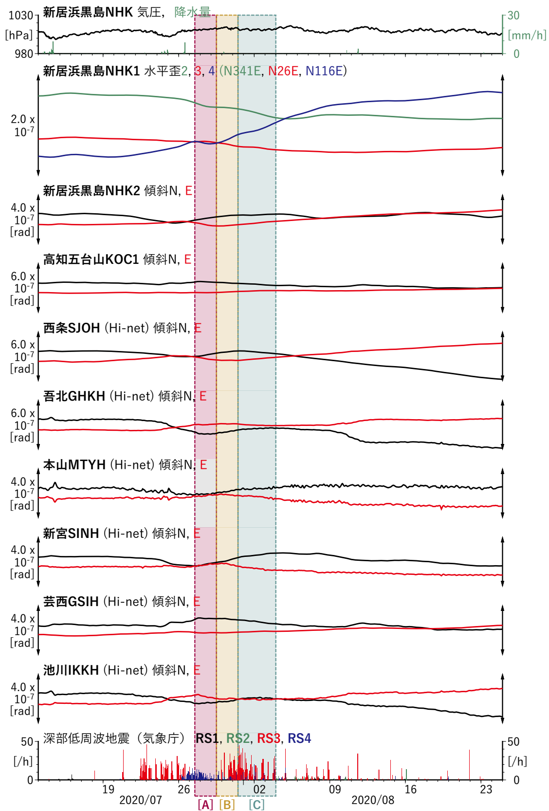
第 16 図 四国地方における歪・傾斜の観測結果と深部低周波地震の検出数 (2) (2020/07/13 ~ 2020/08/25).
