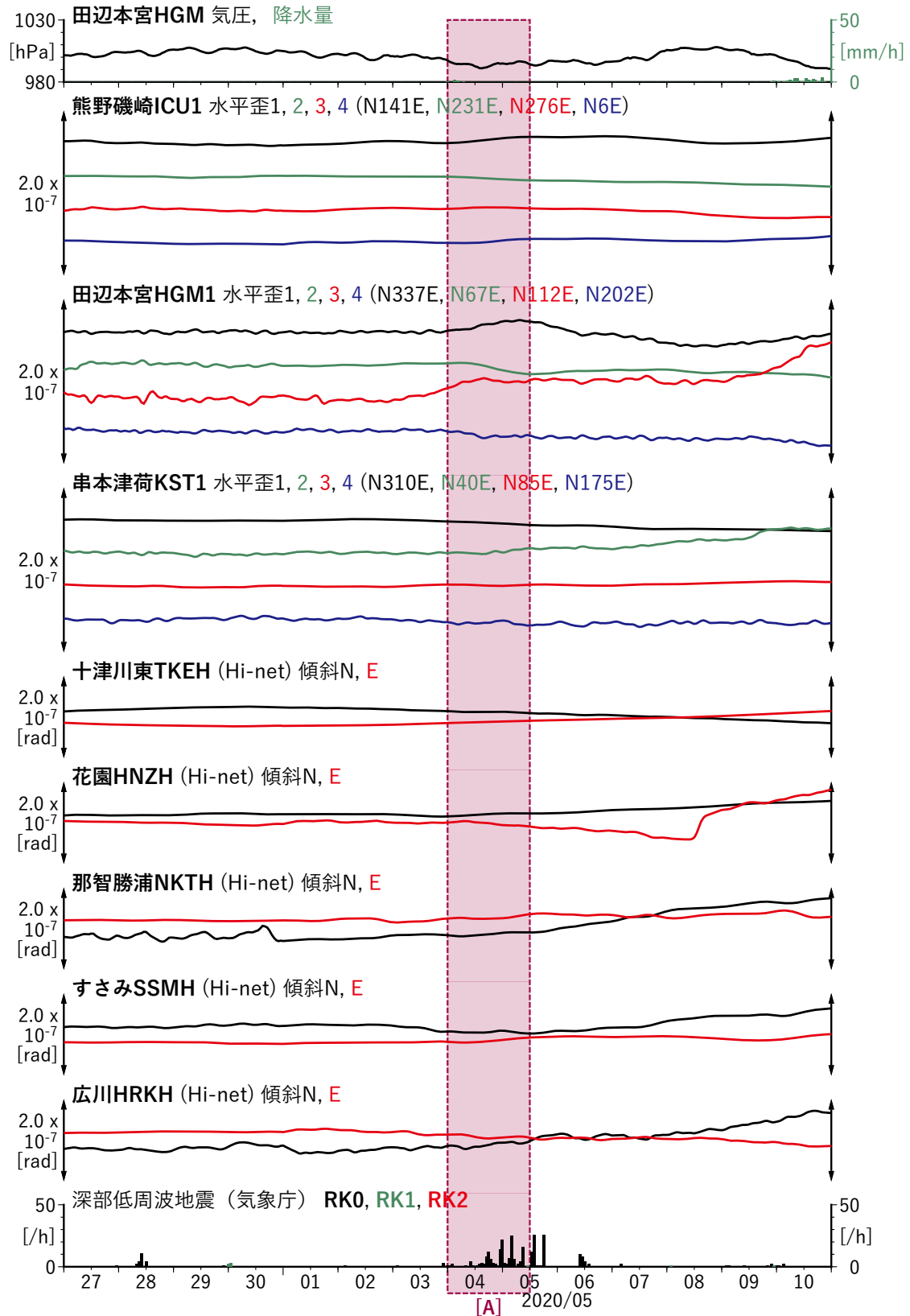
第 2 図 紀伊半島における歪・傾斜の観測結果と深部低周波地震の検出数 (2020/04/27 ~ 2020/05/11)。
