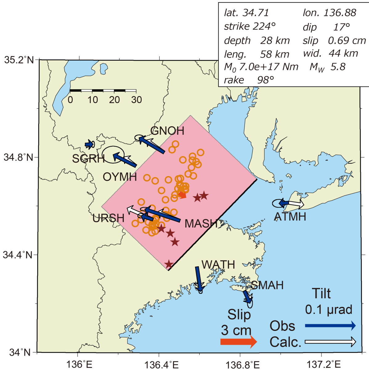
第 5 図 2020 年 10 ～ 11 月紀伊半島北部の SSE の断層モデル。図の見方は第 3 図と同じ。
