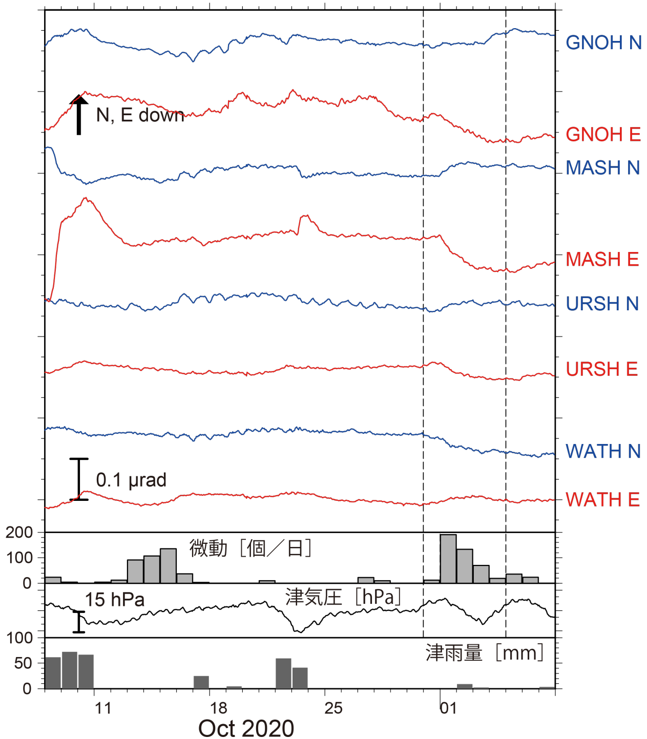
第 4 図 2020 年 10 月 8 日～11 月 7 日までの傾斜時系列. 図の見方は第 2 図と同様. 観測点位置は第 5 図に示した. 10 月 31 日～11 月 4 日の傾斜変化量を SSE によるものと仮定した. 紀伊半島北部における微動活動度・気象庁津観測点での気圧変化および雨量をあわせて表示した.
