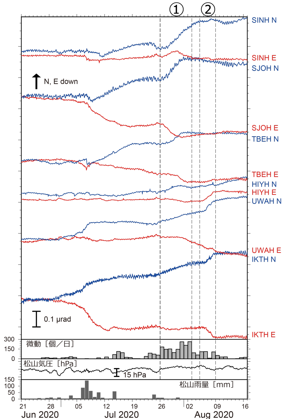
第 2 図 2020 年 6 月 21 日から 8 月 16 日までの傾斜時系列．観測点位置は第 3 図に示した．記録は上方向への変化が北・東下がりの傾斜変動を表す．気圧応答・潮汐成分を BAYTAP-G4) により除去し，直線トレンドを補正した後の記録を示した．期間①②の傾斜変化量を SSE によるものと仮定した．四国中西部での微動活動度・気象庁宇和島観測点での気圧変化および雨量をあわせて表示した．
