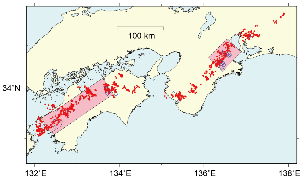
第 1 図 2020 年 5 月 1 日～2020 年 11 月 4 日の期間に検知された短期的 SSE (ピンク矩形). 同期間に発生した深部低周波微動 (赤点) 及び VLFE の震央 (青菱形) を重ねて表示した.
