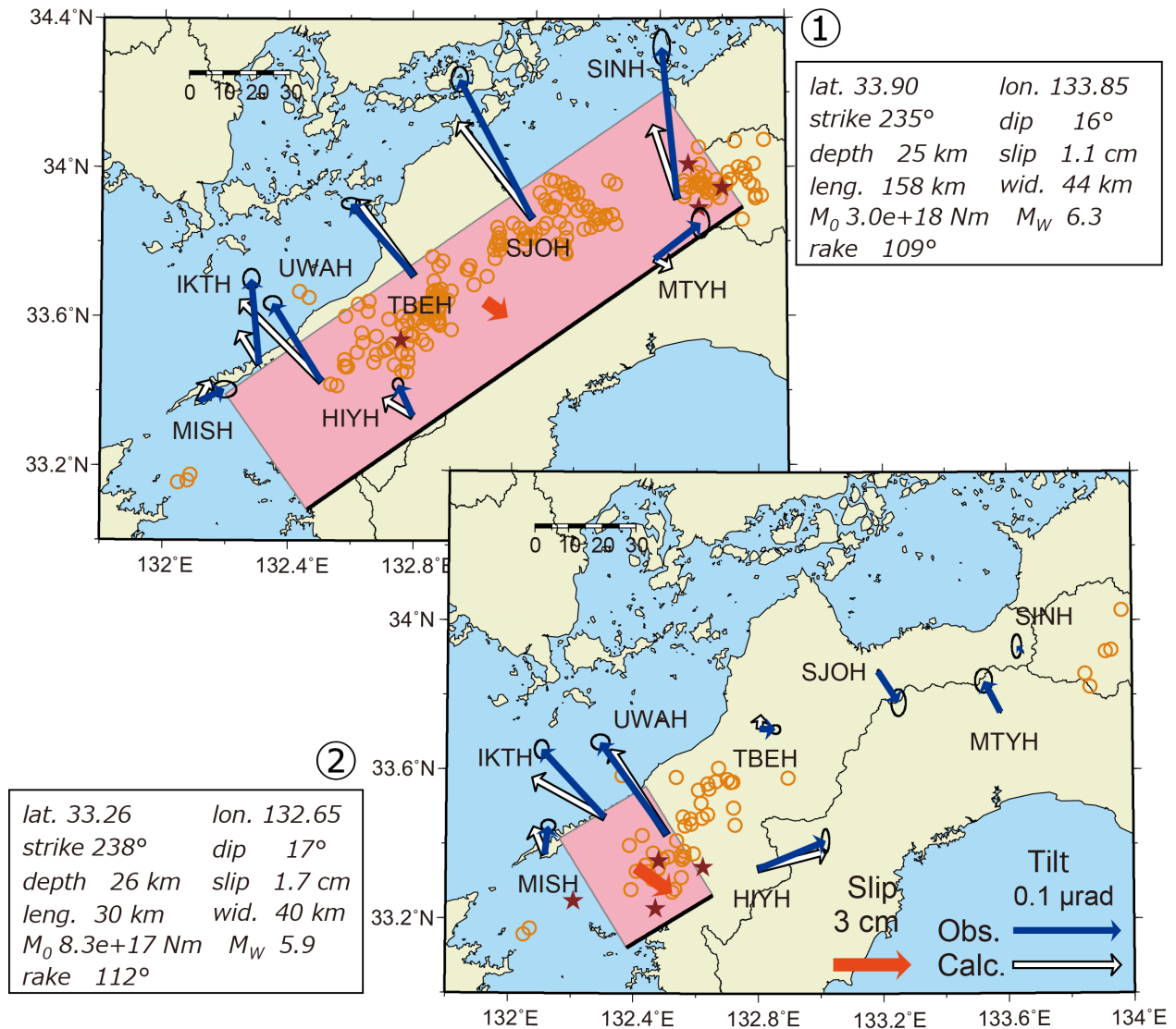
第 3 図 2020 年 10 ～ 11 月四国中西部の短期的 SSE の断層モデル。第 2 図の破線で示された期間に観測された傾斜変化ベクトル（青矢印）・このデータから推定された SSE の断層モデル（赤矩形・矢印）・モデルから計算される傾斜変化ベクトル（白抜き矢印）を示す。同じ期間の微動と深部超低周波地震の震央を橙円と茶星印で示した。
