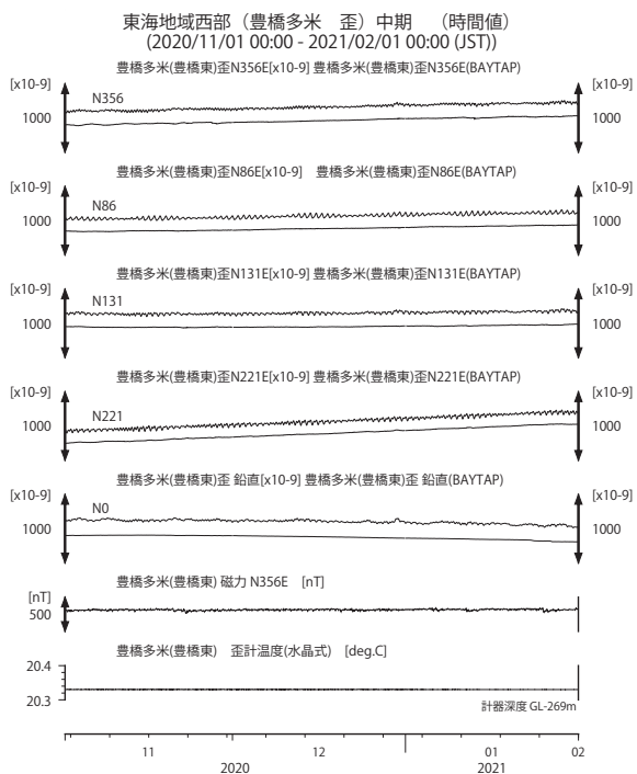
第 9 図 東海地域西部(豊橋多米)の歪等の 観測結果(2020 年 11 月~2021 年 1 月) Fig. 9 Observed strain and others at the Toyohashi- tame observation site in the western Tokai district from Nov. 2020 to Jan. 2021.
