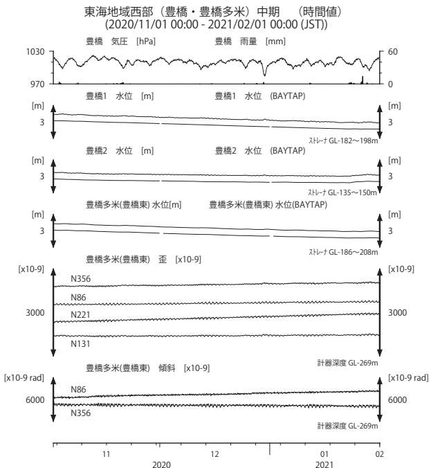
第 7 図 東海地域西部(豊橋・豊橋多米)の地下水等の観測結果(2020 年 11 月～2021 年 1 月)
