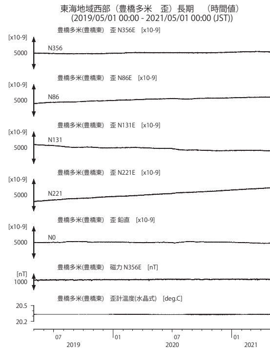
第 18 図 東海地域西部（豊橋多米）の歪等の観測結果 (2019 年 5 月～2021 年 4 月)
