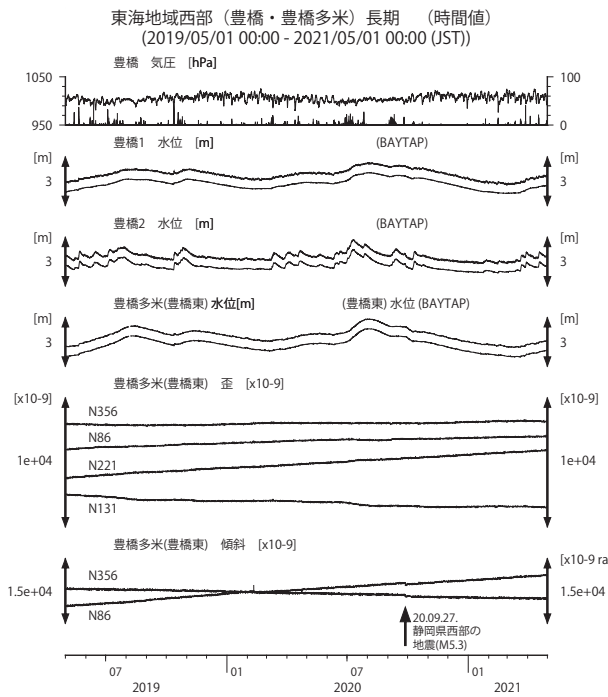
第 17 図 東海地域西部（豊橋・豊橋多米）の地下水等の観測結果 (2019 年 5 月～2021 年 4 月)
