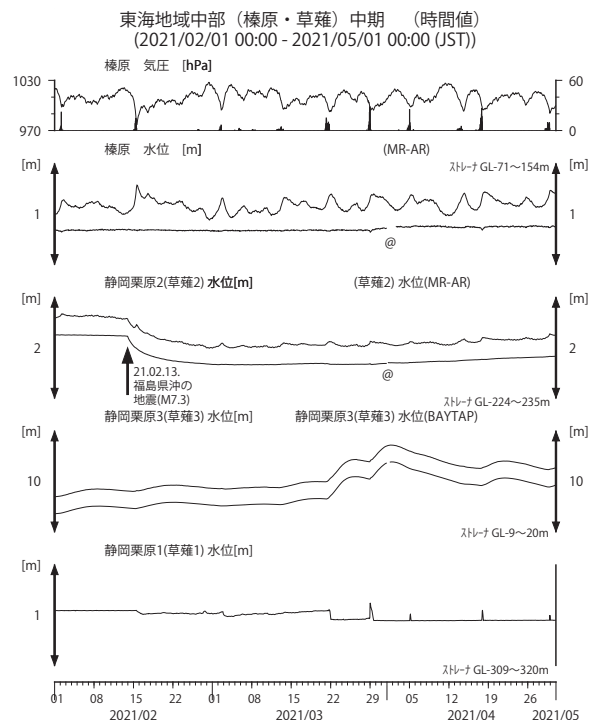
第 4 図 東海地域中部の地下水等の観測結果 (2021 年 2 月～2021 年 4 月)
