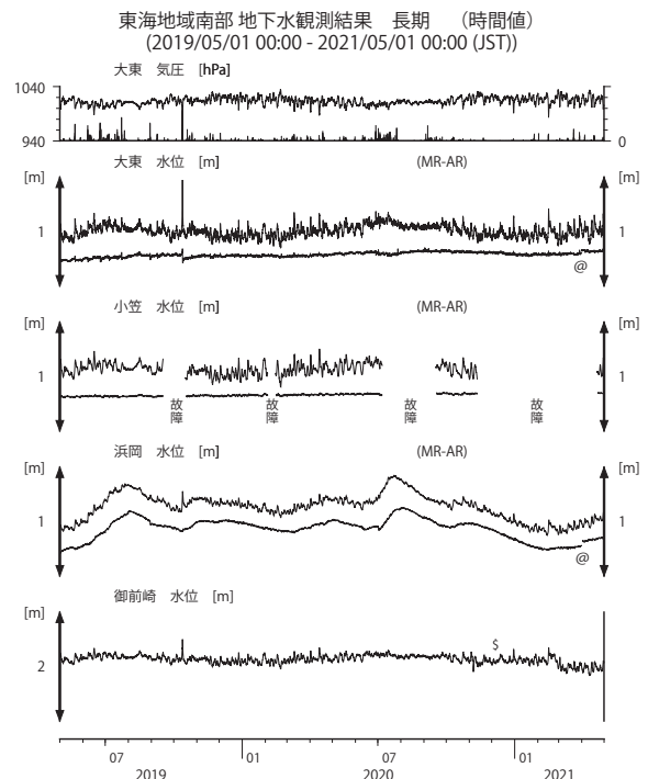
第 16 図 東海地域南部の地下水等の観測結果 (2019 年 5 月～2021 年 4 月)
