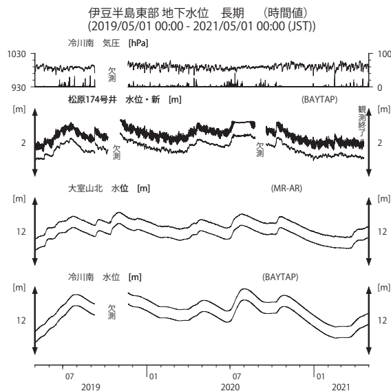
第 19 図 伊豆半島東部の地下水等の観測結果 (2019 年 5 月～2021 年 4 月)
