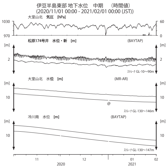
第 11 図 伊豆半島東部の地下水等の観測結果 (2020 年 11 月～2021 年 1 月) Fig. 11 Observed groundwater levels and others in the eastern Izu peninsula district from Nov. 2020 to Jan. 2021.
