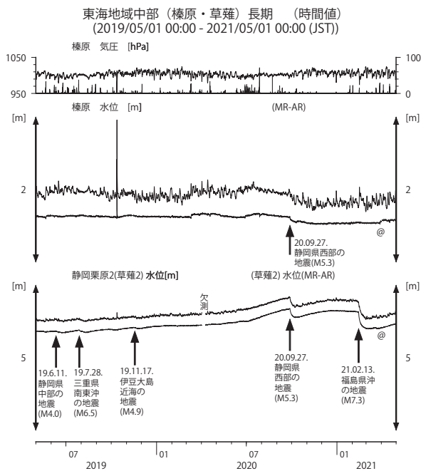
第 15 図 東海地域中部の地下水等の観測結果 (2019 年 5 月～2021 年 4 月)
