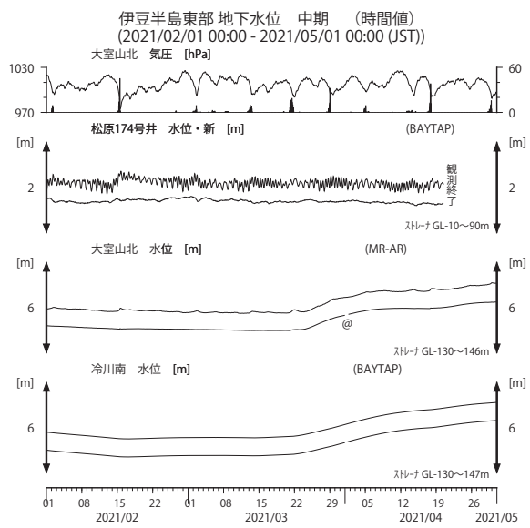
第 12 図 伊豆半島東部の地下水等の観測結果 (2021 年 2 月～2021 年 4 月) Fig. 12 Observed groundwater levels and others in the eastern Izu peninsula district from Feb. 2021 to Apr. 2021.
