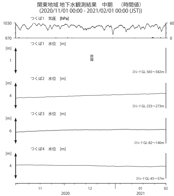
第 13 図 関東地域の地下水等の観測結果 (2020 年 11 月～2021 年 1 月)
