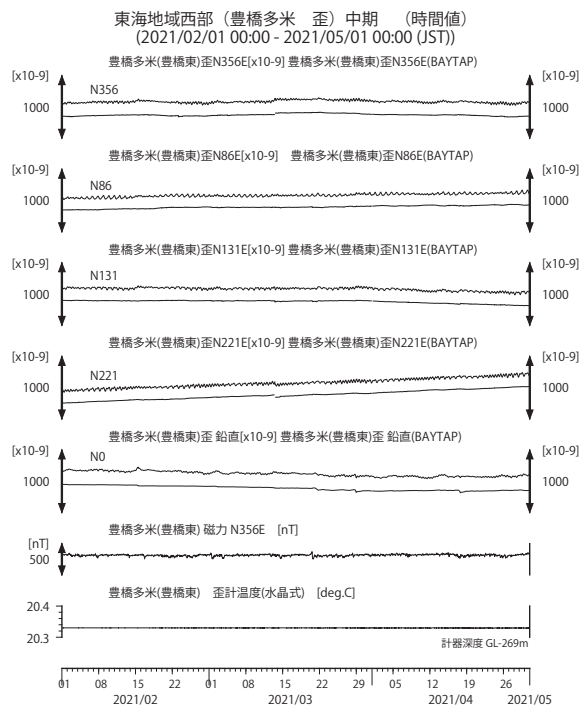
第 10 図 東海地域西部(豊橋多米)の歪等の 観測結果(2021 年 2 月~2021 年 4 月) Fig. 10 Observed strain and others at the Toyohashi- tame observation site in the western Tokai district from Feb. 2021 to Apr. 2021.
