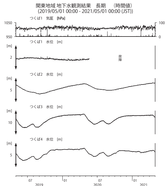
第 20 図 関東地域の地下水等の観測結果 (2019 年 5 月～2021 年 4 月)
