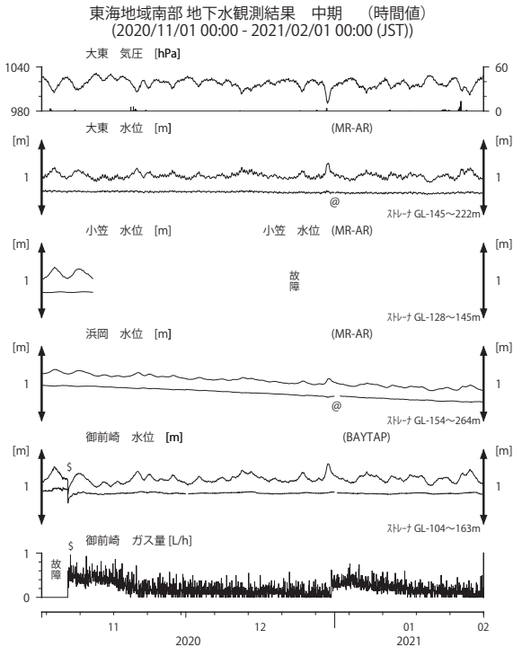
第 5 図 東海地域南部の地下水等の観測結果 (2020 年 11 月～2021 年 1 月)
