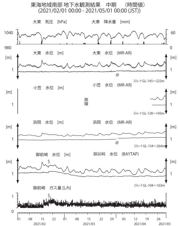
第 6 図 東海地域南部の地下水等の観測結果 (2021 年 2 月～2021 年 4 月)
