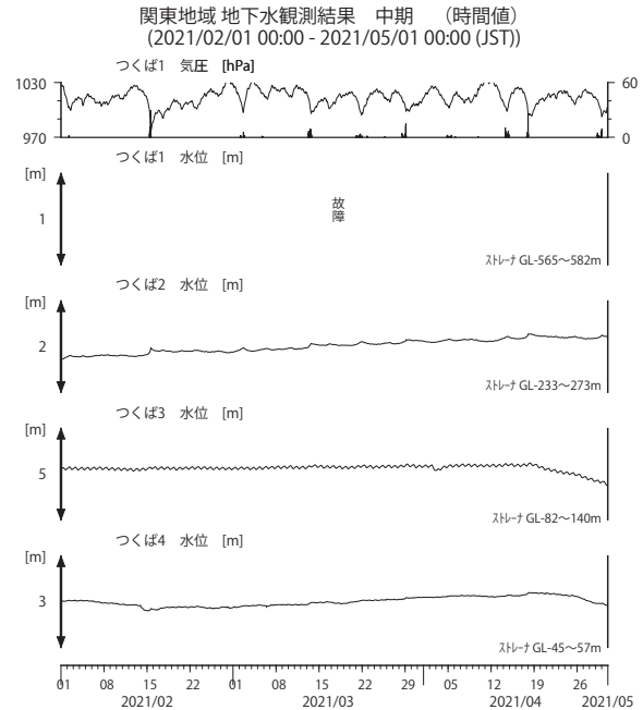
第 14 図 関東地域の地下水等の観測結果 (2021 年 2 月～2021 年 4 月)
