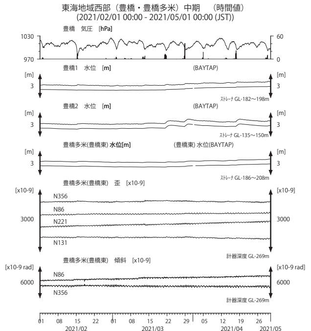
第 8 図 東海地域西部(豊橋・豊橋多米)の地下水等の観測結果(2021 年 2 月～2021 年 4 月)
