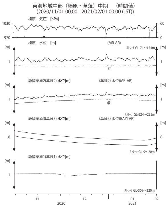
第 3 図 東海地域中部の地下水等の観測結果 (2020 年 11 月～2021 年 1 月)
