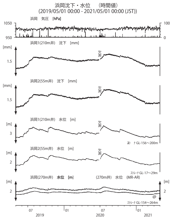
第 21 図 浜岡における沈下等の観測結果 (2019 年 5 月～2021 年 4 月)
