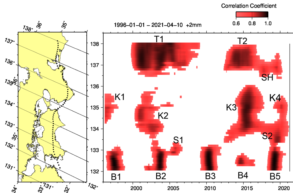
第 1 図 長期的スロースリップ客観検知図（1996 年から 2021 年 4 月）
