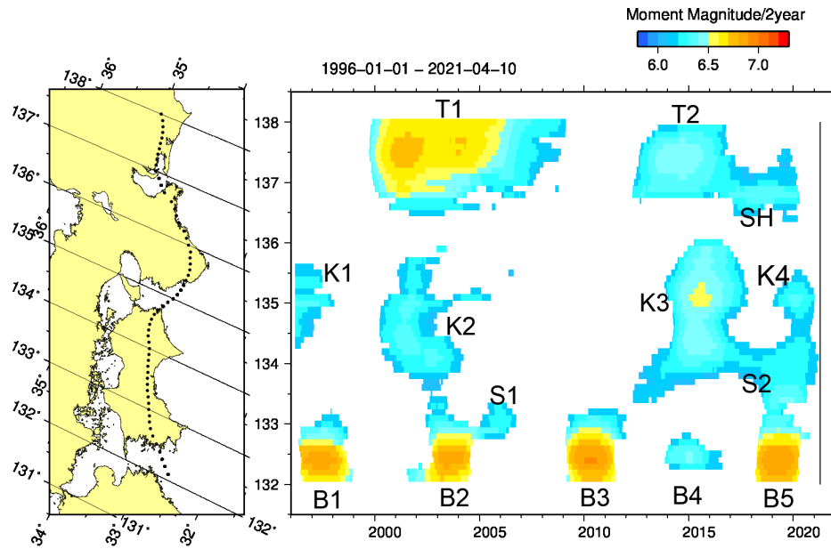
第 2 図 期的スロースリップの規模分布（1996 年から 2021 年 4 月）
