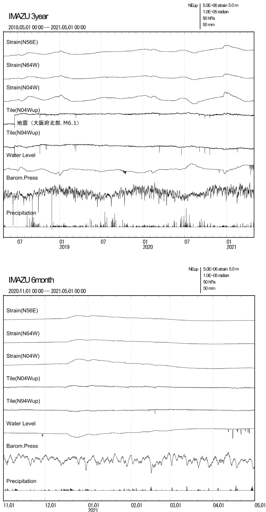
第 2 図 今津観測点における(上)2018 年 5 月～2021 年 4 月, (下)2020 年 11 月～2021 年 4 月のひずみ・傾斜変化(時間値)。毎年冬のひずみ・水位変化は、観測点付近の融雪のための地下水汲み上げに伴うもの。
