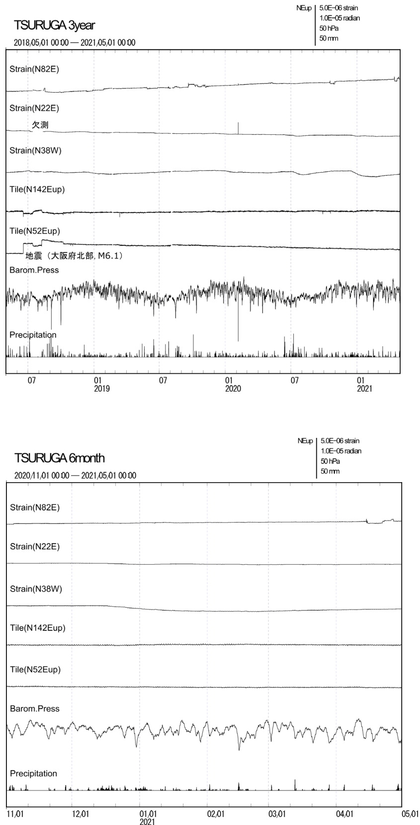
第 3 図 敦賀観測点における(上)2018 年 5 月～2021 年 4 月, (下)2020 年 11 月～2021 年 4 月のひずみ・傾斜変化(時間値)。
