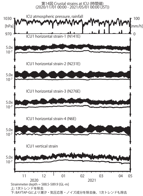
第 14 図 ICU における歪観測結果 (2020 年 11 月～2021 年 4 月) Fig. 14 Observed strains at the ICU observation site from November 2020 to April 2021.
