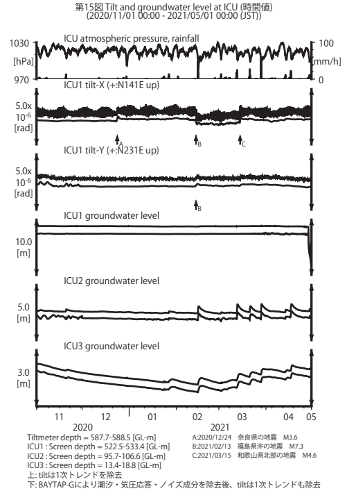
第 15 図 ICU における傾斜・地下水位観測結果 (2020 年 11 月～2021 年 4 月) Fig. 15 Observed tilts and groundwater levels at the ICU observation site from November 2020 to April 2021.
