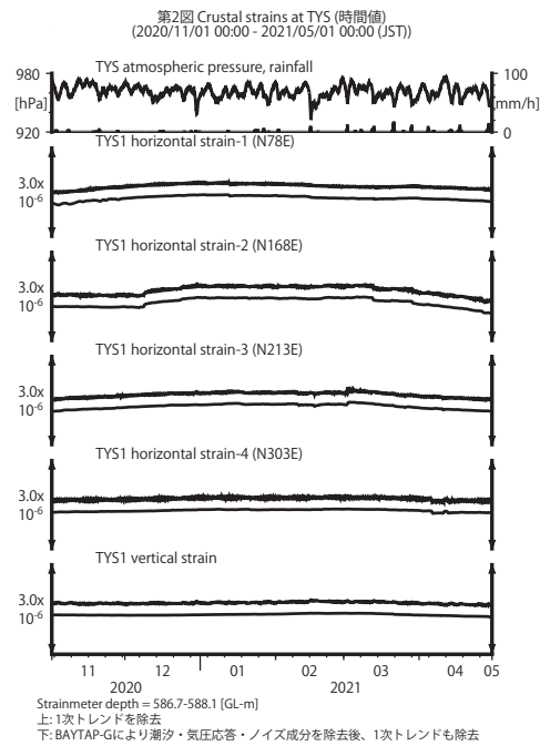
第 2 図 TYS における歪観測結果 (2020 年 11 月～2021 年 4 月) Fig. 2 Observed strains at the TYS observation site from November 2020 to April 2021.
