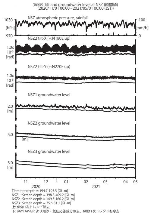
第 5 図 NSZ における傾斜・地下水位観測結果 (2020 年 11 月～2021 年 4 月) Fig. 5 Observed tilts and groundwater levels at the NSZ observation site from November 2020 to April 2021.
