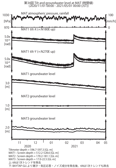
第 34 図 MAT における傾斜・地下水位観測結果 (2020 年 11 月～2021 年 4 月)
