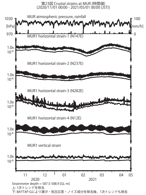
第 23 図 MUR における歪観測結果 (2020 年 11 月～2021 年 4 月)
