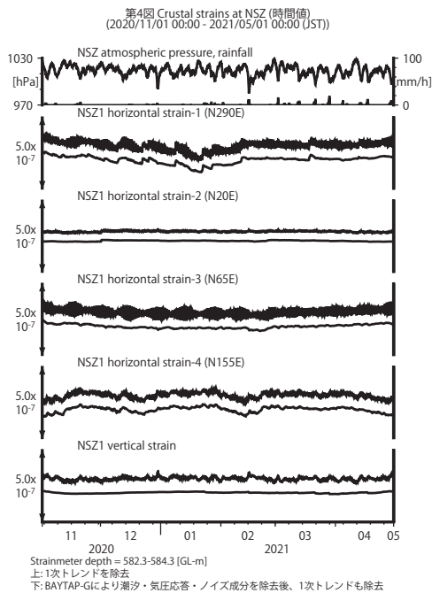
第 4 図 NSZ における歪観測結果 (2020 年 11 月～2021 年 4 月) Fig. 4 Observed strains at the NSZ observation site from November 2020 to April 2021.
