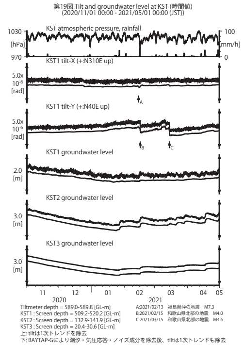
第 19 図 KST における傾斜・地下水位観測結果 (2020 年 11 月～2021 年 4 月) Fig. 19 Observed tilts and groundwater levels at the KST observation site from November 2020 to April 2021.
