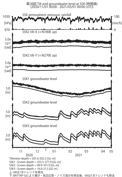
第 28 図 SSK における傾斜・地下水位観測結果 (2020 年 11 月～2021 年 4 月) Fig. 28 Observed tilts and groundwater levels at the SSK observation site from November 2020 to April 2021.
