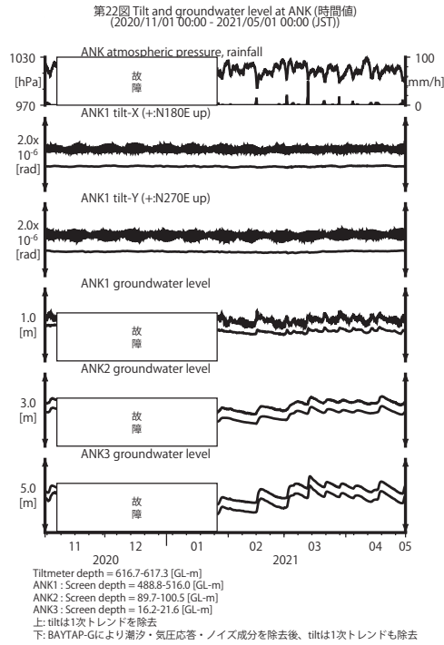
第 22 図 ANK における傾斜・地下水位観測結果 (2020 年 11 月～2021 年 4 月)
