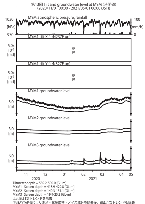
第 13 図 MYM における傾斜・地下水位観測結果 (2020 年 11 月～2021 年 4 月)
