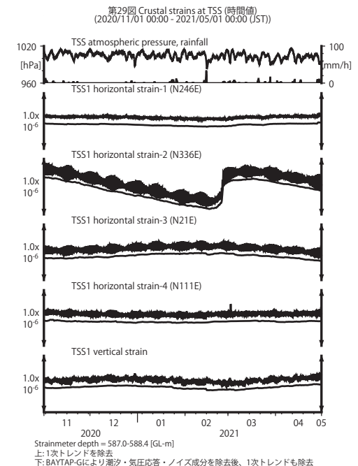
第 29 図 TSS における歪観測結果 (2020 年 11 月～2021 年 4 月) Fig. 29 Observed strains at the TSS observation site from November 2020 to April 2021.
