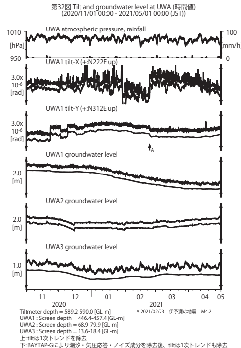
第 32 図 UWA における傾斜・地下水位観測結果 (2020 年 11 月～2021 年 4 月)
