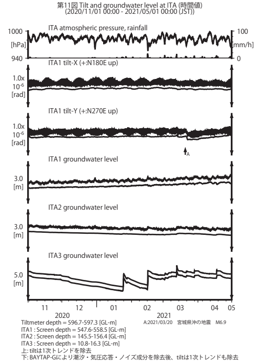
第 11 図 ITA における傾斜・地下水位観測結果 (2020 年 11 月～2021 年 4 月) Fig. 11 Observed tilts and groundwater levels at the ITA observation site from November 2020 to April 2021.
