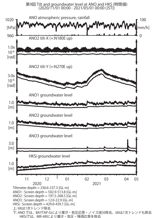
第 9 図 ANO および HKS における傾斜・地下水位観測結果
