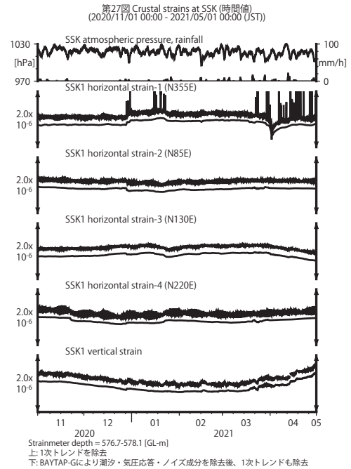
第 27 図 SSK における歪観測結果 (2020 年 11 月～2021 年 4 月) Fig. 27 Observed strains at the SSK observation site from November 2020 to April 2021.
