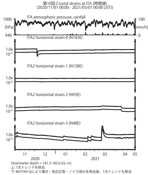
第 10 図 ITA における歪観測結果 (2020 年 11 月～2021 年 4 月) Fig. 10 Observed strains at the ITA observation site from November 2020 to April 2021.
