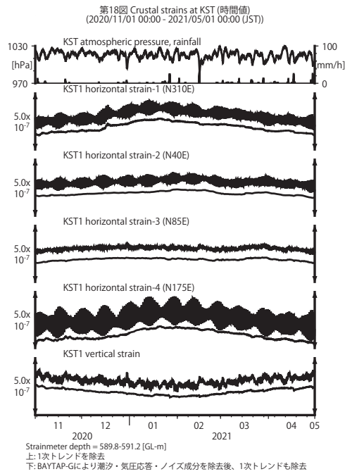
第 18 図 KST における歪観測結果 (2020 年 11 月～2021 年 4 月) Fig. 18 Observed strains at the KST observation site from November 2020 to April 2021.
