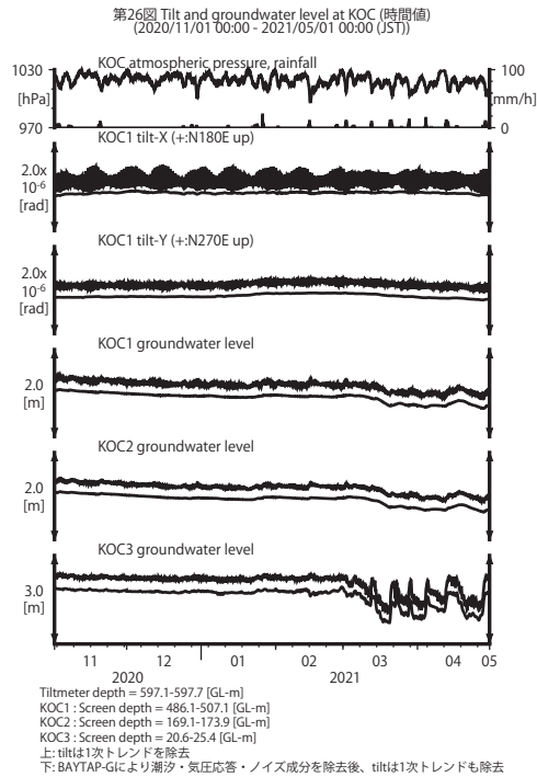
第 26 図 KOC における傾斜・地下水位観測結果 (2020 年 11 月～2021 年 4 月) Fig. 26 Observed tilts and groundwater levels at the KOC observation site from November 2020 to April 2021.
