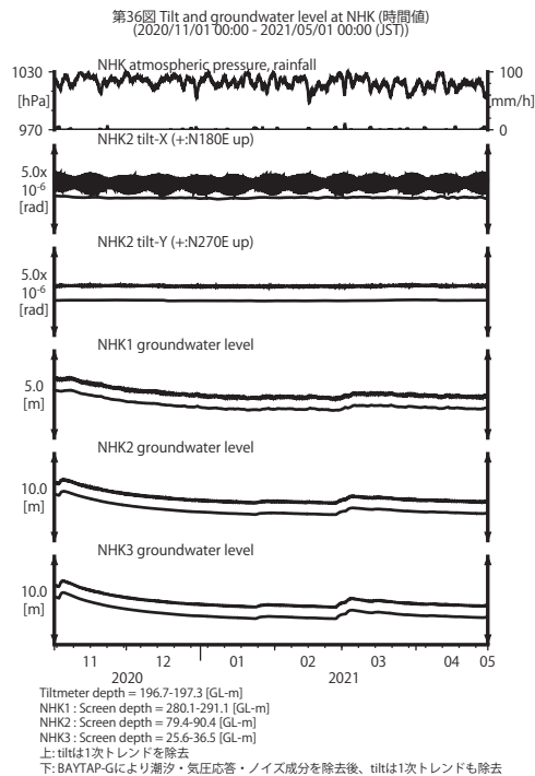
第 36 図 NHK における傾斜・地下水位観測結果 (2020 年 11 月～2021 年 4 月)
