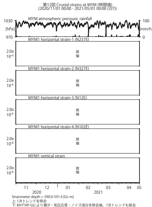
第 12 図 MYM における歪観測結果 (2020 年 11 月～2021 年 4 月) Fig. 12 Observed strains at the MYM observation site from November 2020 to April 2021.
