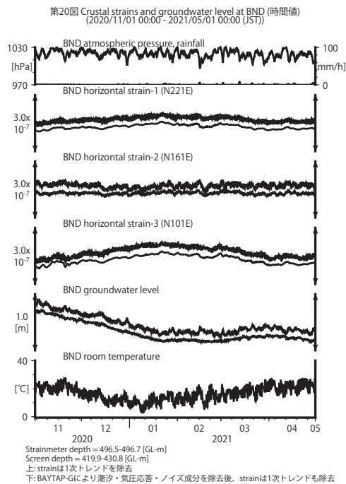
第 20 図 BND における歪・地下水位観測結果 (2020 年 11 月～2021 年 4 月) Fig. 20 Observed strains and groundwater level at the BND observation site from November 2020 to April 2021.
