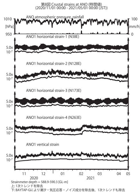
第 8 図 ANO における歪観測結果
