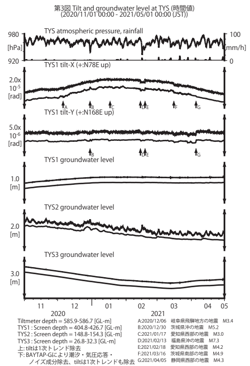
第 3 図 TYS における傾斜・地下水位観測結果 (2020 年 11 月～2021 年 4 月) Fig. 3 Observed tilts and groundwater levels at the TYS observation site from November 2020 to April 2021.
