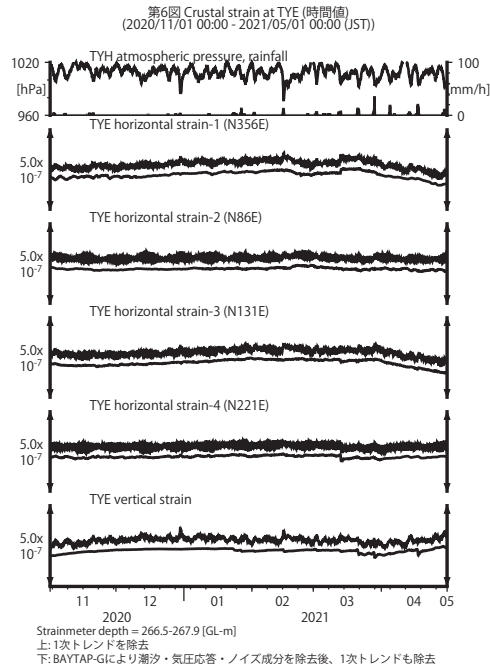
第 6 図 TYE における歪観測結果
