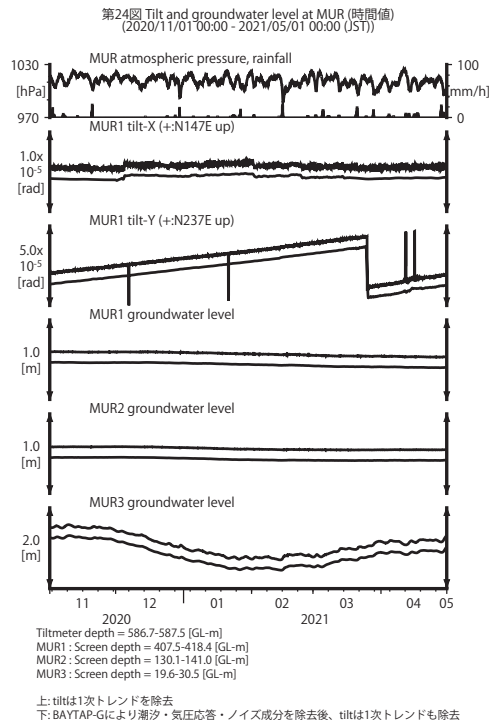
第 24 図 MUR における傾斜・地下水位観測結果 (2020 年 11 月～2021 年 4 月)
