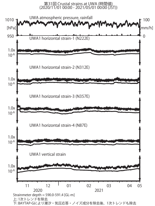
第 31 図 UWA における歪観測結果 (2020 年 11 月～2021 年 4 月)
