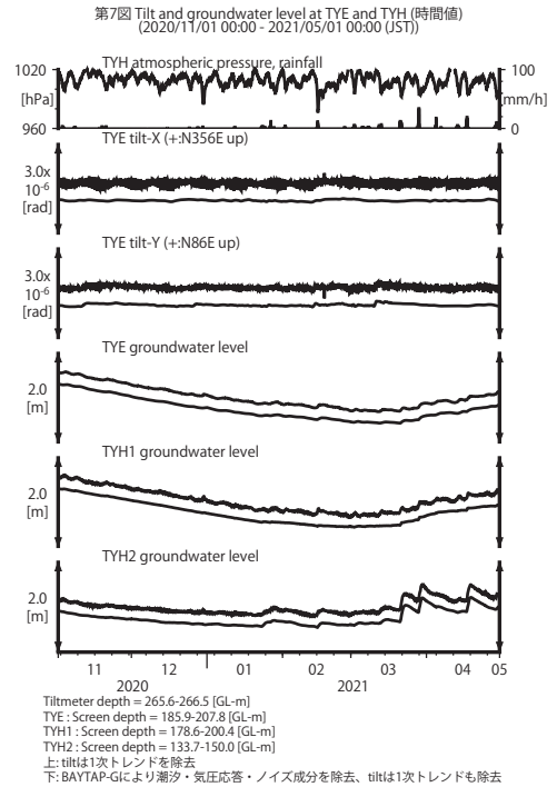
第 7 図 TYE および TYH における傾斜・地下水位観測結果
