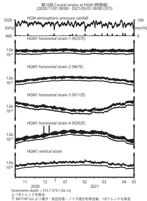
第 16 図 HGM における歪観測結果 (2020 年 11 月～2021 年 4 月) Fig. 16 Observed strains at the HGM observation site from November 2020 to April 2021.
