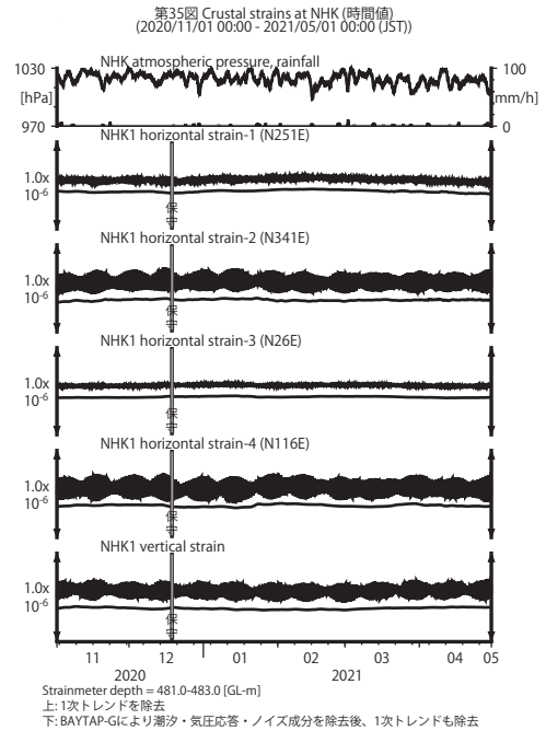
第 35 図 NHK における歪観測結果 (2020 年 11 月～2021 年 4 月)
