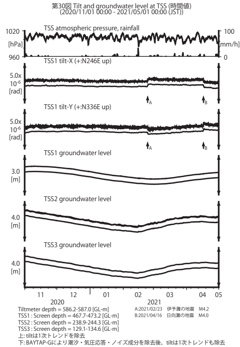
第 30 図 TSS における傾斜・地下水位観測結果 (2020 年 11 月～2021 年 4 月)
