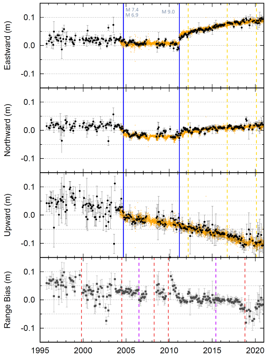
第 2 図 ITRF 2014 の速度を適用した上で求めた下里レーザー不動点の変位（黒丸）及びレンジバイアスの値（1 か月解）並びに GNSS 観測点「SMST」の変位（黄丸、1 日解）。変位量は、解が比較的安定している 2005 年 1 月の局位置解（北緯 33.57769313 度、東経 135.93703761 度、楕円体高 101.644 m）を基準とし、局直交座標系において示している。ITRF 2014 における地震に伴う変位は補正していない。エラーバーは 1\sigma の範囲を示す。青線は、2004 年紀伊半島南東沖地震（M 7.4 及び M 6.9、2004 年 9 月 5 日）及び 2011 年東北地方太平洋沖地震（M 9.0、2011 年 3 月 11 日）の発生日を示す。黄破線、赤破線及び紫破線は、それぞれ GNSS アンテナ・レドーム、SLR 観測装置及び SLR キャリブレーションターゲットの更新日のうち主要なものを示す。
