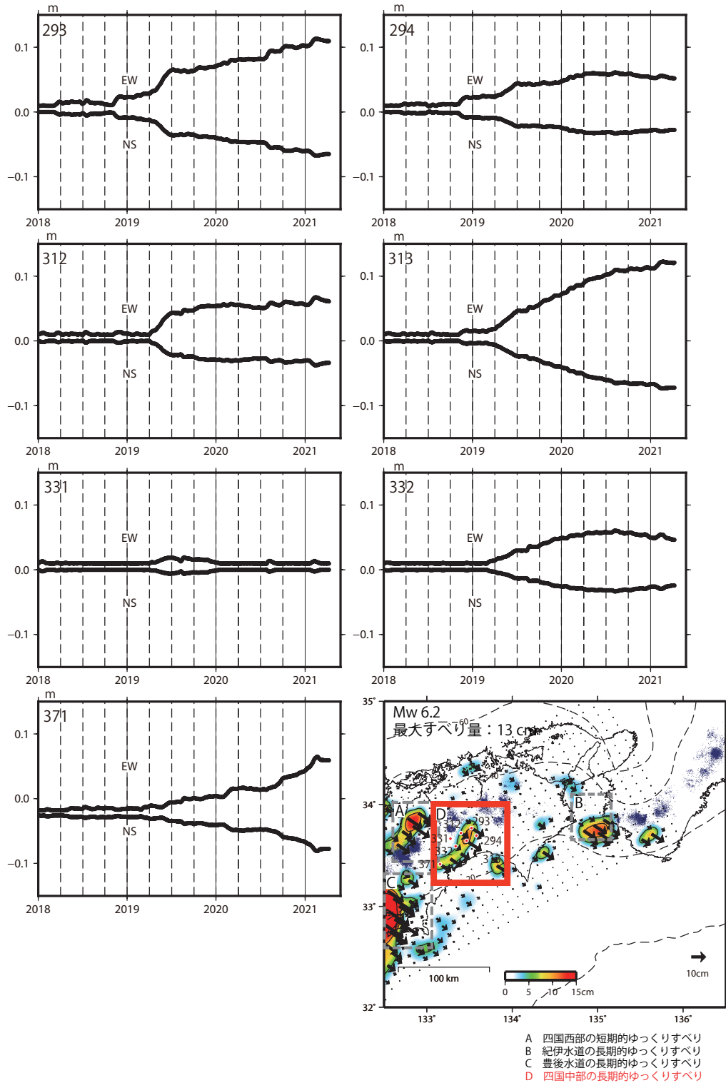
第 7 図 時間依存インバージョンで推定されたプレート間滑りの時間変化
