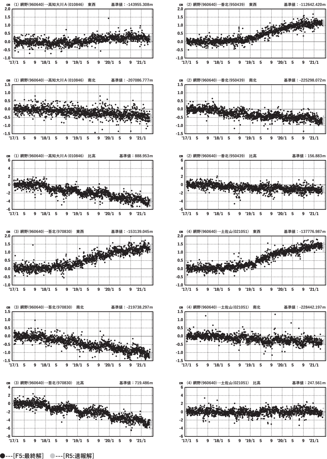
第 3 図 四国中部の GNSS 連続観測時系列
