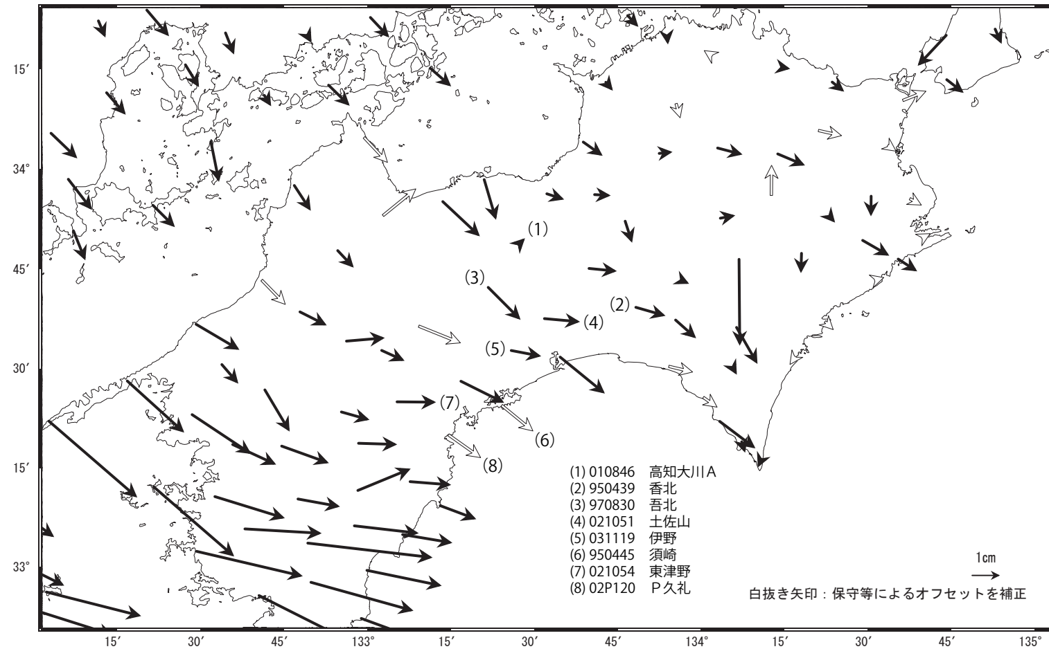
第2図 四国中部の非定常水平地殻変動
