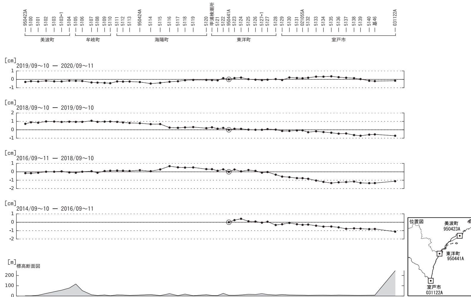
第 10 図 美波町～室戸市間の上下変動
