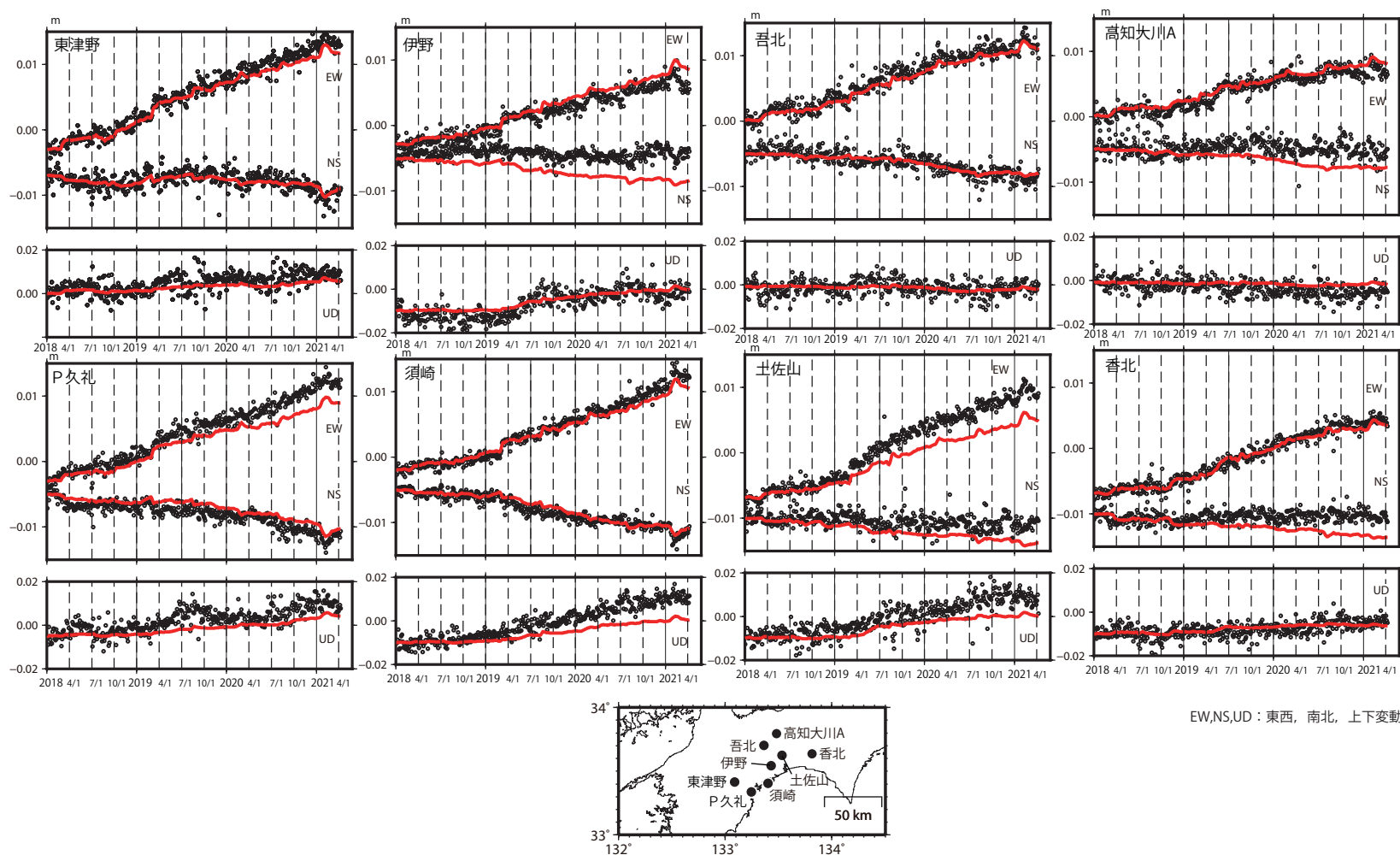
第 6 図 四国中部の観測点の座標時系列(黒丸)と計算値(赤線)
