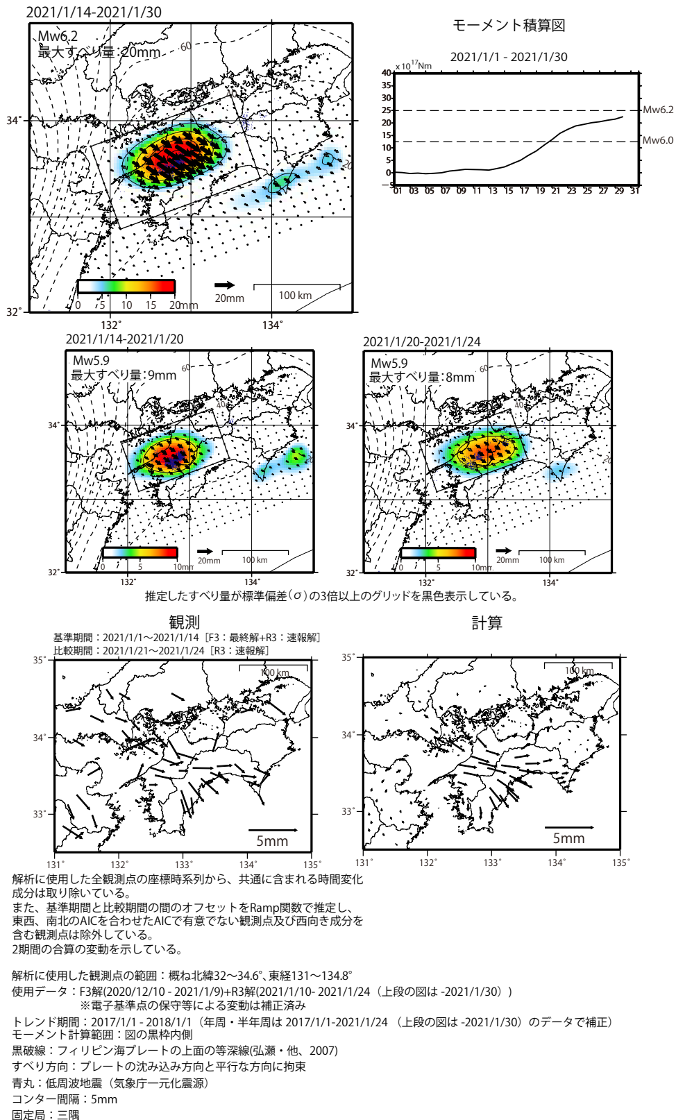
第1図 四国西部の深部低周波微動と同期したスロースリップ
