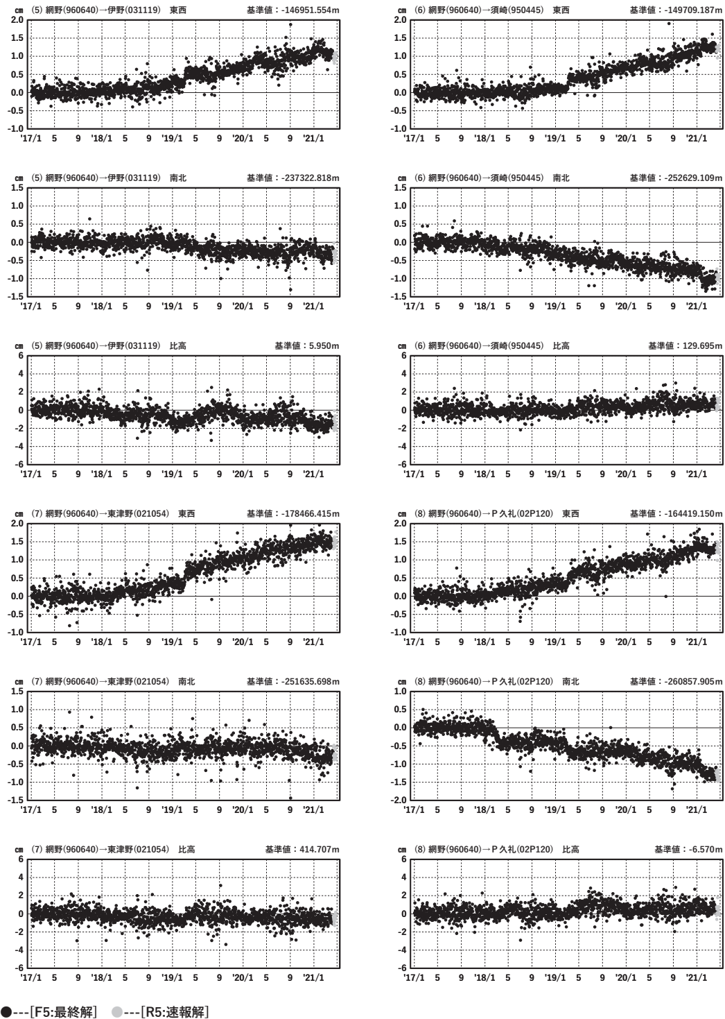
第 4 図 四国中部の GNSS 連続観測時系列
