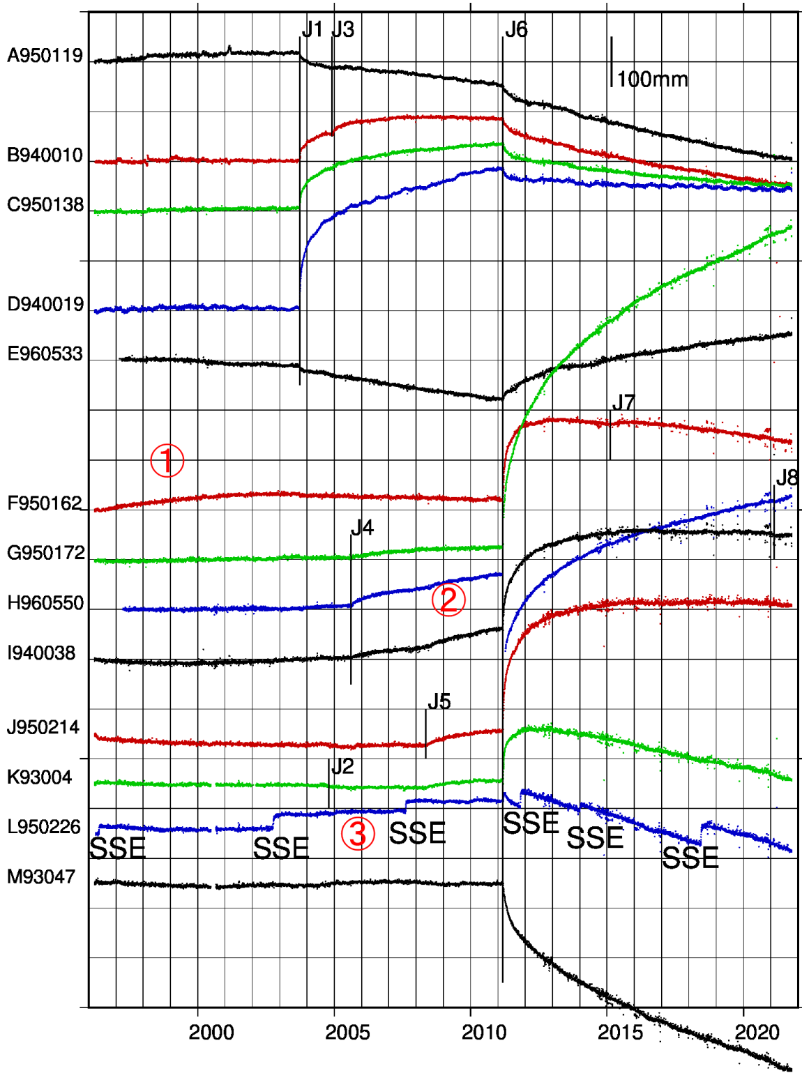
第 2a 図 プレート沈み込み方向の位置変化（東日本；1996 年から 2021 年 10 月） 沈み込みと逆方向が上向き。地点番号は、第 1 図の観測点記号に GEONET 観測点番号を付加したもの。 J1:2003 年十勝沖地震 (M8.0), J2:2004 年新潟県中越地震 (M6.8), J3:2004 年 11 月 29 日釧路沖の地震 (M7.1), J4:2005 年 8 月 16 日宮城県沖の地震 (M7.2), J5:2008 年 5 月 8 日茨城県沖の地震 (M7.0), J6:2011 年東北地 方太平洋沖地震 (M9.0), J7:2015 年 2 月 17 日三陸沖の地震 (M6.9), J8:2021 年 2 月 13 日福島県沖の地震 (M7.3).
