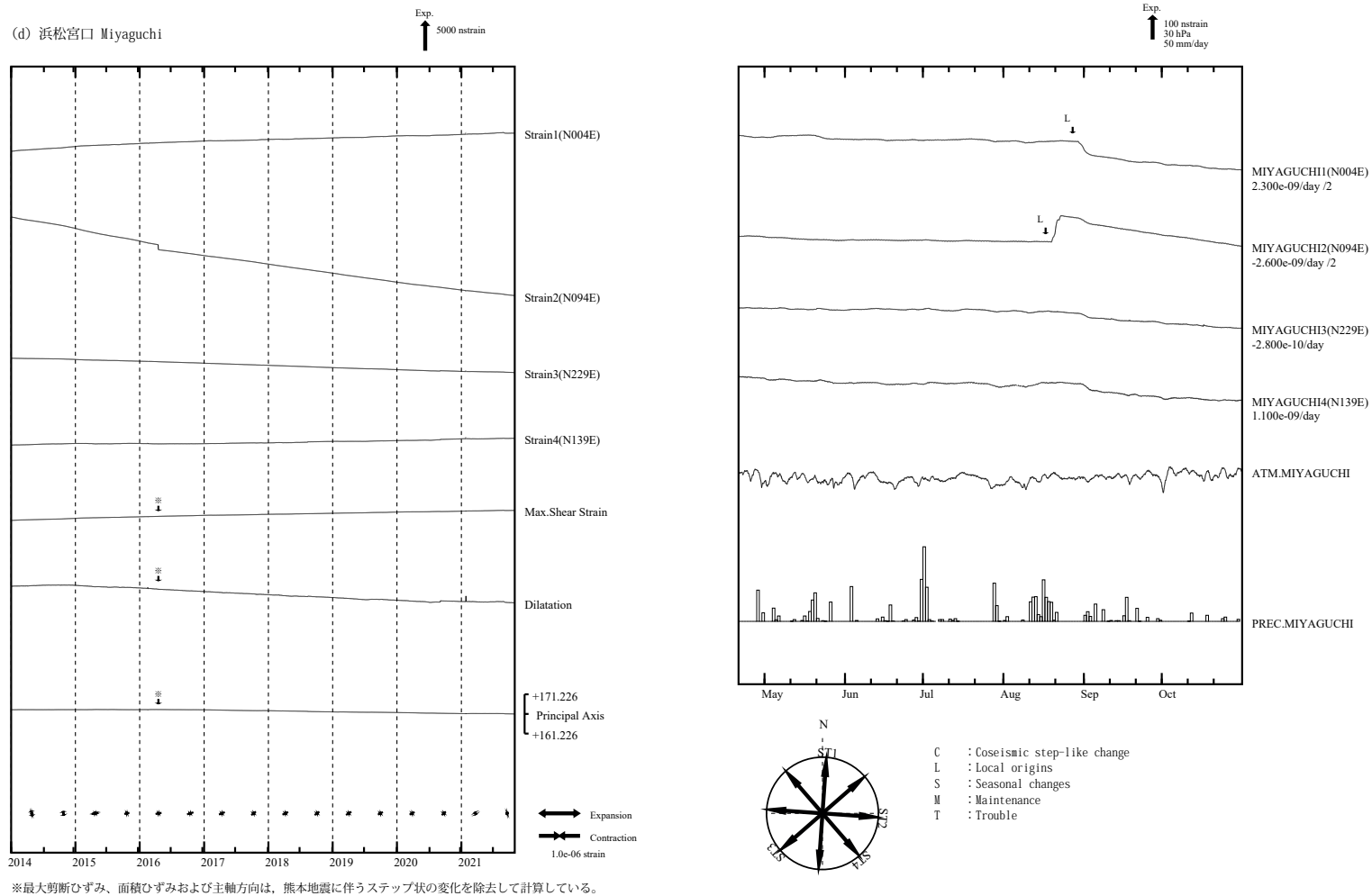
第 4 図 (d) 左：2014 年 1 月以後の多成分ひずみ計変化（日平均値）。主ひずみ・最大せん断ひずみ・面積ひずみは各方向成分から計算されている。 右：2021 年 5 月～10 月の多成分ひずみ計変化（時間値：気圧・潮汐・地磁気・降水補正した値）。各図下部に気圧変化と降水量を示す。ゆっくりすべりが発生している期間を表示するため、4 月 21 日から表示している。
