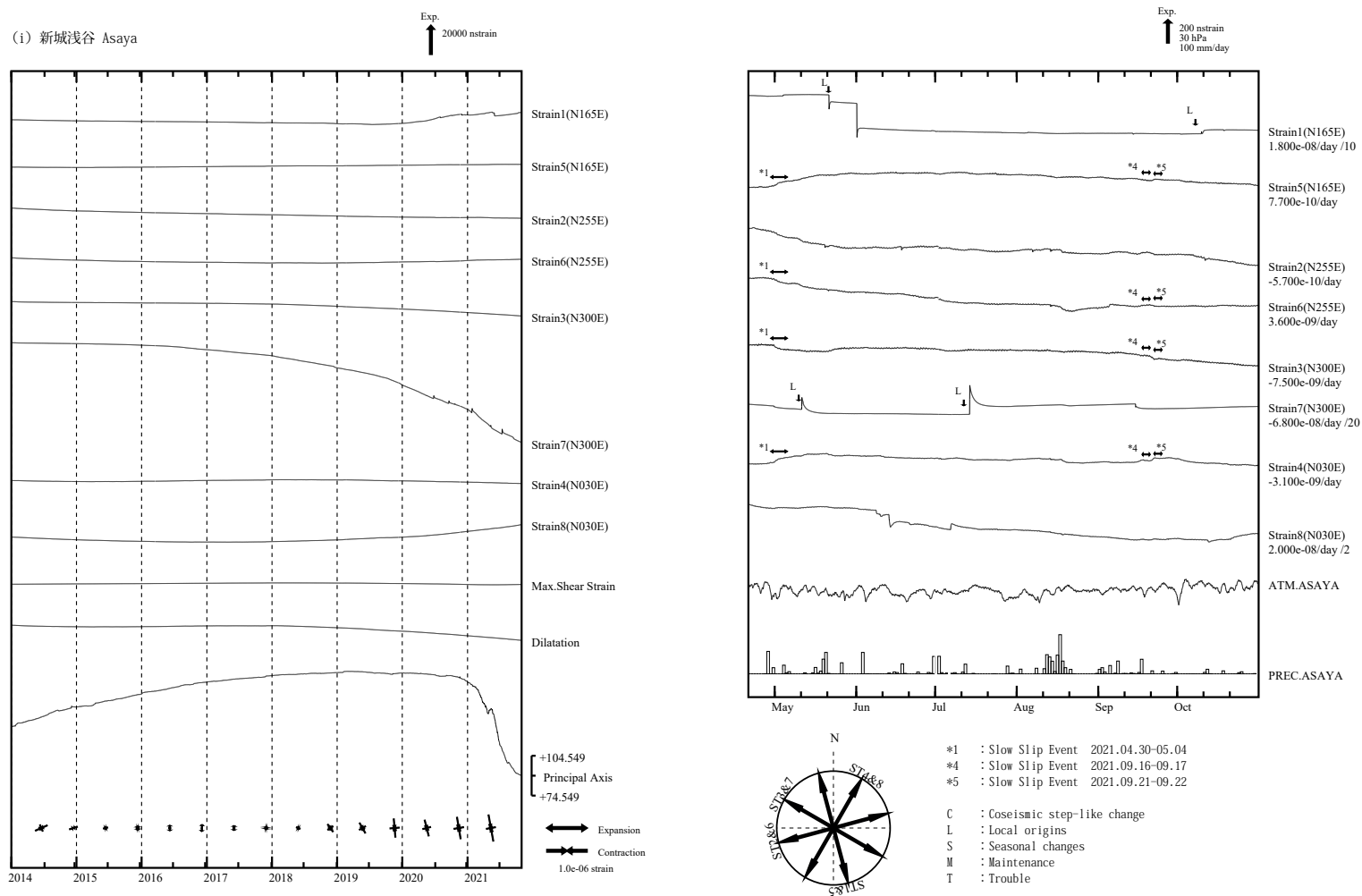
第 4 図 (i) 左：2014 年 1 月以後の多成分ひずみ計変化（日平均値）。主ひずみ・最大せん断ひずみ・面積ひずみは各方向成分から計算されている。 右：2021 年 5 月～10 月の多成分ひずみ計変化（時間値：気圧・潮汐・地磁気・降水補正した値）。各図下部に気圧変化と降水量を示す。ゆっくりすべりが発生している期間を表示するため、4 月 21 日から表示している。
