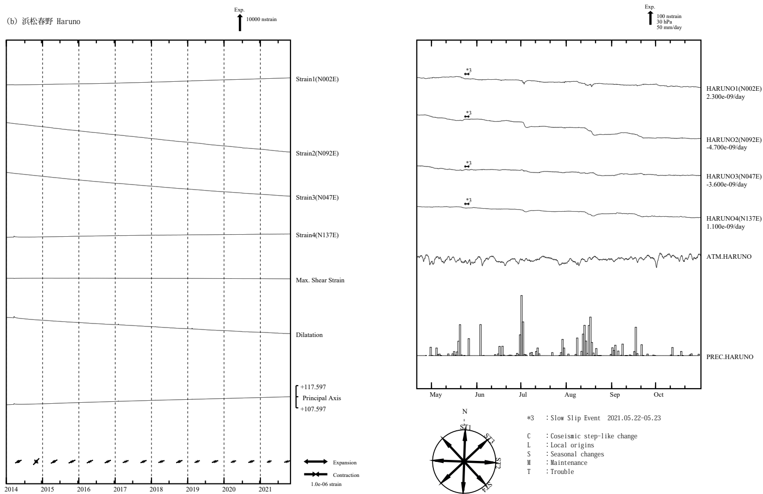
第 4 図 (b) 左：2014 年 1 月以後の多成分ひずみ計変化（日平均値）。主ひずみ・最大せん断ひずみ・面積ひずみは各方向成分から計算されている。 右：2021 年 5 月～10 月の多成分ひずみ計変化（時間値：気圧・潮汐・地磁気・降水補正した値）。各図下部に気圧変化と降水量を示す。ゆっくりすべりが発生している期間を表示するため、4 月 21 日から表示している。 Fig. 4(b) (Left) Strain changes observed by multi-component borehole strainmeters since January 2014 (daily mean values). Principal strain, maximum shear strain and dilatation are calculated with strain values obtained from each component. (Right) Strain changes from May to October 2021 (hourly values where changes due to barometric pressure, tidal effects, geomagnetic effects and rain effects are corrected) observed by multi-component borehole strainmeters. The start date of the figure is set to April 21 to include the period of slow slip event.
