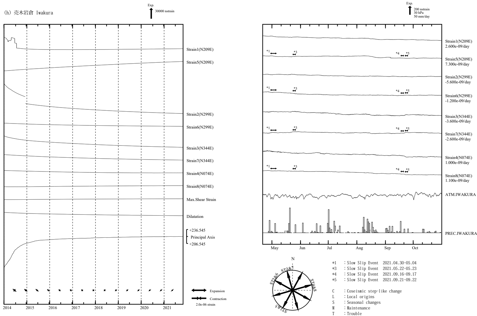
第 4 図 (h) 左：2014 年 1 月以後の多成分ひずみ計変化（日平均値）。主ひずみ・最大せん断ひずみ・面積ひずみは各方向成分から計算されている。 右：2021 年 5 月～10 月の多成分ひずみ計変化（時間値：気圧・潮汐・地磁気・降水補正した値）。各図下部に気圧変化と降水量を示す。ゆっくりすべりが発生している期間を表示するため、4 月 21 日から表示している。
