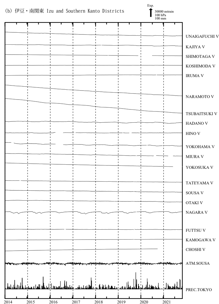
第 2 図 (a), (b) 2014 年 1 月以後の東海・伊豆・南関東地域における区域別体積ひずみ (V) 及び面積ひずみ (S) の変化 (日平均値)。各図下部に区域を代表する気圧変化と降水量を示す。
