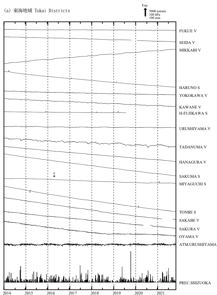
第 2 図 (a), (b) 2014 年 1 月以後の東海・伊豆・南関東地域における区域別体積ひずみ (V) 及び面積ひずみ (S) の変化 (日平均値)。各図下部に区域を代表する気圧変化と降水量を示す。
