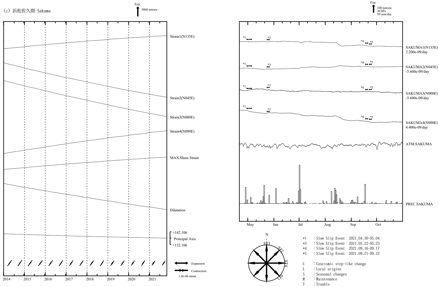
第 4 図 (c) 左：2014 年 1 月以後の多成分ひずみ計変化（日平均値）。主ひずみ・最大せん断ひずみ・面積ひずみは各方向成分から計算されている。 右：2021 年 5 月～10 月の多成分ひずみ計変化（時間値：気圧・潮汐・地磁気・降水補正した値）。各図下部に気圧変化と降水量を示す。ゆっくりすべりが発生している期間を表示するため、4 月 21 日から表示している。
