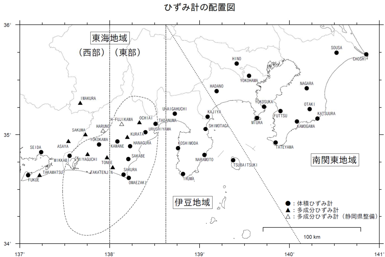
第 1 図 観測点の配置図 ● : 体積ひずみ計, ▲ : 多成分ひずみ計 (気象庁), △ : 同 (静岡県)
