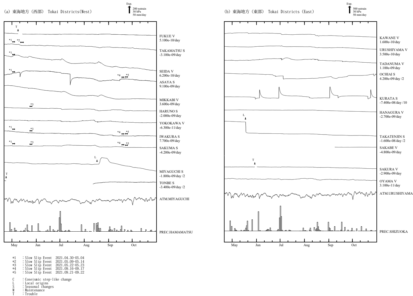
第 3 図 (a), (b) 2021 年 5 月～10 月の東海・伊豆・南関東地域における区域別体積ひずみ (V) 及び面積ひずみ (S) の変化 (時間値: 気圧・潮汐・降水補正した値)。各図下部に区域を代表する気圧変化と降水量を示す。地点名の下の D strain/day 及び /M はそれぞれ 1 日あたりのトレンド変化量を D として補正していること及び縮尺を 1/M 倍にして表示していることを示している。ゆっくりすべりが発生している期間を表示するため、4 月 21 日から表示している。
