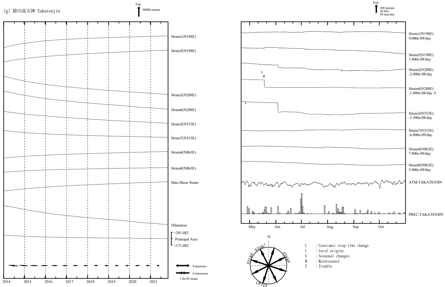
第 4 図 (g) 左：2014 年 1 月以後の多成分ひずみ計変化（日平均値）。主ひずみ・最大せん断ひずみ・面積ひずみは各方向成分から計算されている。 右：2021 年 5 月～10 月の多成分ひずみ計変化（時間値：気圧・潮汐・地磁気・降水補正した値）。各図下部に気圧変化と降水量を示す。ゆっくりすべりが発生している期間を表示するため、4 月 21 日から表示している。 Fig. 4(g) (Left) Strain changes observed by multi-component borehole strainmeters since January 2014 (daily mean values). Principal strain, maximum shear strain and dilatation are calculated with strain values obtained from each component. (Right) Strain changes from May to October 2021 (hourly values where changes due to barometric pressure, tidal effects, geomagnetic effects and rain effects are corrected) observed by multi-component borehole strainmeters. The start date of the figure is set to April 21 to include the period of slow slip event.
