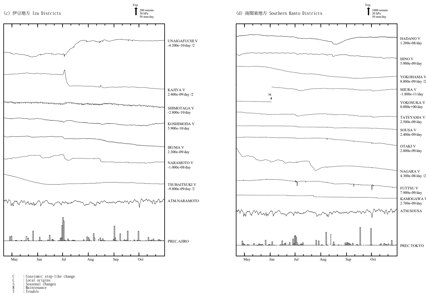
第 3 図 (c), (d) 2021 年 5 月～10 月の東海・伊豆・南関東地域における区域別体積ひずみ (V) 及び面積ひずみ (S) の変化 (時間値: 気圧・潮汐・降水補正した値)。各図下部に区域を代表する気圧変化と降水量を示す。地点名の下に D strain/day 及び /M はそれぞれ 1 日あたりのトレンド変化量を D として補正していること及び縮尺を 1/M 倍にして表示していることを示している。ゆっくりすべりが発生している期間を表示するため、4 月 21 日から表示している。
