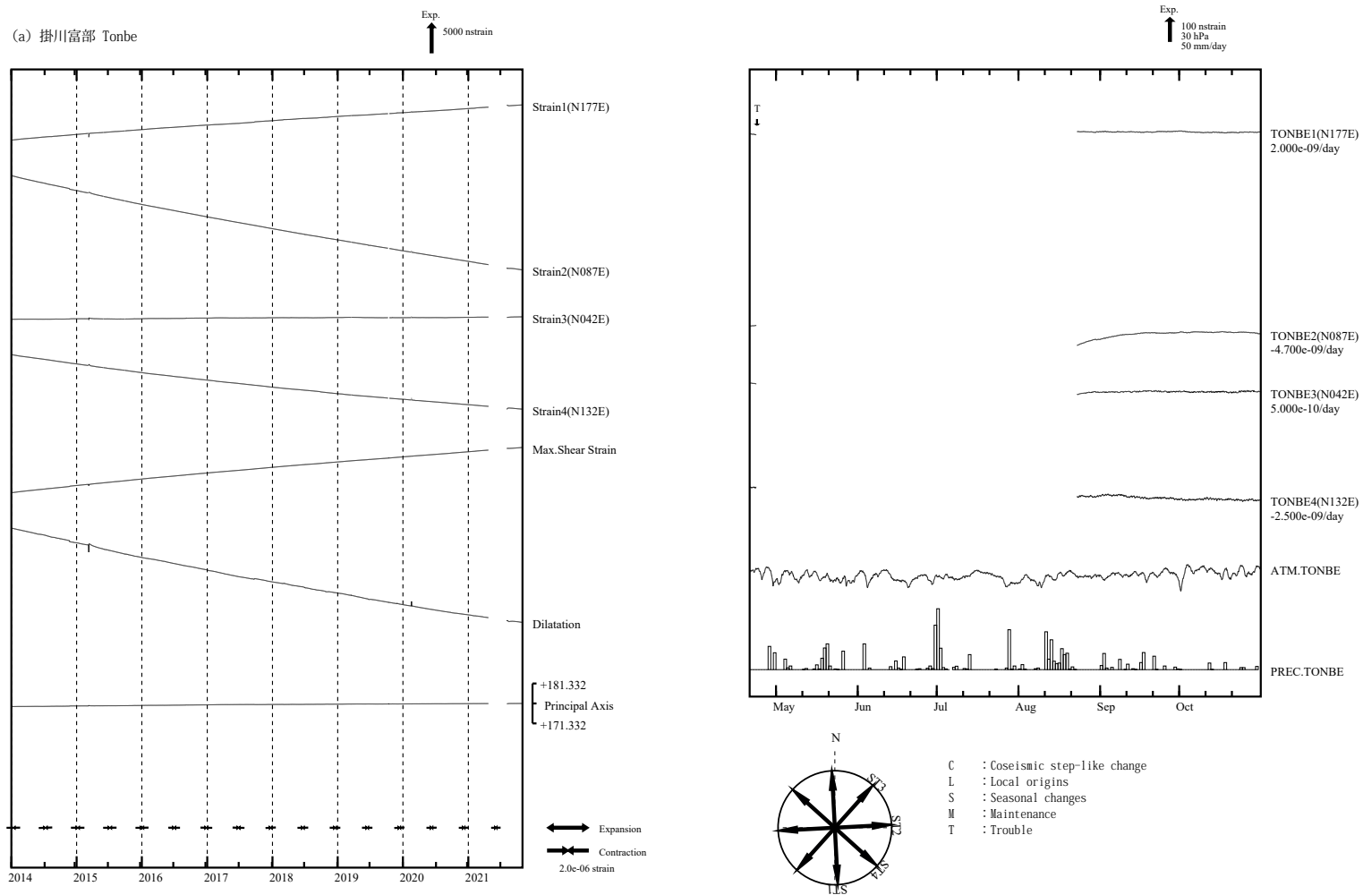
第 4 図 (a) 左：2014 年 1 月以後の多成分ひずみ計変化（日平均値）。主ひずみ・最大せん断ひずみ・面積ひずみは各方向成分から計算されている。 右：2021 年 5 月～10 月の多成分ひずみ計変化（時間値：気圧・潮汐・地磁気・降水補正した値）。各図下部に気圧変化と降水量を示す。ゆっくりすべりが発生している期間を表示するため、4 月 21 日から表示している。
