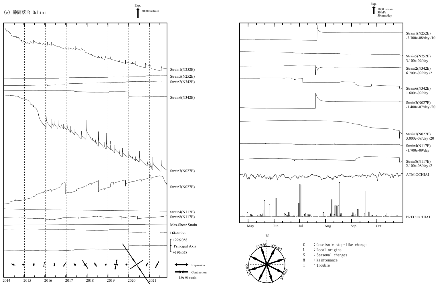
第 4 図 (e) 左：2014 年 1 月以後の多成分ひずみ計変化（日平均値）。主ひずみ・最大せん断ひずみ・面積ひずみは各方向成分から計算されている。 右：2021 年 5 月～10 月の多成分ひずみ計変化（時間値：気圧・潮汐・地磁気・降水補正した値）。各図下部に気圧変化と降水量を示す。ゆっくりすべりが発生している期間を表示するため、4 月 21 日から表示している。
