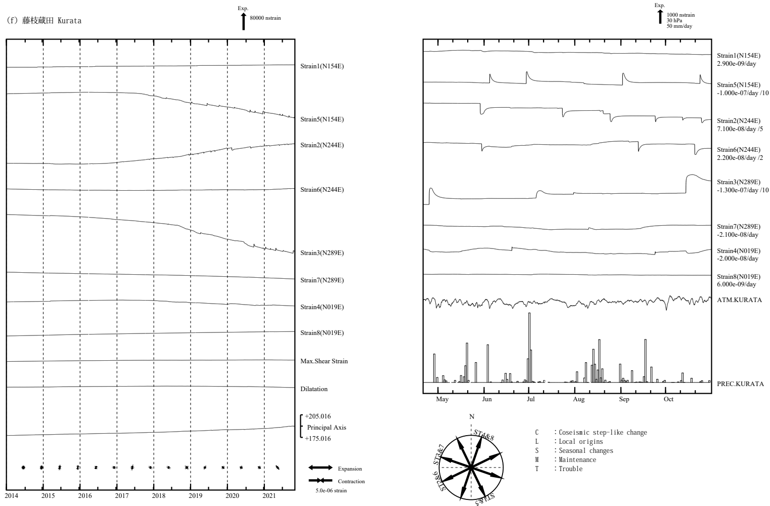
第 4 図 (f) 左：2014 年 1 月以後の多成分ひずみ計変化（日平均値）。主ひずみ・最大せん断ひずみ・面積ひずみは各方向成分から計算されている。 右：2021 年 5 月～10 月の多成分ひずみ計変化（時間値：気圧・潮汐・地磁気・降水補正した値）。各図下部に気圧変化と降水量を示す。ゆっくりすべりが発生している期間を表示するため、4 月 21 日から表示している。
