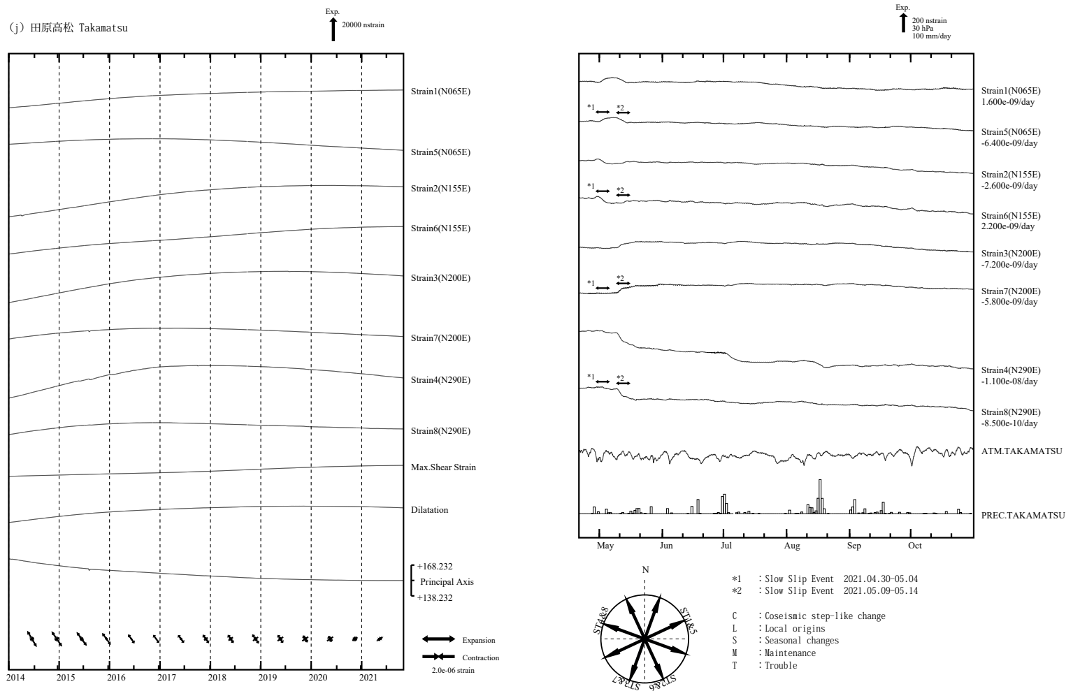
第 4 図 (j) 左：2014 年 1 月以後の多成分ひずみ計変化（日平均値）。主ひずみ・最大せん断ひずみ・面積ひずみは各方向成分から計算されている。 右：2021 年 5 月～10 月の多成分ひずみ計変化（時間値：気圧・潮汐・地磁気・降水補正した値）。各図下部に気圧変化と降水量を示す。ゆっくりすべりが発生している期間を表示するため、4 月 21 日から表示している。
