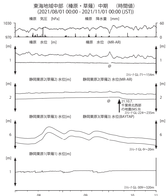
第 4 図 東海地域中部の地下水等の観測結果 (2021 年 8 月～2021 年 10 月)
