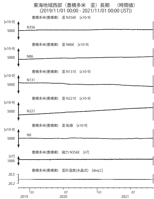
第 18 図 東海地域西部 (豊橋多米) の歪等の観測結果 (2019 年 11 月～2021 年 10 月)
