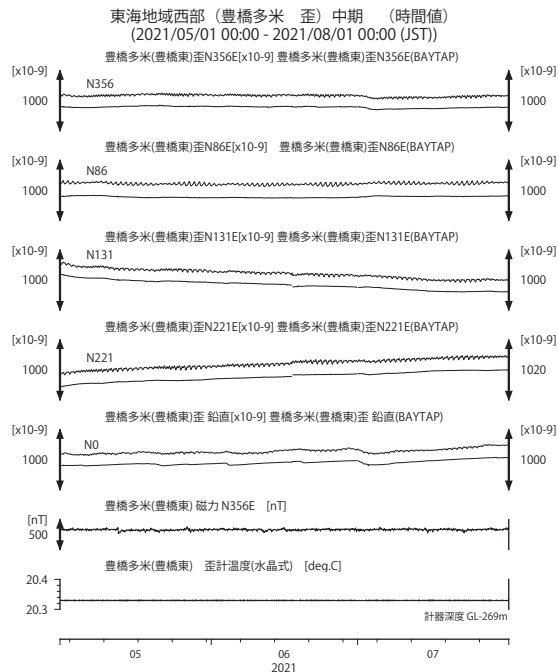
第 9 図 東海地域西部 (豊橋多米) の歪等の観測結果 (2021 年 5 月～2021 年 7 月)
