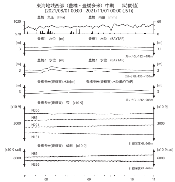
第 8 図 東海地域西部 (豊橋・豊橋多米) の地下水等の観測結果 (2021 年 8 月～2021 年 10 月)
