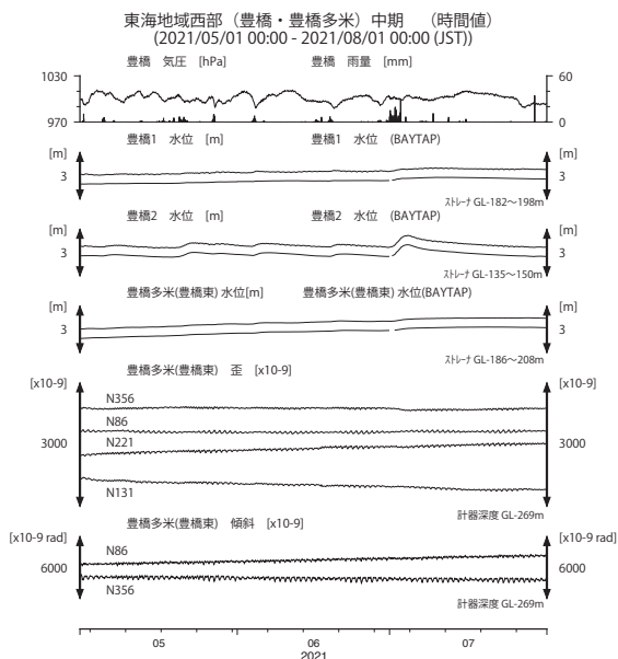
第 7 図 東海地域西部 (豊橋・豊橋多米) の地下水等の観測結果 (2021 年 5 月～2021 年 7 月)
