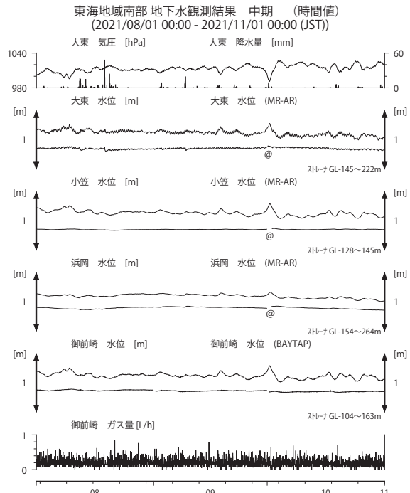
第 6 図 東海地域南部の地下水等の観測結果 (2021 年 8 月～2021 年 10 月)
