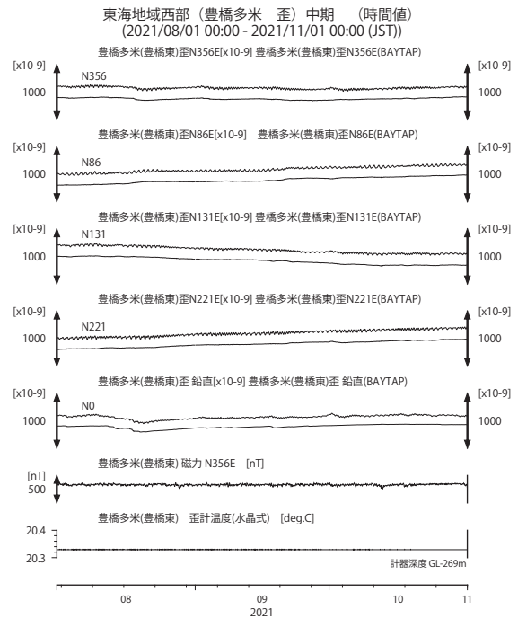
第 10 図 東海地域西部 (豊橋多米) の歪等の観測結果 (2021 年 8 月～2021 年 10 月)
