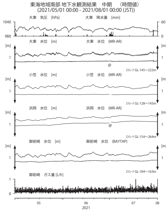
第 5 図 東海地域南部の地下水等の観測結果 (2021 年 5 月～2021 年 7 月)
