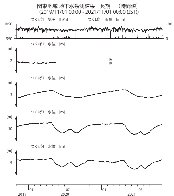
第 20 図 関東地域の地下水等の観測結果 (2019 年 11 月～2021 年 10 月)
