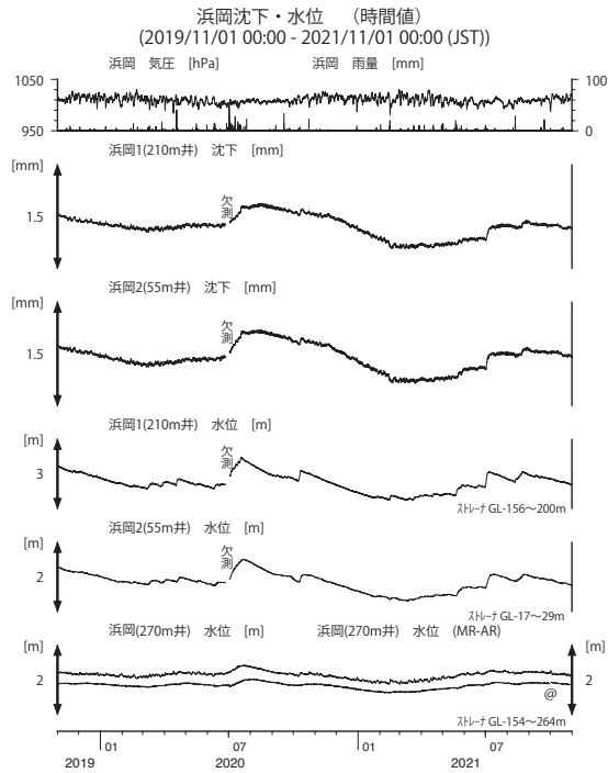
第 21 図 浜岡における沈下等の観測結果 (2019 年 11 月～2021 年 10 月)
