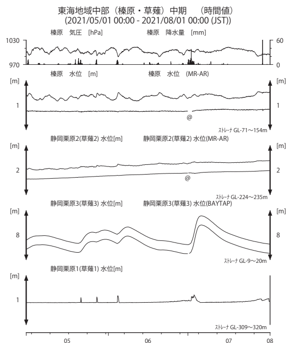
第 3 図 東海地域中部の地下水等の観測結果 (2021 年 5 月～2021 年 7 月)
