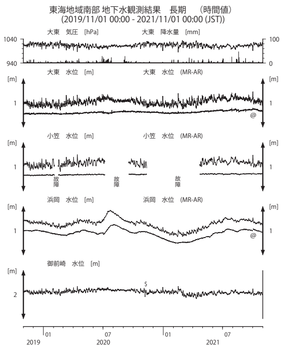
第 16 図 東海地域南部の地下水等の観測結果 (2019 年 11 月 ~ 2021 年 10 月)
