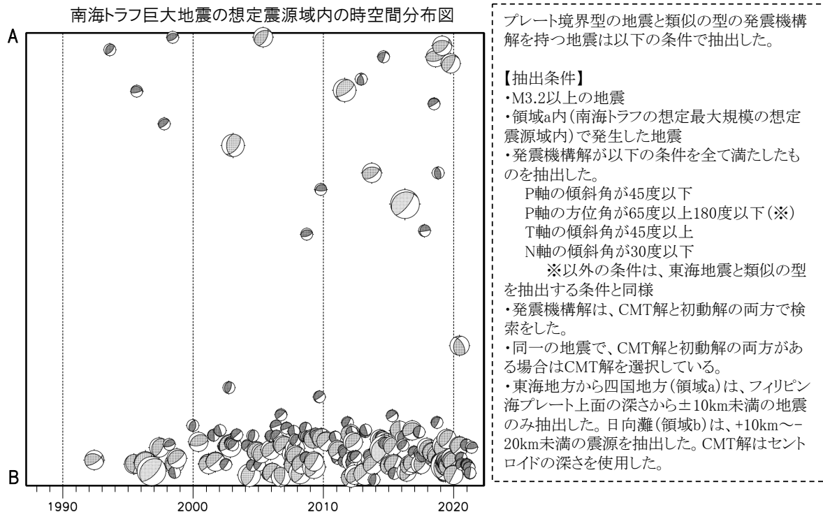
第 14 図 想定南海トラフ地震の発震機構解と類似の型の地震
