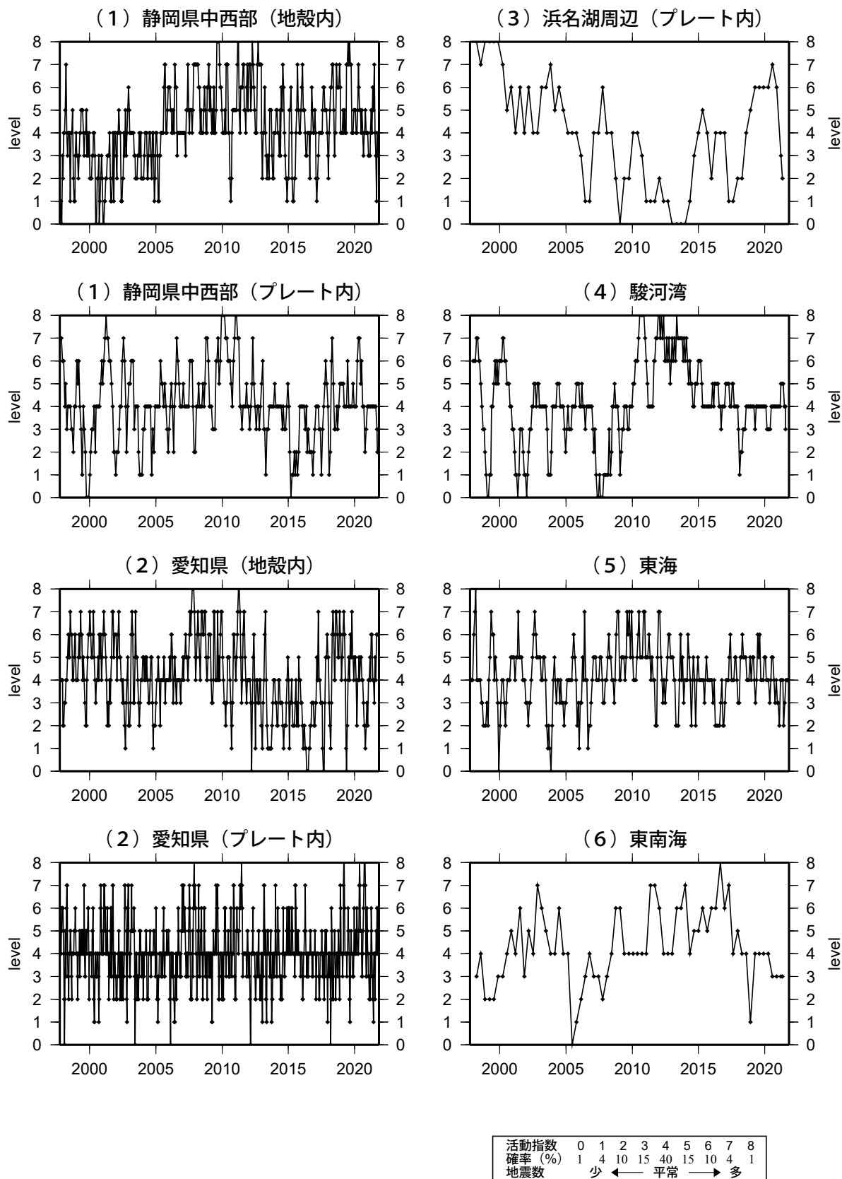
第 16 図 (a) 南海トラフ周辺の地震活動指数の推移
