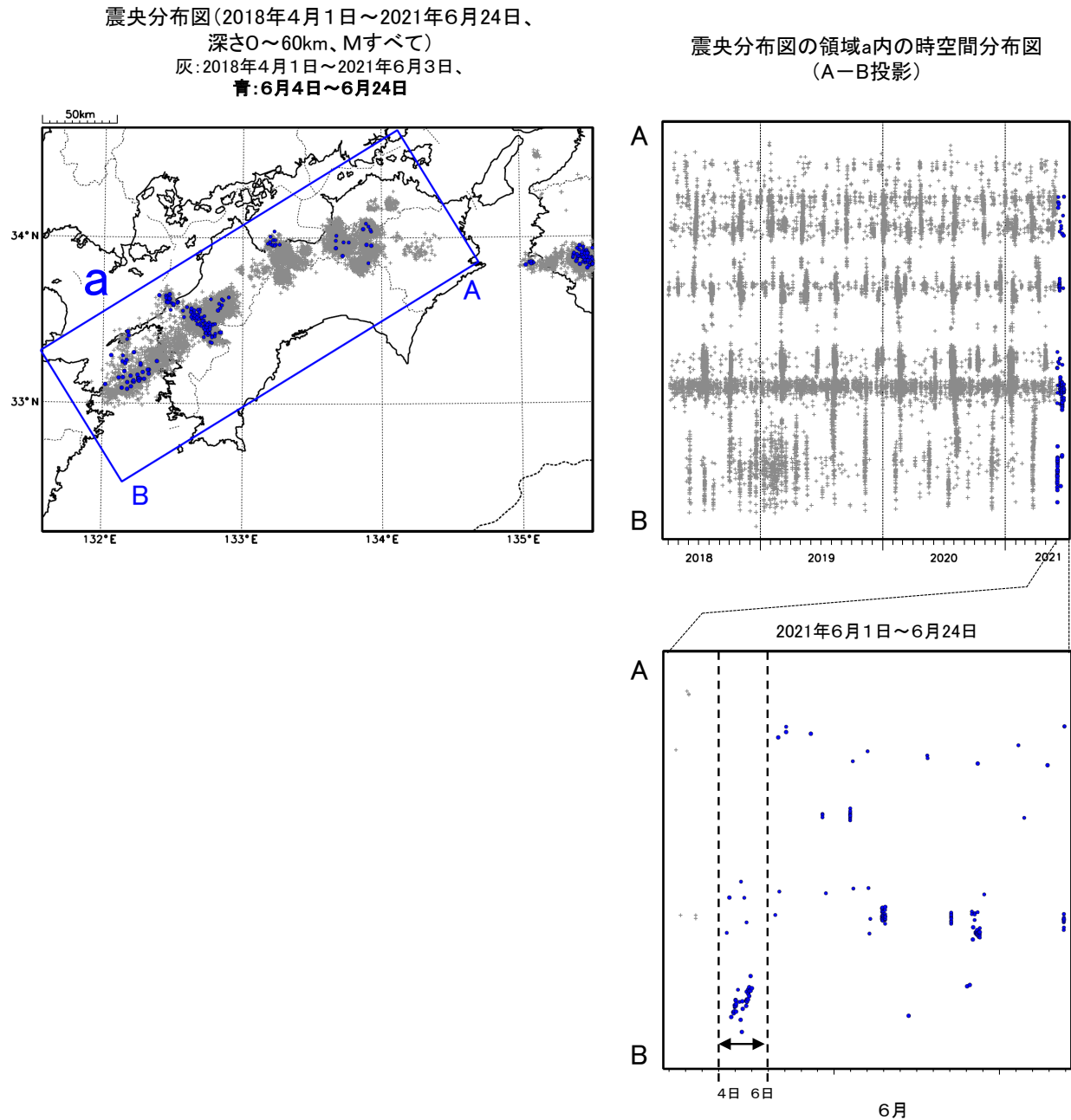
第 9 図 (a) 四国西部の深部低周波地震活動とひずみ変化，及び推定されるゆっくりすべり領域
