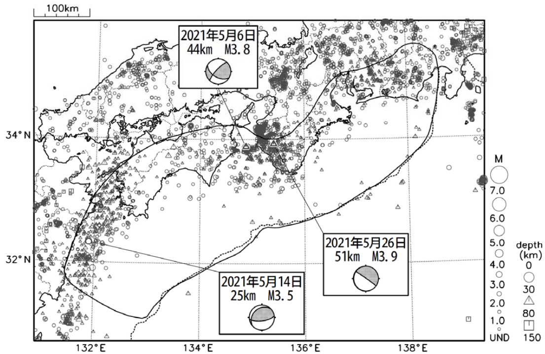
第 1 図 (a) 南海トラフ周辺の月別震央分布 (2021 年 5 月)
