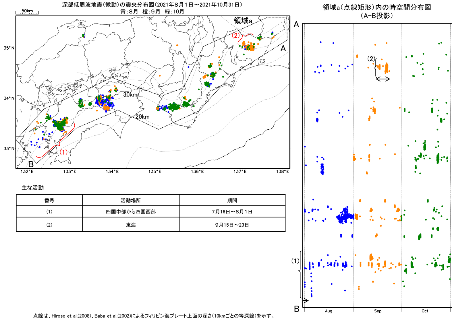
第2図(c) 東海地域から豊後水道にかけての深部低周波地震活動(2021年8月～10月)。
