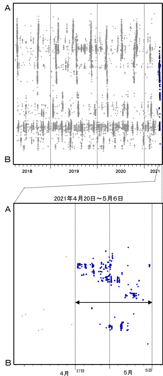
第4図(a) 紀伊半島北部から紀伊半島中部の深部低周波地震活動とひずみ変化、及び推定されるゆっくりすべり領域
