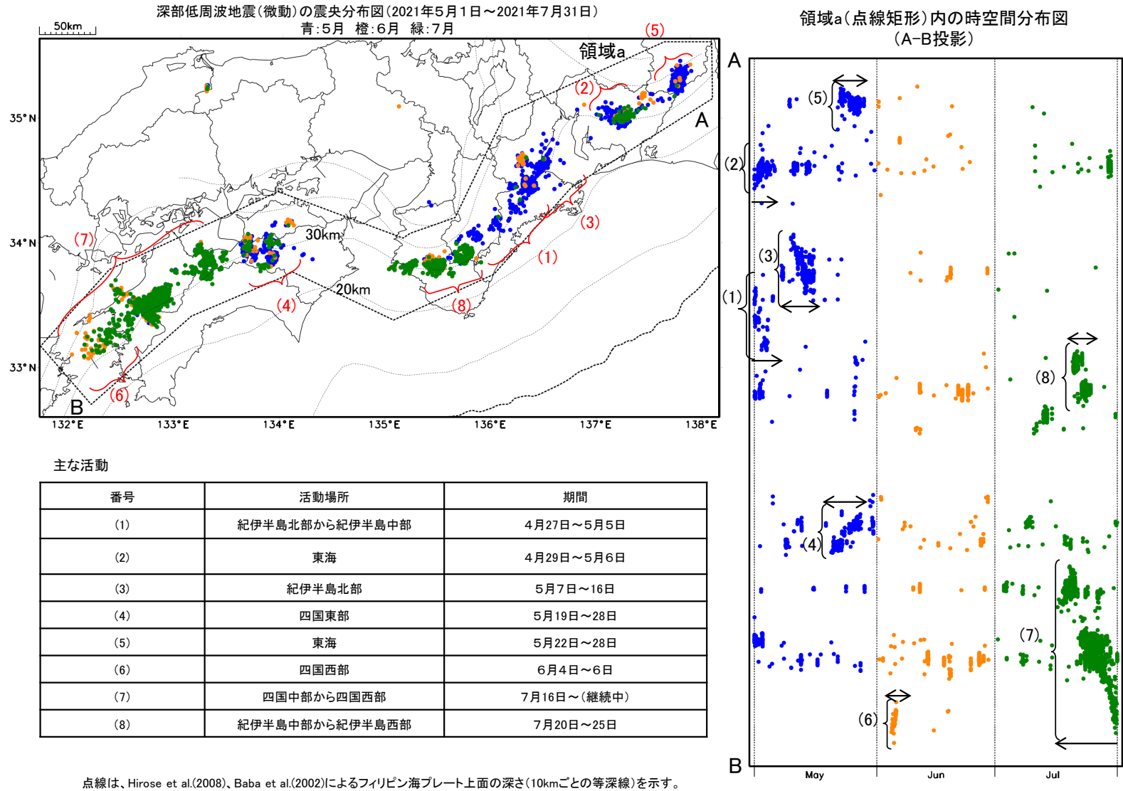
第2図 (a) 東海地域から豊後水道にかけての深部低周波地震活動 (2021年5月～7月)。
