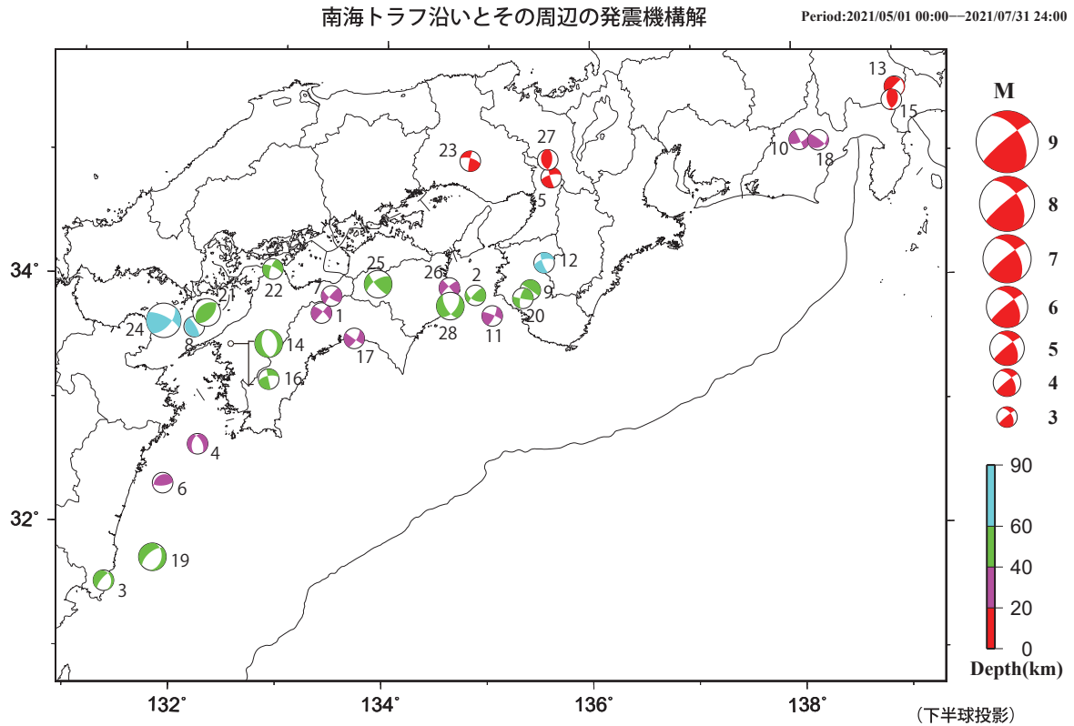
第 3 図 (a) 南海トラフ周辺で発生した主な地震の発震機構解 (2021 年 5 月～7 月)
