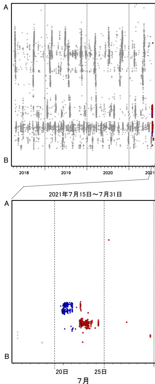
第 11 図 (a) 紀伊半島中部から紀伊半島西部の深部低周波地震活動とひずみ変化、及び推定されるゆっくりすべり領域
