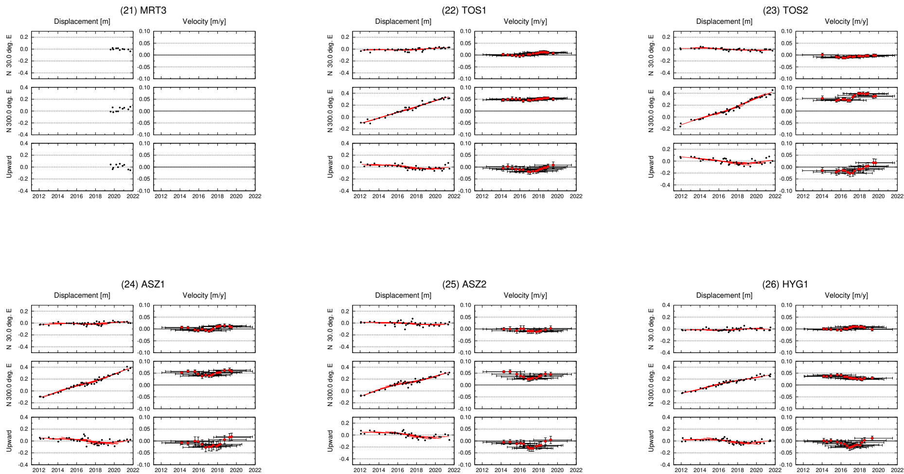
第 2 図 GNSS-A 観測時系列【アムールプレート固定】
