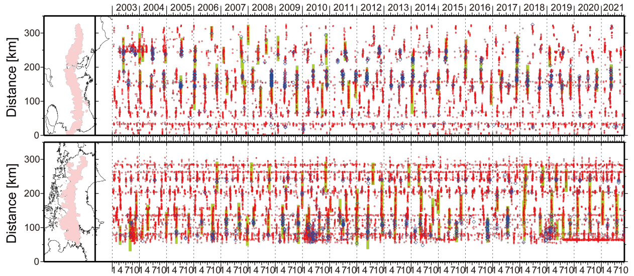
第 3 図 西南日本で発生した深部低周波微動（赤丸）及び深部超低周波地震（青菱形）の 2003 年から約 19 年間の時空間分布。黄緑色太線は、傾斜変動から検出された短期的スロースリップイベントを示す。
