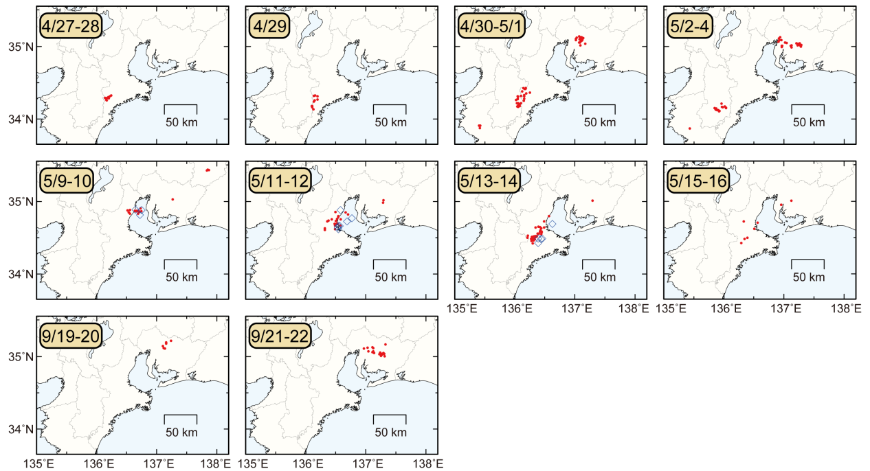
第 4 図 2021 年 5 月から 2021 年 10 月までの期間に東海・紀伊半島地域で発生した、主な深部低周波微動及び深部超低周波地震の活動における震央分布スナップショット。赤丸が当該期間の微動、青菱形が超低周波地震を表す。
