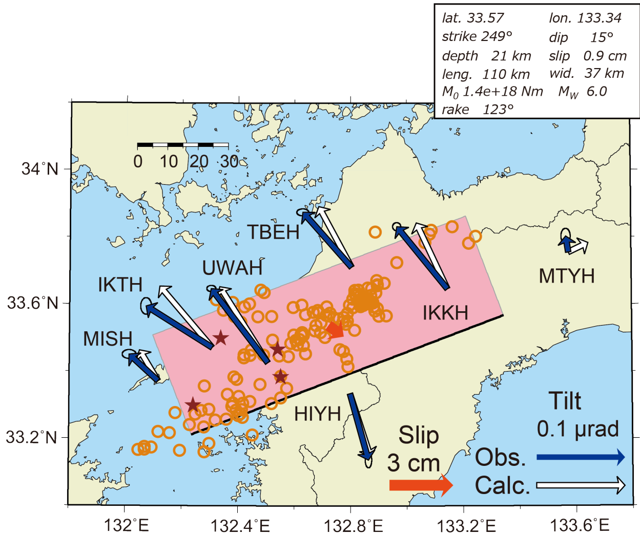
第 5 図 2021 年 7 月～8 月四国中西部の短期的 SSE の断層モデル。図の見方は第 3 図と同じ。
