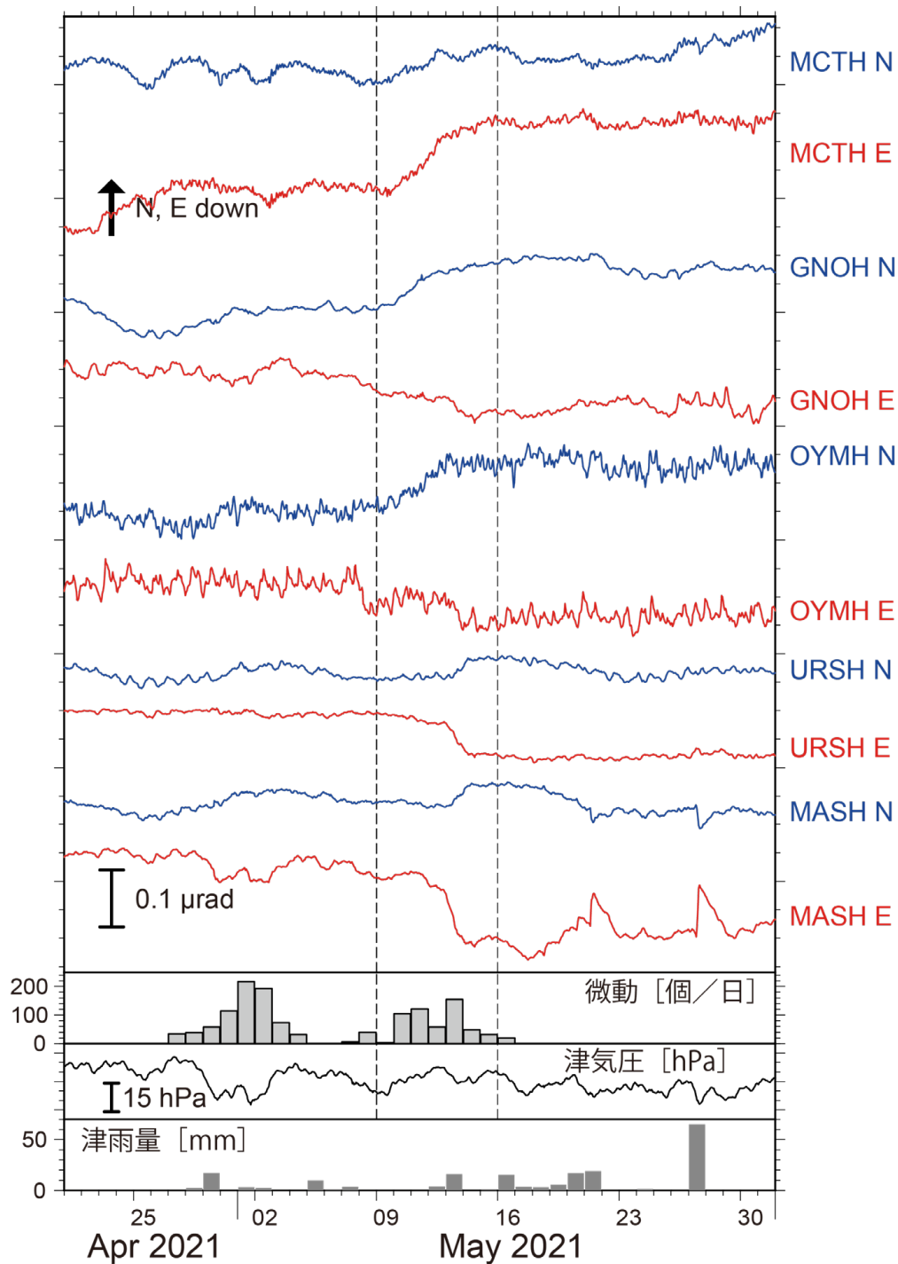
第 2 図 2021 年 4 月 21 日～5 月 31 日までの傾斜時系列。観測点位置は第 3 図に示した。記録は上方向への変化が北・東下がりの傾斜変動を表す。気圧応答・潮汐成分を BAYTAP-G4) により除去し、直線トレンドを補正した後の記録を示した。5 月 9 日～15 日の傾斜変化量を SSE によるものと仮定した。紀伊半島北部での微動活動度・気象庁津観測点での気圧変化および雨量をあわせて表示した。
