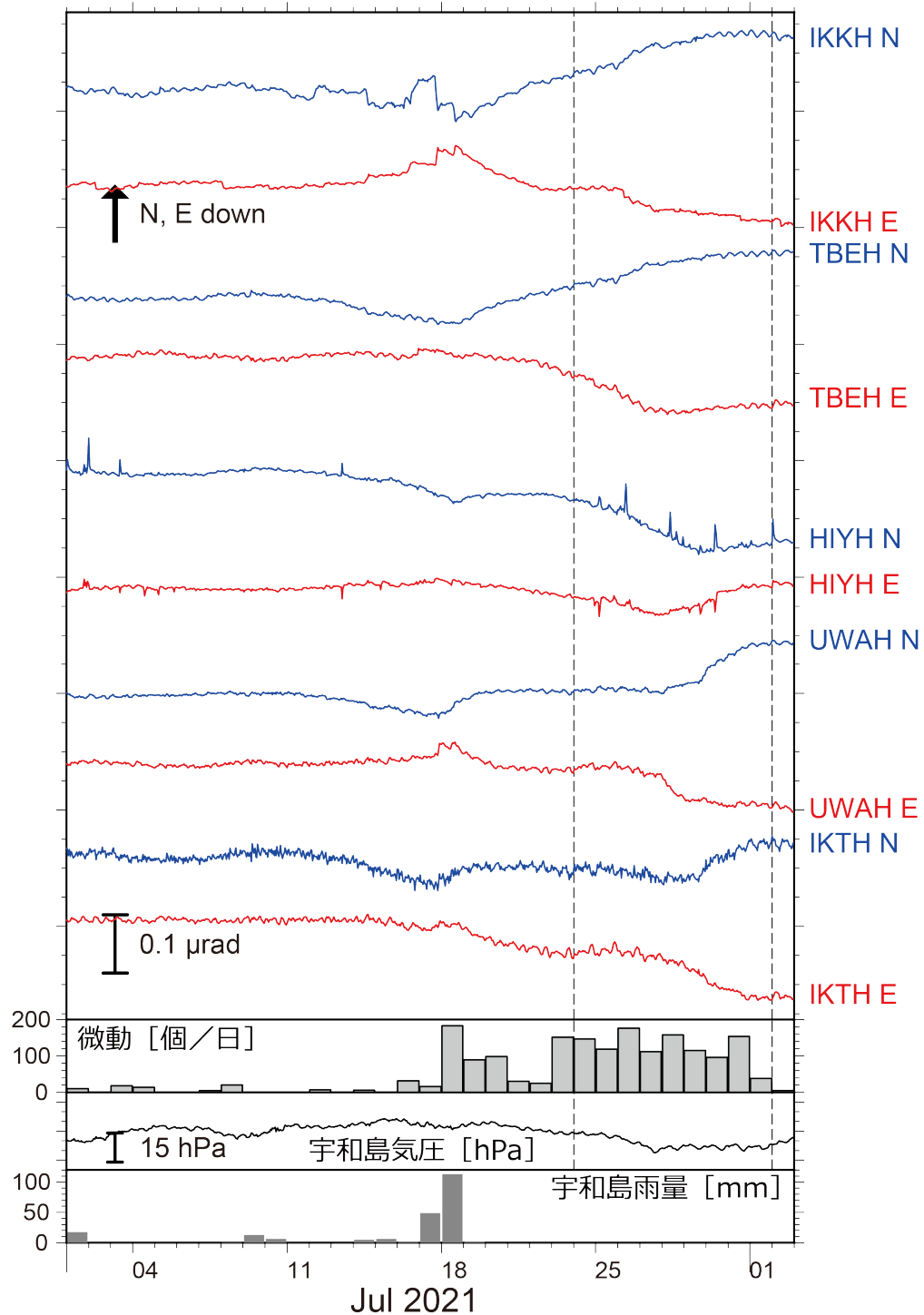
第 4 図 2021 年 7 月 1 日～8 月 2 日までの傾斜時系列。図の見方は第 2 図と同様。観測点位置は第 5 図に示した。7 月 24 日～8 月 1 日の傾斜変化量を SSE によるものと仮定した。四国中西部での微動活動度・気象庁宇和島観測点での気圧変化および雨量をあわせて表示した。
