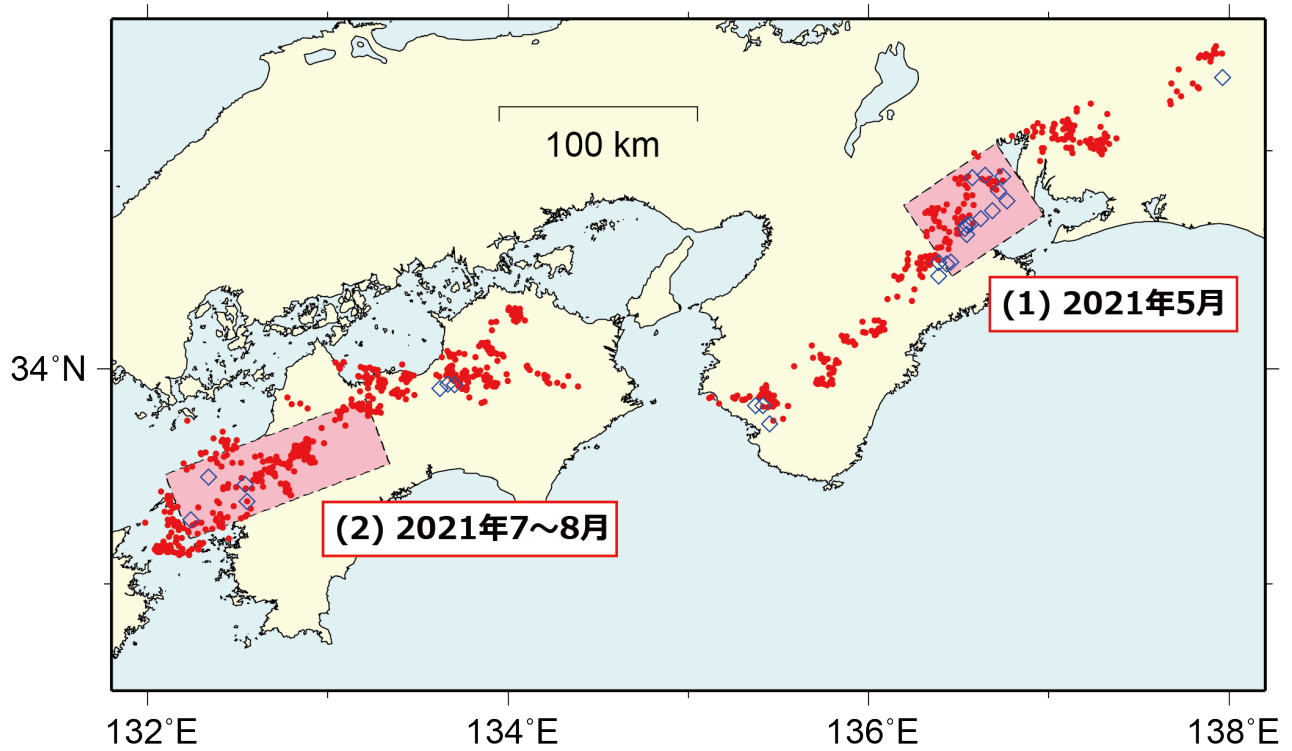
第 1 図 2021 年 5 月 1 日～2021 年 10 月 31 日の期間に検知された短期的 SSE (ピンク矩形). 同期間に発生した深部低周波微動 (赤点) 及び VLFE の震央 (青菱形) を重ねて表示した.
