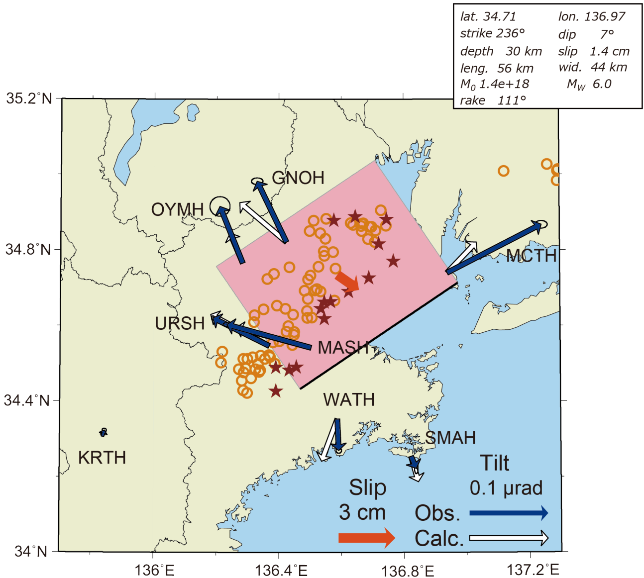
第 3 図 2021 年 5 月紀伊半島北部の短期的 SSE の断層モデル。2021 年 5 月 9 日～15 日に観測された傾斜変化ベクトル（青矢印）・このデータから推定された SSE の断層モデル（赤矩形・矢印）・モデルから計算される傾斜変化ベクトル（白抜き矢印）を示す。同じ期間の微動と深部超低周波地震の震央を橙円と茶星印で示した。
