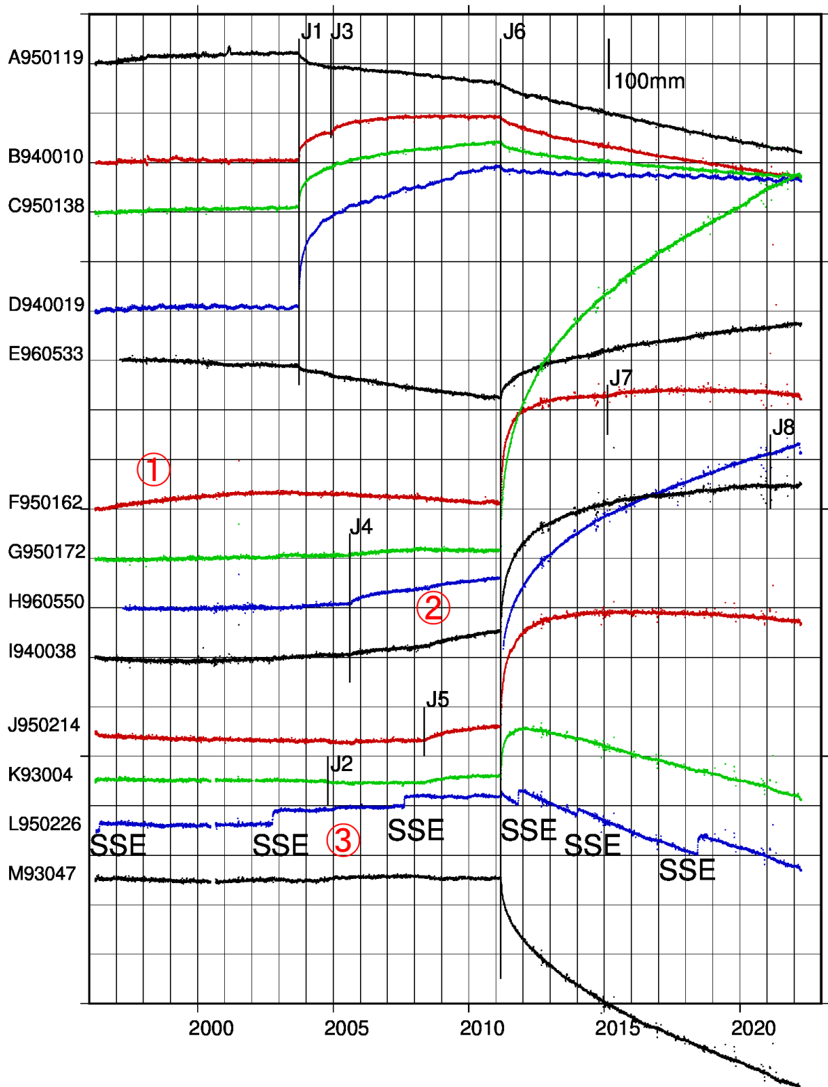
第 2a 図 プレート沈み込み方向の位置変化（東日本；1996 年から 2022 年 4 月） 沈み込みと逆方向が上向き。地点番号は、第 1 図の観測点記号に GEONET 観測点番号を付加したもの。 J1:2003 年十勝沖地震 (M8.0), J2:2004 年新潟県中越地震 (M6.8), J3:2004 年 11 月 29 日釧路沖の地震 (M7.1), J4:2005 年 8 月 16 日宮城県沖の地震 (M7.2), J5:2008 年 5 月 8 日茨城県沖の地震 (M7.0), J6:2011 年東北地 方太平洋沖地震 (M9.0), J7:2015 年 2 月 17 日三陸沖の地震 (M6.9), J8:2021 年 2 月 13 日福島県沖の地震 (M7.3).
