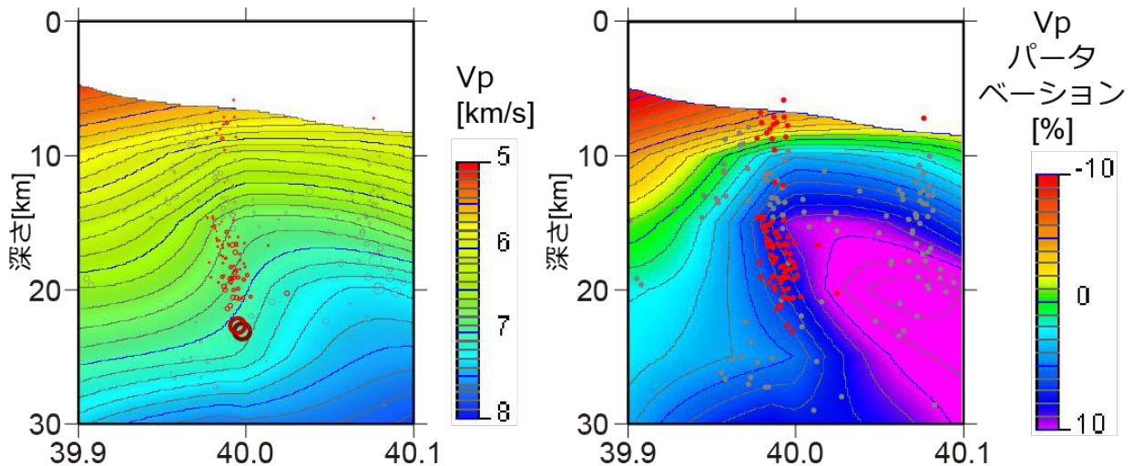
第 2 図 防災科研 F-net による発震機構解の走向に直交する断面における震源分布と P 波速度構造および P 波速度パータベーション構造. 第 1 図の青枠内の震源を示す.
