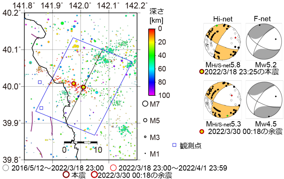
第 1 図 三次元地震波速度構造と観測点補正値 1) を用いて再決定した震源分布と主な地震の発震機構解. 青枠は第 2 図の断面図と震源分布の範囲を示す. シンボル内の色は地震の深さを示す.
