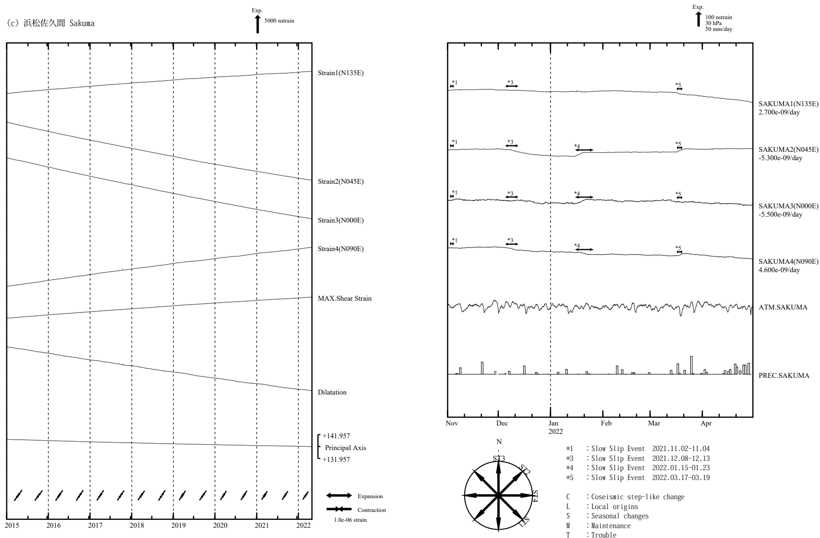
第 4 図 (c) 左 : 2015 年 1 月以後の多成分ひずみ計変化 (日平均値)。主ひずみ・最大せん断ひずみ・面積ひずみは各方向成分から計算されている。 右 : 2021 年 11 月～2022 年 4 月の多成分ひずみ計変化 (時間値 : 気圧・潮汐・地磁気・降水補正した値)。各図下部に気圧変化と降水量を示す。
