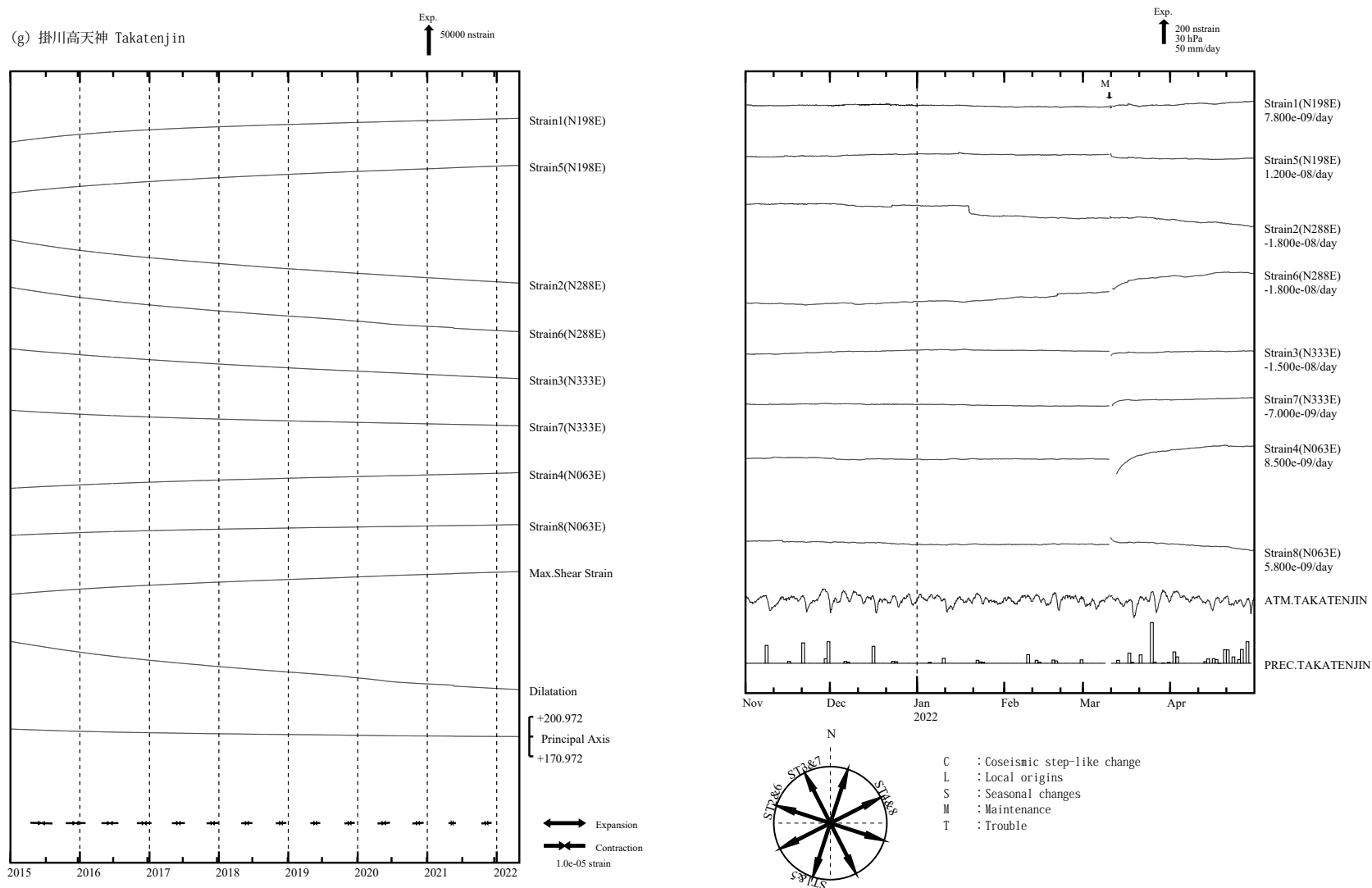
第 4 図 (g) 左：2015 年 1 月以後の多成分ひずみ計変化（日平均値）。主ひずみ・最大せん断ひずみ・面積ひずみは各方向成分から計算されている。 右：2021 年 11 月～2022 年 4 月の多成分ひずみ計変化（時間値：気圧・潮汐・地磁気・降水補正した値）。各図下部に気圧変化と降水量を示す。
