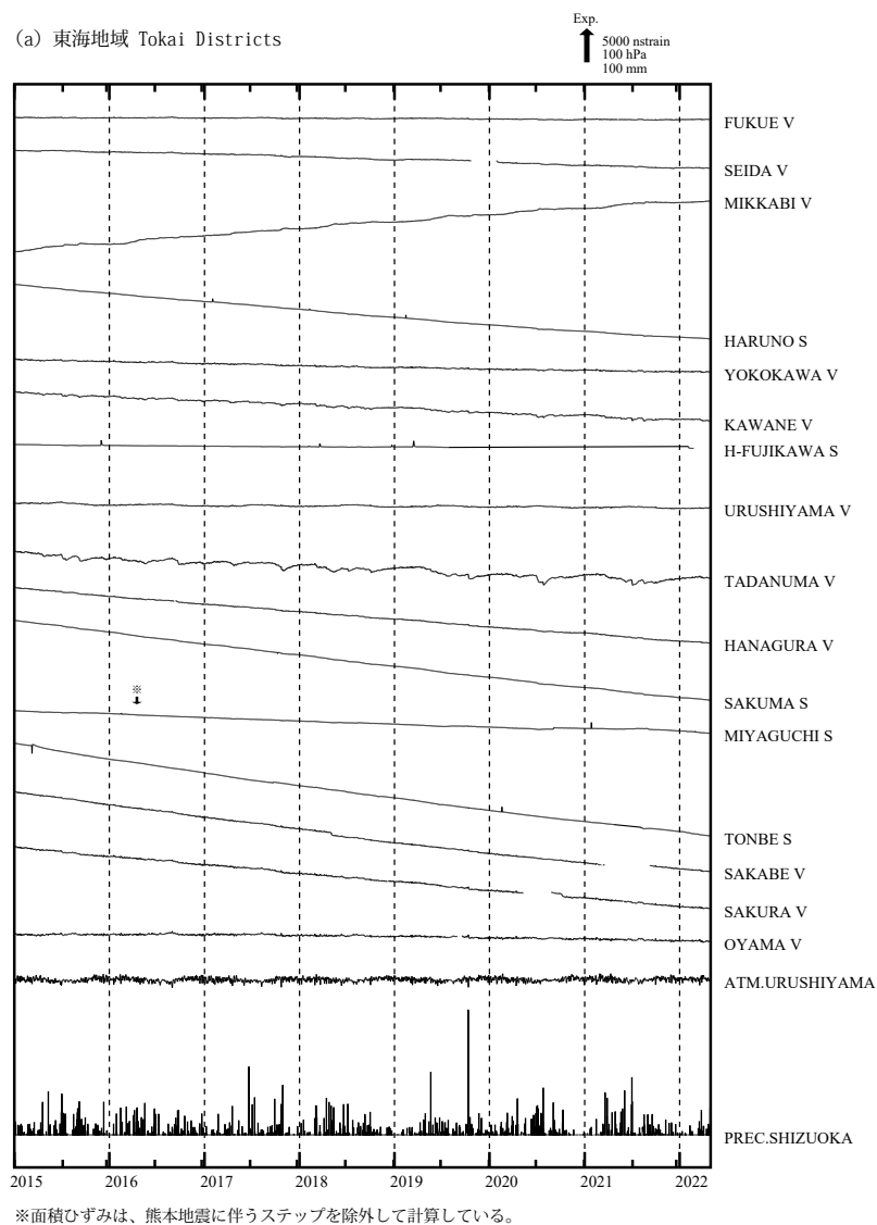
第 2 図 (a),(b) 2015 年 1 月以後の東海・伊豆・南関東地域における区域別体積ひずみ (V) 及び面積ひずみ (S) の変化 (日平均値). 各図下部に区域を代表する気圧変化と降水量を示す.
