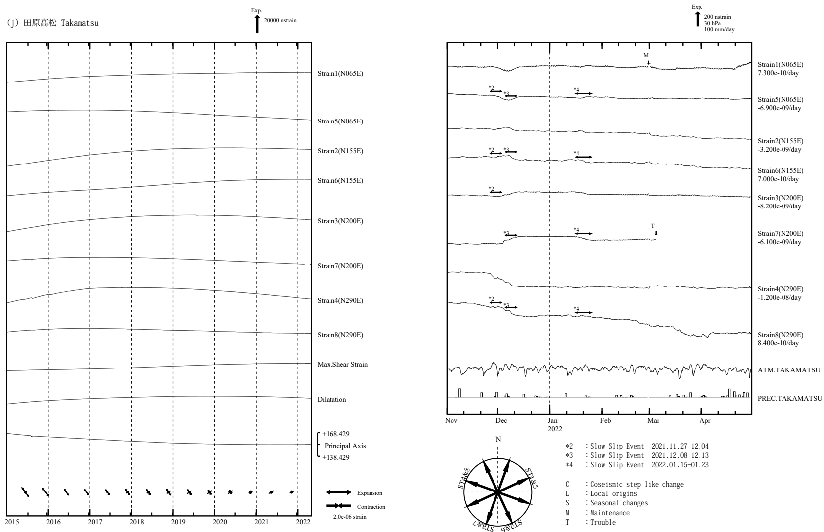
第 4 図 (j) 左 : 2015 年 1 月以後の多成分ひずみ計変化 (日平均値)。主ひずみ・最大せん断ひずみ・面積ひずみは各方向成分から計算されている。 右 : 2021 年 11 月～2022 年 4 月の多成分ひずみ計変化 (時間値 : 気圧・潮汐・地磁気・降水補正した値)。各図下部に気圧変化と降水量を示す。
