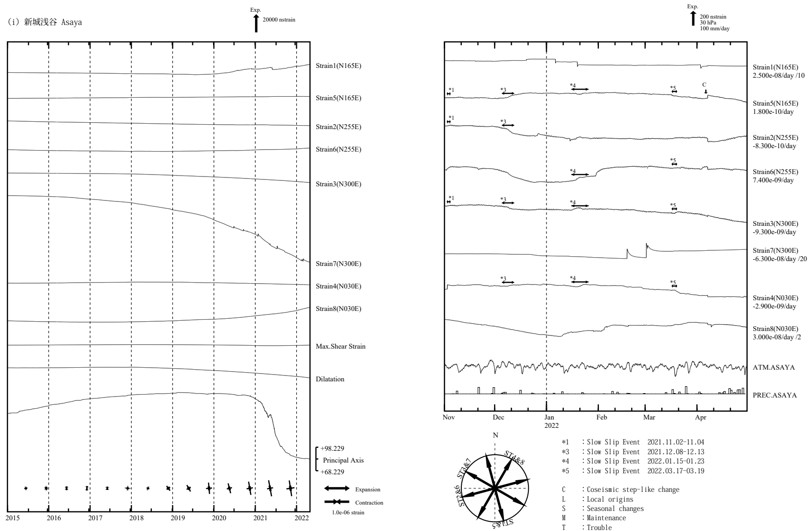
第 4 図 (i) 左 : 2015 年 1 月以後の多成分ひずみ計変化 (日平均値). 主ひずみ・最大せん断ひずみ・面積ひずみは各方向成分から計算されている. 右 : 2021 年 11 月～2022 年 4 月の多成分ひずみ計変化 (時間値 : 気圧・潮汐・地磁気・降水補正した値). 各図下部に気圧変化と降水量を示す.
