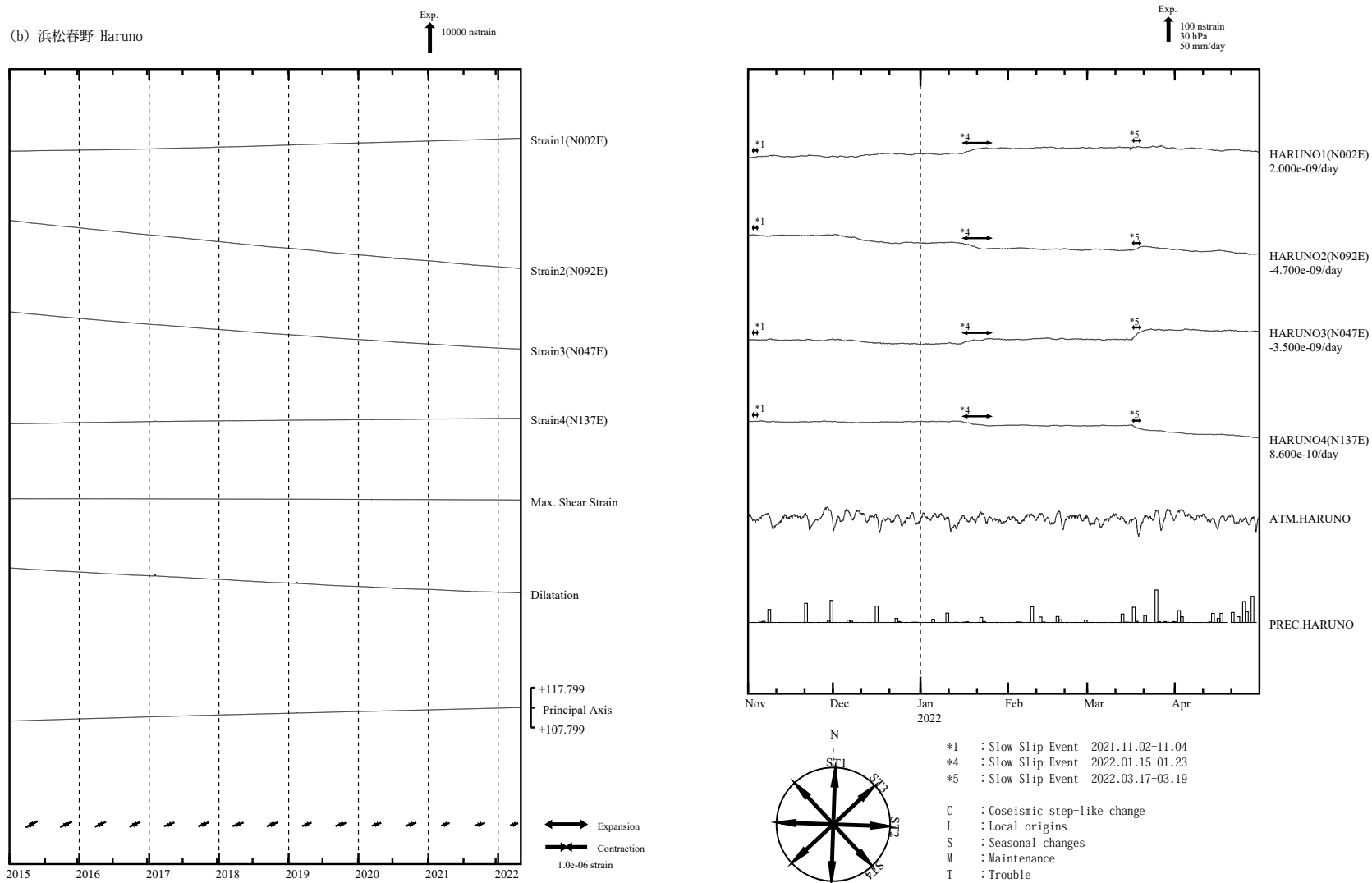
第 4 図 (b) 左：2015 年 1 月以後の多成分ひずみ計変化（日平均値）。主ひずみ・最大せん断ひずみ・面積ひずみは各方向成分から計算されている。 右：2021 年 11 月～2022 年 4 月の多成分ひずみ計変化（時間値：気圧・潮汐・地磁気・降水補正した値）。各図下部に気圧変化と降水量を示す。
