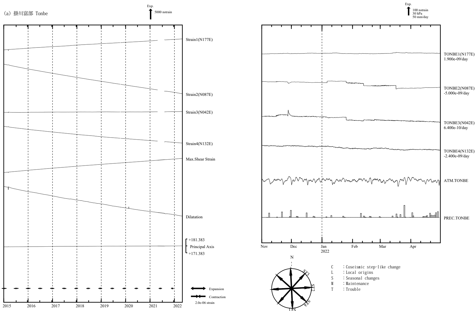
第 4 図 (a) 左：2015 年 1 月以後の多成分ひずみ計変化（日平均値）。主ひずみ・最大せん断ひずみ・面積ひずみは各方向成分から計算されている。 右：2021 年 11 月～2022 年 4 月の多成分ひずみ計変化（時間値：気圧・潮汐・地磁気・降水補正した値）。各図下部に気圧変化と降水量を示す。
