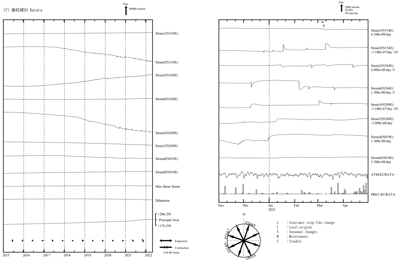
第 4 図 (f) 左：2015 年 1 月以後の多成分ひずみ計変化（日平均値）。主ひずみ・最大せん断ひずみ・面積ひずみは各方向成分から計算されている。 右：2021 年 11 月～2022 年 4 月の多成分ひずみ計変化（時間値：気圧・潮汐・地磁気・降水補正した値）。各図下部に気圧変化と降水量を示す。
