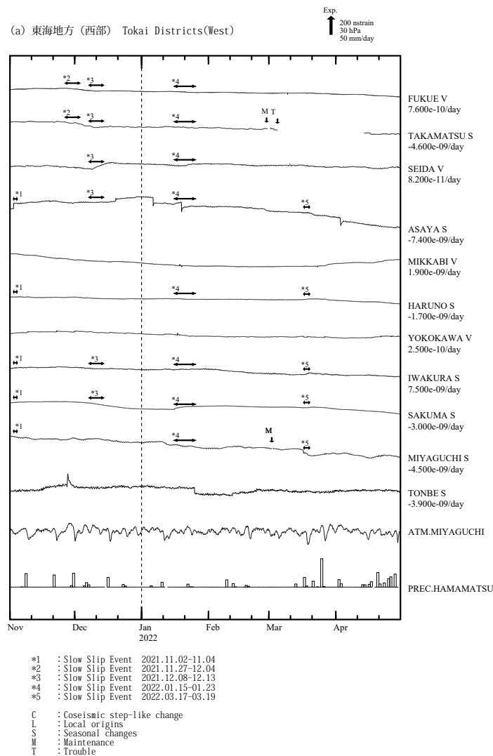
第 3 図 (a),(b) 2021 年 11 月～2022 年 4 月の東海・伊豆・南関東地域における区域別体積ひずみ (V) 及び面積ひずみ (S) の変化 (時間値: 気圧・潮汐・降水補正した値)。各図下部に区域を代表する気圧変化と降水量を示す。地点名の下に D strain/day 及び /M はそれぞれ 1 日あたりのトレンド変化量を D として補正していること及び縮尺を 1/M 倍にして表示していることを示している。
