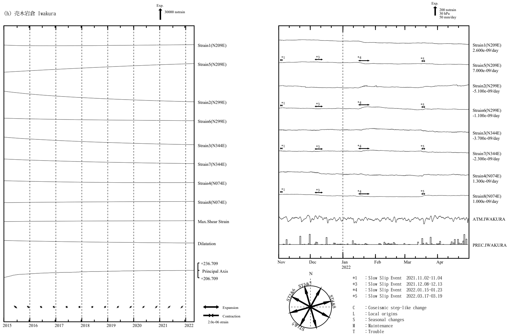
第 4 図 (h) 左：2015 年 1 月以後の多成分ひずみ計変化（日平均値）。主ひずみ・最大せん断ひずみ・面積ひずみは各方向成分から計算されている。 右：2021 年 11 月～2022 年 4 月の多成分ひずみ計変化（時間値：気圧・潮汐・地磁気・降水補正した値）。各図下部に気圧変化と降水量を示す。
