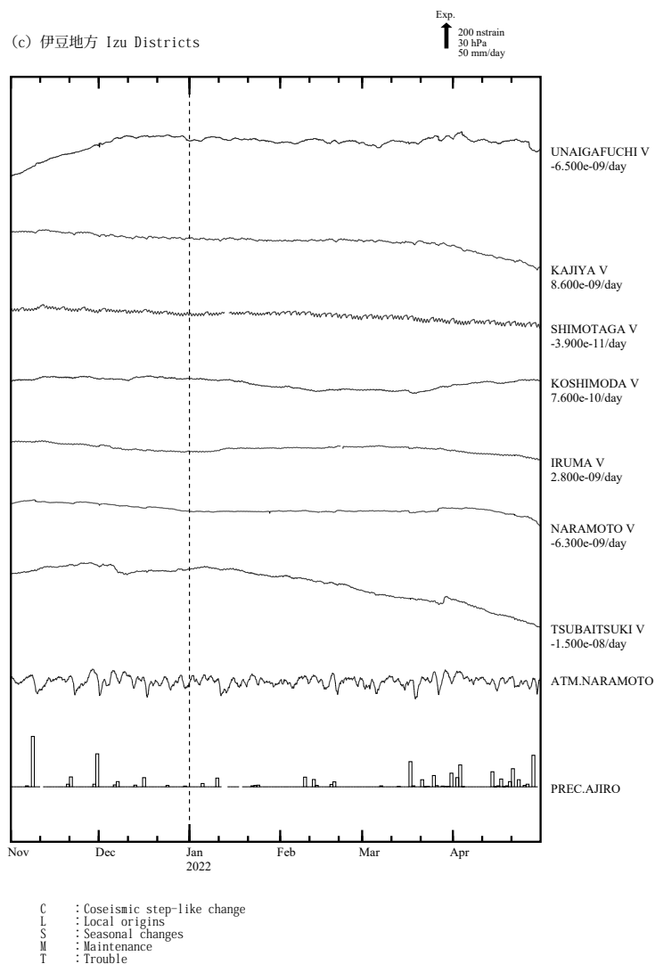
第 3 図 (c),(d) 2021 年 11 月～2022 年 4 月の東海・伊豆・南関東地域における区域別体積ひずみ (V) 及び面積ひずみ (S) の変化 (時間値: 気圧・潮汐・降水補正した値)。各図下部に区域を代表する気圧変化と降水量を示す。地点名の下に D strain/day 及び /M はそれぞれ 1 日あたりのトレンド変化量を D として補正していること及び縮尺を 1/M 倍にして表示していることを示している。
