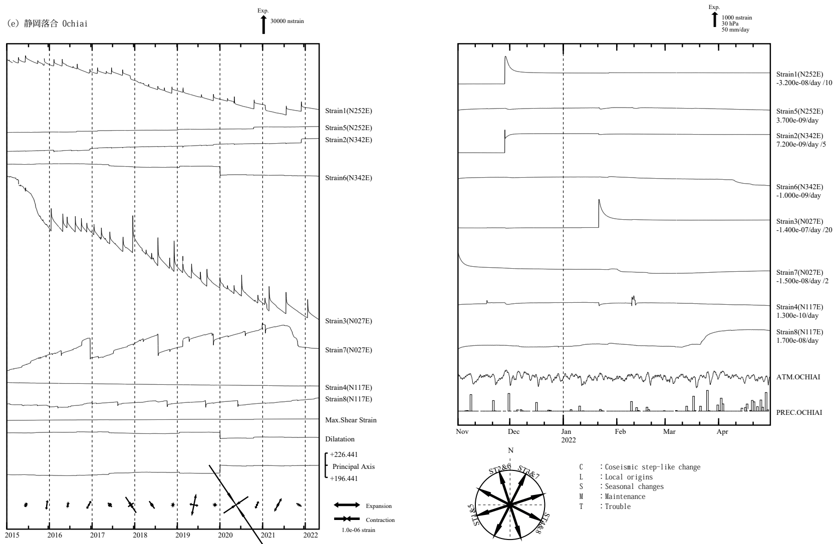
第 4 図 (e) 左：2015 年 1 月以後の多成分ひずみ計変化（日平均値）。主ひずみ・最大せん断ひずみ・面積ひずみは各方向成分から計算されている。 右：2021 年 11 月～2022 年 4 月の多成分ひずみ計変化（時間値：気圧・潮汐・地磁気・降水補正した値）。各図下部に気圧変化と降水量を示す。
