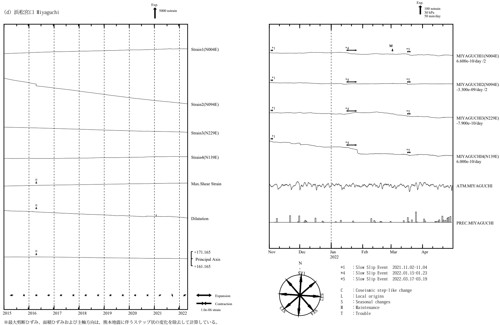
第4図(d) 左：2015年1月以後の多成分ひずみ計変化（日平均値）。主ひずみ・最大せん断ひずみ・面積ひずみは各方向成分から計算されている。 右：2021年11月～2022年4月の多成分ひずみ計変化（時間値：気圧・潮汐・地磁気・降水補正した値）。各図下部に気圧変化と降水量を示す。
