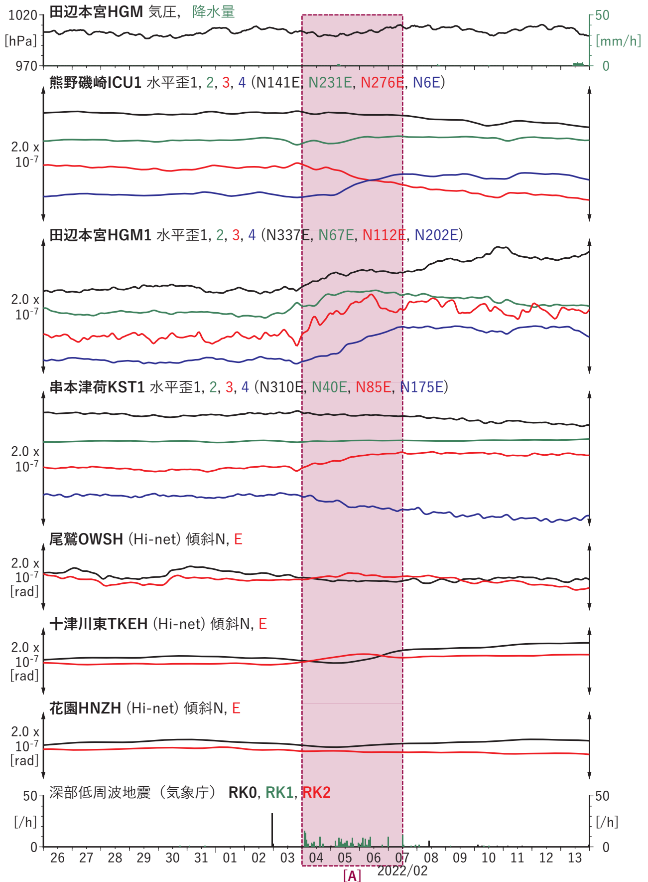
第 34 図 紀伊半島における歪・傾斜の観測結果と低周波地震の検出数 (2022/01/26 ~ 2022/02/13)。
