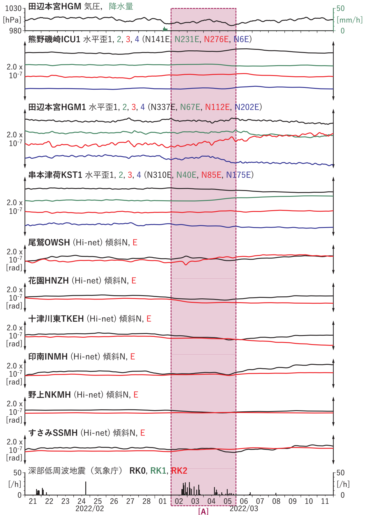
第 40 図 紀伊半島における歪・傾斜の観測結果と低周波地震の検出数 (2022/02/21 ~ 2022/03/11).
