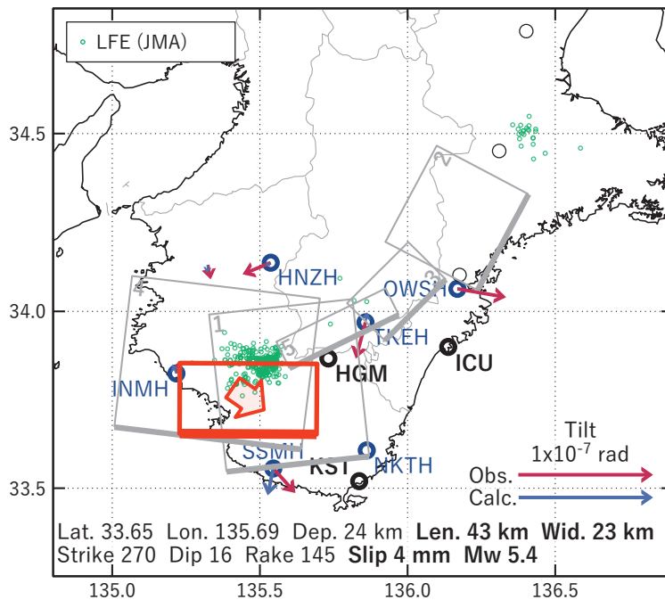
第 41 図 第 40 図 [A] を説明する断層モデル. 各図の説明は第 3 図を参照. Fig. 41 Inferred fault models for Fig. 40[A]. See also the caption of Fig. 3.
