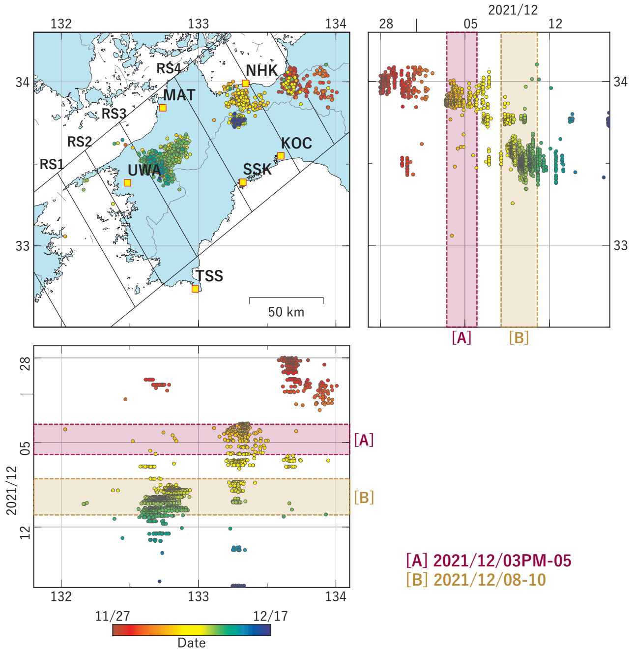
第 13 図 四国西部における低周波地震（気象庁一元化カタログによる）の時空間分布（2021/11/27 ～ 2021/12/16）. Fig. 13 Space-time distribution of low-frequency earthquakes by JMA unified hypocenter catalog in the Western Shikoku from November 27 to December 16, 2021.
