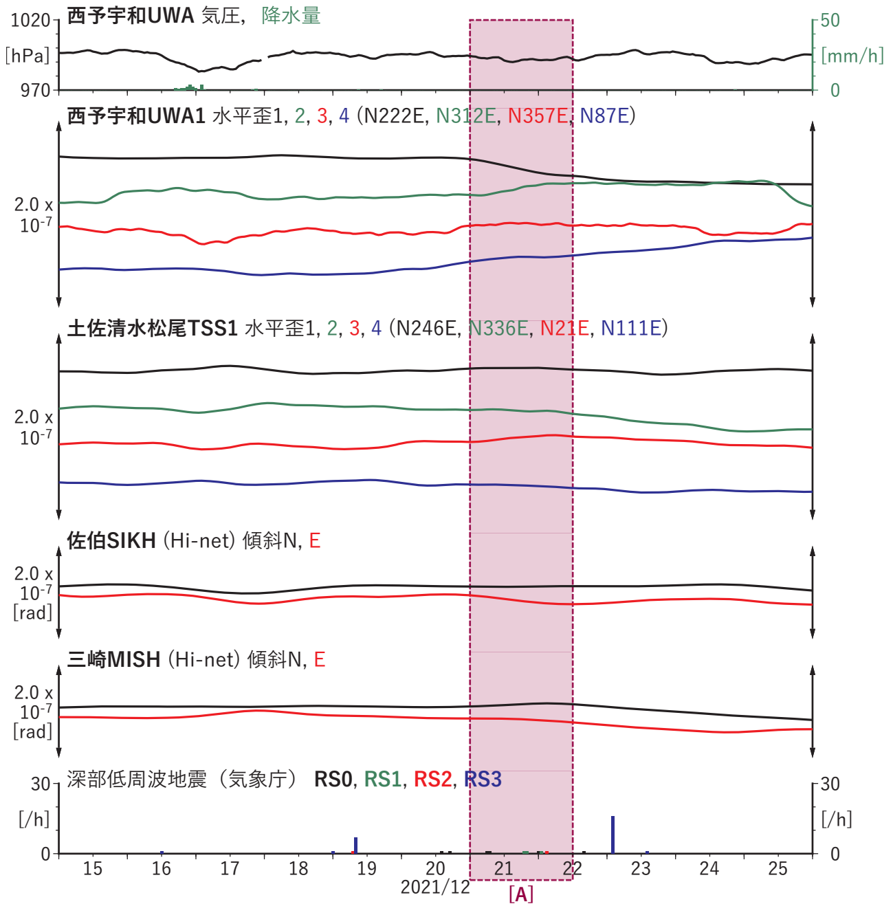
第 23 図 四国西部における歪・傾斜の観測結果と低周波地震の検出数 (2021/12/15 ~ 2021/12/25)。
