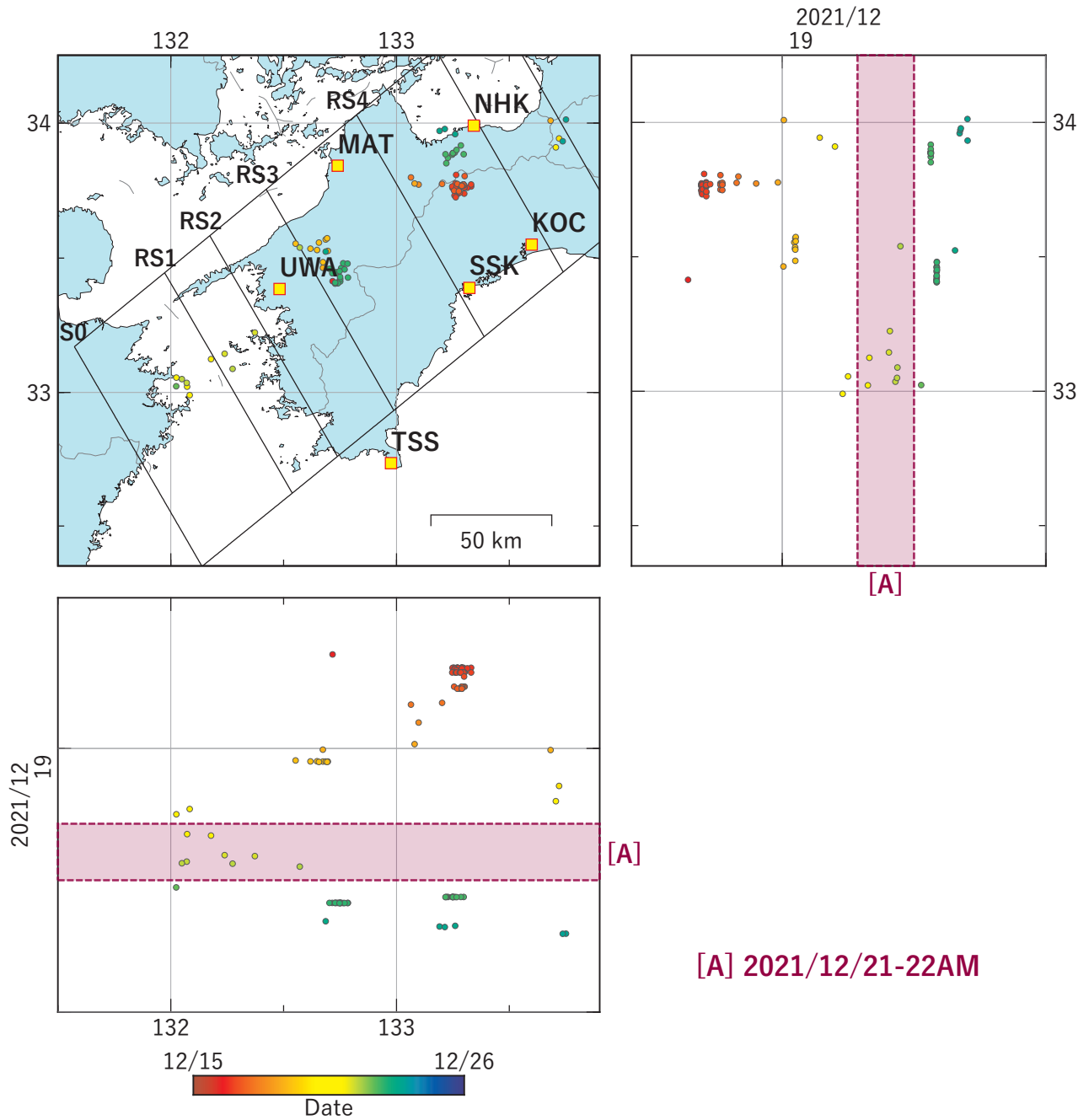
第 22 図 四国西部における低周波地震（気象庁一元化カタログによる）の時空間分布（2021/12/15 ～ 2021/12/25）. Fig. 22 Space-time distribution of low-frequency earthquakes by JMA unified hypocenter catalog in the Western Shikoku from December 15 to 25, 2021.
