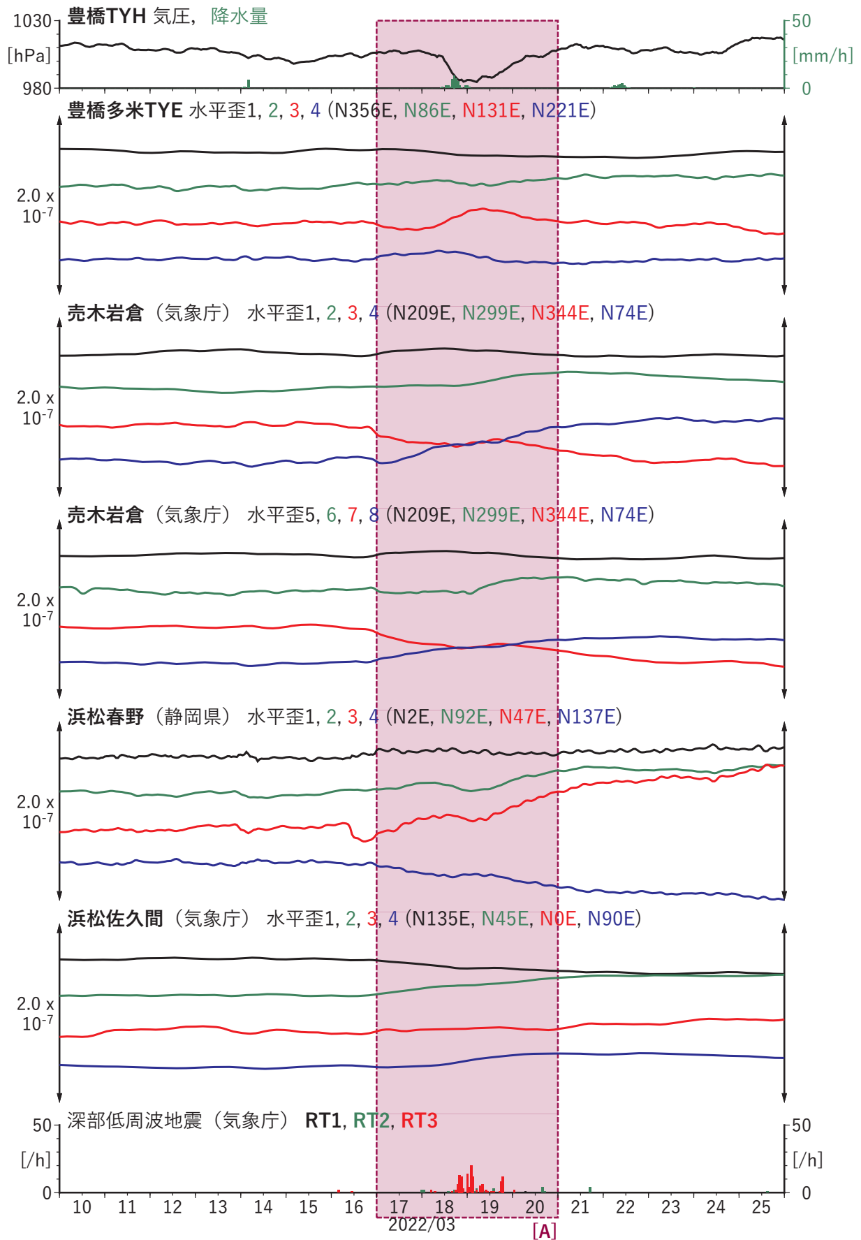
第 43 図 東海地域における歪・傾斜の観測結果と低周波地震の検出数 (2022/03/10 ~ 2022/03/25).
