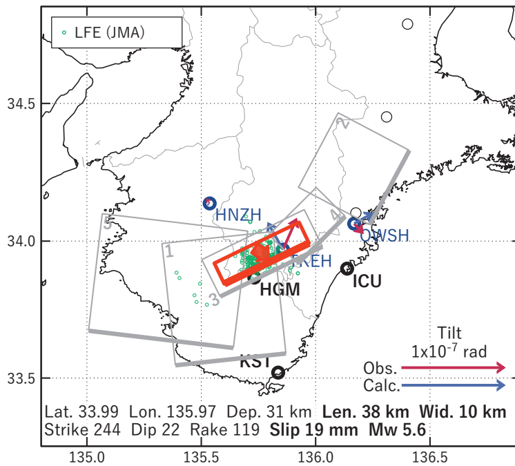
第 35 図 第 34 図 [A] を説明する断層モデル. 各図の説明は第 3 図を参照. Fig. 35 Inferred fault models for Fig. 34[A]. See also the caption of Fig. 3.
