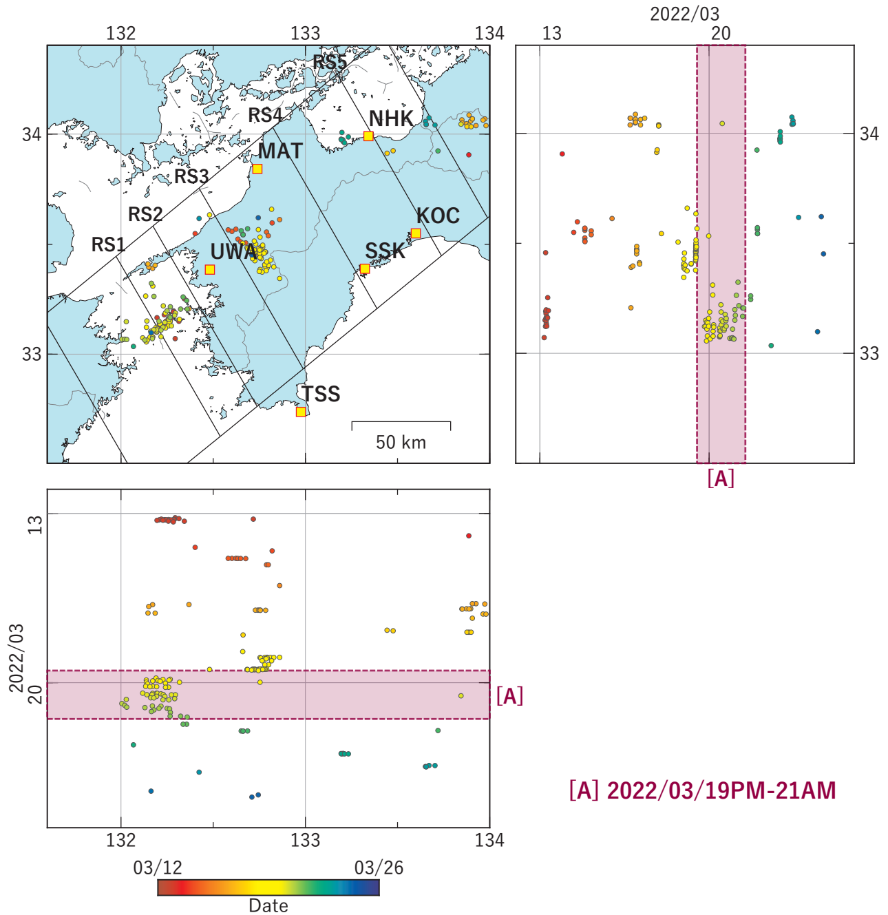
第 45 図 四国西部における低周波地震（気象庁一元化カタログによる）の時空間分布（2022/03/12 ～ 2022/03/25）. Fig. 45 Space-time distribution of low-frequency earthquakes by JMA unified hypocenter catalog in the Western Shikoku from March 12 to 25, 2022.
