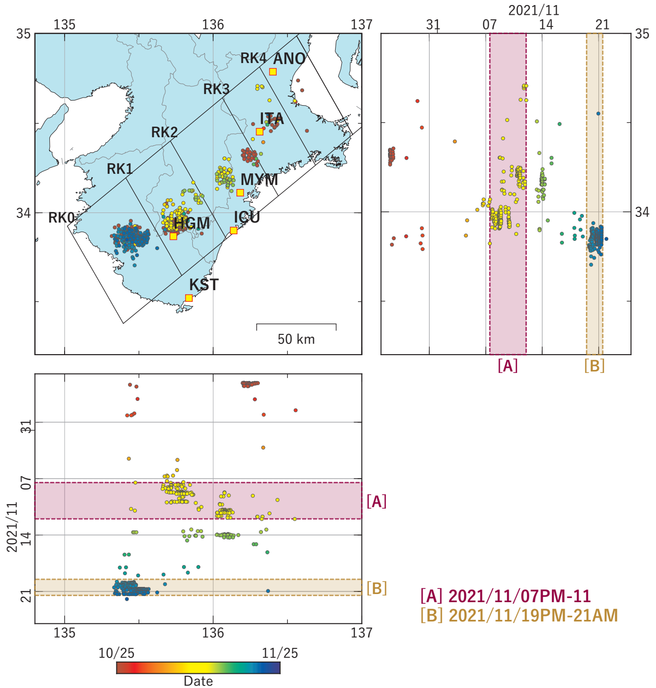
第 4 図 紀伊半島における低周波地震（気象庁一元化カタログによる）の時空間分布（2021/10/25 ～ 2021/11/24）.
