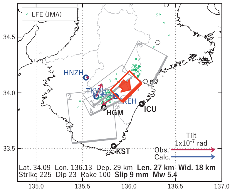
第 6 図 第 5 図 [A] を説明する断層モデル。各図の説明は第 3 図を参照。
