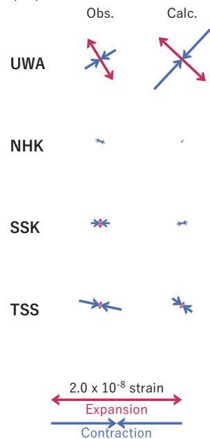
第 3 図 第 2 図 [A] を説明する断層モデル。以下の凡例の説明は以降の同様の図に共通。(図によっては気象庁・静岡県・防災科研 Hi-net の観測点や (b3) 体積歪の結果はない場合がある。) 黒・緑・青の丸印はそれぞれ産総研・気象庁および静岡県・防災科研 Hi-net の観測点。緑の小さな丸印は気象庁の推定した低周波地震。(a) 1 段階目の結果。灰色の濃淡は残差の総和で、赤色矩形が残差の総和が最小となる断層面の位置(大きさは 20x20 km で固定)。(b1) 2 段階目の結果。赤色矩形が残差の総和が最小となる断層面。矢印は傾斜の観測値と計算値の比較。灰色矩形は最近周辺で発生した短期的 SSE の推定断層面(番号との対応は本文参照)。(b2) 主歪の観測値と(b1)に示した断層モデルから求めた計算値との比較。(b3) 体積歪の観測値と(b1)に示した断層モデルから求めた計算値との比較。
