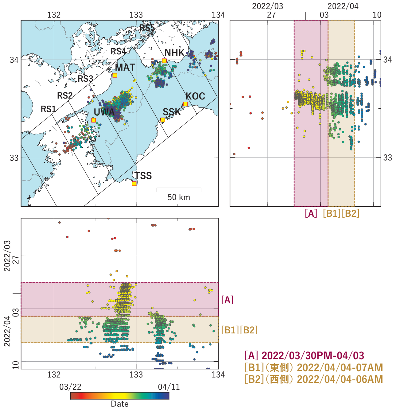
第 48 図 四国西部における低周波地震（気象庁一元化カタログによる）の時空間分布（2022/03/22 ～ 2022/04/10）. Fig. 48 Space-time distribution of low-frequency earthquakes by JMA unified hypocenter catalog in the Western Shikoku from March 22 to April 10, 2022.
