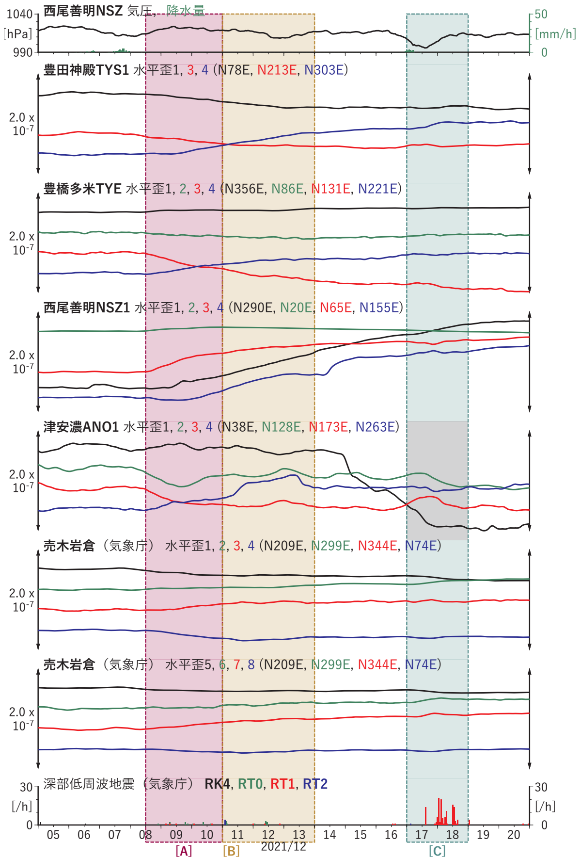
第 18 図 東海地域における歪・傾斜の観測結果と低周波地震の検出数 (2021/12/05 ~ 2021/12/20).
