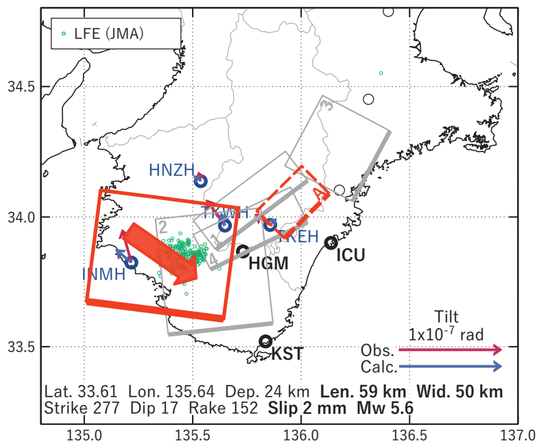
第 7 図 第 5 図 [B] を説明する断層モデル。各図の説明は第 3 図を参照。
