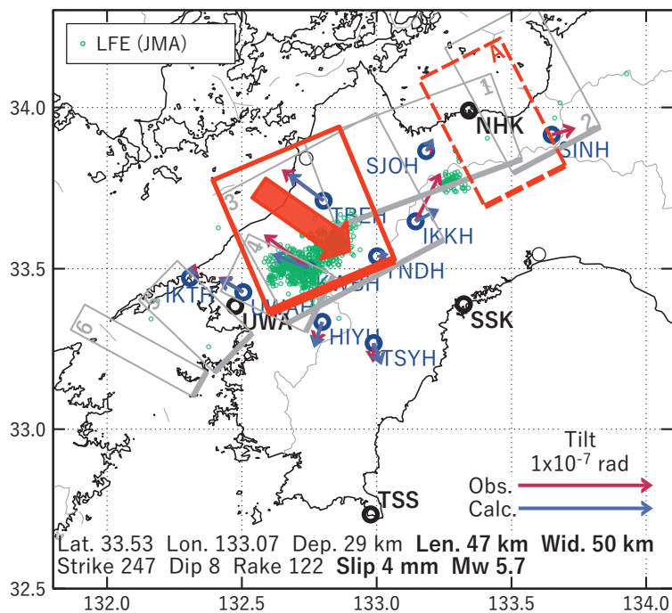
第 16 図 第 14 図 [B] を説明する断層モデル. 各図の説明は第 3 図を参照.
