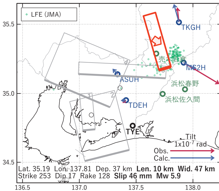
第 44 図 第 43 図 [A] を説明する断層モデル. 各図の説明は第 3 図を参照.
