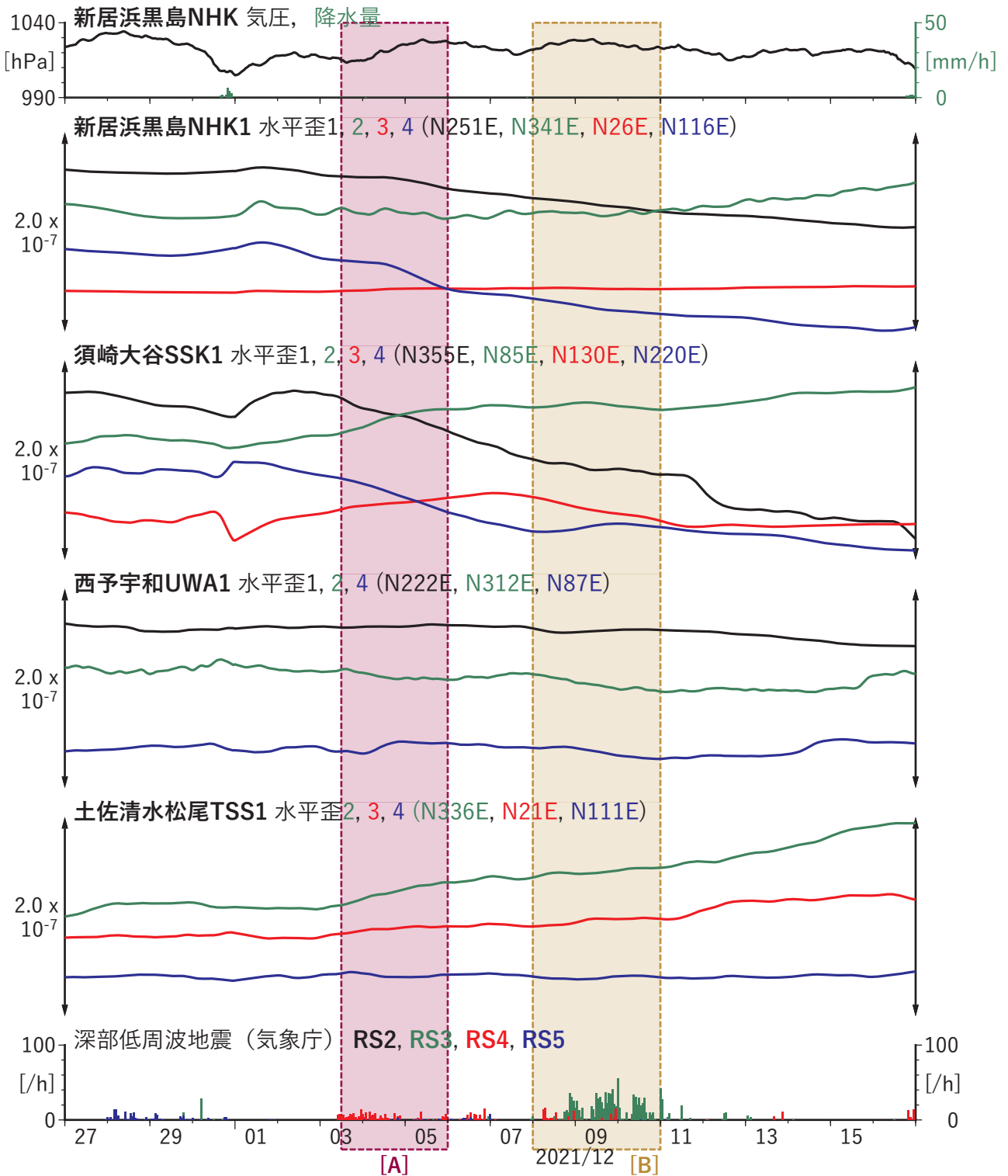
第 14 図 四国西部における歪・傾斜の観測結果と低周波地震の検出数 (2021/11/27 ~ 2021/12/16)。
