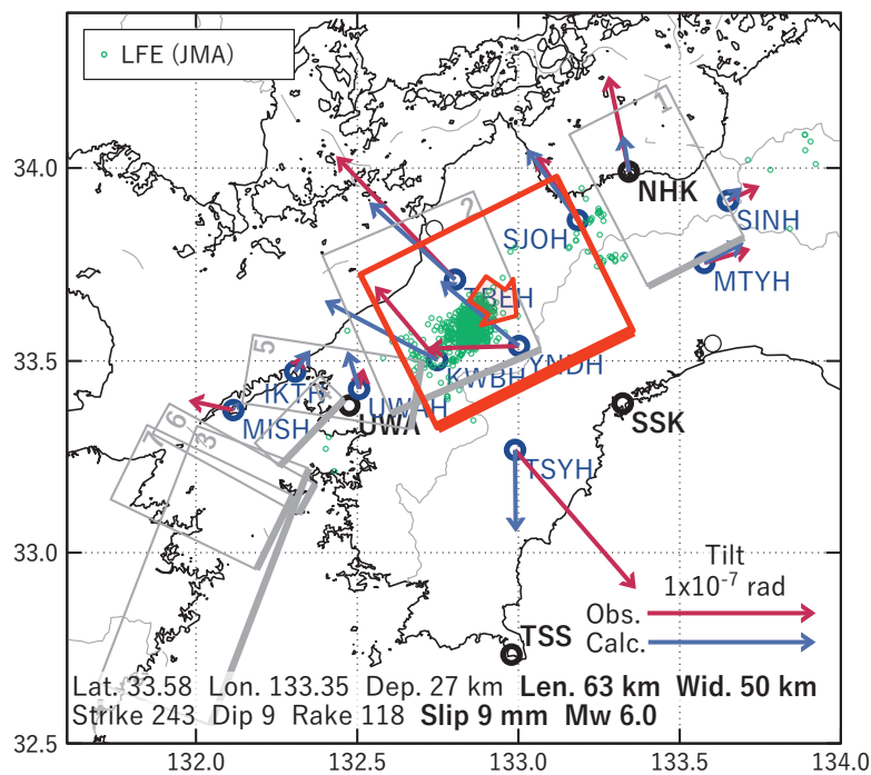
第 50 図 第 49 図 [A] を説明する断層モデル. 各図の説明は第 3 図を参照. Fig. 50 Inferred fault models for Fig. 49[A]. See also the caption of Fig. 3.
