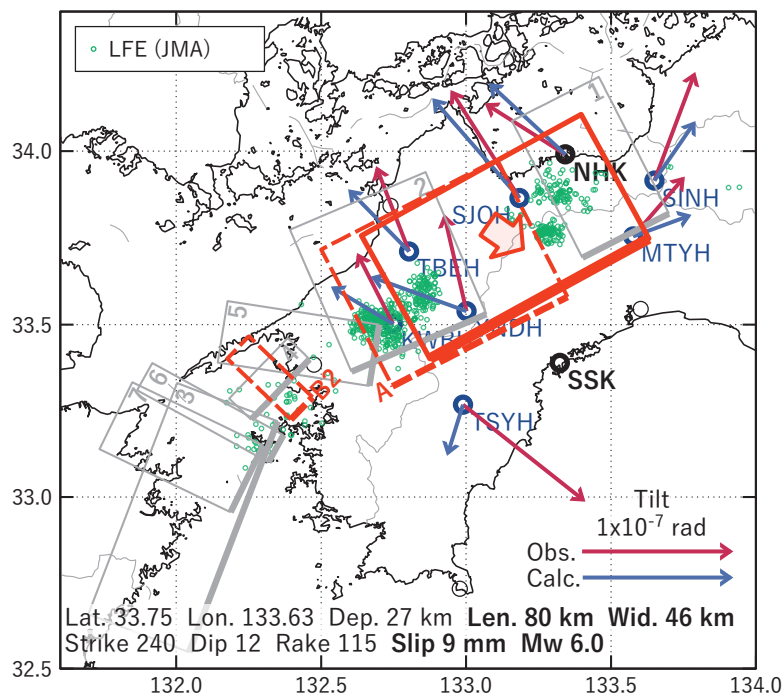
第 51 図 第 49 図 [B1] を説明する断層モデル。各図の説明は第 3 図を参照。
