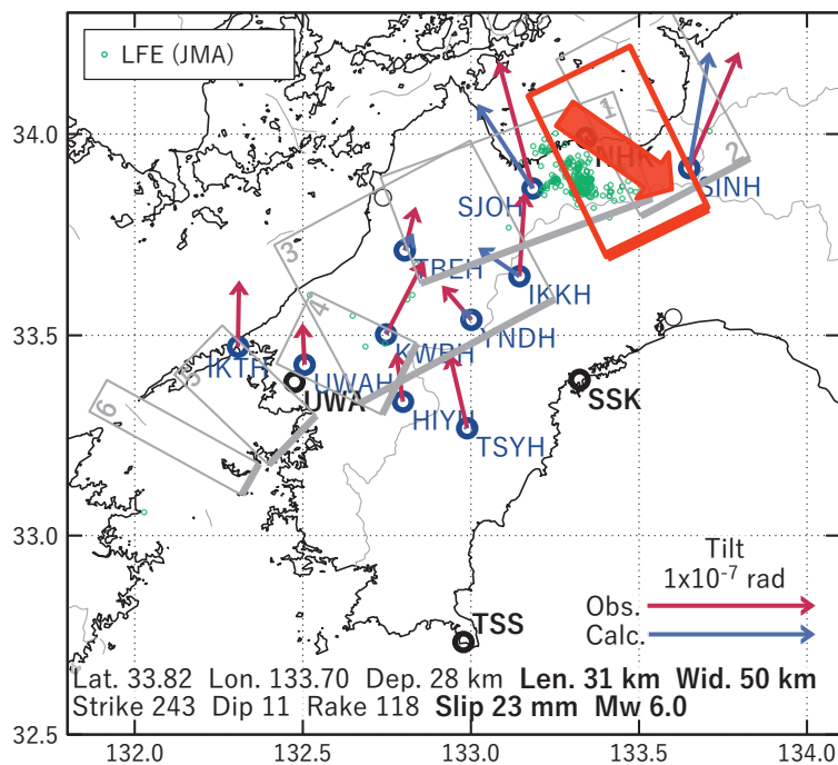
第 15 図 第 14 図 [A] を説明する断層モデル。各図の説明は第 3 図を参照。 Fig. 15 Inferred fault models for Fig. 14[A]. See also the caption of Fig. 3.
