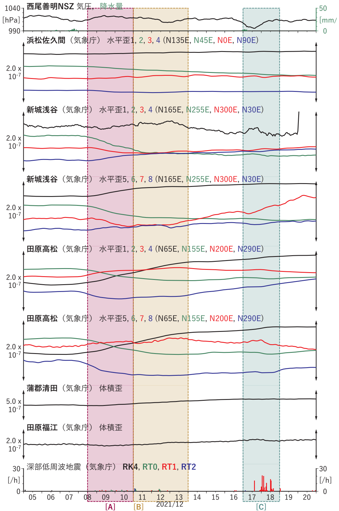
第 18 図 つづき. Fig. 18 Continued.
