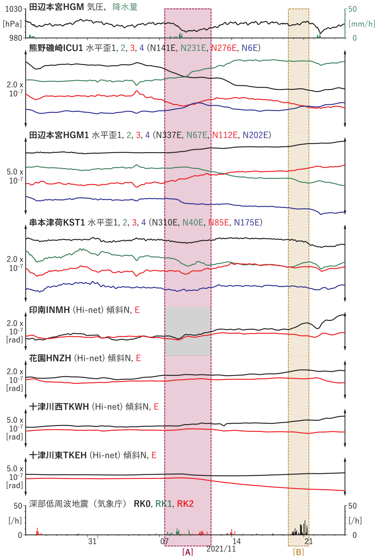
第 5 図 紀伊半島における歪・傾斜の観測結果と低周波地震の検出数 (2021/10/25 ~ 2021/11/24)。
