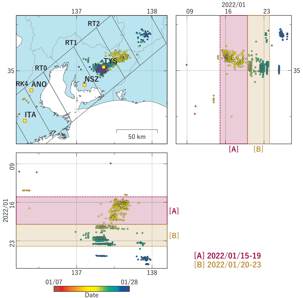
第 29 図 東海地域における低周波地震（気象庁一元化カタログによる）の時空間分布（2022/01/07 ～ 2022/01/27）. Fig. 29 Space-time distribution of low-frequency earthquakes by JMA unified hypocenter catalog in the Tokai region from January 07 to 27, 2022.
