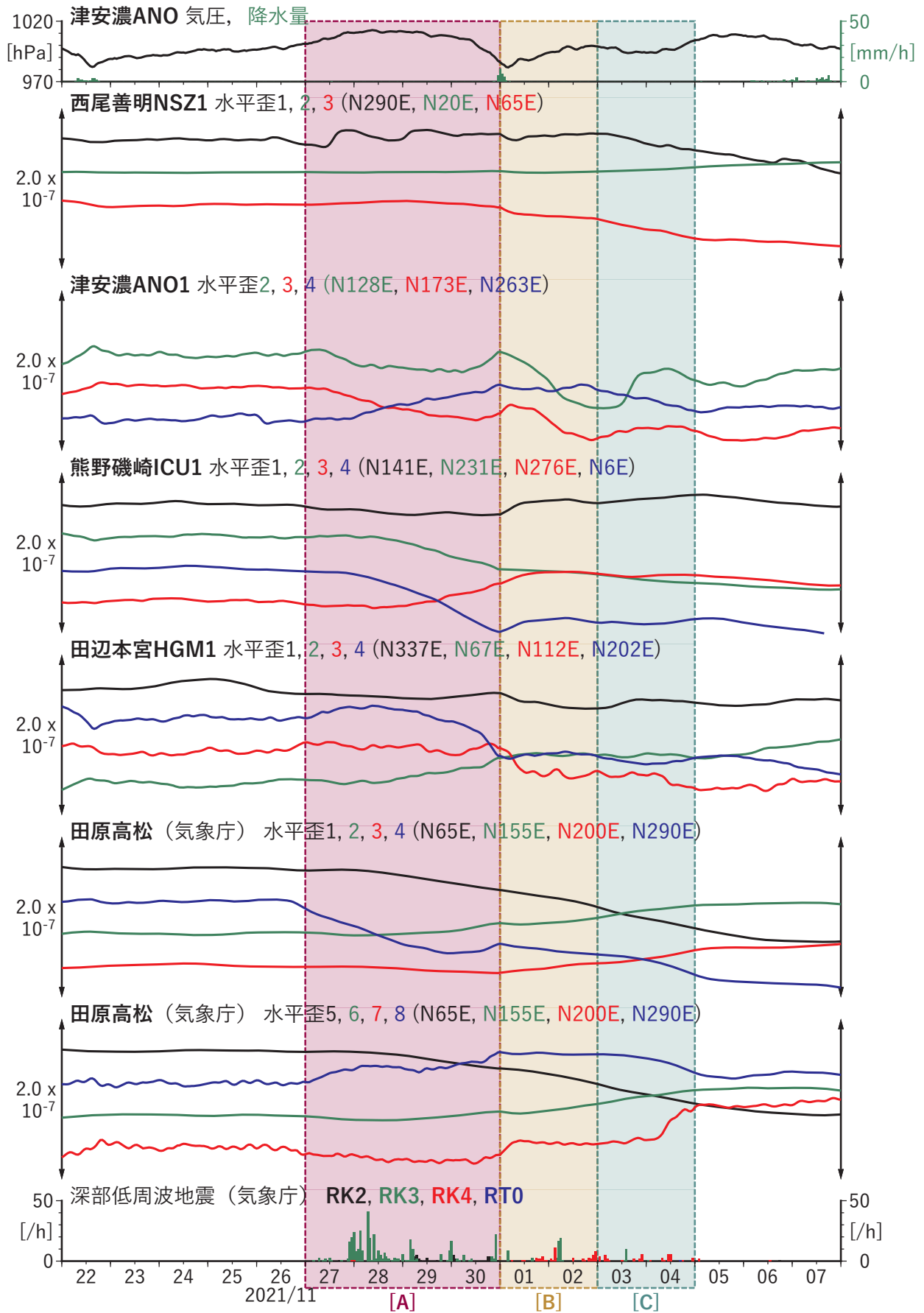
第9図 紀伊半島における歪・傾斜・地下水位の観測結果と低周波地震の検出数 (2021/11/22 ~ 2021/12/07)。
