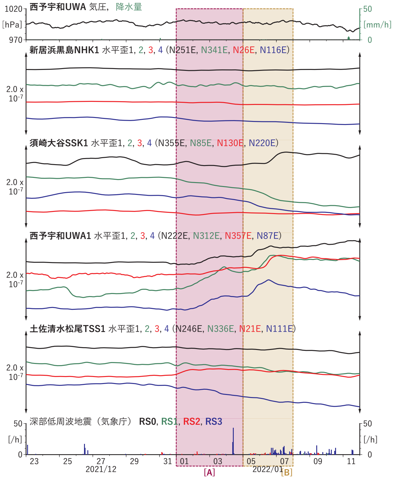
第 26 図 四国西部における歪・傾斜の観測結果と低周波地震の検出数（2021/12/23 ～ 2022/01/11）。
