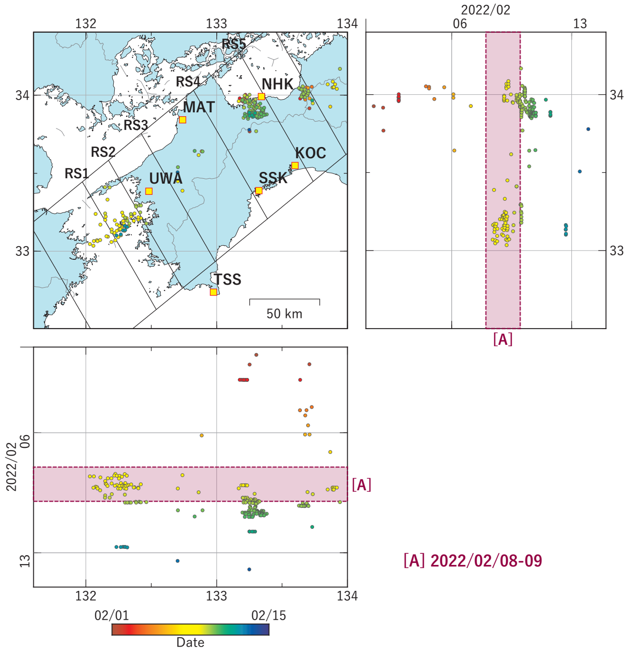
第 36 図 四国西部における低周波地震（気象庁一元化カタログによる）の時空間分布（2022/02/01 ～ 2022/02/14）. Fig. 36 Space-time distribution of low-frequency earthquakes by JMA unified hypocenter catalog in the Western Shikoku from February 01 to 14, 2022.
