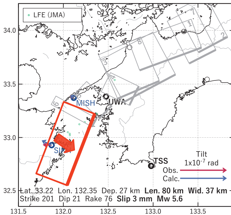
第 24 図 第 23 図 [A] を説明する断層モデル。各図の説明は第 3 図を参照。 Fig. 24 Inferred fault models for Fig. 23[A]. See also the caption of Fig. 3.
