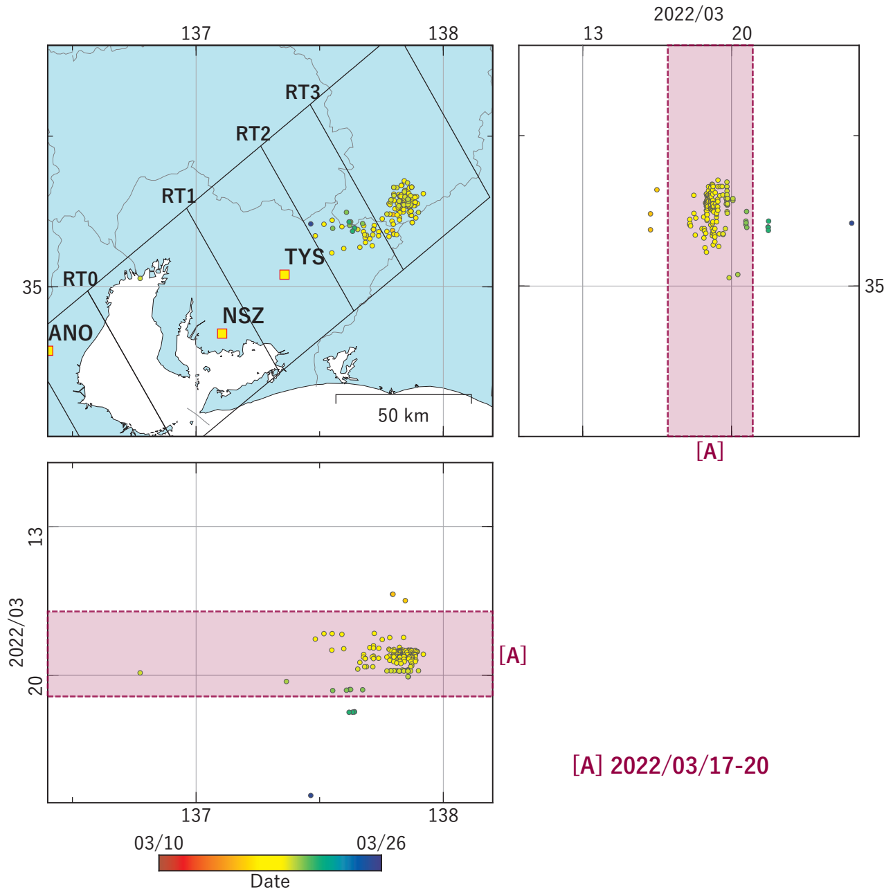
第 42 図 東海地域における低周波地震（気象庁一元化カタログによる）の時空間分布（2022/03/10 ～ 2022/03/25）. Fig. 42 Space-time distribution of low-frequency earthquakes by JMA unified hypocenter catalog in the Tokai region from March 10 to 25, 2022.
