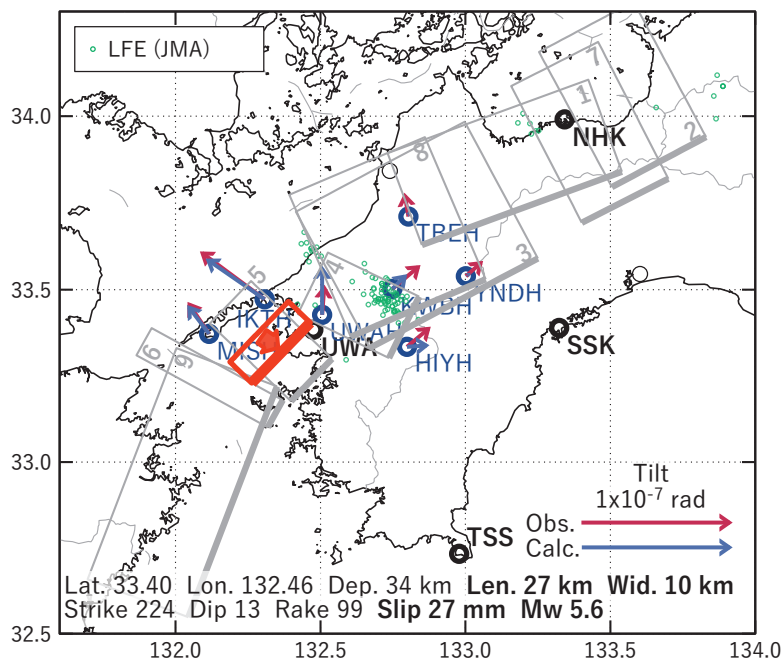
第 27 図 第 26 図 [A] を説明する断層モデル。各図の説明は第 3 図を参照。
