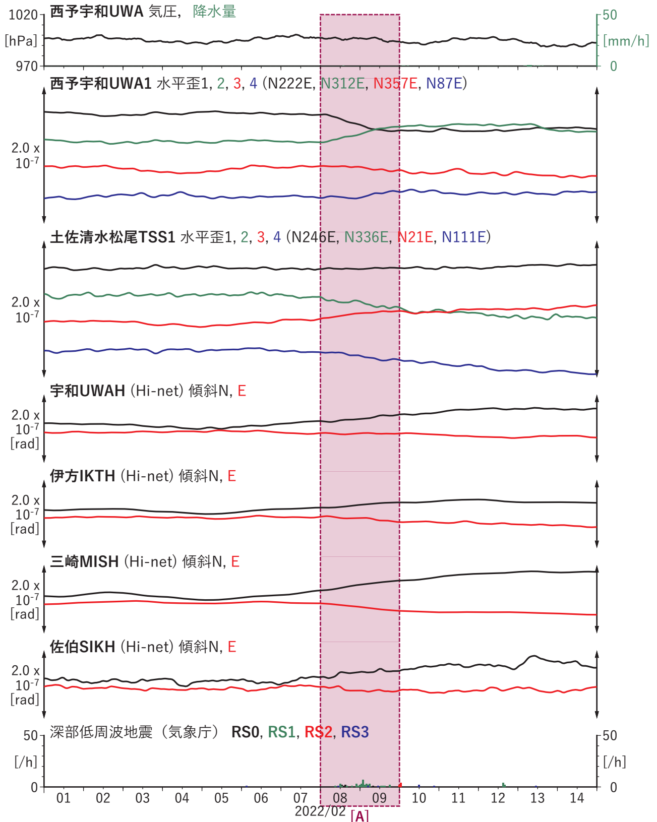
第 37 図 四国西部における歪・傾斜の観測結果と低周波地震の検出数 (2022/02/01 ~ 2022/02/14).
