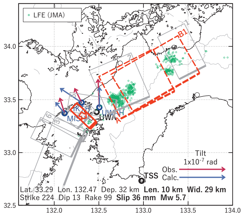
第 52 図 第 49 図 [B2] を説明する断層モデル。各図の説明は第 3 図を参照。 Fig. 52 Inferred fault models for Fig. 49[B2]. See also the caption of Fig. 3.
