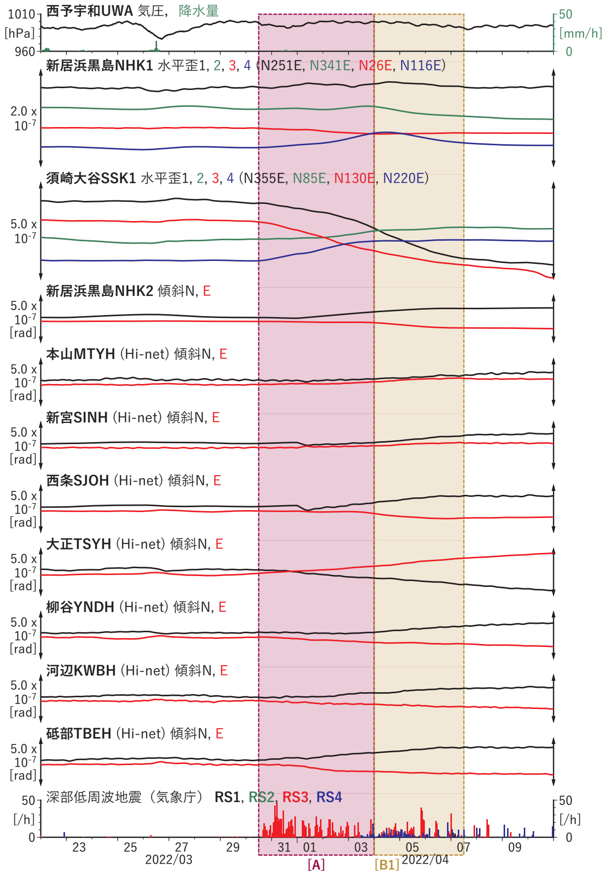
第 49 図 四国西部における歪・傾斜の観測結果と低周波地震の検出数 (2022/03/22 ~ 2022/04/10)。
