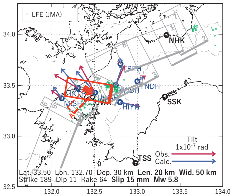
第 28 図 第 26 図 [B] を説明する断層モデル。各図の説明は第 3 図を参照。
