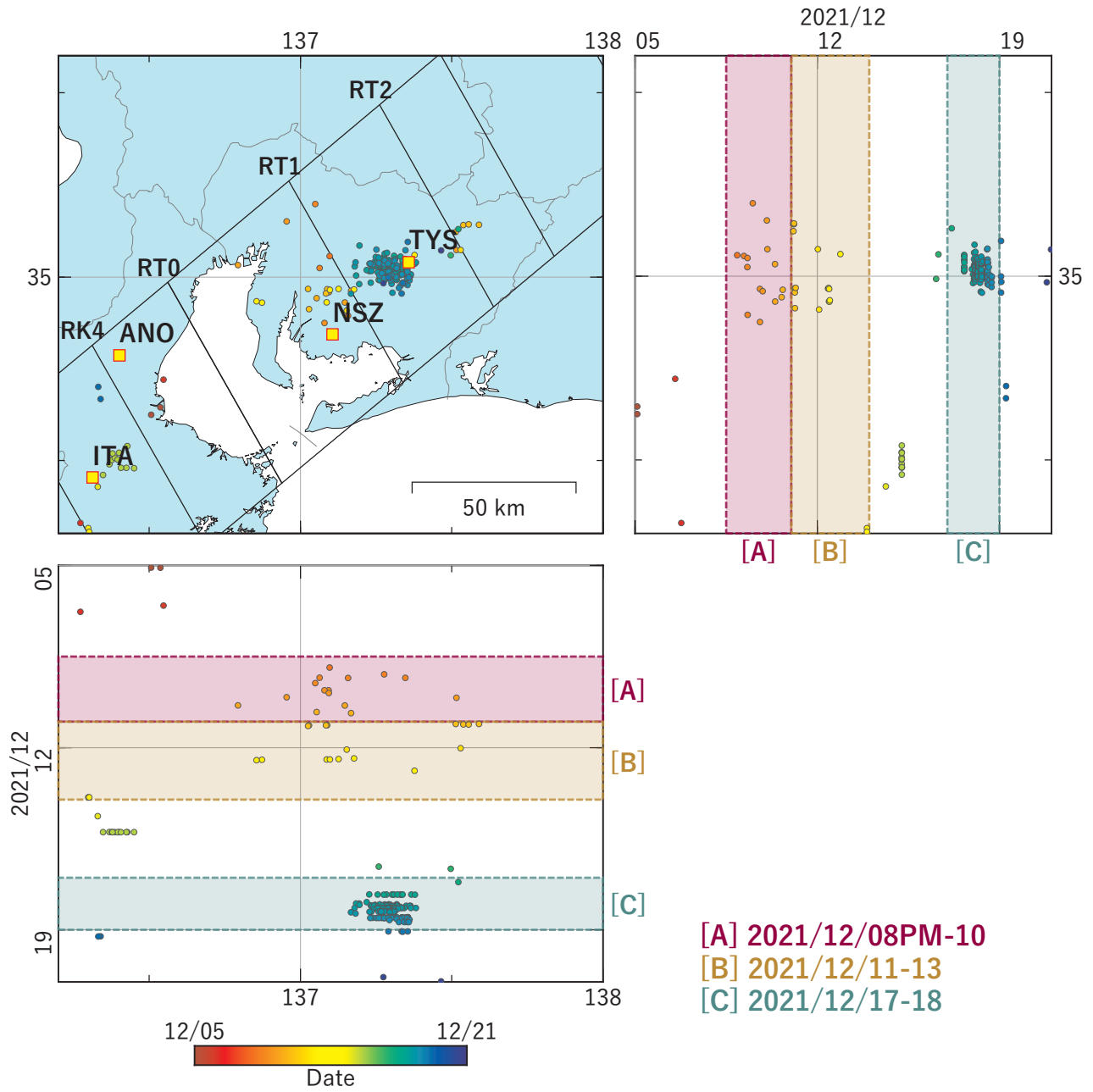
第 17 図 東海地域における低周波地震（気象庁一元化カタログによる）の時空間分布（2021/12/05 ～ 2021/12/20）. Fig. 17 Space-time distribution of low-frequency earthquakes by JMA unified hypocenter catalog in the Tokai region from December 05 to 20, 2021.
