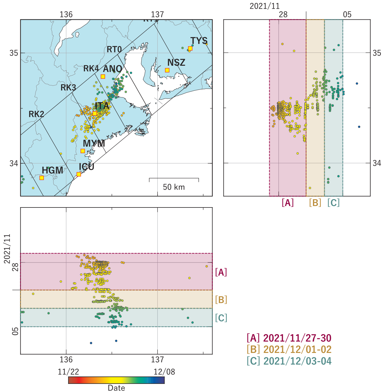
第 8 図 紀伊半島における低周波地震（気象庁一元化カタログによる）の時空間分布（2021/11/22 ～ 2021/12/07）。
