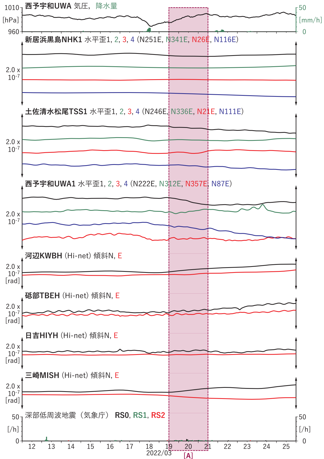
第 46 図 四国西部における歪・傾斜の観測結果と低周波地震の検出数 (2022/03/12 ~ 2022/03/25)。
