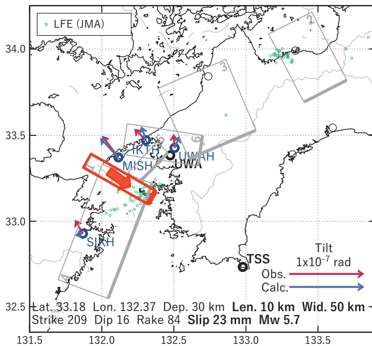
第 38 図 第 37 図 [A] を説明する断層モデル。各図の説明は第 3 図を参照。 Fig. 38 Inferred fault models for Fig. 37[A]. See also the caption of Fig. 3.
