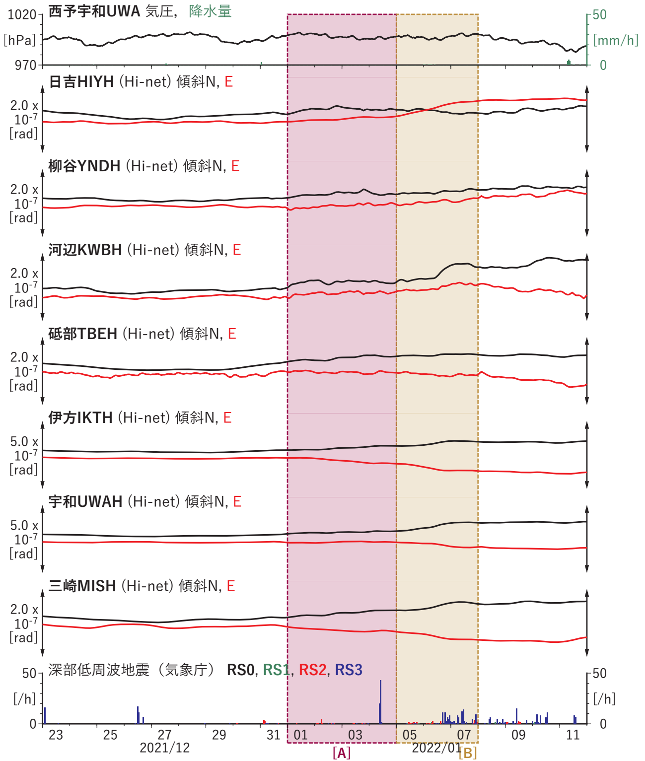
第 26 図 つづき. Fig. 26 Continued.
