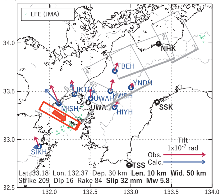
第 3 図 第 2 図 [A] を説明する断層モデル。以下の凡例の説明は以降の同様の図に共通。(図によっては気象庁・静岡県・防災科研 Hi-net の観測点や (b3) 体積歪の結果はない場合がある。) 黒・緑・青の丸印はそれぞれ産総研・気象庁および静岡県・防災科研 Hi-net の観測点。緑の小さな丸印は気象庁の推定した低周波地震。(a) 1 段階目の結果。灰色の濃淡は残差の総和で、赤色矩形が残差の総和が最小となる断層面の位置(大きさは 20x20 km で固定)。(b1) 2 段階目の結果。赤色矩形が残差の総和が最小となる断層面。矢印は傾斜の観測値と計算値の比較。灰色矩形は最近周辺で発生した短期的 SSE の推定断層面(番号との対応は本文参照)。(b2) 主歪の観測値と(b1)に示した断層モデルから求めた計算値との比較。(b3) 体積歪の観測値と(b1)に示した断層モデルから求めた計算値との比較。
