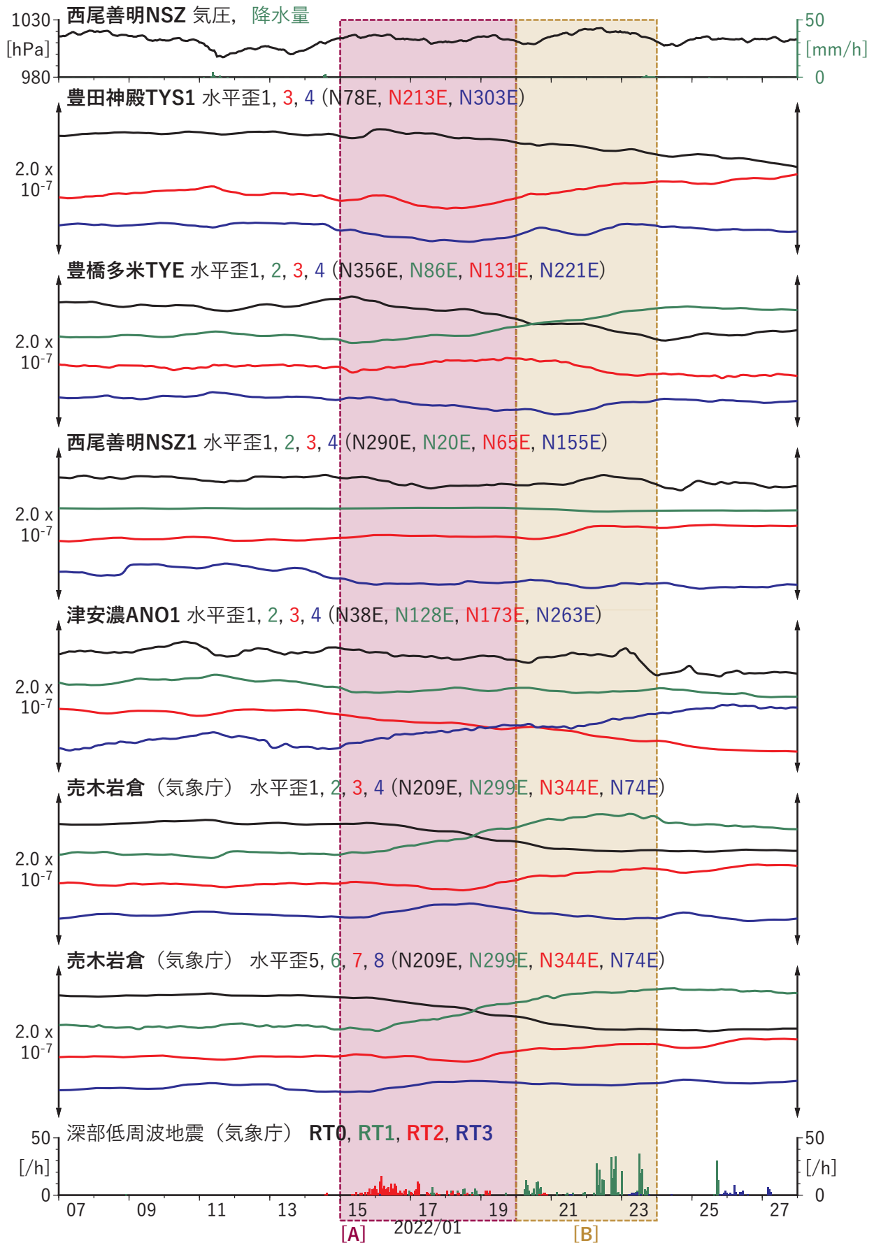
第 30 図 東海地域における歪・傾斜の観測結果と低周波地震の検出数 (2022/01/07 ~ 2022/01/27)。
