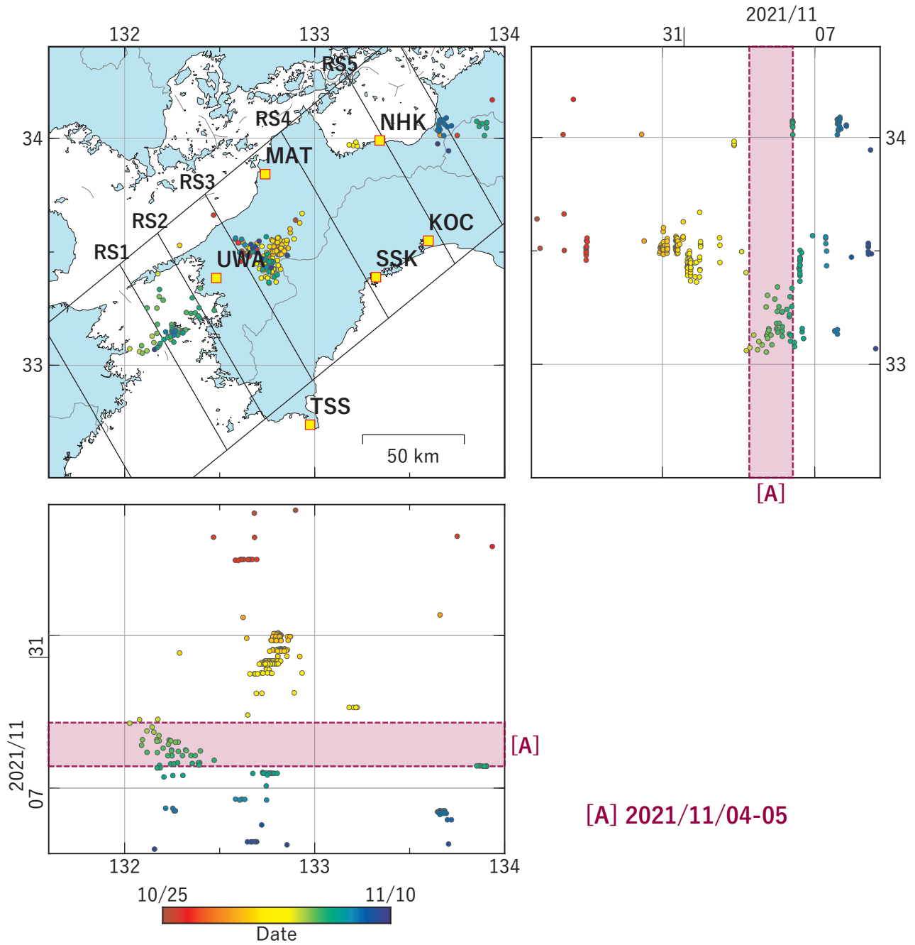
第 1 図 四国西部における低周波地震（気象庁一元化カタログによる）の時空間分布（2021/10/25 ～ 2021/11/09）。
