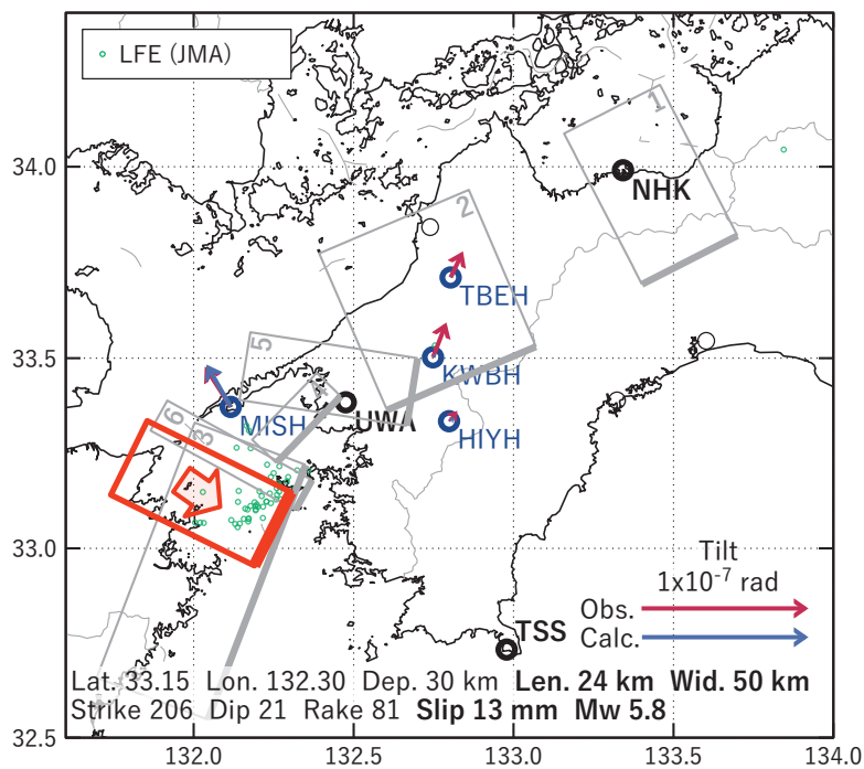
第 47 図 第 46 図 [A] を説明する断層モデル。各図の説明は第 3 図を参照。
