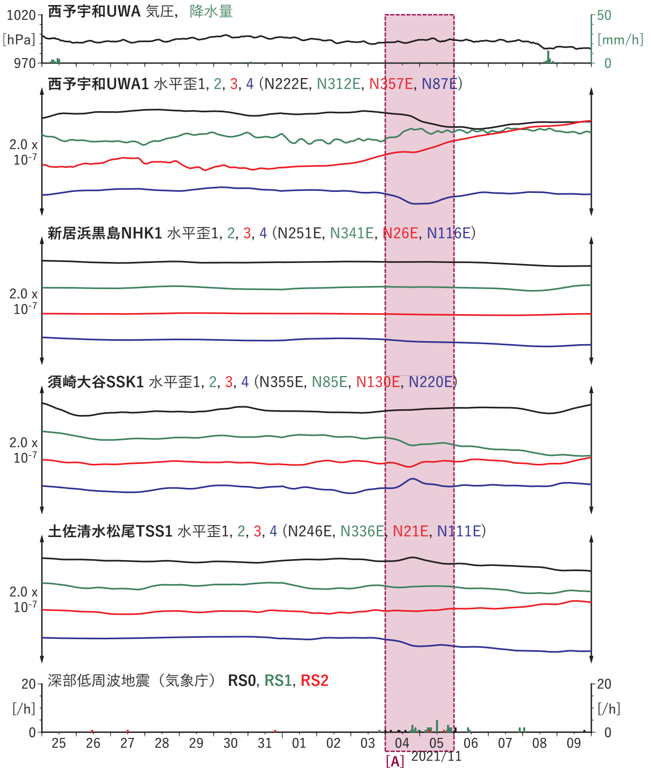
第 2 図 四国西部における歪・傾斜の観測結果と低周波地震の検出数 (2021/10/25 ~ 2021/11/09)。
