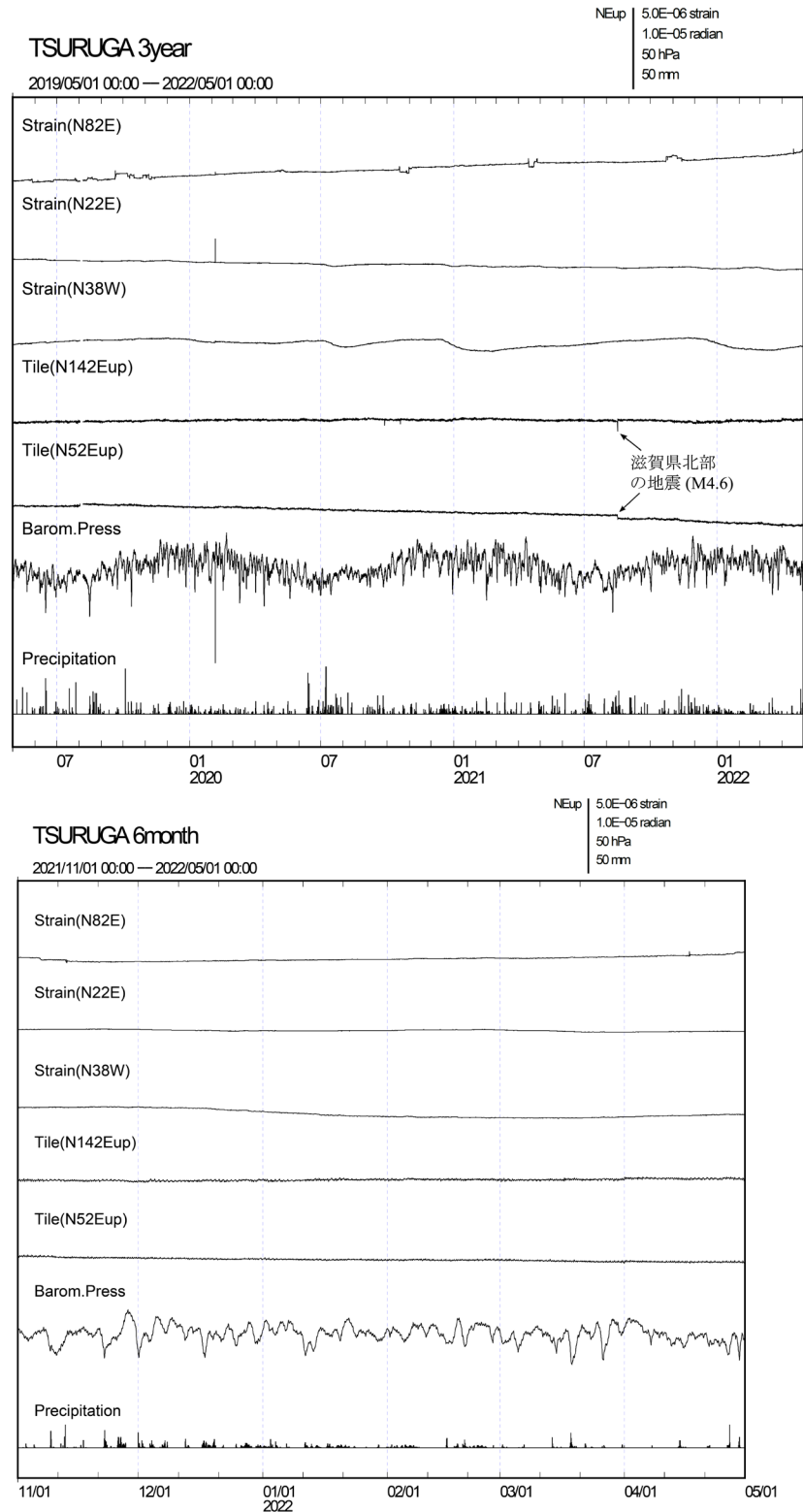
第 3 図 敦賀観測点における (上) 2019 年 5 月～2022 年 4 月, (下) 2021 年 11 月～2022 年 4 月のひずみ・傾斜変化 (時間値)。
