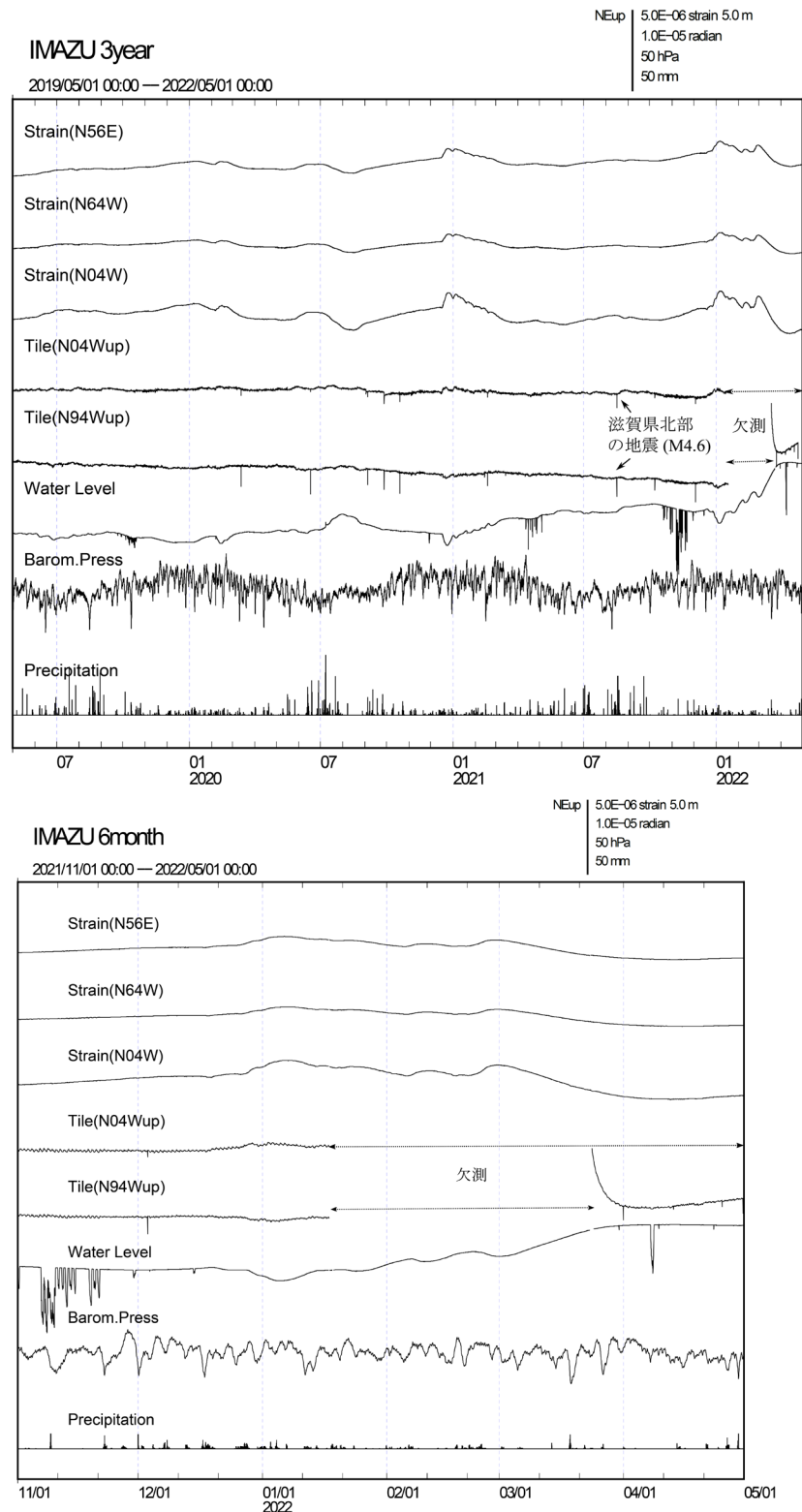
第 2 図 今津観測点における (上) 2019 年 5 月～2022 年 4 月, (下) 2021 年 11 月～2022 年 4 月のひずみ・傾斜変化 (時間値)。毎年冬のひずみ・水位変化は、観測点付近の融雪のための地下水汲み上げに伴うもの。
