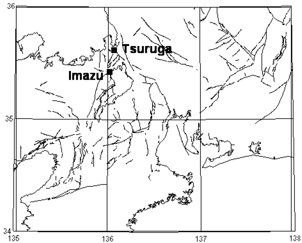
第 1 図 今津・敦賀観測点の位置. 図中の線は活断層研究会 (1991) 4) による活断層の位置.
