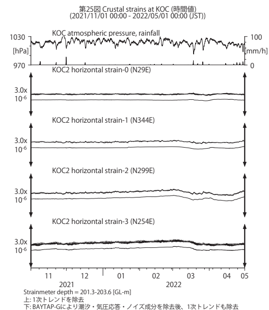
第 25 図 KOC における歪観測結果 (2021 年 11 月～2022 年 4 月)。
