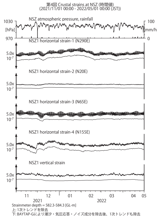
第4図 NSZにおける歪観測結果(2021年11月～2022年4月)。
