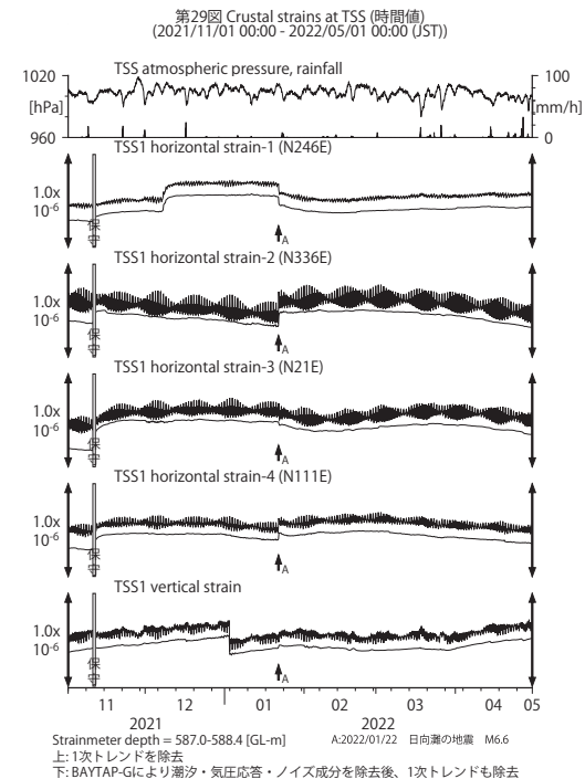
第 29 図 TSS における歪観測結果 (2021 年 11 月～2022 年 4 月)。
