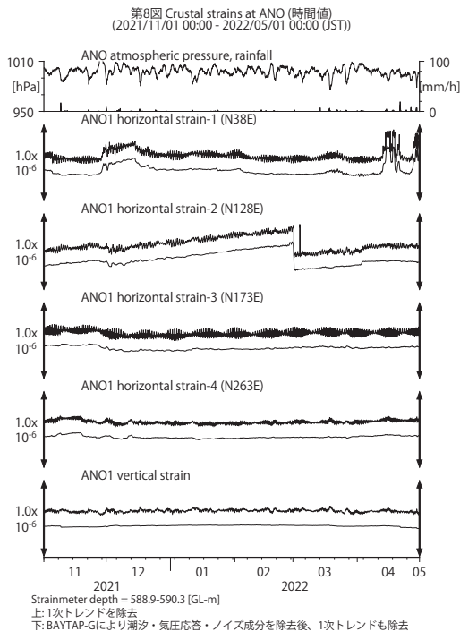
第 8 図 ANO における歪観測結果 (2021 年 11 月～2022 年 4 月)。
