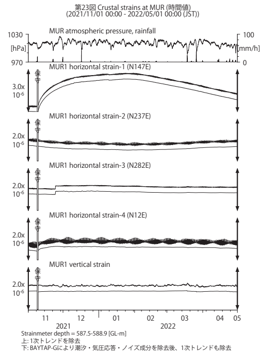
第 23 図 MUR における歪観測結果 (2021 年 11 月～2022 年 4 月)。
