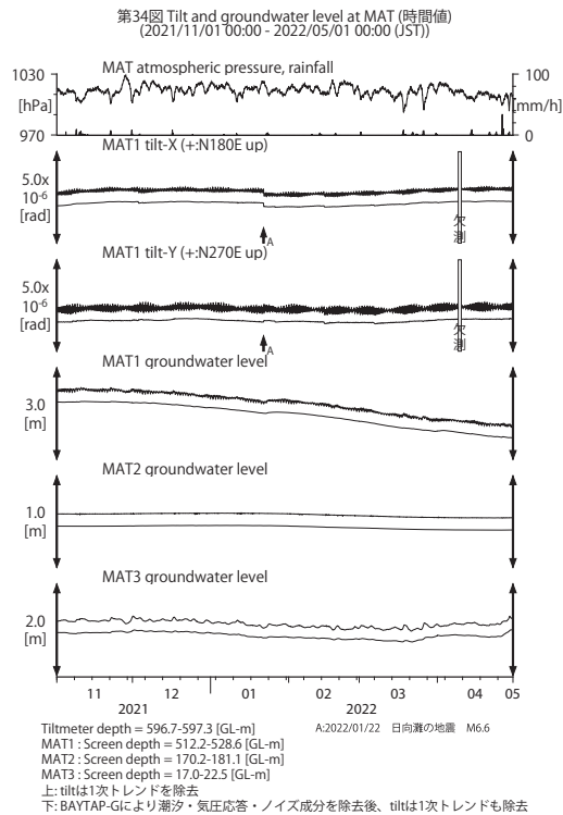
第 34 図 MAT における傾斜・地下水位観測結果 (2021 年 11 月～2022 年 4 月)。
