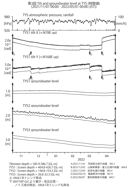
第3図 TYSにおける傾斜・地下水位観測結果(2021年11月～2022年4月)。
