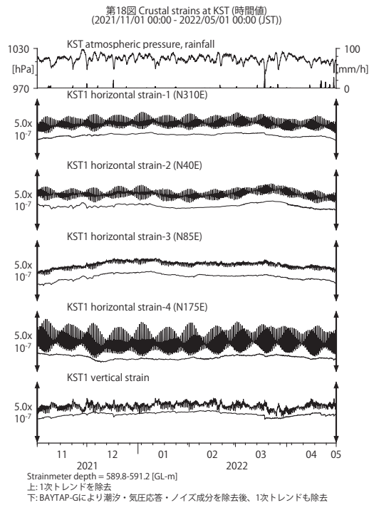
第 18 図 KST における歪観測結果 (2021 年 11 月 ~ 2022 年 4 月)。
