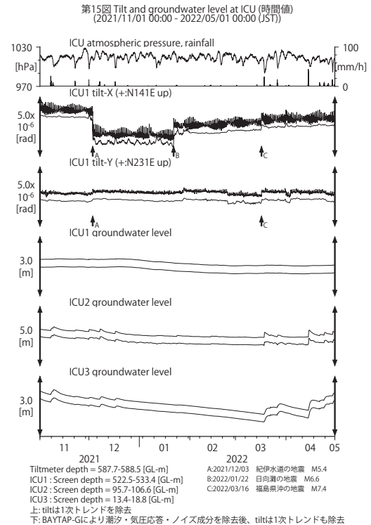
第 15 図 ICU における傾斜・地下水位観測結果 (2021 年 11 月～2022 年 4 月)。
