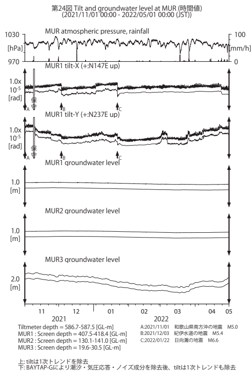
第 24 図 MUR における傾斜・地下水位観測結果 (2021 年 11 月～2022 年 4 月)。
