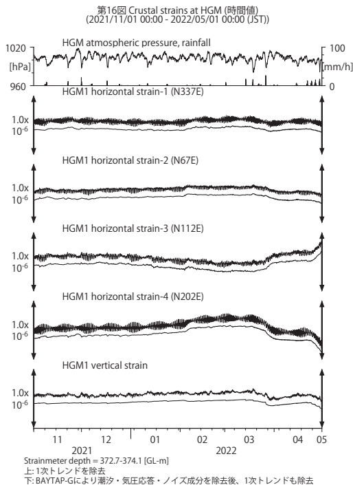
第 16 図 HGM における歪観測結果 (2021 年 11 月～2022 年 4 月)。
