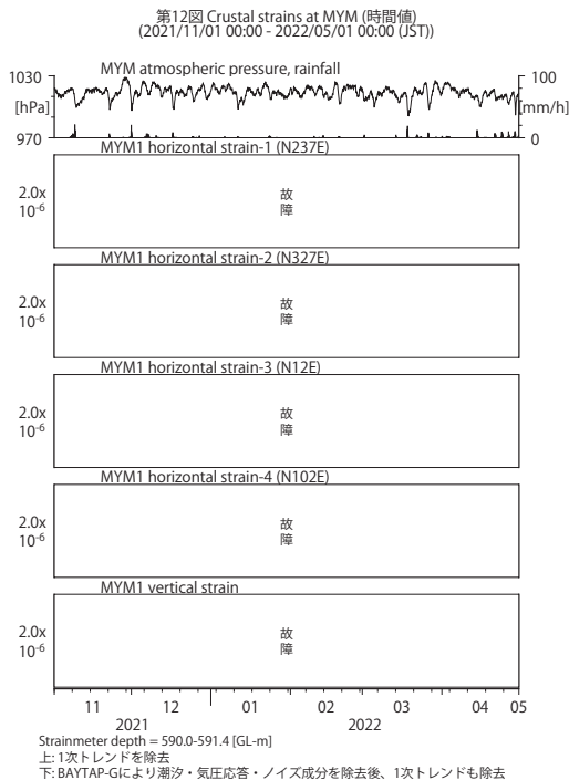
第 12 図 MYM における歪観測結果 (2021 年 11 月～2022 年 4 月)。
