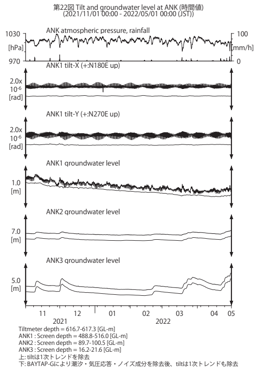
第 22 図 ANK における傾斜・地下水位観測結果 (2021 年 11 月～2022 年 4 月)。
