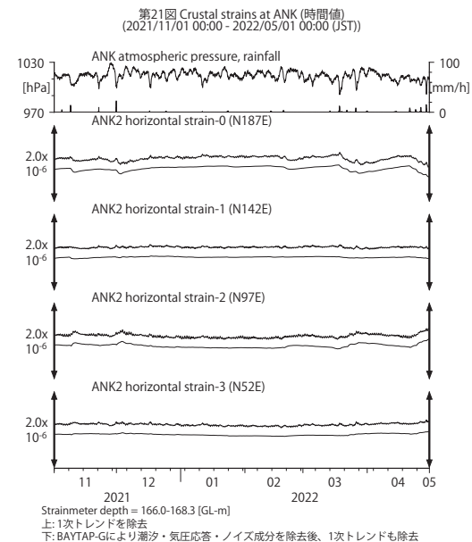
第 21 図 ANK における歪観測結果 (2021 年 11 月 ~ 2022 年 4 月)。
