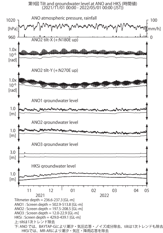
第 9 図 ANO および HKS における傾斜・地下水位観測結果 (2021 年 11 月～2022 年 4 月)。
