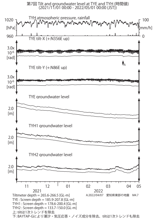
第 7 図 TYE および TYH における傾斜・地下水位観測結果 (2021 年 11 月～2022 年 4 月)。
