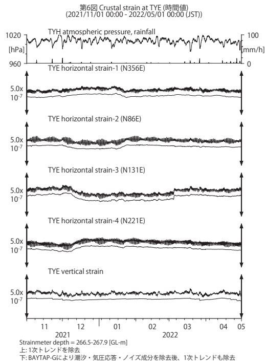
第 6 図 TYE における歪観測結果 (2021 年 11 月～2022 年 4 月)。
