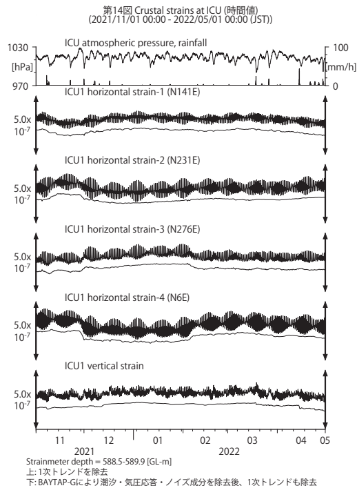
第 14 図 ICU における歪観測結果 (2021 年 11 月～2022 年 4 月)。
