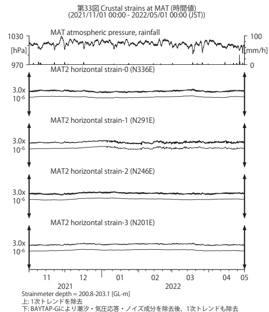
第 33 図 MAT における歪観測結果 (2021 年 11 月～2022 年 4 月)。
