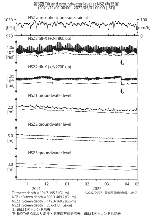
第5図 NSZにおける傾斜・地下水位観測結果(2021年11月～2022年4月)。
