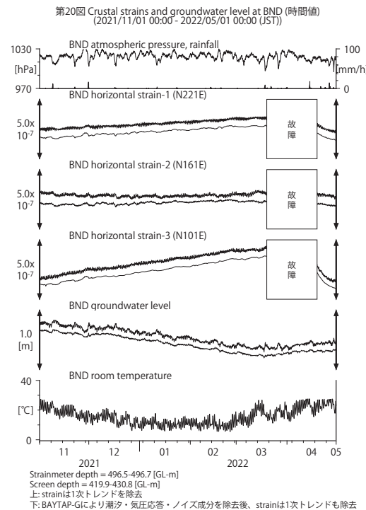
第 20 図 BND における歪・地下水位観測結果 (2021 年 11 月 ~ 2022 年 4 月)。
