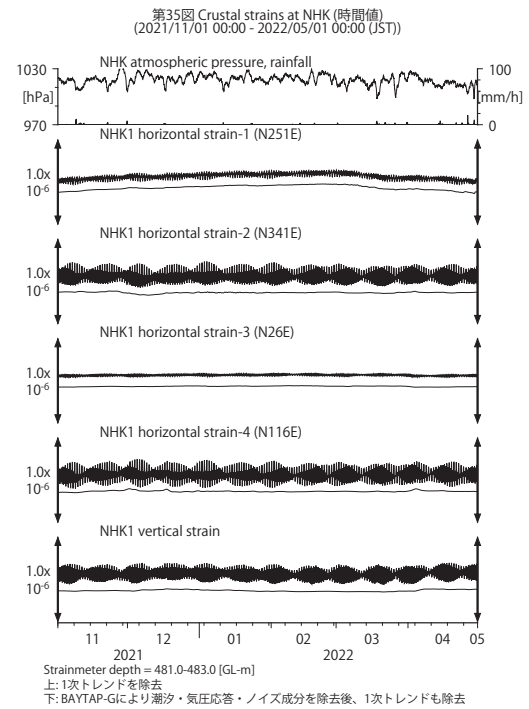
第 35 図 NHK における歪観測結果 (2021 年 11 月～2022 年 4 月)。
