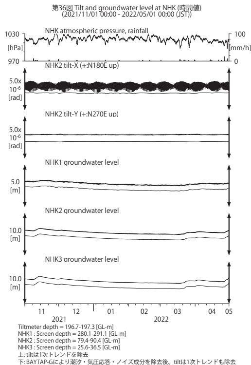
第 36 図 NHK における傾斜・地下水位観測結果 (2021 年 11 月～2022 年 4 月)。
