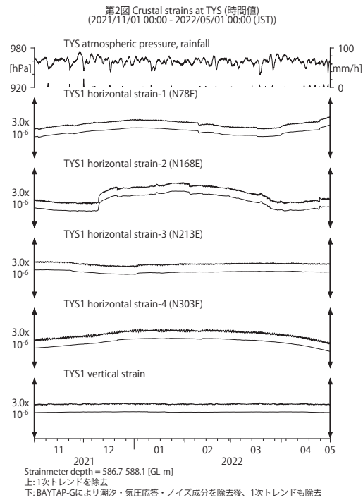
第2図 TYSにおける歪観測結果(2021年11月～2022年4月)。
