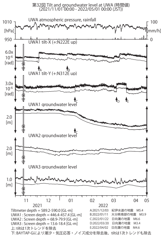
第 32 図 UWA における傾斜・地下水位観測結果 (2021 年 11 月～2022 年 4 月)。
