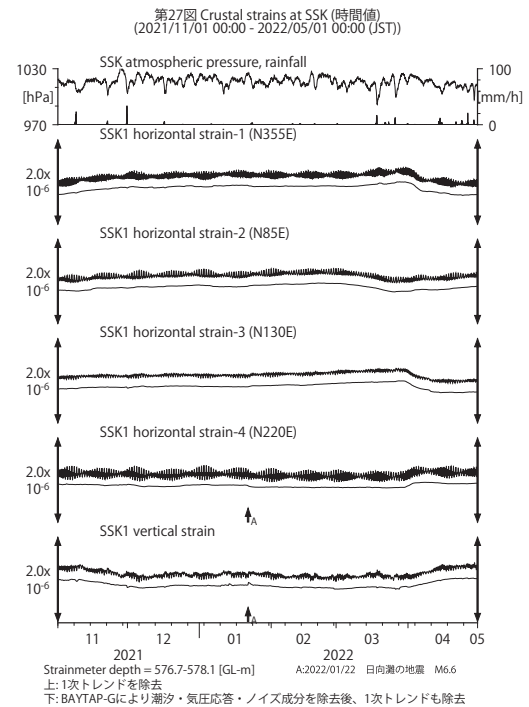
第 27 図 SSK における歪観測結果 (2021 年 11 月～2022 年 4 月)。
