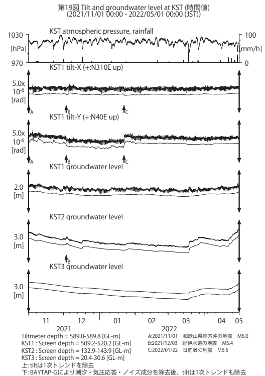
第 19 図 KST における傾斜・地下水位観測結果 (2021 年 11 月 ~ 2022 年 4 月)。
