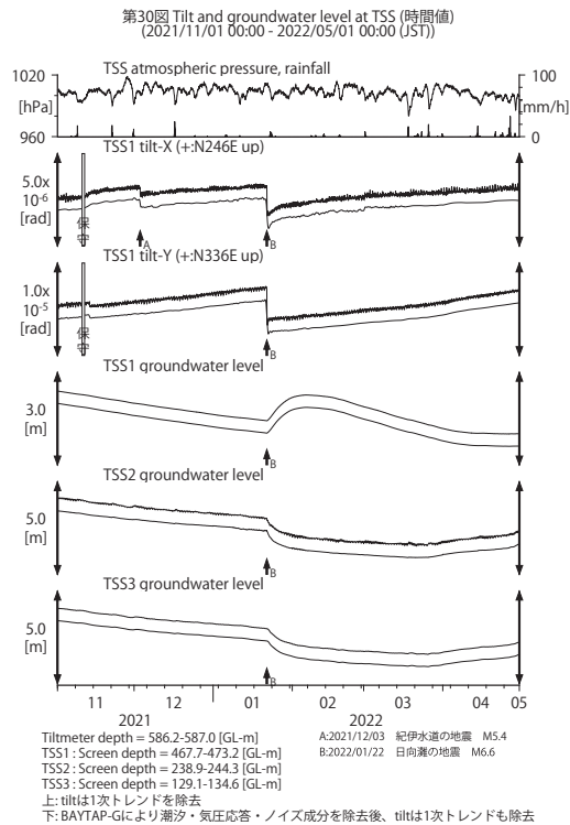
第 30 図 TSS における傾斜・地下水位観測結果 (2021 年 11 月～2022 年 4 月)。
