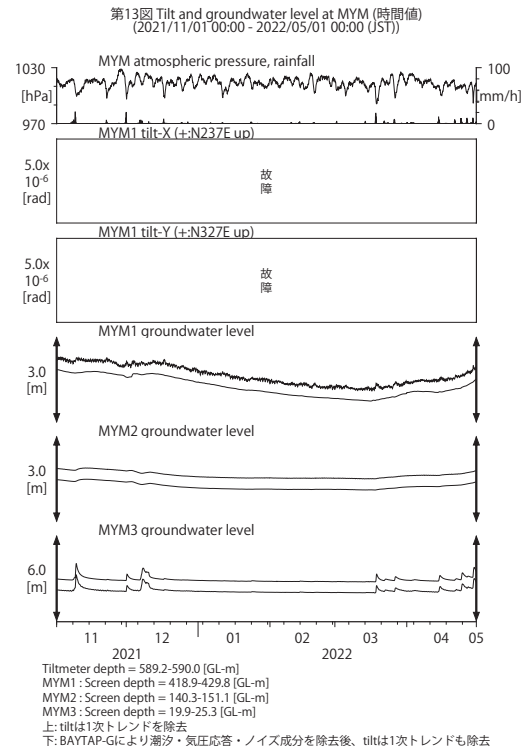
第 13 図 MYM における傾斜・地下水位観測結果 (2021 年 11 月～2022 年 4 月)。
