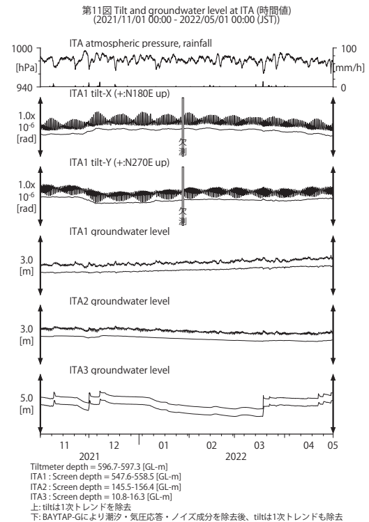
第 11 図 ITA における傾斜・地下水位観測結果 (2021 年 11 月～2022 年 4 月)。
