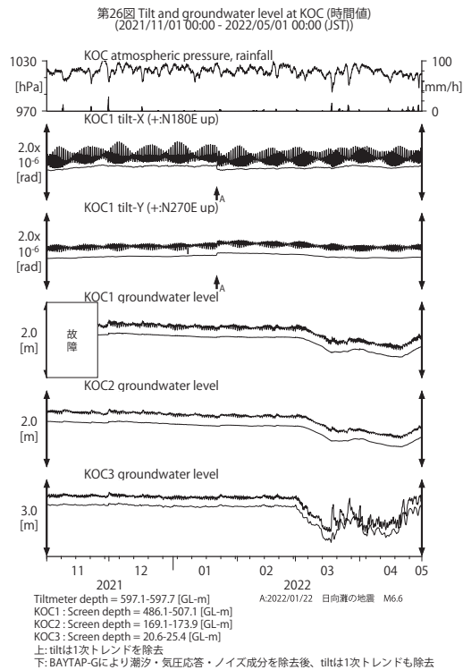
第 26 図 KOC における傾斜・地下水位観測結果 (2021 年 11 月～2022 年 4 月)。
