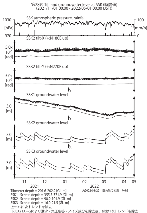
第 28 図 SSK における傾斜・地下水位観測結果 (2021 年 11 月～2022 年 4 月)。
