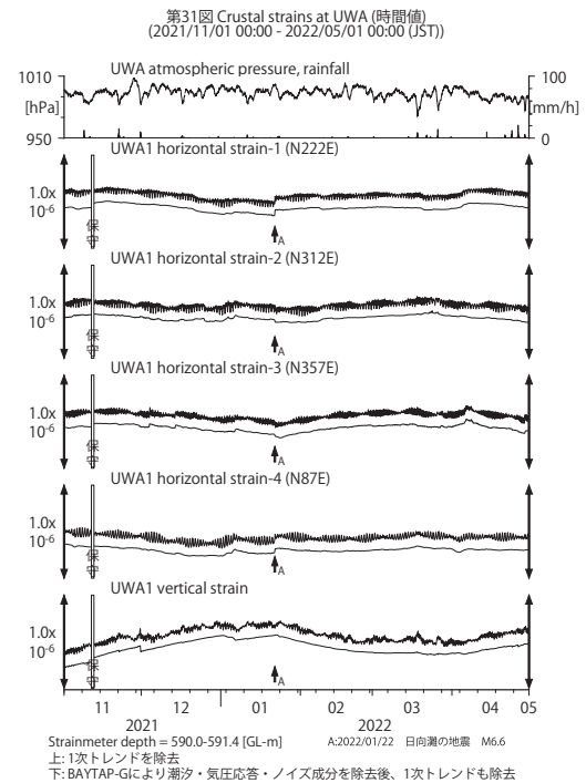
第 31 図 UWA における歪観測結果 (2021 年 11 月～2022 年 4 月)。
