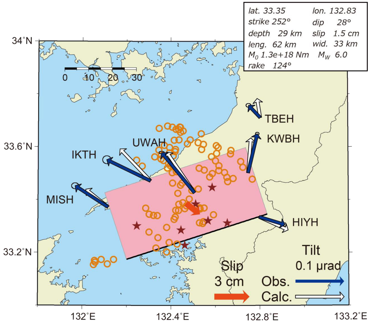
第 5 図 2021 年 12 月～2022 年 1 月四国西部の短期的 SSE の断層モデル。図の見方は第 3 図と同じ。
