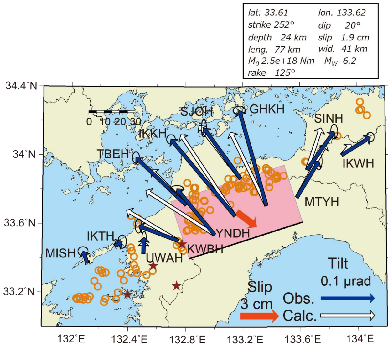
第 7 図 2022 年 3 月～4 月四国西部の短期的 SSE の断層モデル。図の見方は第 3 図と同じ。
