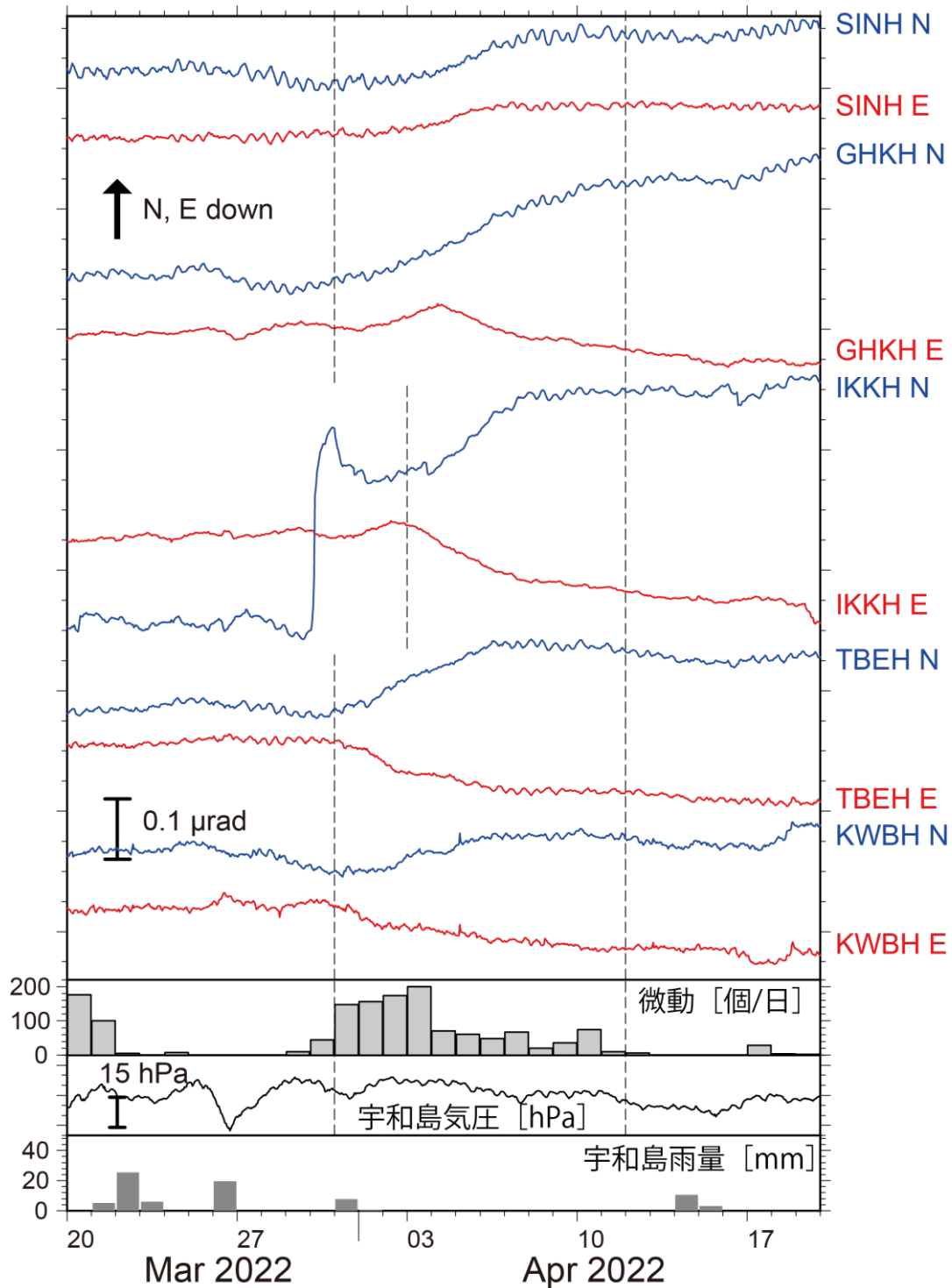
第 6 図 2022 年 3 月 20 日～4 月 19 日までの傾斜時系列. 図の見方は第 2 図と同様. 観測点位置は第 7 図に示した. 3 月 31 日 (IKKH は 4 月 3 日) ～4 月 11 日の傾斜変化量を SSE によるものと仮定した. 四国中西部での微動活動度・気象庁宇和島観測点での気圧変化および雨量をあわせて表示した.
