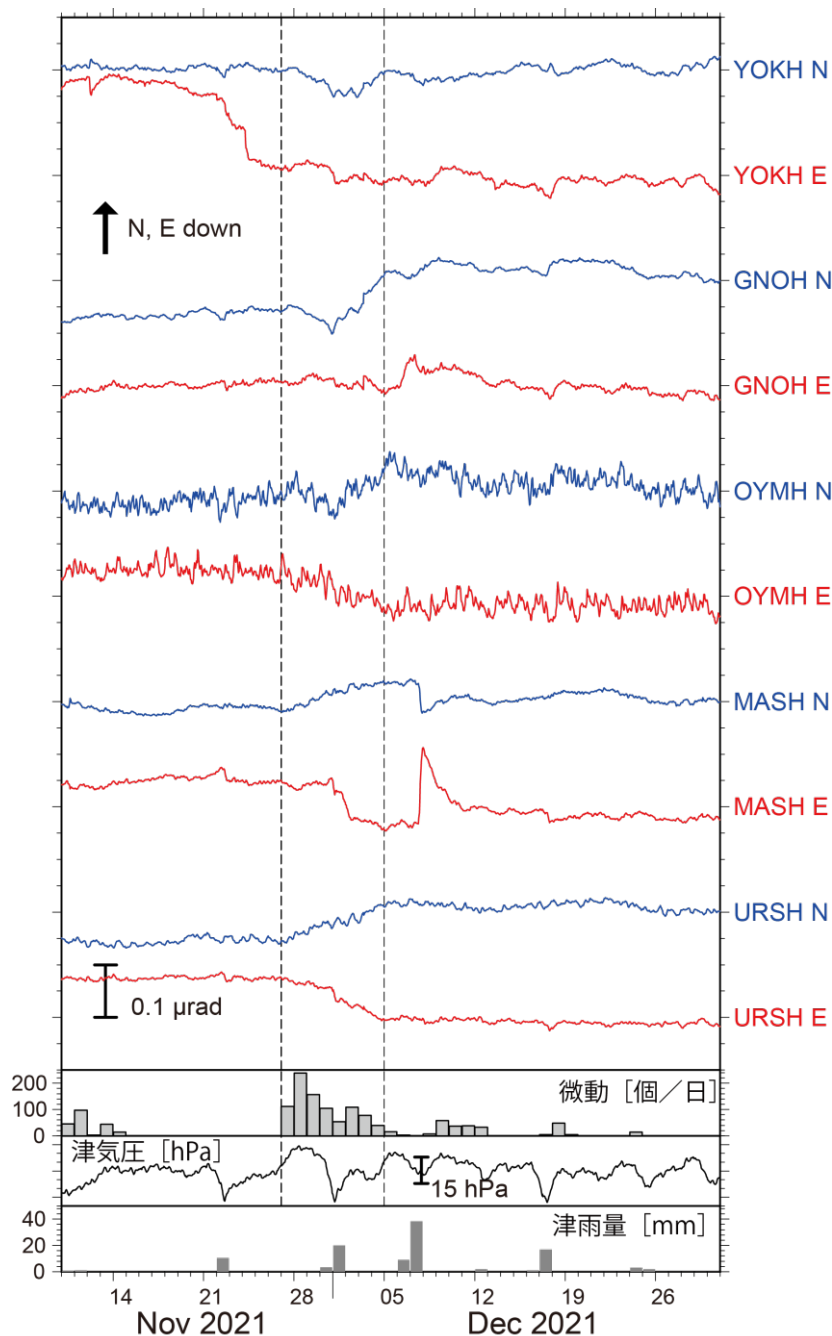
第 2 図 2021 年 11 月 10 日から 12 月 30 日までの傾斜時系列。観測点位置は第 3 図に示した。記録は上方向への変化が北・東下がり傾斜変動を表す。気圧応答・潮汐成分を BAYTAP-G 4) により除去し、直線トレンドを補正した後の記録を示した。11 月 27 日～12 月 4 日の傾斜変化量を SSE によるものと仮定した。紀伊半島北部～愛知県での微動活動度・気象庁津観測点での気圧変化および雨量をあわせて表示した。
