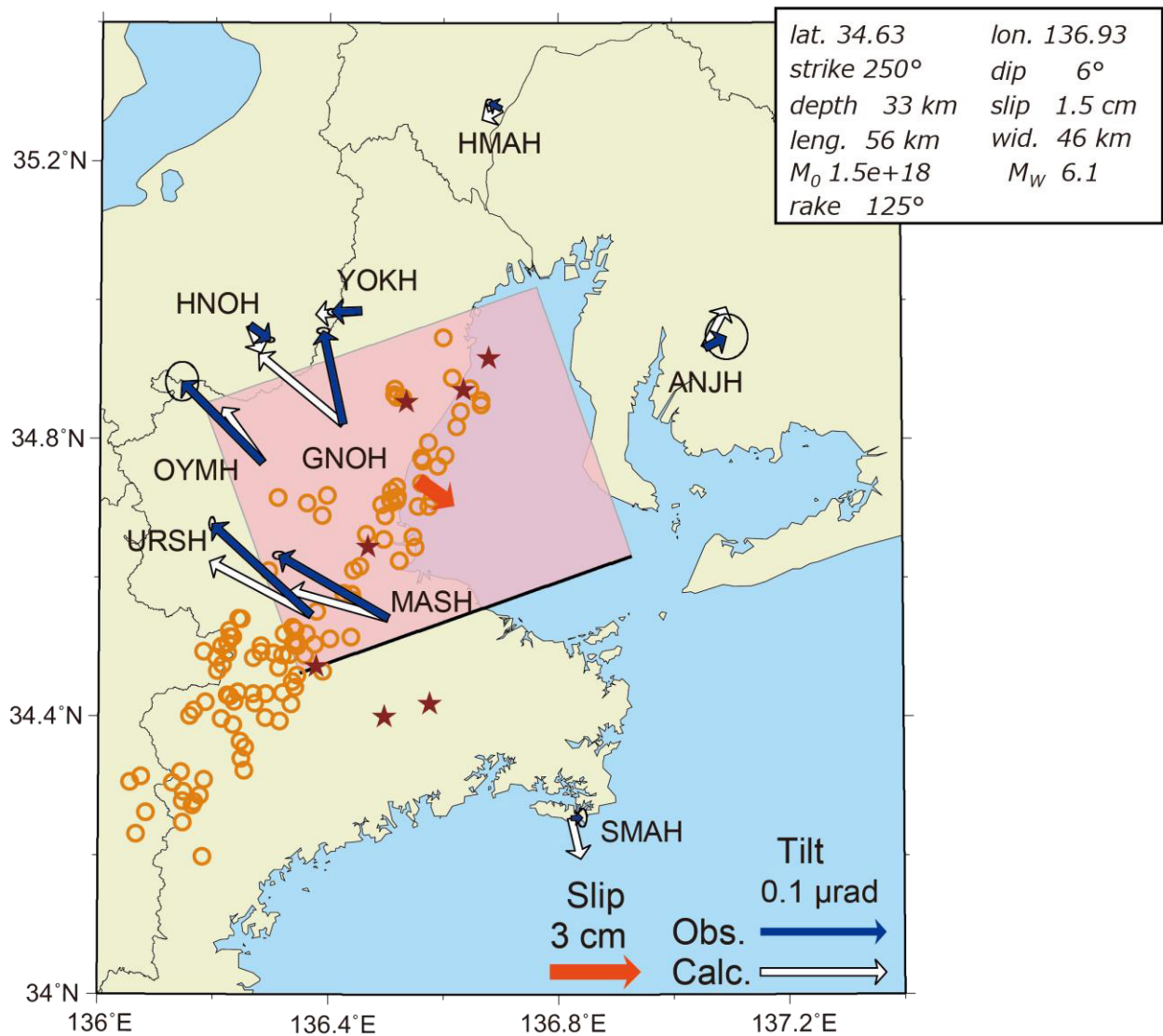
第 3 図 2021 年 11 月～12 月紀伊半島北部の短期的 SSE の断層モデル。第 2 図の破線で示された期間に観測された傾斜変化ベクトル（青矢印）・このデータから推定された SSE の断層モデル（赤矩形・矢印）・モデルから計算される傾斜変化ベクトル（白抜き矢印）を示す。同じ期間の微動と深部超低周波地震の震央を橙円と茶星印で示した。
