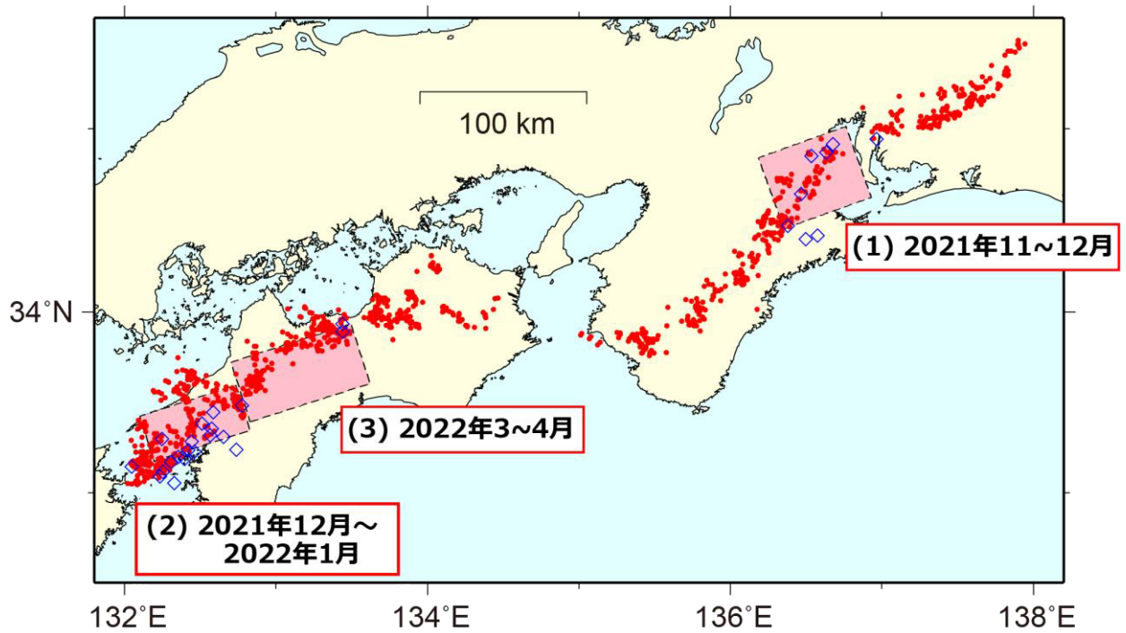
第 1 図 2021 年 11 月 1 日～2022 年 4 月 30 日の期間に検知された短期的 SSE (ピンク矩形). 同期間に発生した深部低周波微動 (赤点) 及び VLFE の震央 (青菱形) を重ねて表示した.
