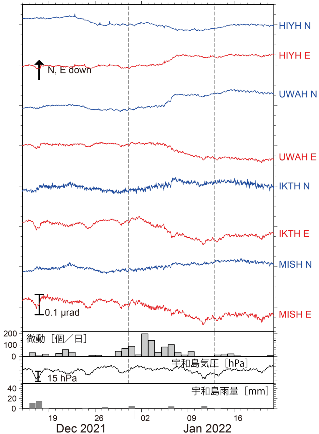
第 4 図 2021 年 12 月 15 日～2022 年 1 月 21 日までの傾斜時系列。図の見方は第 2 図と同様。観測点位置は第 5 図に示した。12 月 31 日～1 月 12 日の傾斜変化量を SSE によるものと仮定した。四国西部での微動活動度・気象庁宇和島観測点での気圧変化および雨量をあわせて表示した。
