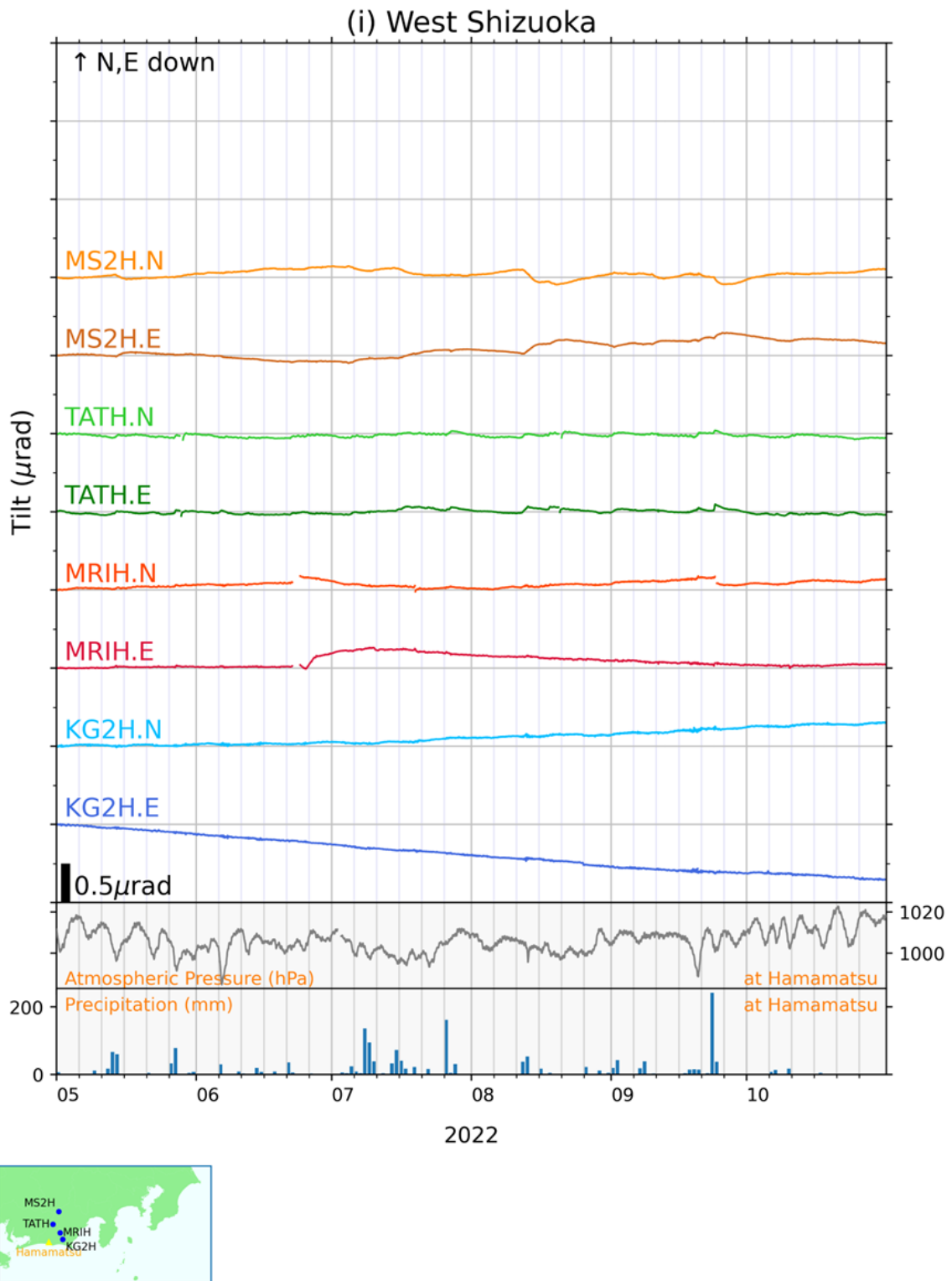
第 2 図 (i) 傾斜の時間値記録（静岡西部）及び気圧・日雨量（浜松）.
