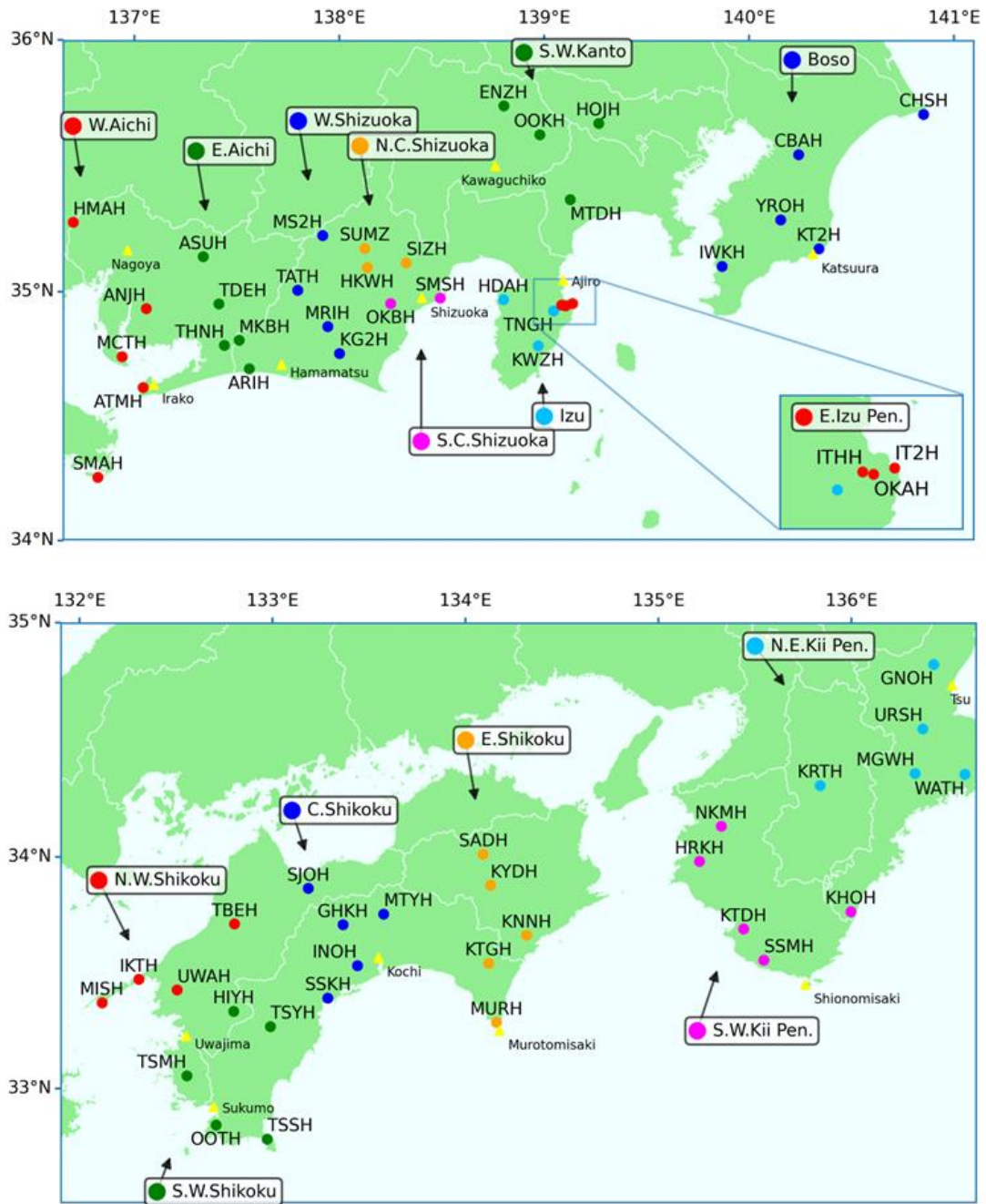
第 1 図 傾斜観測点配置 (丸印). 図 2 では観測点シンボルの色で分けしたグループ毎に記録を示している. 使用した気象庁気象観測点を三角形 (黄色) であわせて示す.
