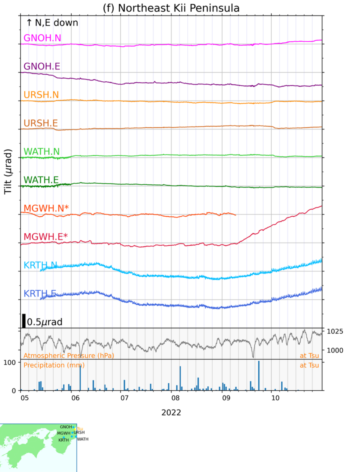
第 2 図 (f) 傾斜の時間値記録（紀伊半島北東部）及び気圧・日雨量（津）.
