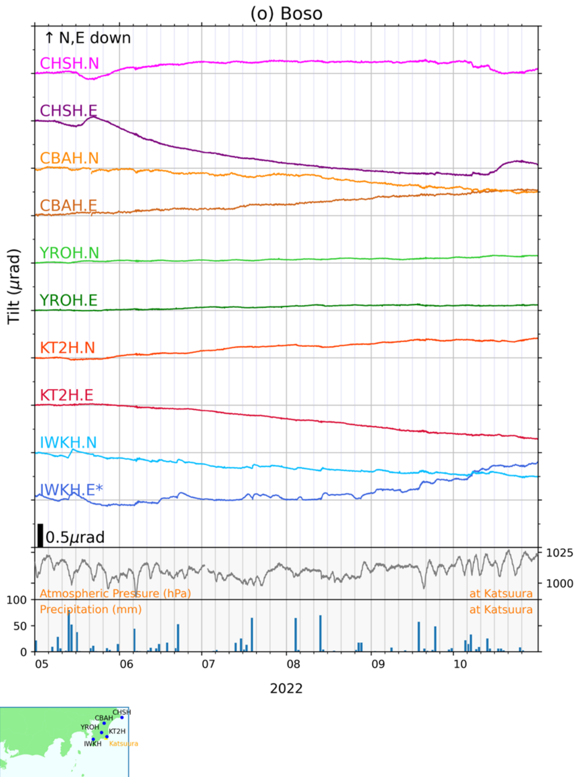
第 2 図 (o) 傾斜の時間値記録 (房総) 及び気圧・日雨量 (勝浦).
