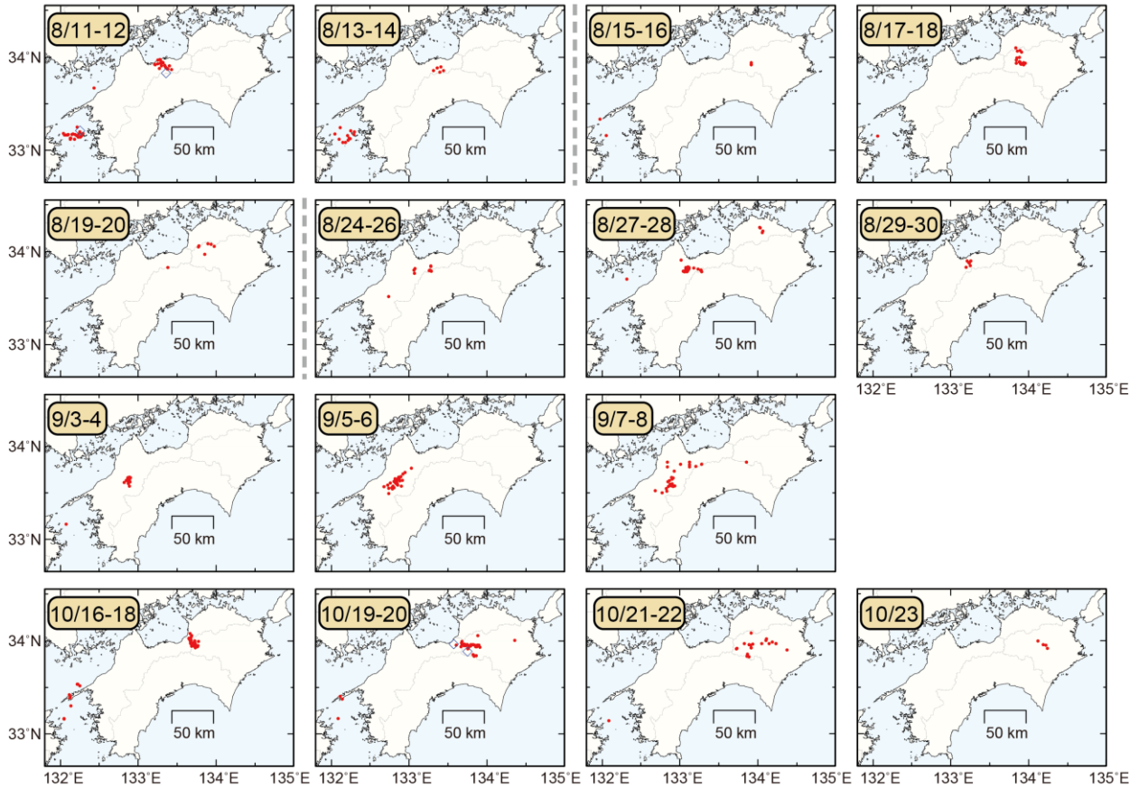
第 6 図 2022 年 8 月から 2022 年 10 月までの期間に四国地域で発生した、主な深部低周波微動及び超低周波地震の活動における震央分布スナップショット。赤丸が当該期間の微動、青菱形が超低周波地震を表す。
