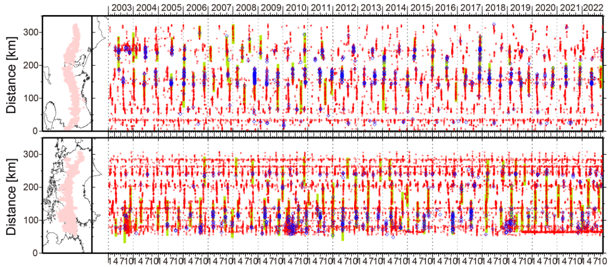
第 3 図 西南日本で発生した深部低周波微動（赤丸）及び深部超低周波地震（青菱形）の 2003 年から約 20 年間の時空間分布。黄緑色太線は、傾斜変動から検出された短期的スロースリップイベントを示す。
