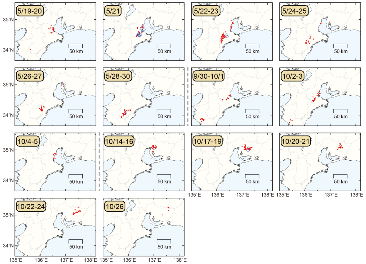
第 4 図 2022 年 5 月から 2022 年 10 月までの期間に東海・紀伊半島地域で発生した、主な深部低周波微動及び深部超低周波地震の活動における震央分布スナップショット。赤丸が当該期間の微動、青菱形が超低周波地震を表す。
