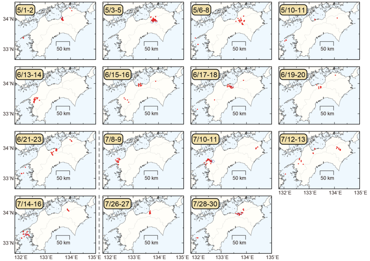
第 5 図 2022 年 5 月から 2022 年 7 月までの期間に四国地域で発生した、主な深部低周波微動及び超低周波地震の活動における震央分布スナップショット。赤丸が当該期間の微動、青菱形が超低周波地震を表す。
