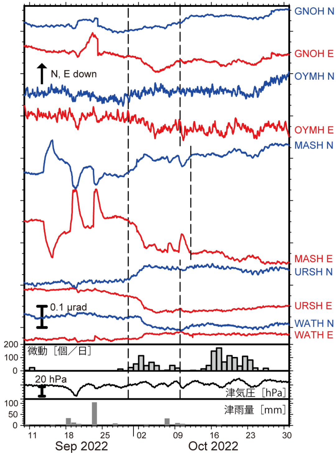
第 6 図 2022 年 9 月 10 日～10 月 30 日までの傾斜時系列。図の見方は第 2 図と同様。観測点位置は第 7 図に示した。9 月 30 日～10 月 9 日（MASH は 10 月 11 日）の傾斜変化量を SSE によるものと仮定した。紀伊半島北部～愛知県での微動活動度・気象庁津観測点での気圧変化および雨量をあわせて表示した。
