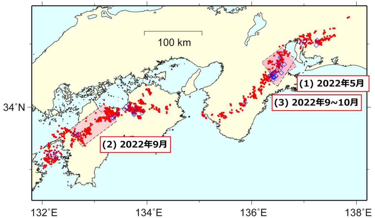
第 1 図 2022 年 5 月 1 日～2022 年 10 月 31 日の期間に検知された短期的 SSE (ピンク矩形). 同期間に発生した深部低周波微動 (赤点) 及び VLFE の震央 (青菱形) を重ねて表示した.
