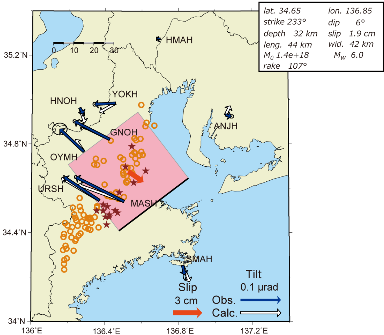
第 3 図 2022 年 5 月紀伊半島北部の短期的 SSE の断層モデル。第 2 図の破線で示された期間に観測された傾斜変化ベクトル（青矢印）・このデータから推定された SSE の断層モデル（赤矩形・矢印）・モデルから計算される傾斜変化ベクトル（白抜き矢印）を示す。同じ期間の微動と深部超低周波地震の震央を橙円と茶星印で示した。
