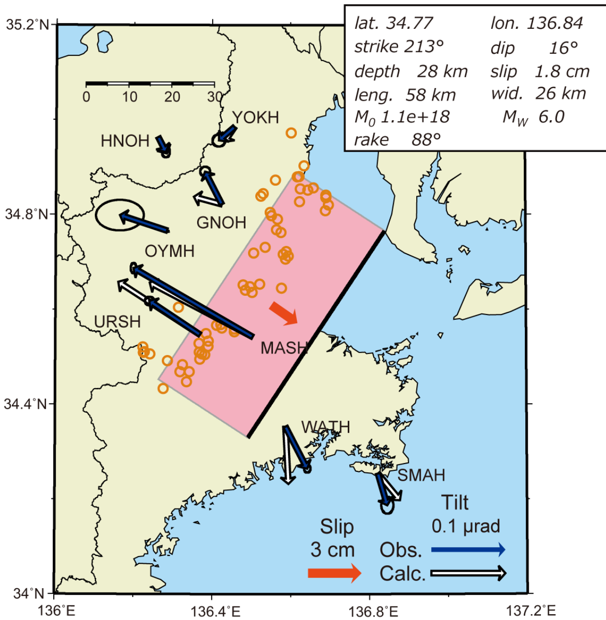
第 7 図 2022 年 9 月～10 月紀伊半島北部の短期的 SSE の断層モデル。図の見方は第 3 図と同じ。
