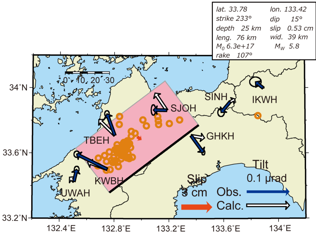
第 5 図 2022 年 9 月四国中西部の短期的 SSE の断層モデル. 図の見方は第 3 図と同じ.
