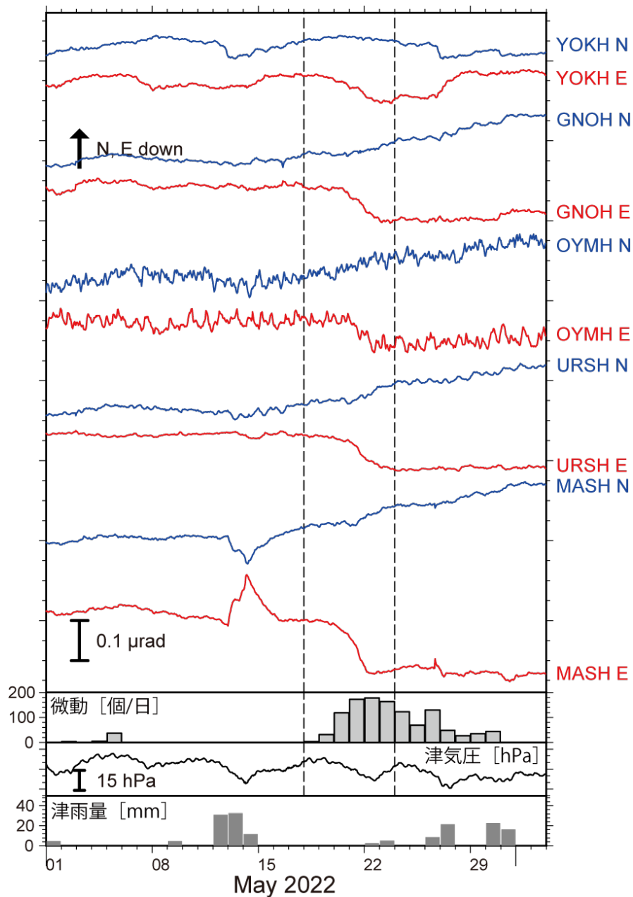
第 2 図 2022 年 5 月 1 日から 6 月 2 日までの傾斜時系列。観測点位置は第 3 図に示した。記録は上方向への変化が北・東下がりの傾斜変動を表す。気圧応答・潮汐成分を BAYTAP-G 4) により除去し、直線トレンドを補正した後の記録を示した。5 月 18 日～5 月 23 日の傾斜変化量を SSE によるものと仮定した。紀伊半島北部～愛知県での微動活動量・気象庁津観測点での気圧変化および雨量をあわせて表示した。
