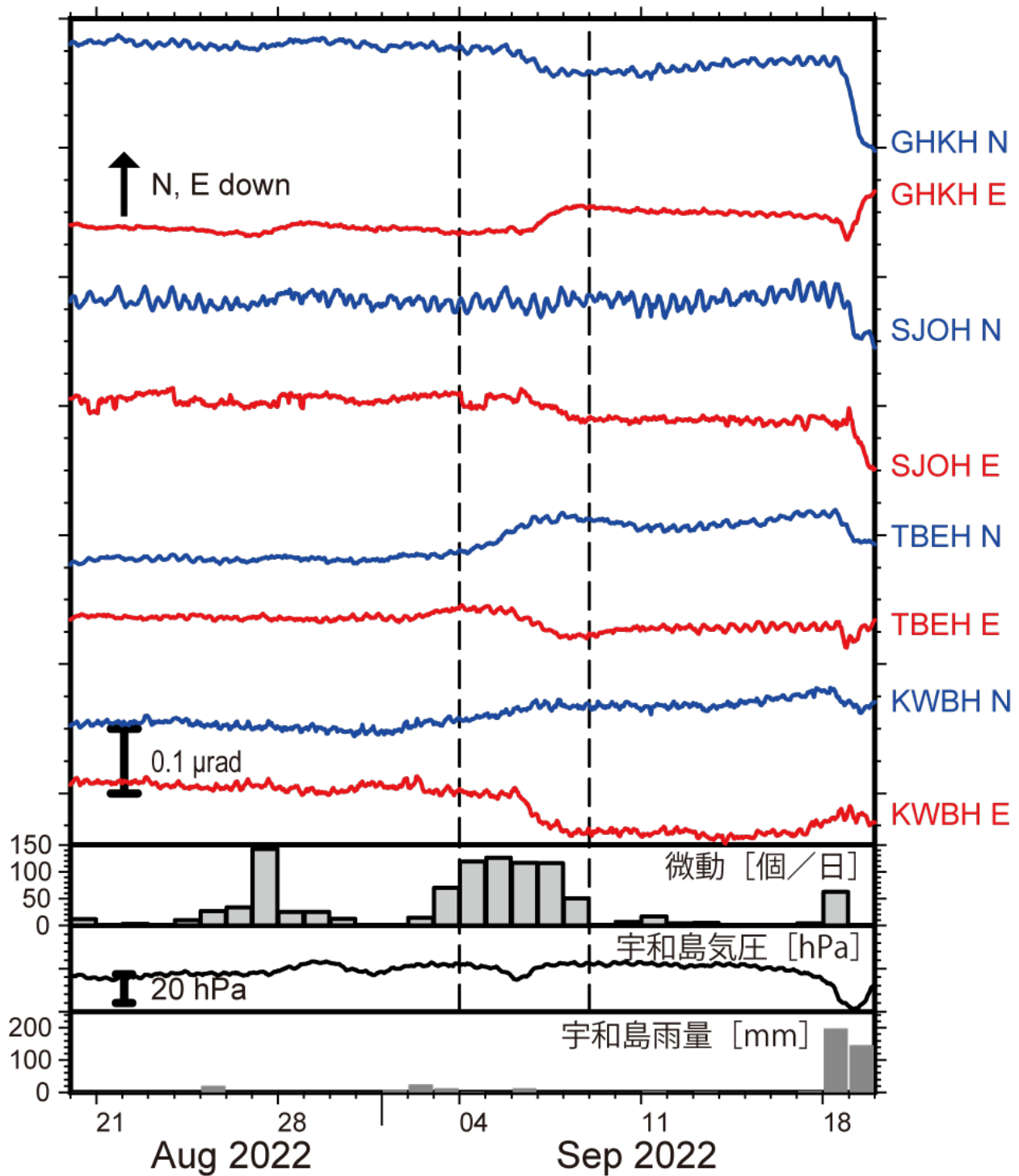
第 4 図 2022 年 8 月 20 日～9 月 19 日までの傾斜時系列. 図の見方は第 2 図と同様. 観測点位置は第 5 図に示した. 9 月 4 日～9 月 8 日の傾斜変化量を SSE によるものと仮定した. 四国西部～中部での微動活動度・気象庁宇和島観測点での気圧変化および雨量をあわせて表示した.
