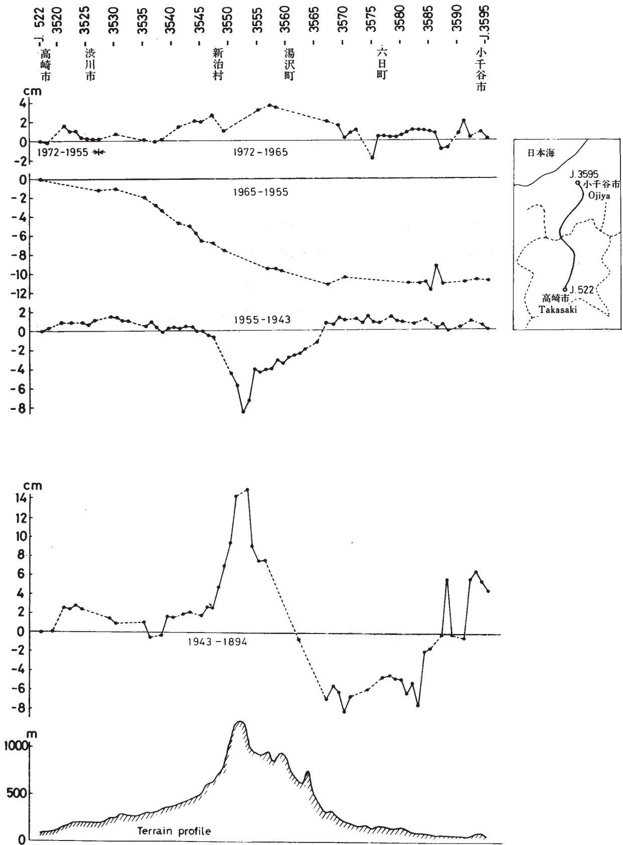
第1図 高崎～小千谷間の上下変動
