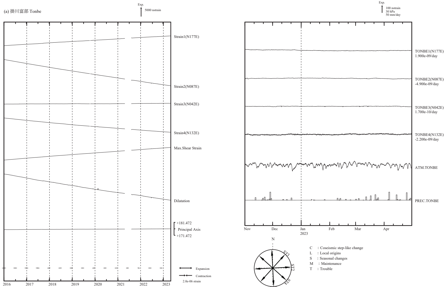
第 4 図 (a) 左:2016 年 1 月以後の多成分ひずみ計変化(日平均値)。主ひずみ・最大せん断ひずみ・面積ひずみは各方向成分から計算されている。右:2022 年 11 ~ 2023 年 4 月の多成分ひずみ計変化(時間値:気圧・潮汐・地磁気・降水補正した値)。各図下部に気圧変化と降水量を示す。
