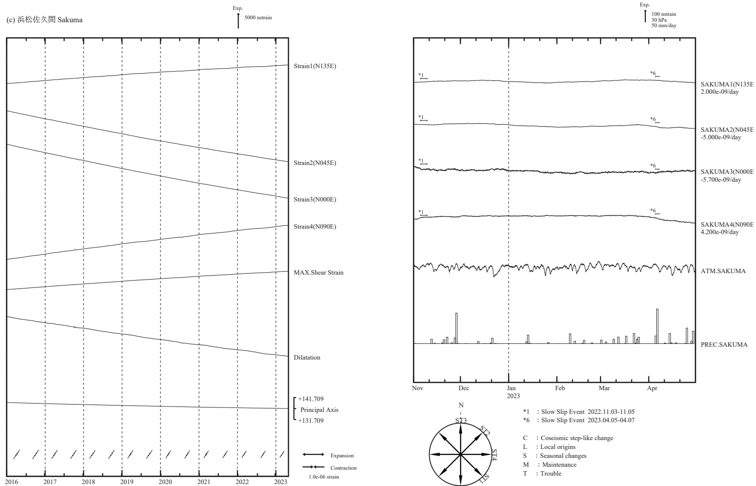
第 4 図 (c) 左:2016 年 1 月以後の多成分ひずみ計変化(日平均値)。主ひずみ・最大せん断ひずみ・面積ひずみは各方向成分から計算されている。右:2022 年 11 ~ 2023 年 4 月の多成分ひずみ計変化(時間値:気圧・潮汐・地磁気・降水補正した値)。各図下部に気圧変化と降水量を示す。
