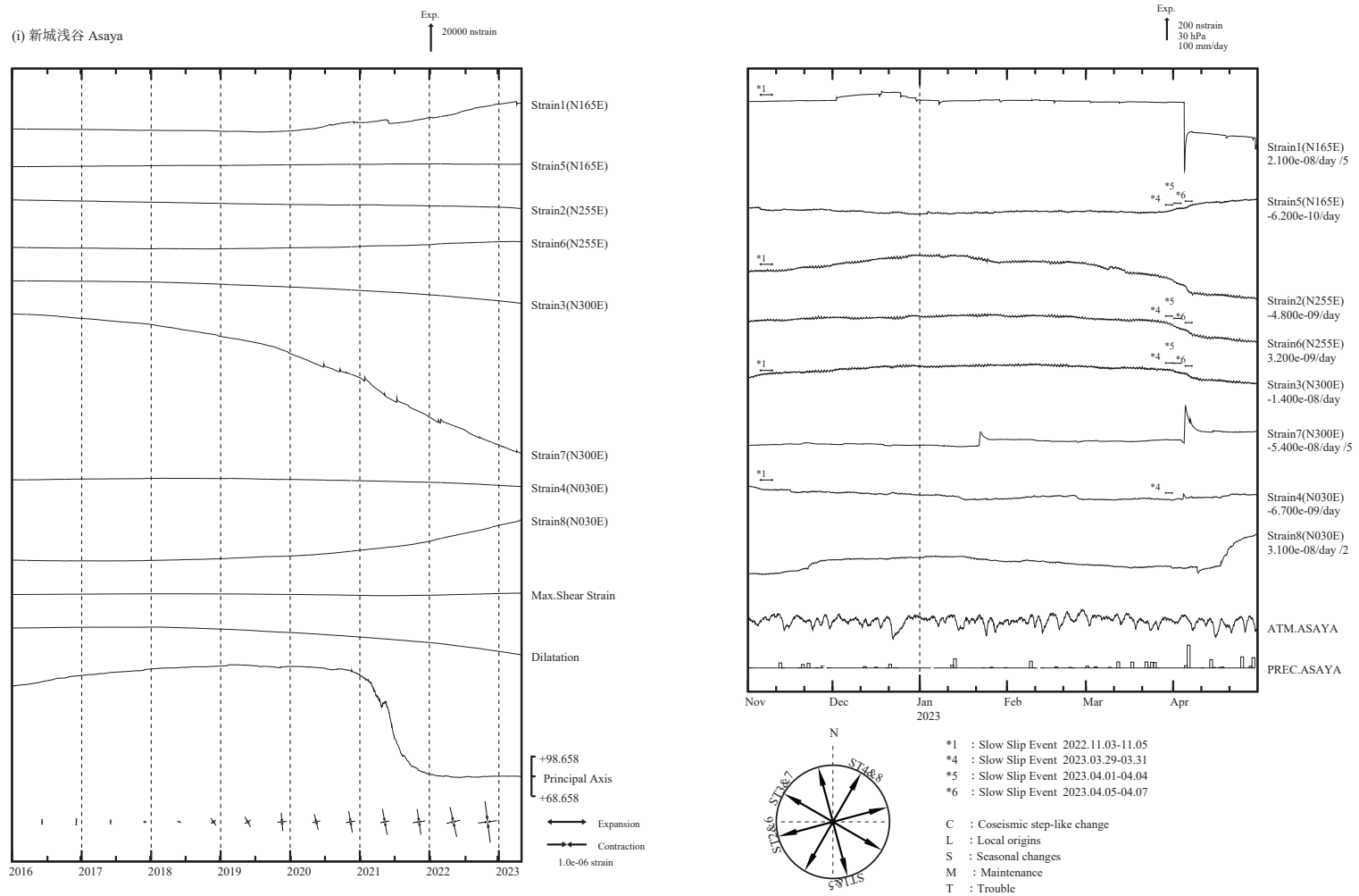
第 4 図 (i) 左: 2016 年 1 月以後の多成分ひずみ計変化 (日平均値)。主ひずみ・最大せん断ひずみ・面積ひずみは各方向成分から計算されている。右: 2022 年 11 ~ 2023 年 4 月の多成分ひずみ計変化 (時間値: 気圧・潮汐・地磁気・降水補正した値)。各図下部に気圧変化と降水量を示す。
