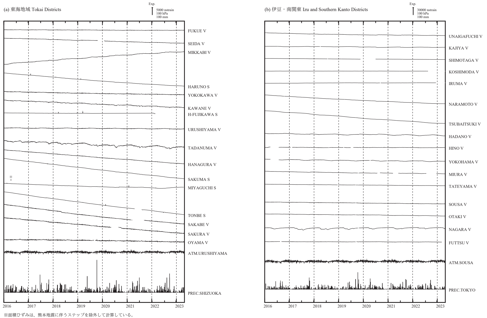
第 2 図 (a), (b) 2016 年 1 月以後の東海・伊豆・南関東地域における区域別体積ひずみ (V) 及び面積ひずみ (S) の変化 (日平均値). 各図下部に区域を代表する気圧変化と降水量を示す.
