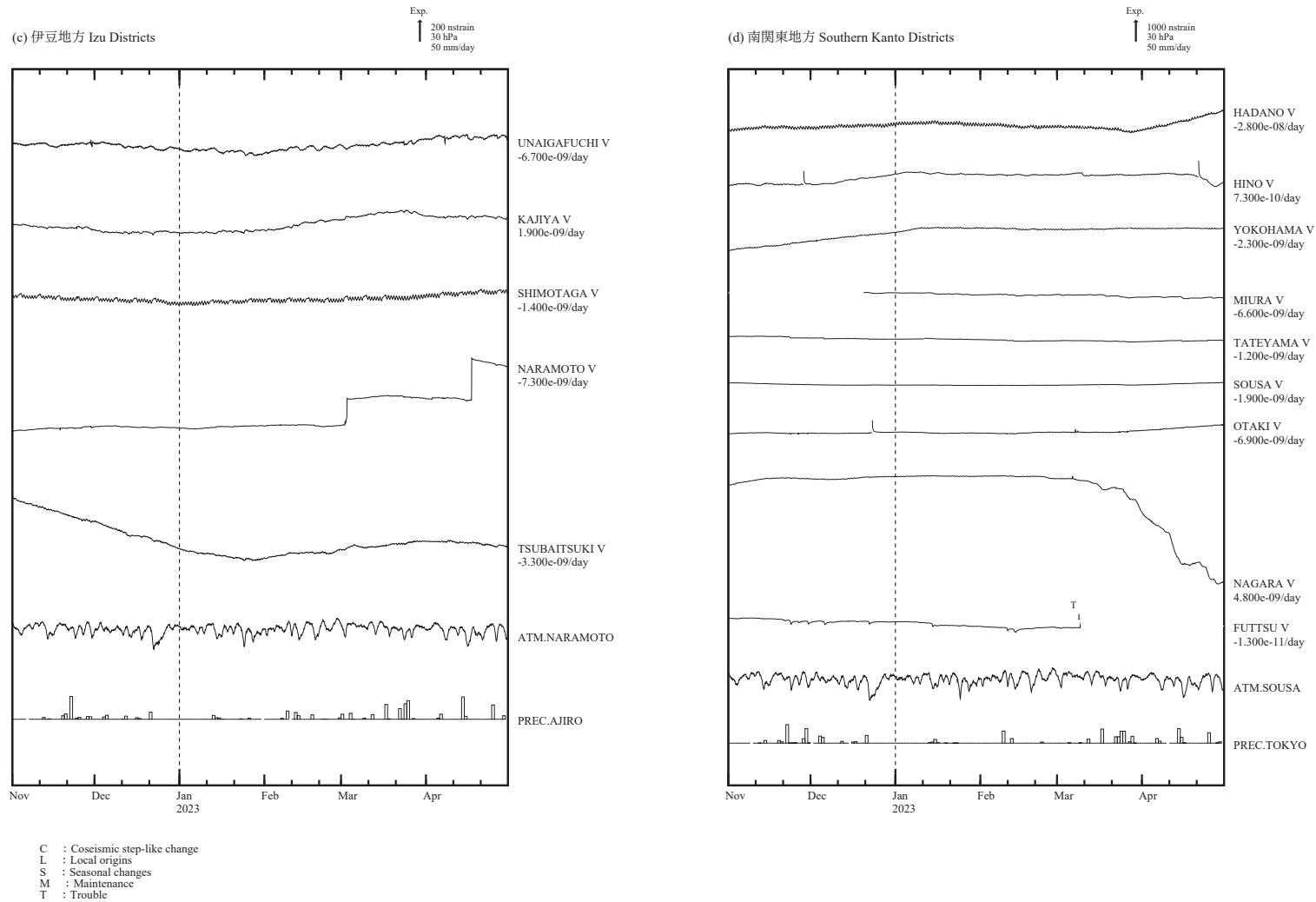
第3図 (c),(d) 2022年11月～2023年4月の東海・伊豆・南関東地域における区域別体積ひずみ (V) 及び面積ひずみ (S) の変化 (時間値: 気圧・潮汐・降水補正した値)。各図下部に区域を代表する気圧変化と降水量を示す。地点名の下に D strain/day 及び /M はそれぞれ1日あたりのトレンド変化量を D として補正していること及び縮尺を 1/M 倍にして表示していることを示している。
