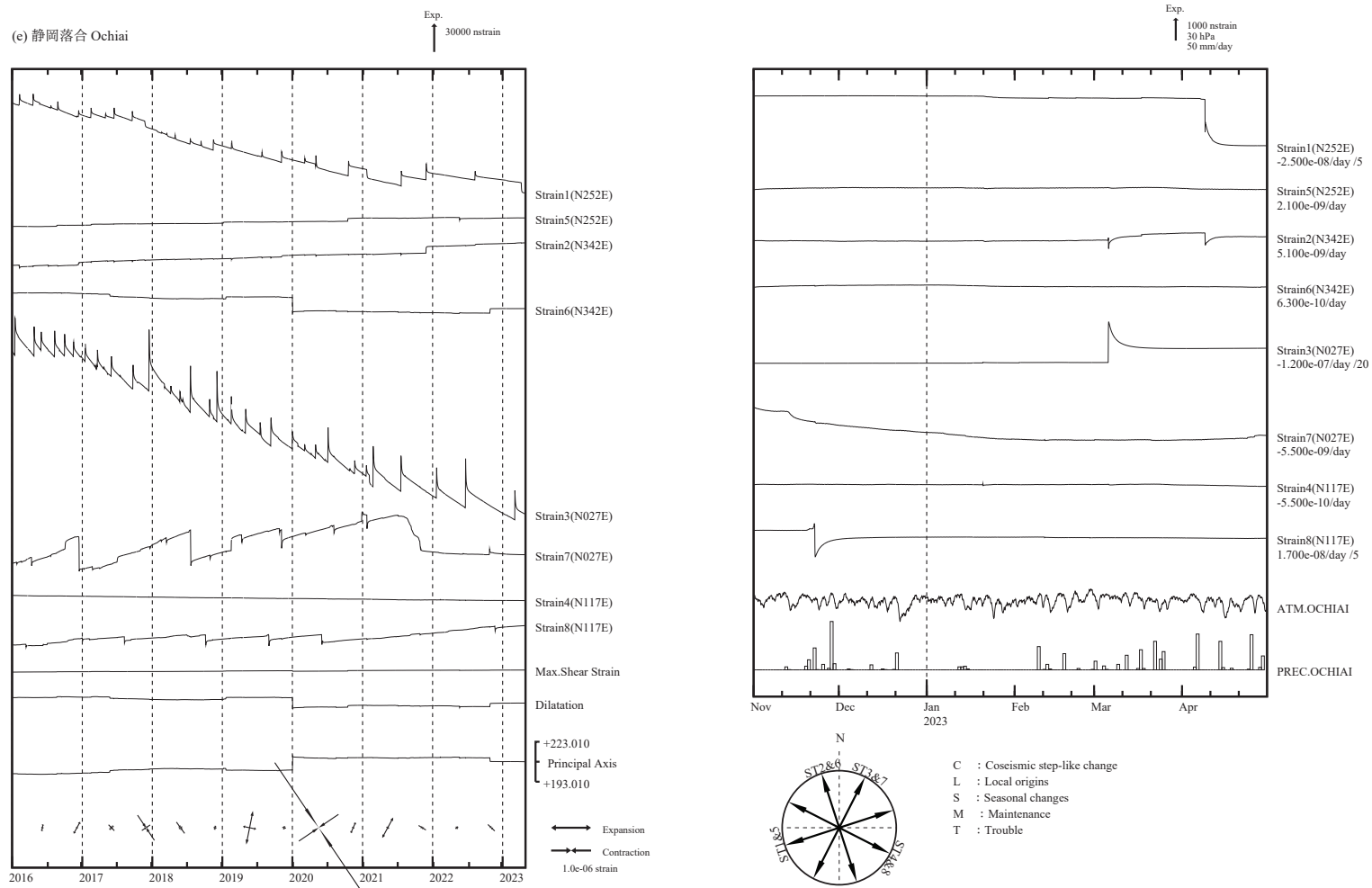
第 4 図 (e) 左: 2016 年 1 月以後の多成分ひずみ計変化 (日平均値)。主ひずみ・最大せん断ひずみ・面積ひずみは各方向成分から計算されている。右: 2022 年 11 ~ 2023 年 4 月の多成分ひずみ計変化 (時間値: 気圧・潮汐・地磁気・降水補正した値)。各図下部に気圧変化と降水量を示す。
