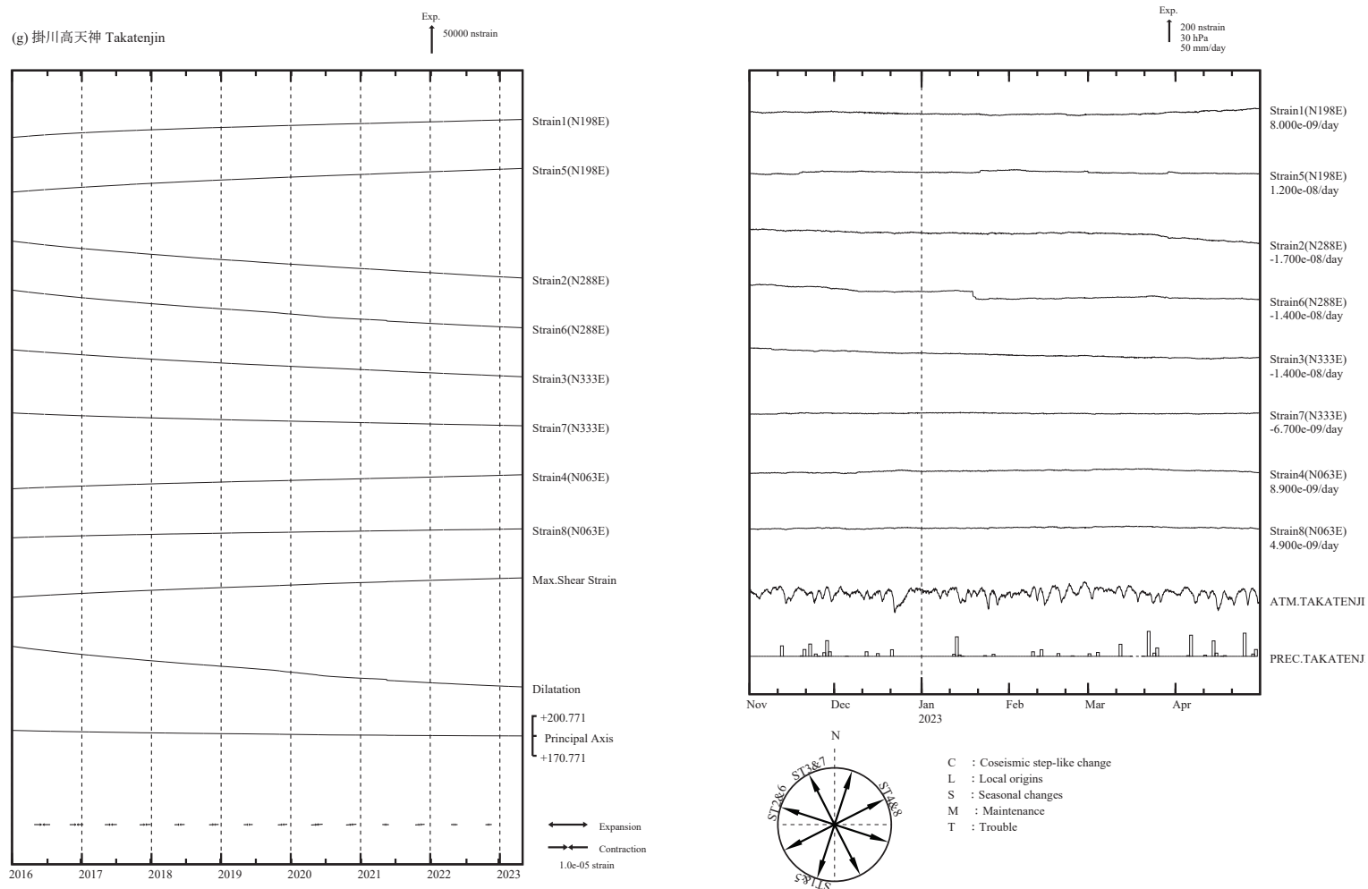
第 4 図 (g) 左: 2016 年 1 月以後の多成分ひずみ計変化 (日平均値)。主ひずみ・最大せん断ひずみ・面積ひずみは各方向成分から計算されている。右: 2022 年 11 ~ 2023 年 4 月の多成分ひずみ計変化 (時間値: 気圧・潮汐・地磁気・降水補正した値)。各図下部に気圧変化と降水量を示す。
