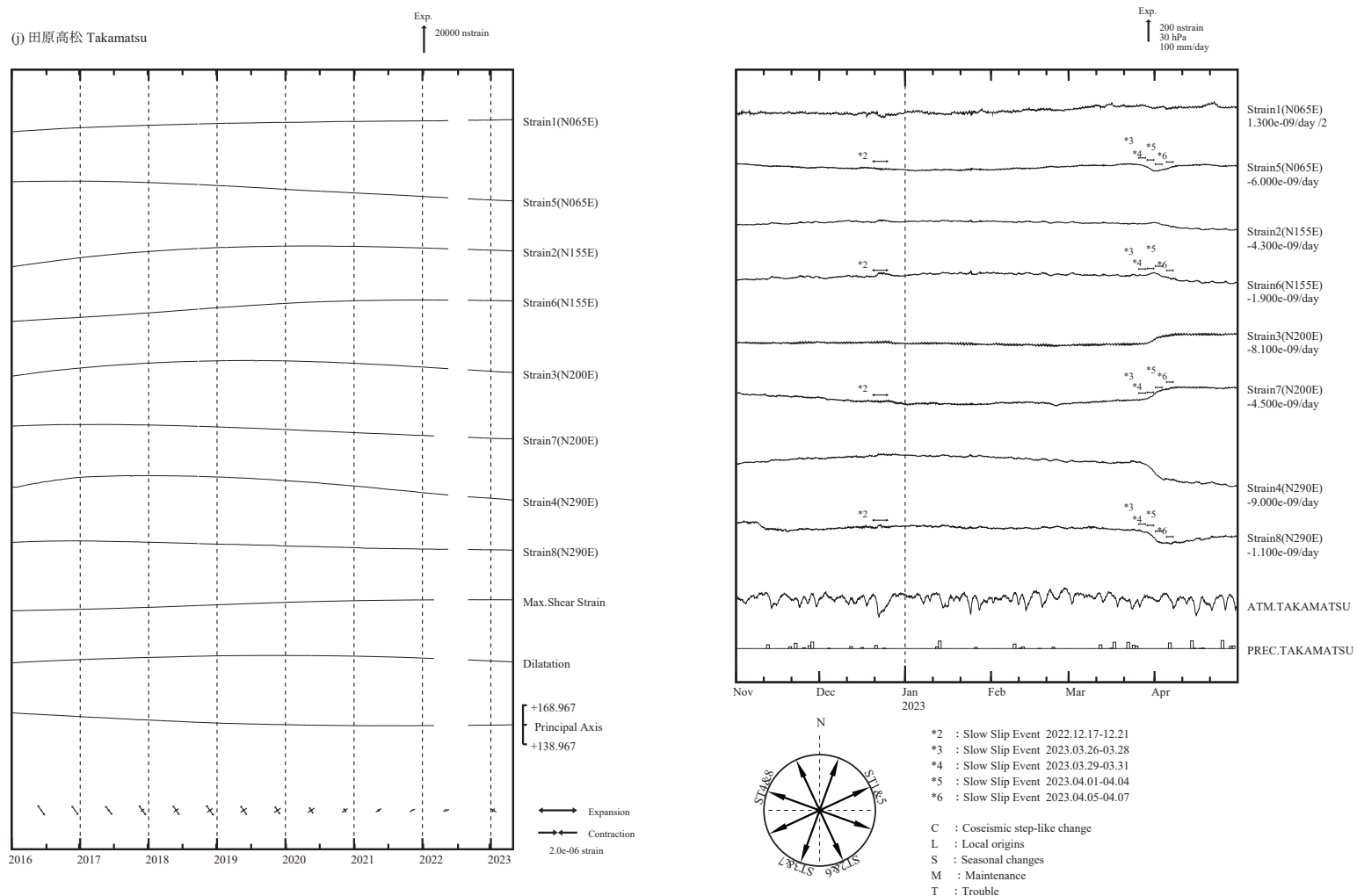
第 4 図 (j) 左:2016 年 1 月以後の多成分ひずみ計変化 (日平均値)。主ひずみ・最大せん断ひずみ・面積ひずみは各方向成分から計算されている。右:2022 年 11 ~ 2023 年 4 月の多成分ひずみ計変化 (時間値: 気圧・潮汐・地磁気・降水補正した値)。各図下部に気圧変化と降水量を示す。
