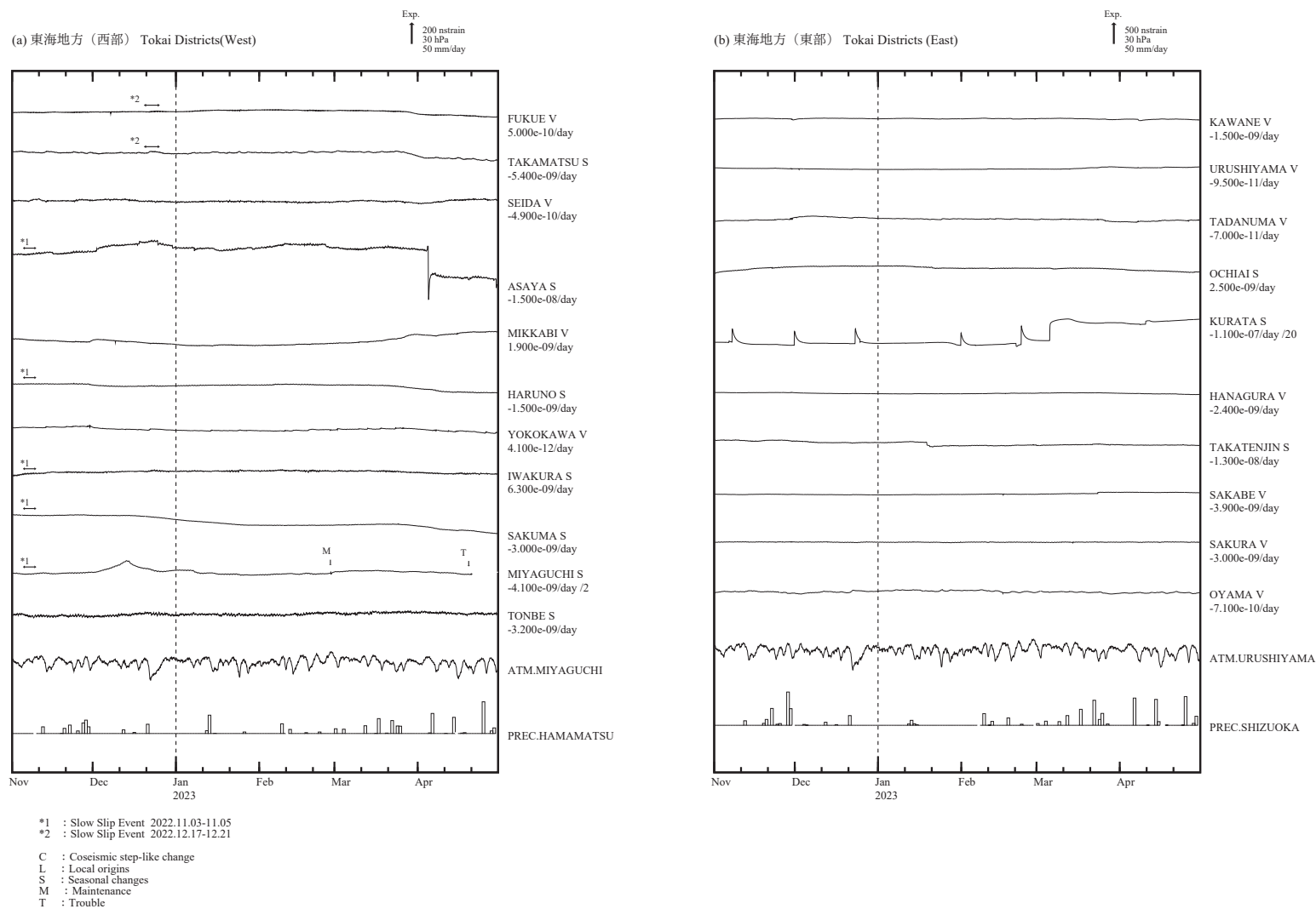
第 3 図 (a),(b) 2022 年 11 月～2023 年 4 月の東海・伊豆・南関東地域における区域別体積ひずみ (V) 及び面積ひずみ (S) の変化 (時間値: 気圧・潮汐・降水補正した値)。各図下部に区域を代表する気圧変化と降水量を示す。地点名の下に D strain/day 及び /M はそれぞれ 1 日あたりのトレンド変化量を D として補正していること及び縮尺を 1/M 倍にして表示していることを示している。
