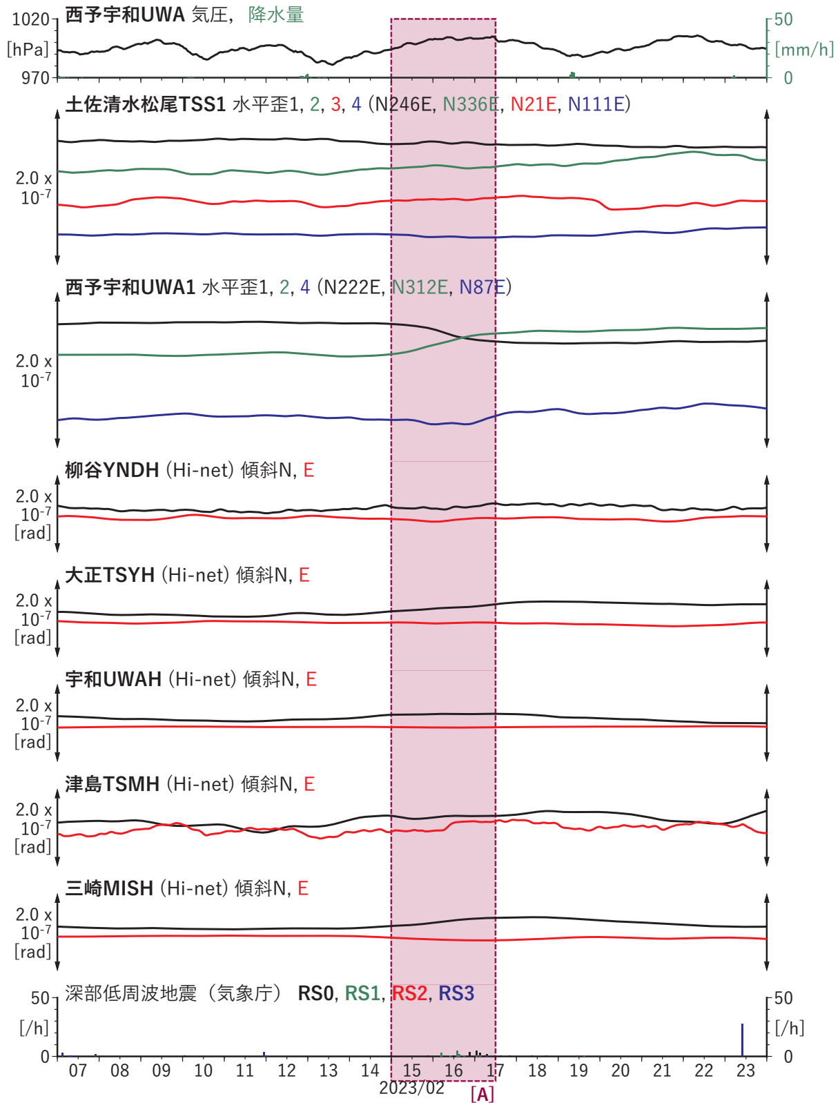
第 21 図 四国西部における歪・傾斜の観測結果と低周波地震の検出数 (2023/02/07 ~ 2023/02/23).
