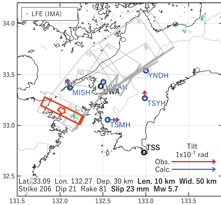
第 22 図 第 21 図 [A] を説明する断層モデル. 各図の説明は第 3 図を参照.
