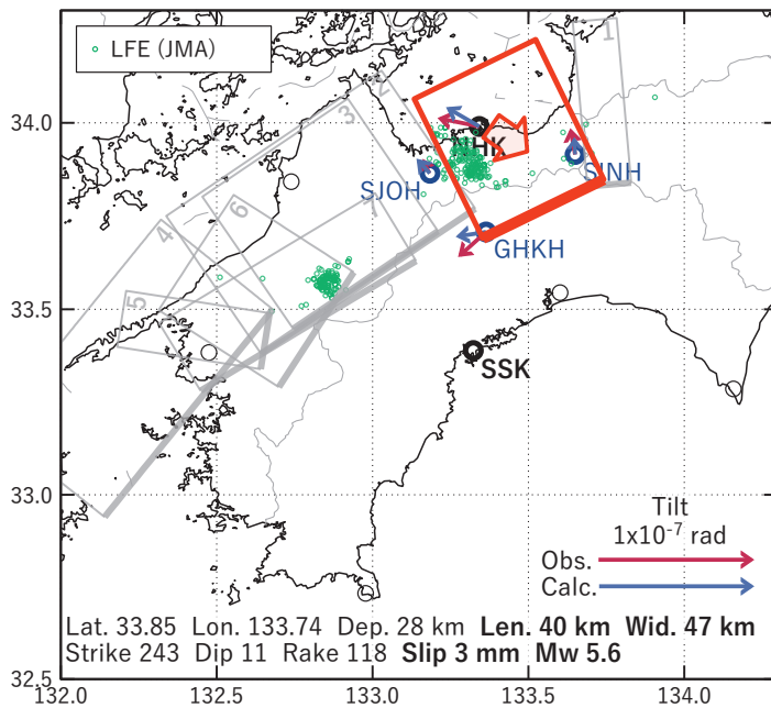
第 34 図 第 33 図 [A] を説明する断層モデル. 各図の説明は第 3 図を参照.
