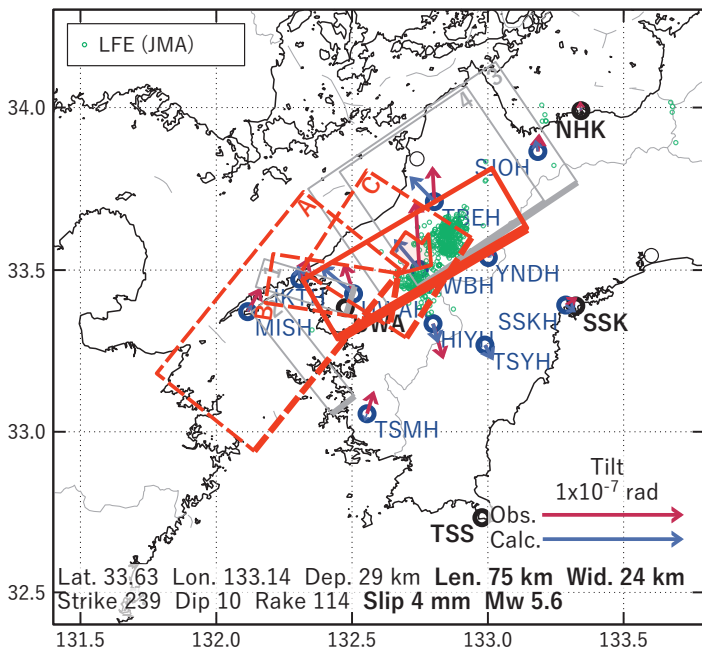
第 12 図 第 8 図 [D] を説明する断層モデル. 各図の説明は第 3 図を参照.
