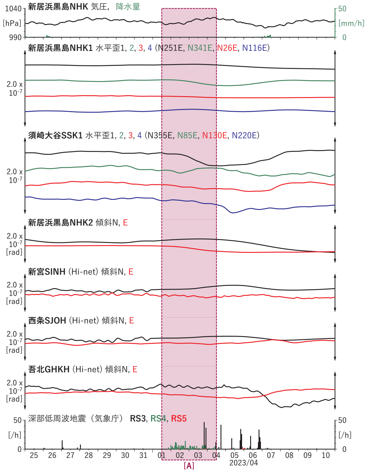
第 33 図 四国西部における歪・傾斜の観測結果と低周波地震の検出数 (2023/03/25 ~ 2023/04/10).
