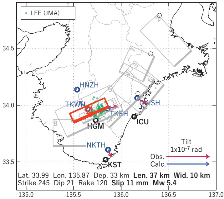
第 25 図 第 24 図 [A] を説明する断層モデル. 各図の説明は第 3 図を参照.
