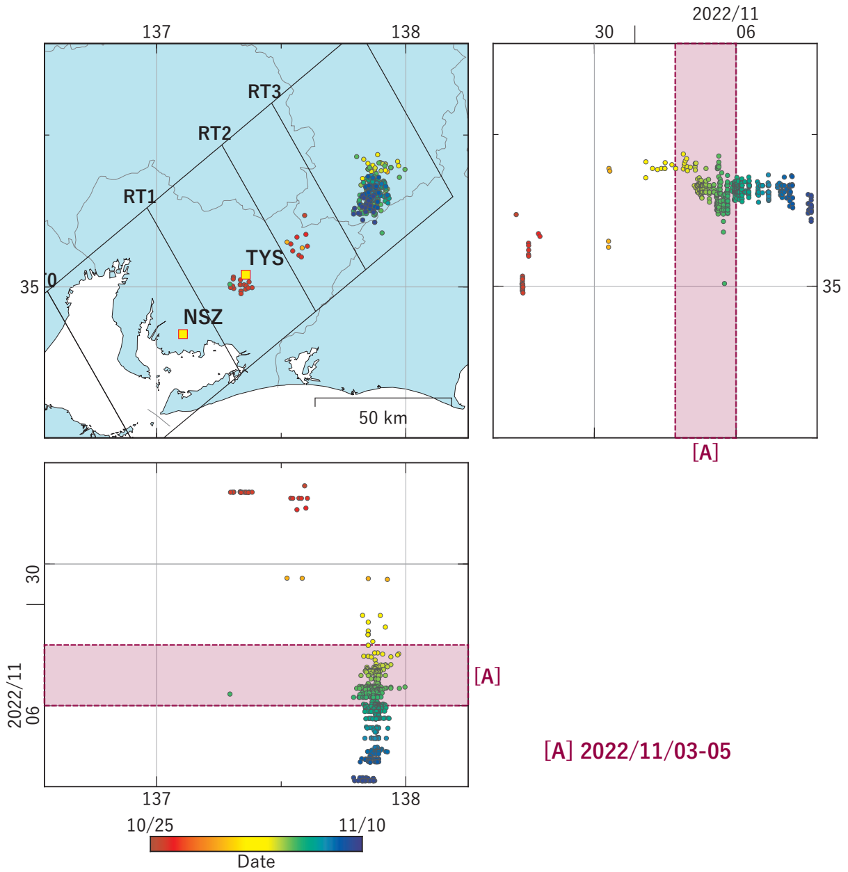
第 1 図 東海地域における低周波地震（気象庁一元化カタログによる）の時空間分布（2022/10/25 ～ 2022/11/09）. Fig. 1 Space-time distribution of low-frequency earthquakes by JMA unified hypocenter catalog in the Tokai region from October 25 to November 09, 2022.
