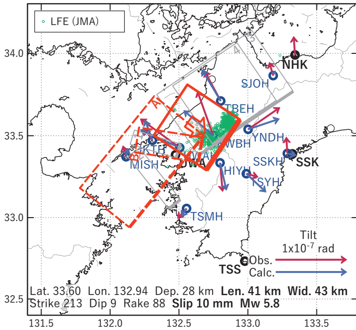
第 11 図 第 8 図 [C] を説明する断層モデル。各図の説明は第 3 図を参照。
