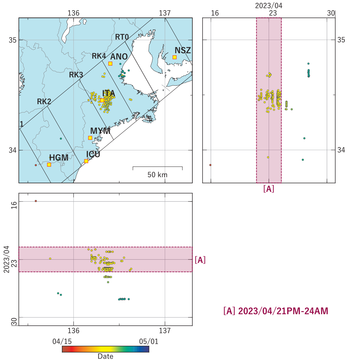
第 35 図 紀伊半島における低周波地震（気象庁一元化カタログによる）の時空間分布（2023/04/15～2023/04/30）. Fig. 35 Space-time distribution of low-frequency earthquakes by JMA unified hypocenter catalog in the Kii Peninsula from April 15 to 30, 2023.
