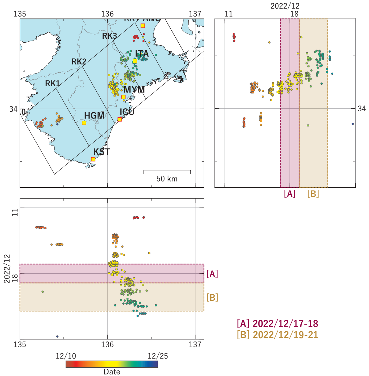
第 13 図 紀伊半島における低周波地震（気象庁一元化カタログによる）の時空間分布（2022/12/10～2022/12/24）. Fig. 13 Space-time distribution of low-frequency earthquakes by JMA unified hypocenter catalog in the Kii Peninsula from December 10 to 24, 2022.
