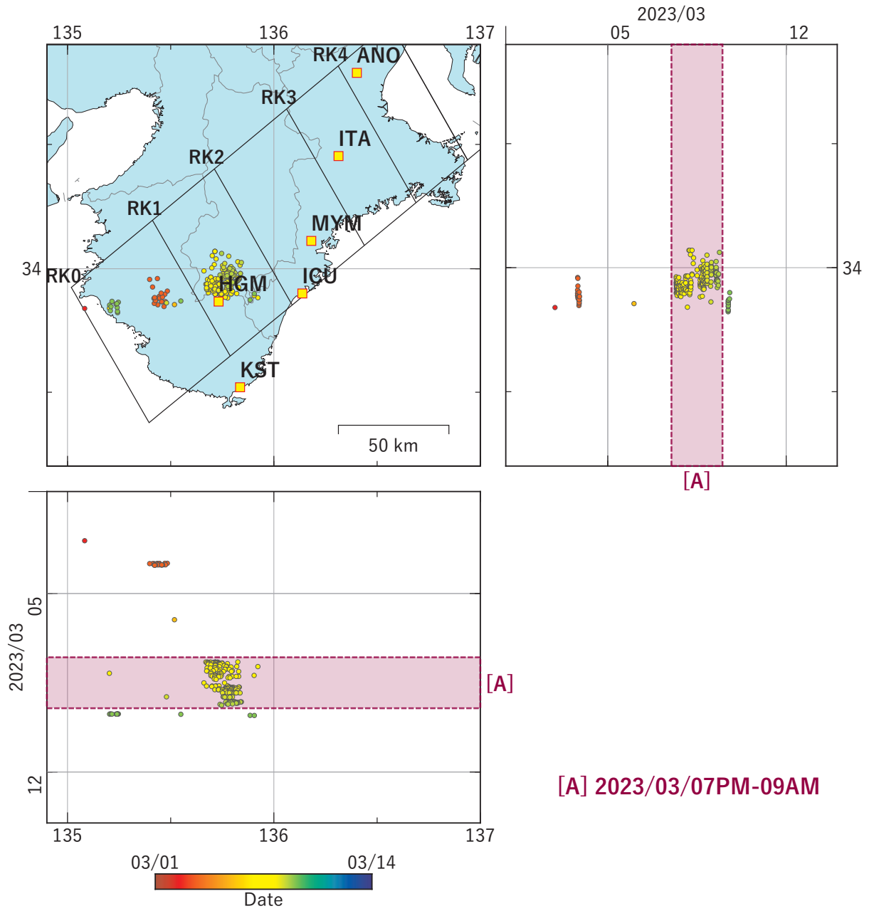
第 23 図 紀伊半島における低周波地震（気象庁一元化カタログによる）の時空間分布（2023/03/01～2023/03/13）。
