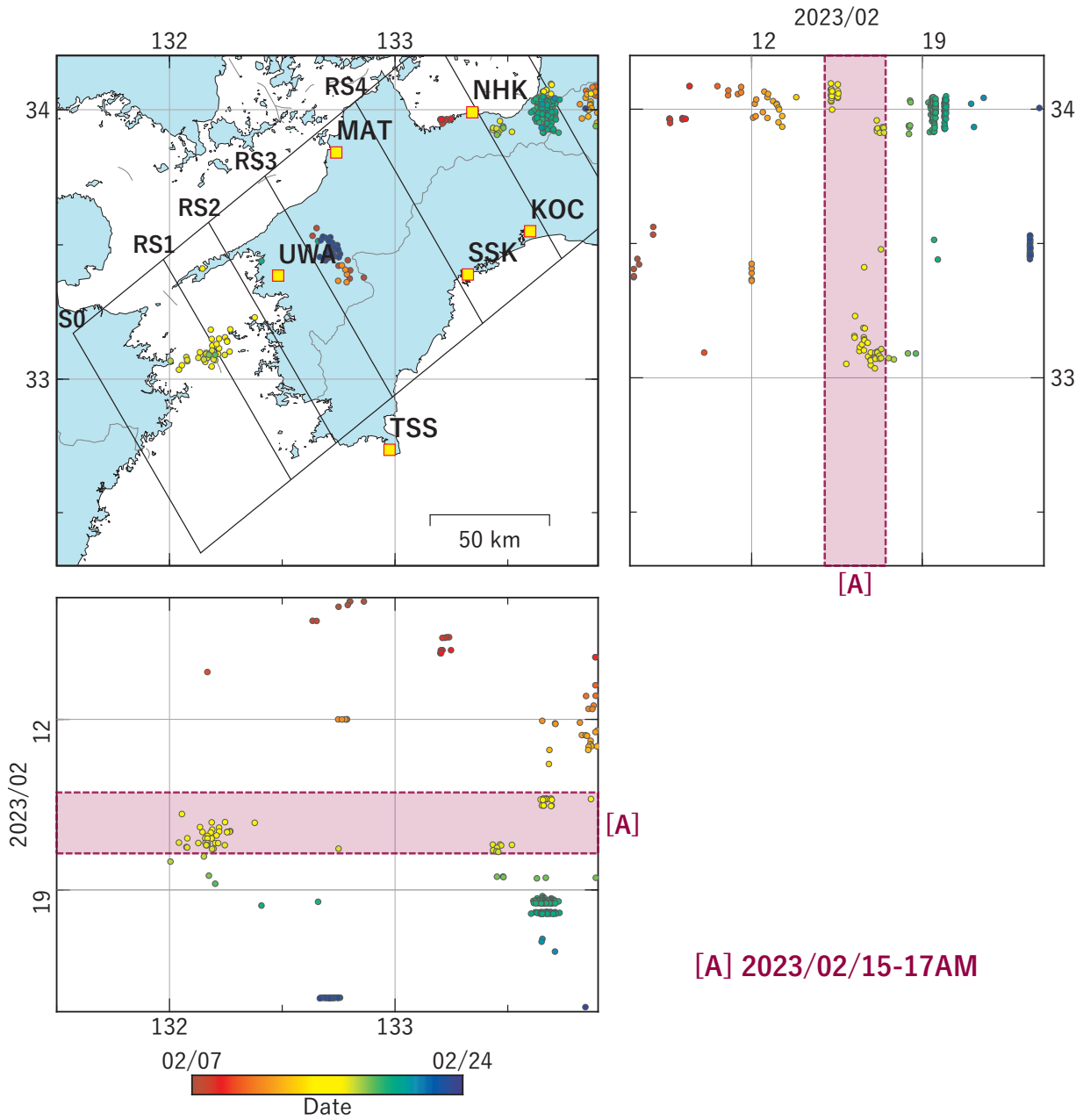
第 20 図 四国西部における低周波地震（気象庁一元化カタログによる）の時空間分布（2023/02/07～2023/02/23）。
