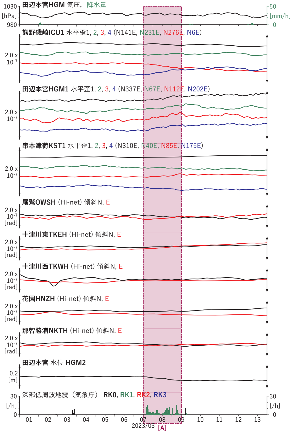
第 24 図 紀伊半島における歪・傾斜・地下水位の観測結果と低周波地震の検出数 (2023/03/01 ~ 2023/03/13).
