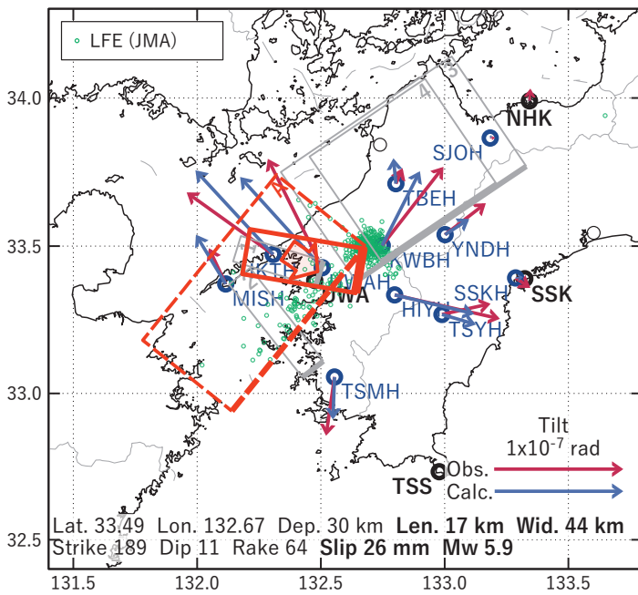
第 10 図 第 8 図 [B] を説明する断層モデル. 各図の説明は第 3 図を参照. Fig. 10 Inferred fault models for Fig. 8[B]. See also the caption of Fig. 3.
