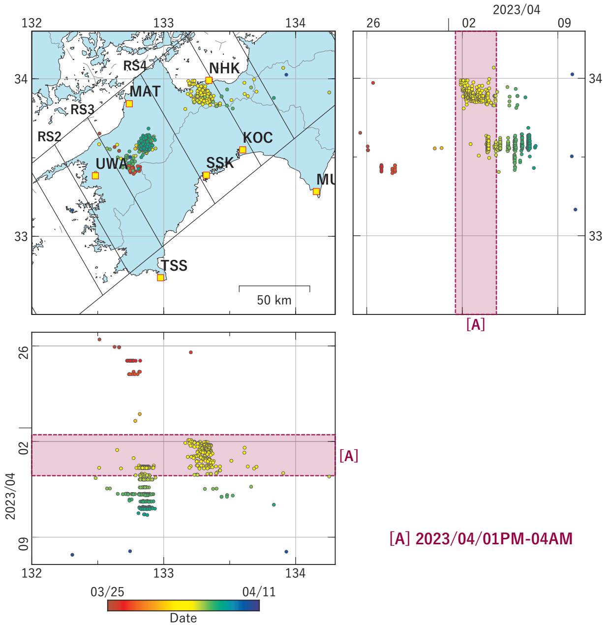
第 32 図 四国西部における低周波地震（気象庁一元化カタログによる）の時空間分布（2023/03/25 ~ 2023/04/10）. Fig. 32 Space-time distribution of low-frequency earthquakes by JMA unified hypocenter catalog in the Western Shikoku from March 25 to April 10, 2023.
