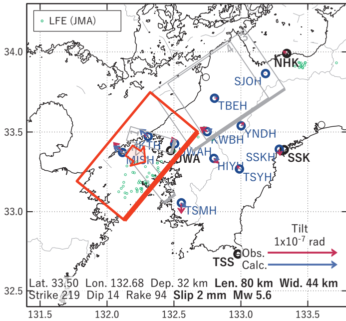
第 9 図 第 8 図 [A] を説明する断層モデル. 各図の説明は第 3 図を参照.
