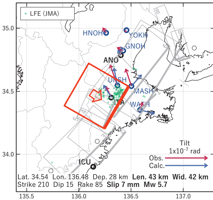
第 37 図 第 36 図 [A] を説明する断層モデル. 各図の説明は第 3 図を参照.
