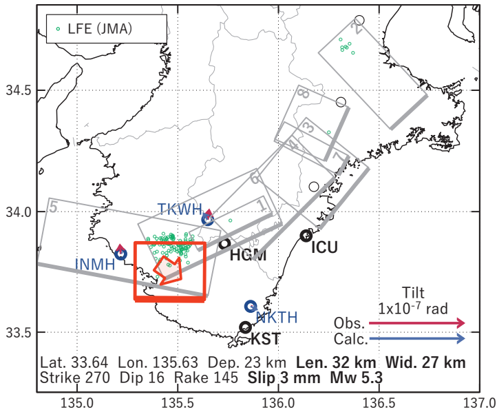
第 19 図 第 18 図 [A] を説明する断層モデル. 各図の説明は第 3 図を参照.
