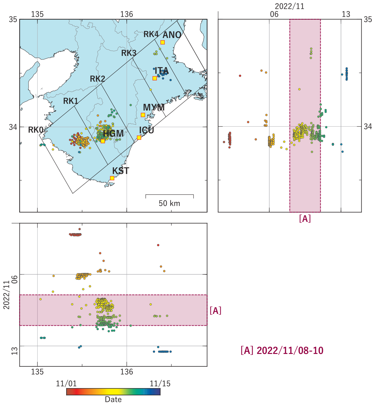
第 4 図 紀伊半島における低周波地震（気象庁一元化カタログによる）の時空間分布（2022/11/01 ～ 2022/11/14）. Fig. 4 Space-time distribution of low-frequency earthquakes by JMA unified hypocenter catalog in the Kii Peninsula from November 01 to 14, 2022.
