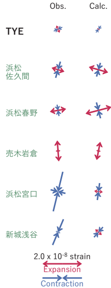
第 3 図 第 2 図 [A] を説明する断層モデル。以下の凡例の説明は以降の同様の図に共通。(図によっては気象庁・静岡県観測点や (b3) 体積歪の結果はない場合がある。) 黒・緑・青の丸印はそれぞれ産総研・気象庁および静岡県・防災科研 Hi-net の観測点、緑の小さな丸印は気象庁の推定した低周波地震。(a) 1 段階目の結果。灰色の濃淡は残差の総和で、赤色矩形が残差の総和が最小となる断層面の位置(大きさは 20x20 km で固定)。(b1) 2 段階目の結果。赤色矩形が残差の総和が最小となる断層面。矢印は傾斜の観測値と計算値の比較。灰色矩形は最近周辺で発生した短期的 SSE の推定断層面(番号との対応は本文参照)。(b2) 主歪の観測値と (b1) に示した断層モデルから求めた計算値との比較。(b3) 体積歪の観測値と (b1) に示した断層モデルから求めた計算値との比較。
