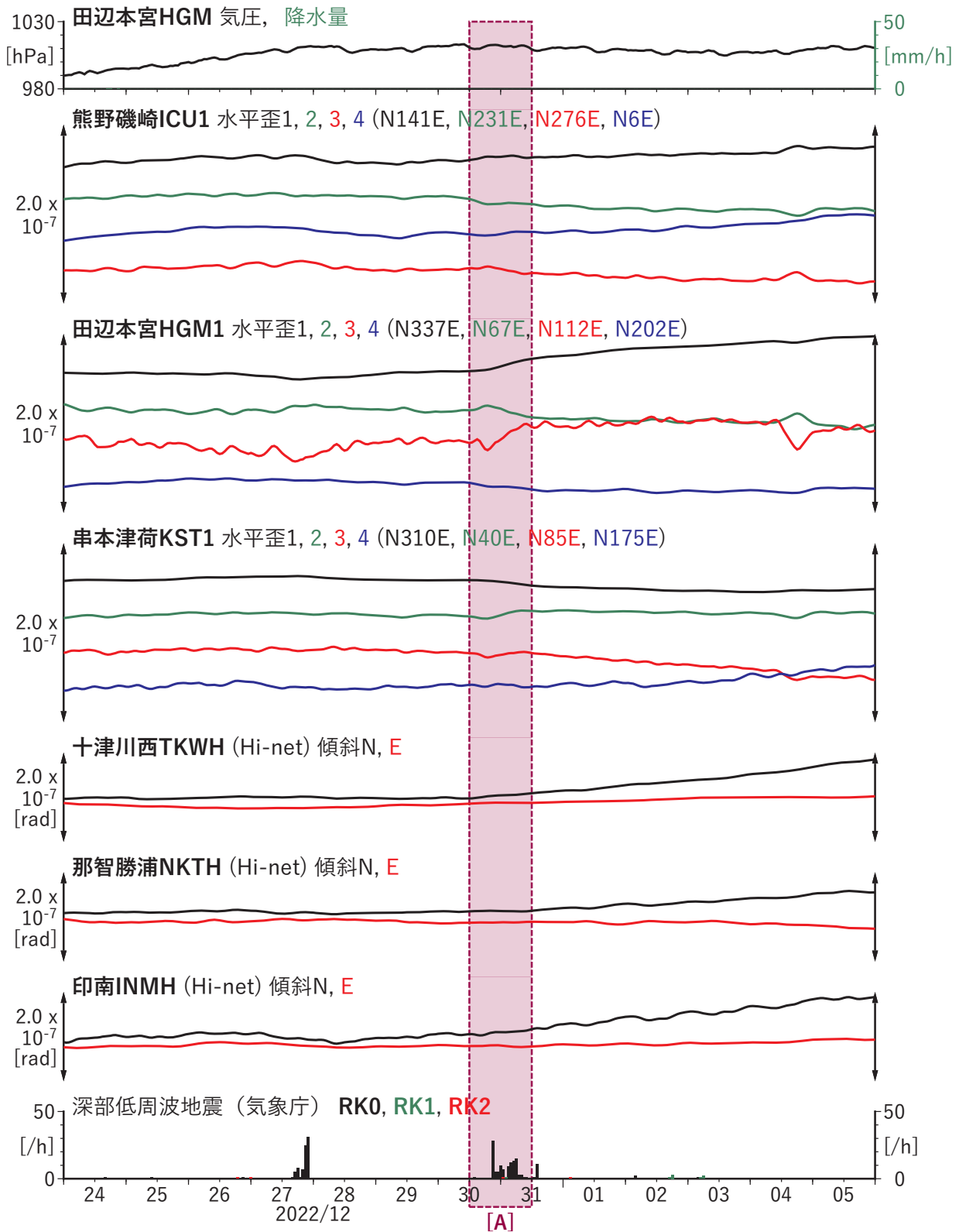
第 18 図 紀伊半島における歪・傾斜の観測結果と低周波地震の検出数 (2022/12/24 ~ 2023/01/05)。
