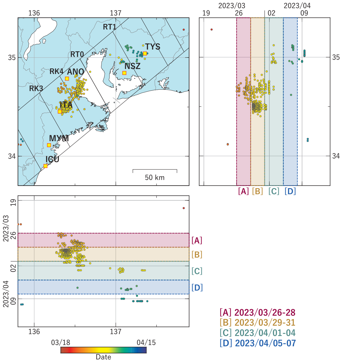
第 26 図 東海地域～紀伊半島における低周波地震（気象庁一元化カタログによる）の時空間分布（2023/03/18 ～ 2023/04/14）.
