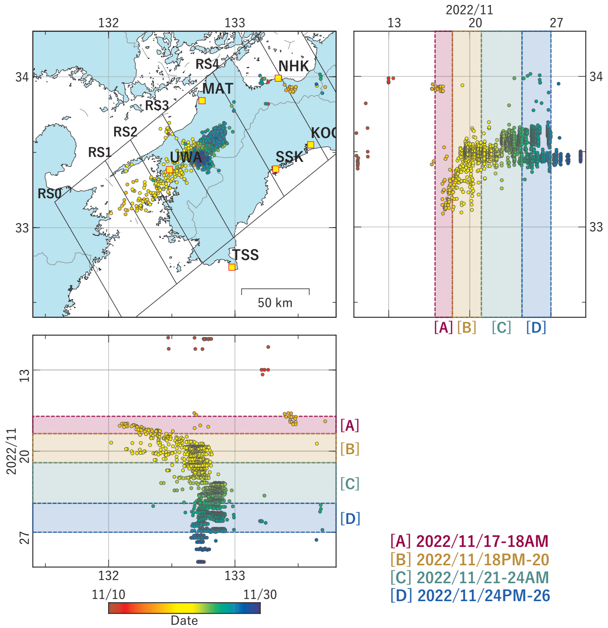
第 7 図 四国西部における低周波地震（気象庁一元化カタログによる）の時空間分布（2022/11/10 ～ 2022/11/29）. Fig. 7 Space-time distribution of low-frequency earthquakes by JMA unified hypocenter catalog in the Western Shikoku from November 10 to 29, 2022.
