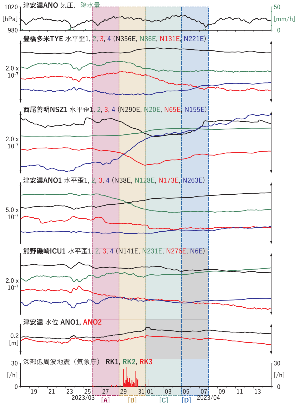
第 27 図 東海地域～紀伊半島における歪・傾斜・地下水位の観測結果と低周波地震の検出数 (2023/03/18 ~ 2023/04/14)。
