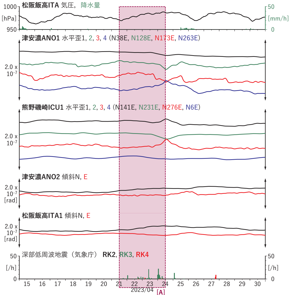
第 36 図 紀伊半島における歪・傾斜の観測結果と低周波地震の検出数 (2023/04/15 ~ 2023/04/30).
