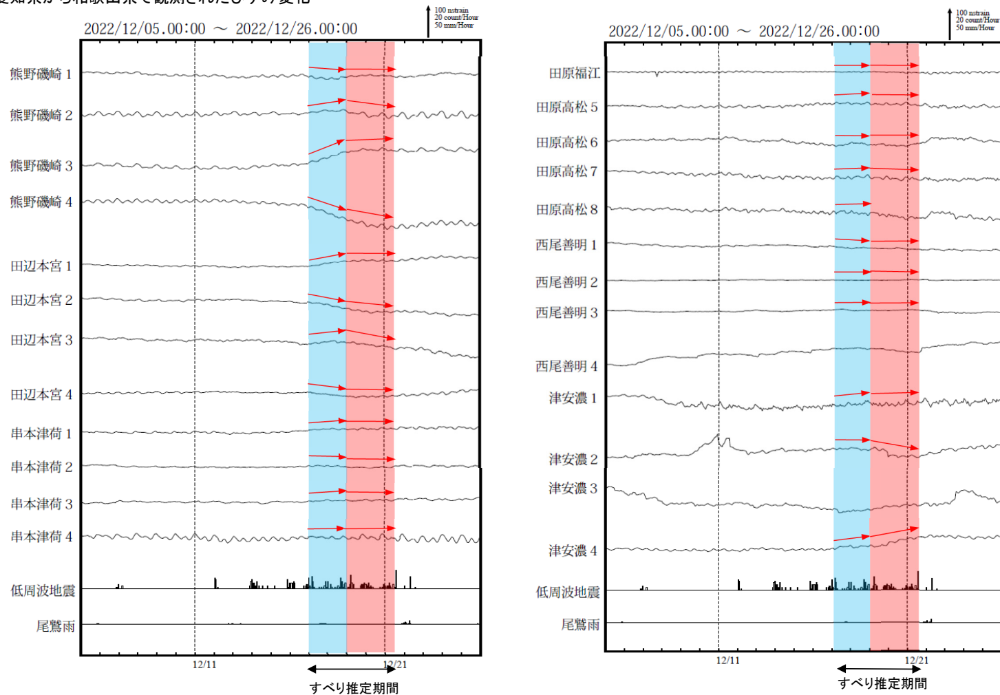
第7図(b) つづき Fig.7(b) Continued.
