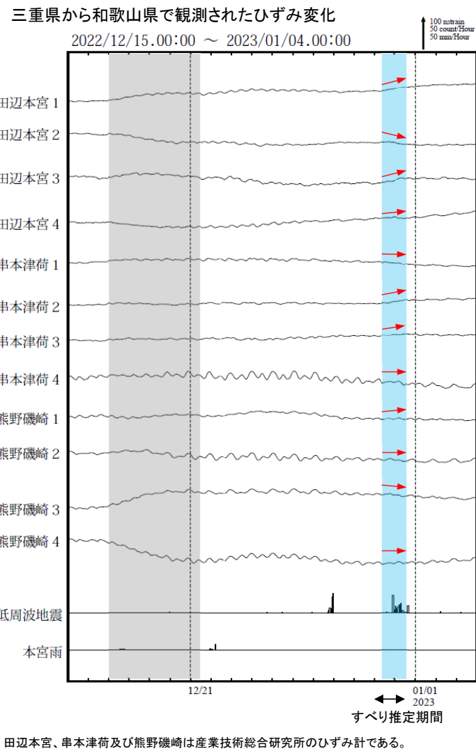
第8図(b) つづき Fig.8(b) Continued.
