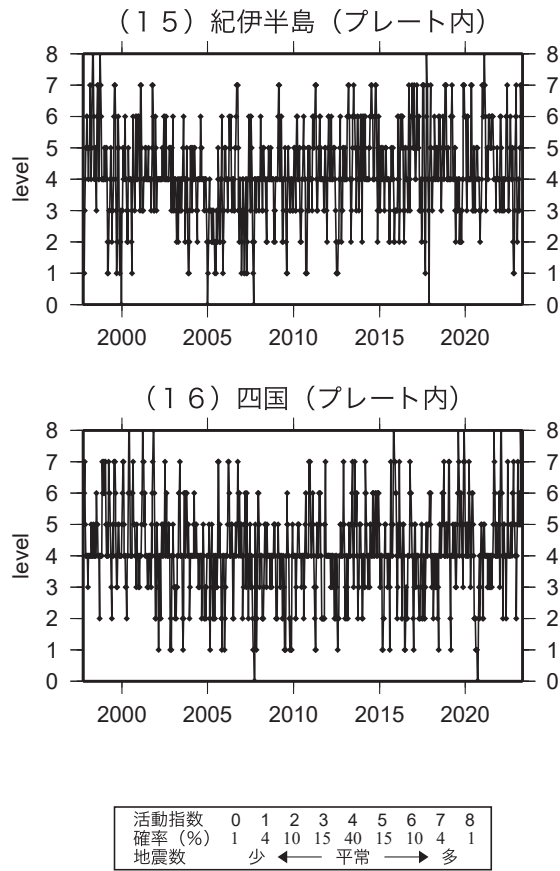
第 17 図 (c) つづき
