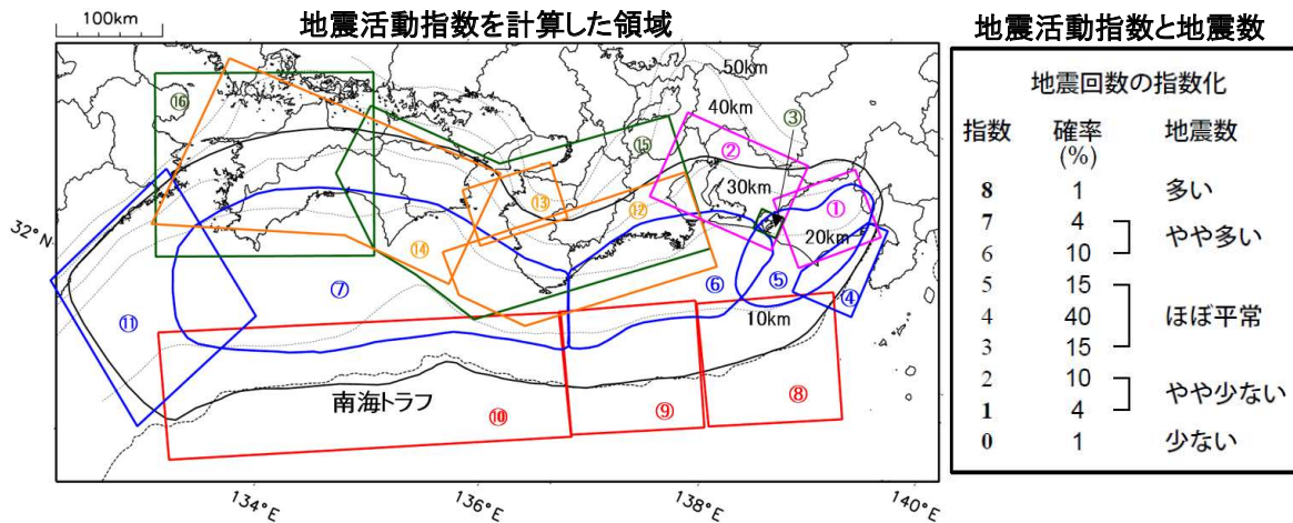
第 16 図 南海トラフ周辺の地震活動指数の表
