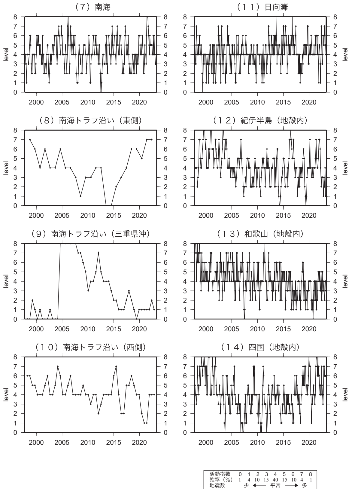
第 17 図 (b) つづき Fig.17(b) Continued.
