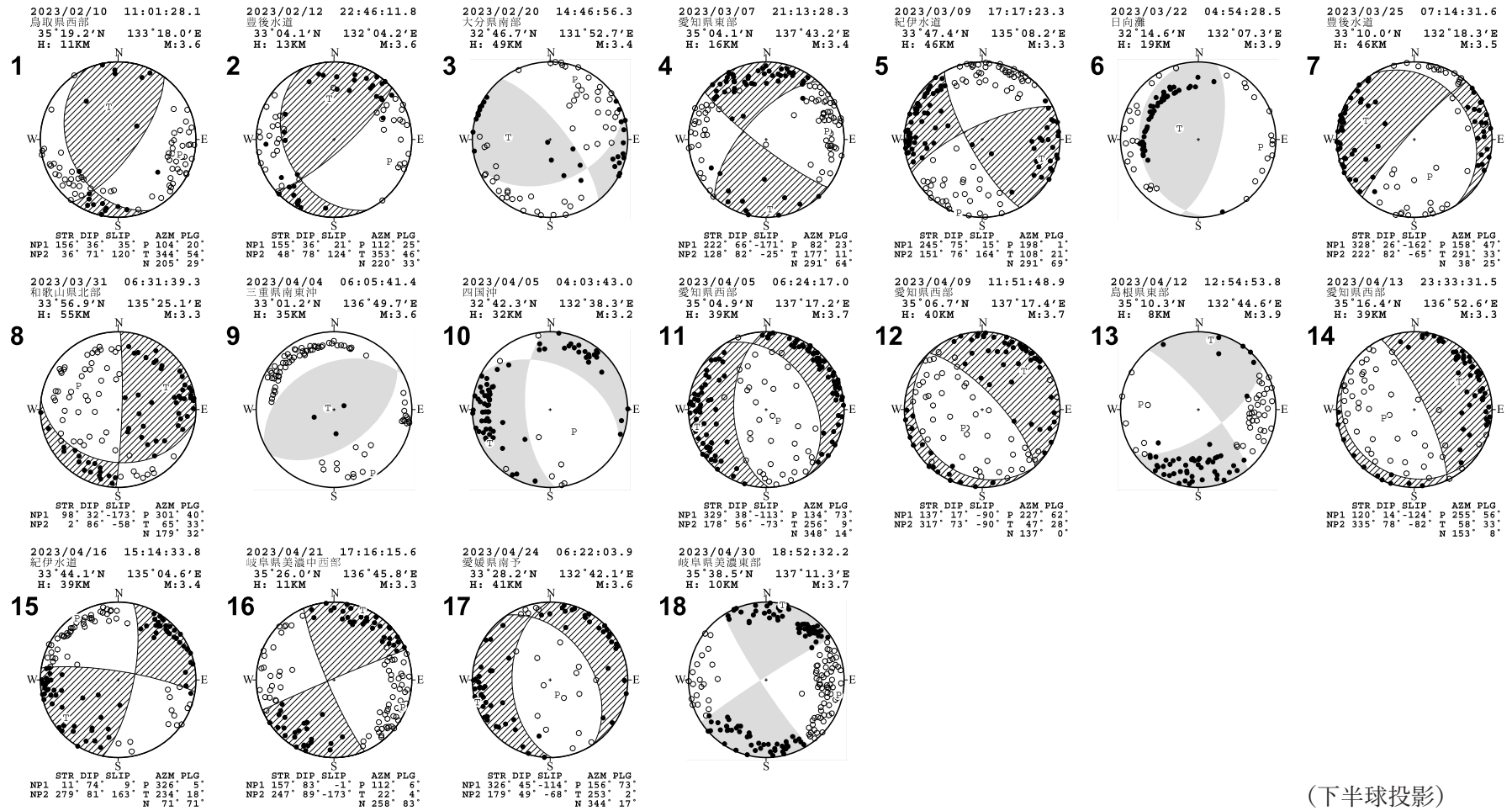
第3図 (d) つづき (2023年2月~4月) Fig.3(d) Continued (February - April 2023).
