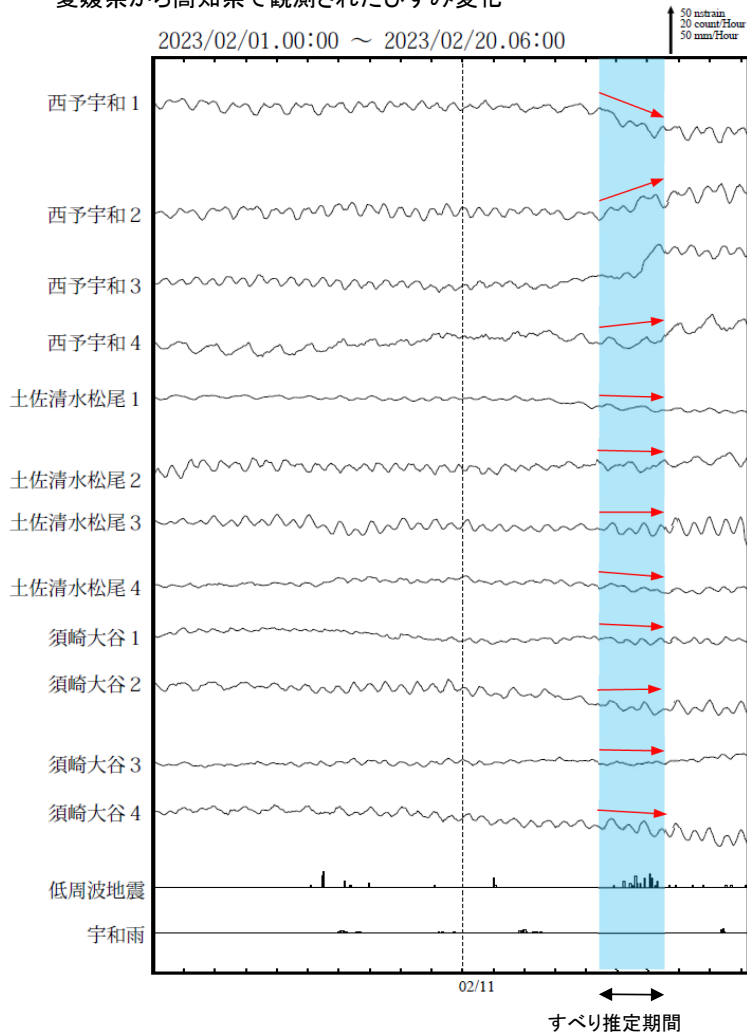
第9図(b) つづき Fig.9(b) Continued.
