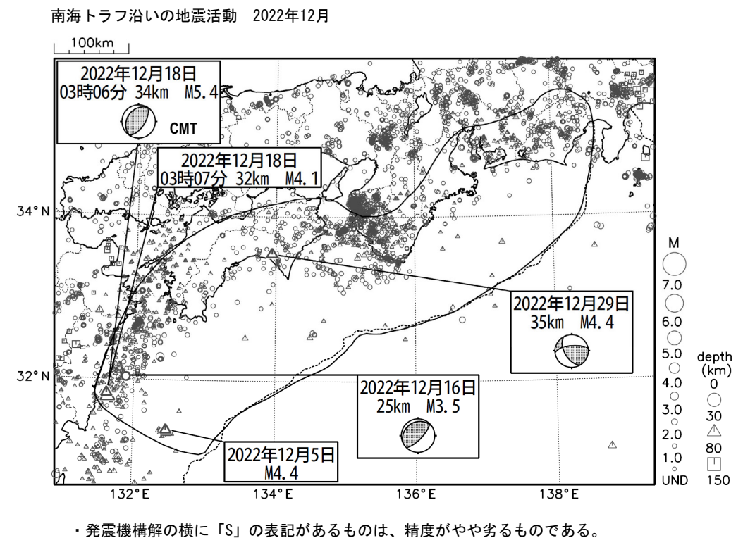
第 1 図 (b) つづき (2022 年 12 月) Fig.1(b) Monthly epicenter distribution in and around the Nankai Trough (December 2022).
