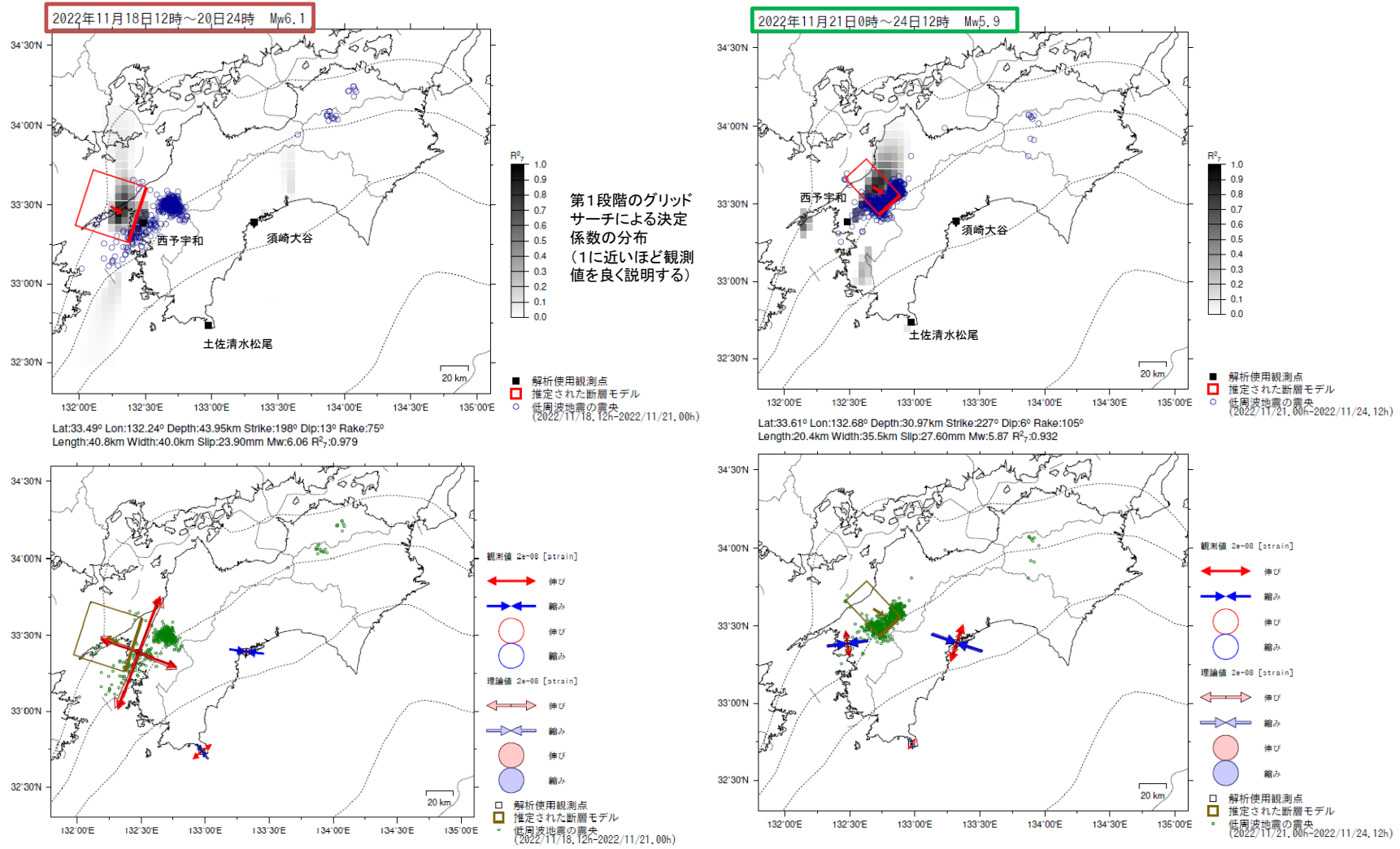
第6図(b) つづき Fig.6(b) Continued.
