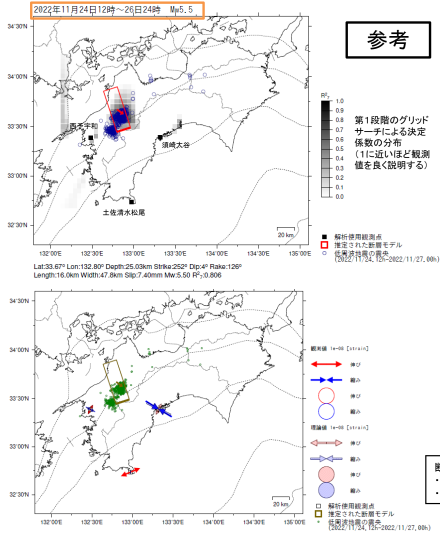
第6図(b) つづき Fig.6(b) Continued.
