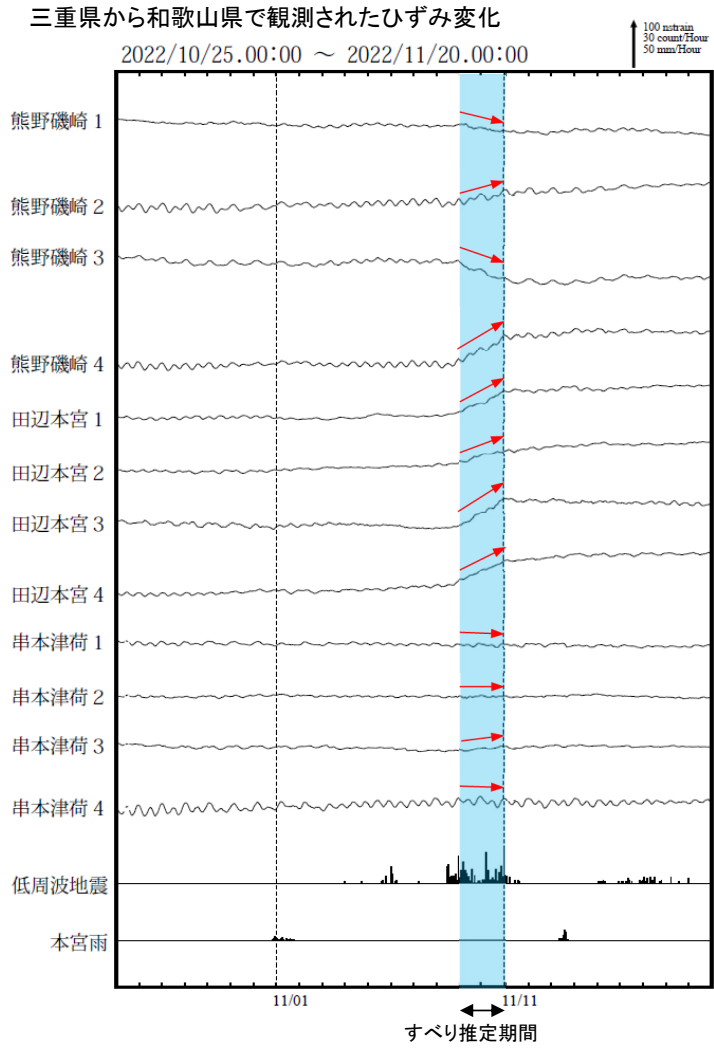
第5図(b) つづき Fig.5(b) Continued.
