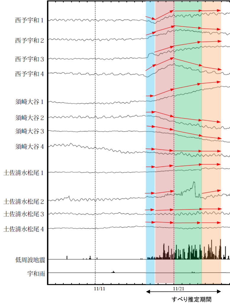
第 6 図 (b) つづき Fig.6(b) Continued.
