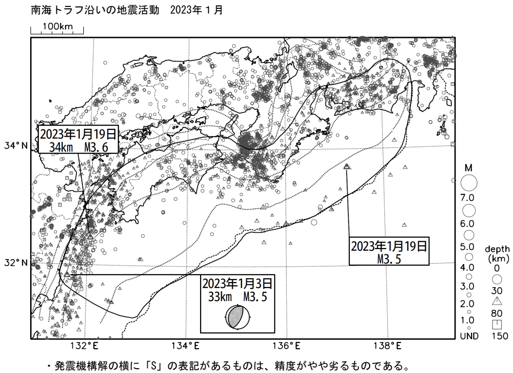
第 1 図 (c) つづき (2023 年 1 月)
