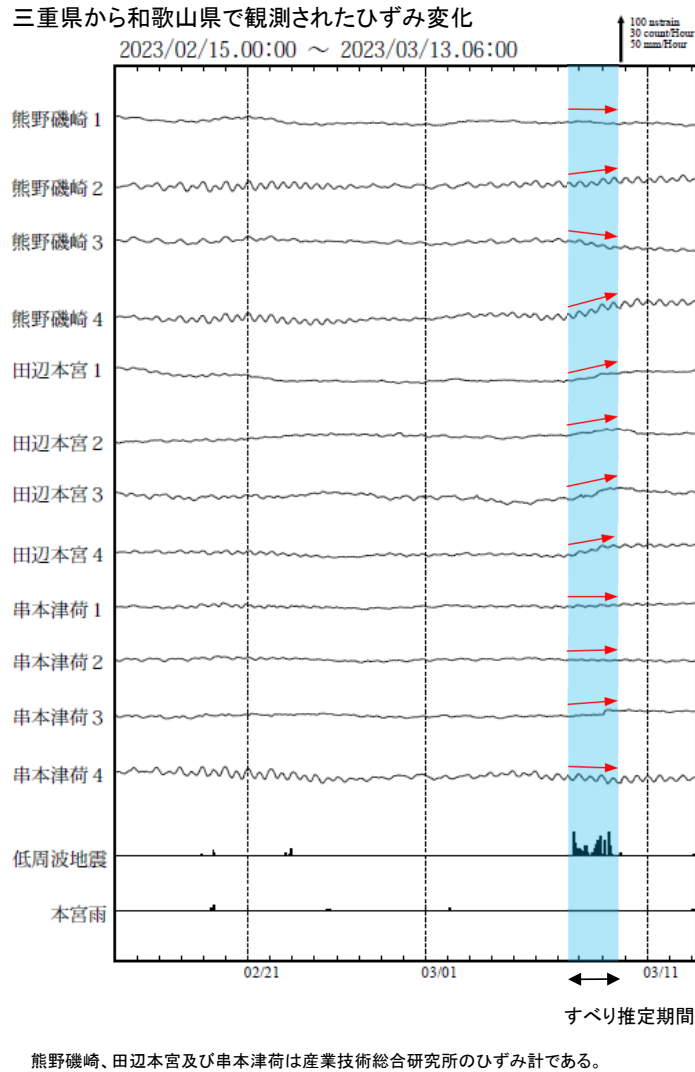
第10図 (b) つづき Fig.10(b) Continued.
