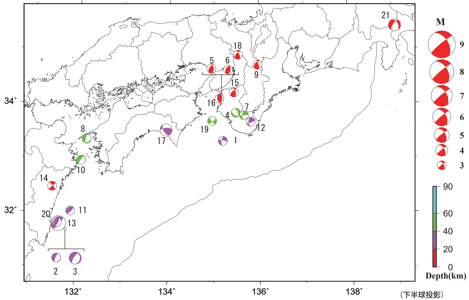
第3図 (a) 南海トラフ周辺で発生した主な地震の発震機構解 (2022年11月～2023年1月)
