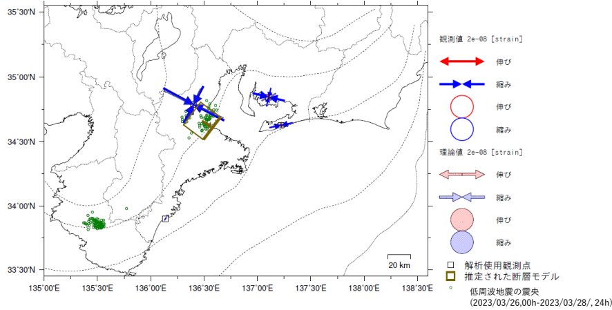
第11図 (b) つづき Fig.11(b) Continued.
