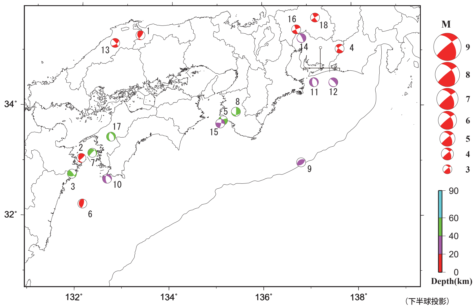
第3図(c) つづき (2023年2月～4月) Fig.3(c) Continued (February – April 2023).
