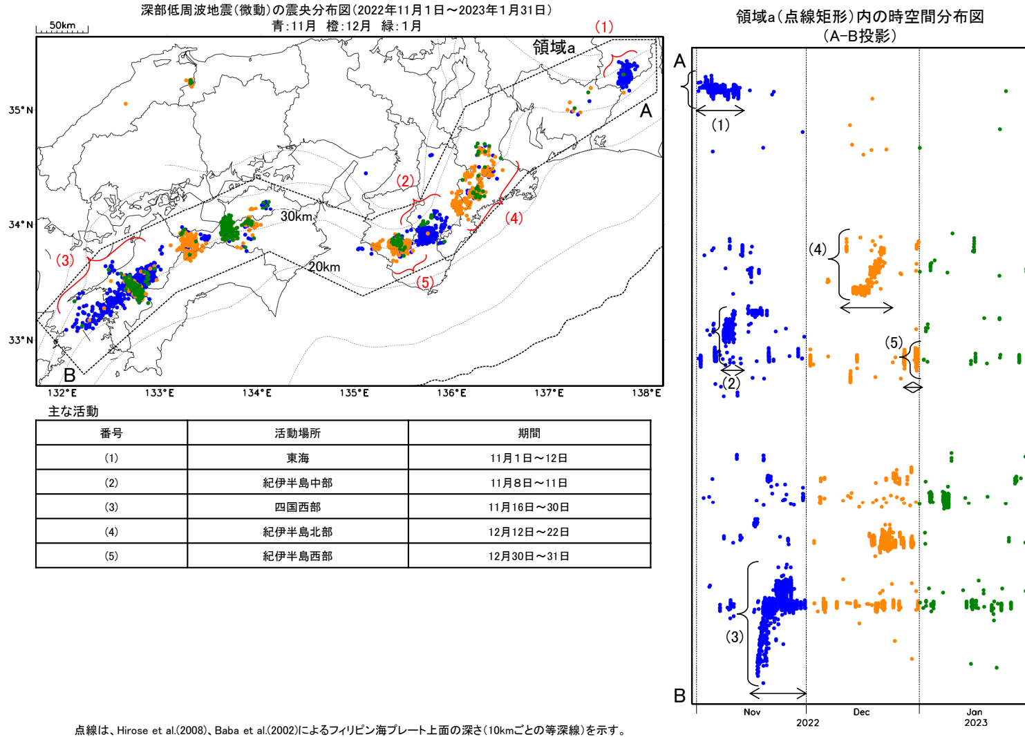
第2図(a) 東海地域から豊後水道にかけての深部低周波地震活動(2022年11月~2023年1月). Fig.2(a) Seismic activity of Low-Frequency Events from the Tokai region to the Bungo Channel (November 2022 – January 2023).
