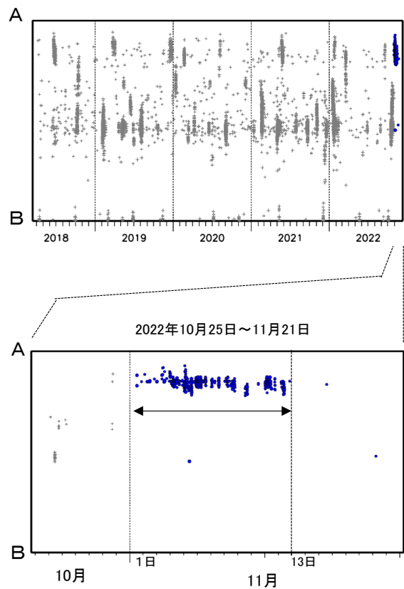
第 4 図 (a) 東海の深部低周波地震活動とひずみ変化, 及び推定されるゆっくりすべり領域
