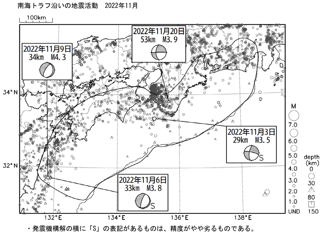
第 1 図 (a) 南海トラフ周辺の月別震央分布 (2022 年 11 月) Fig.1(a) Monthly epicenter distribution in and around the Nankai Trough (November 2022).
