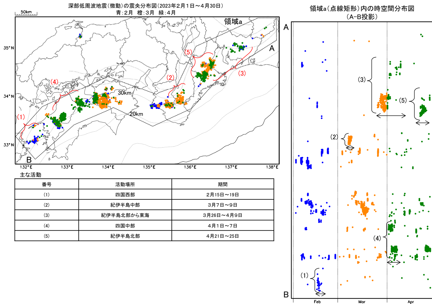
第2図(c) 東海地域から豊後水道にかけての深部低周波地震活動(2023年2月~4月)。
