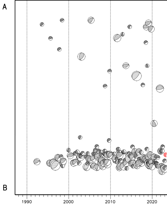
第 15 図 想定南海トラフ地震の発震機構解と類似の型の地震
