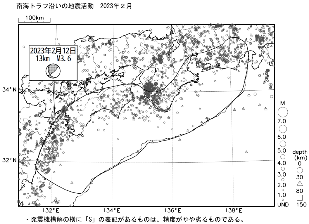
第 1 図 (d) つづき (2023 年 2 月)
