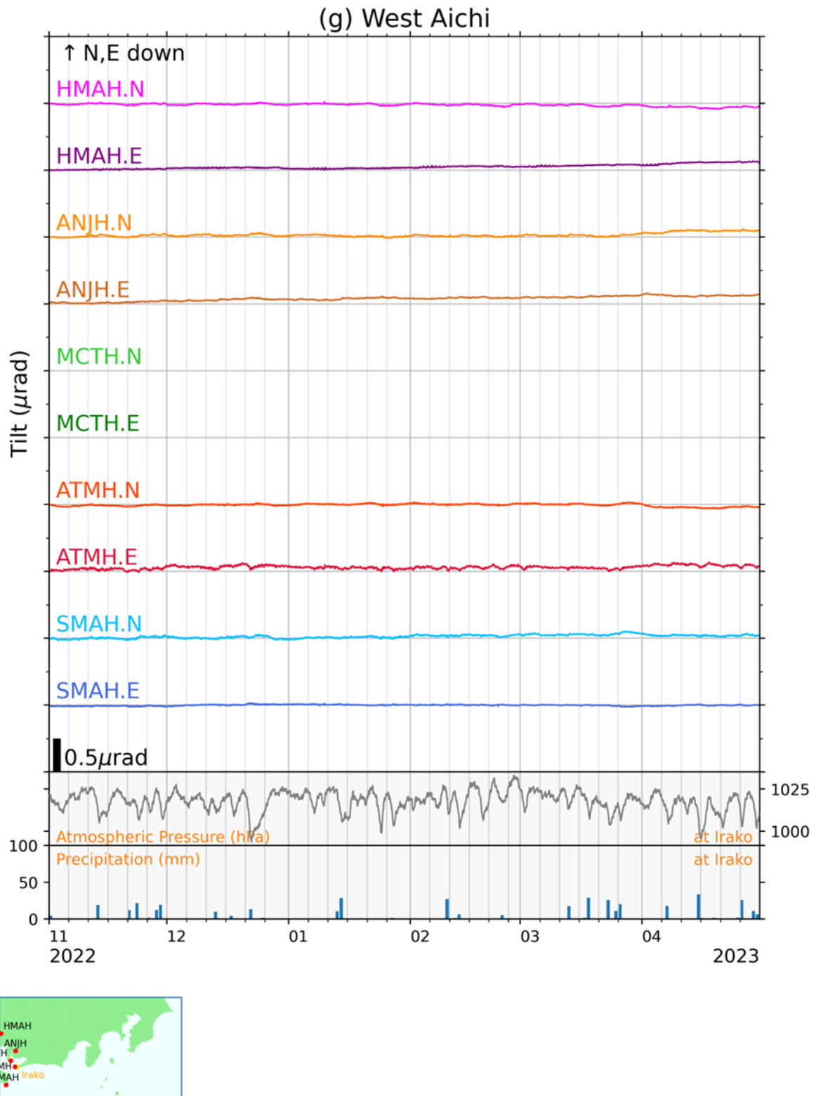
第 2 図 (g) 傾斜の時間値記録（愛知西部）及び気圧・日雨量（伊良湖）. Fig. 2 (g) Hourly tilt record in west Aichi, and atmospheric pressure and daily precipitation at Irako.
