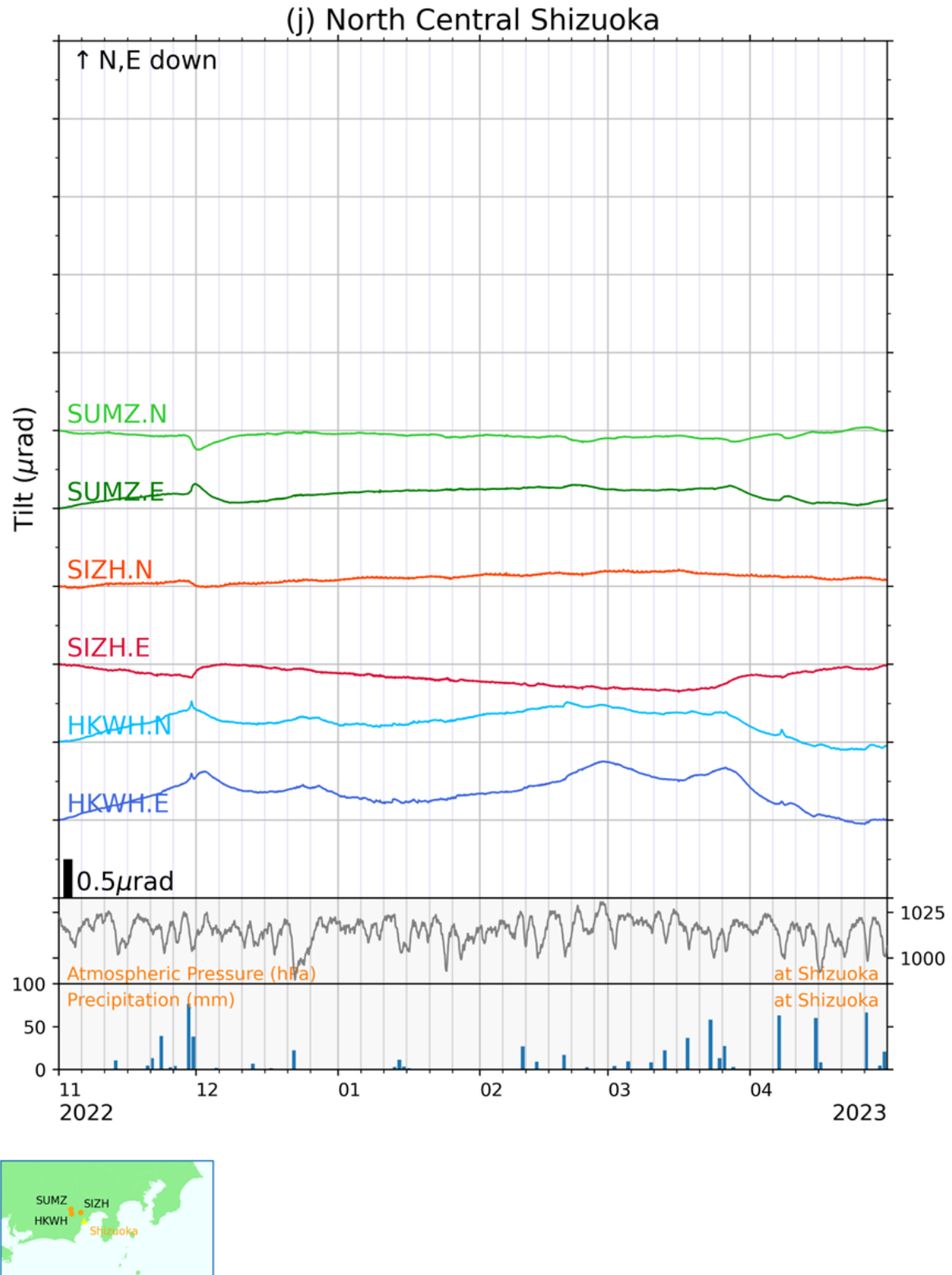
第 2 図 (j) 傾斜の時間値記録（静岡中北部）及び気圧・日雨量（静岡）。
