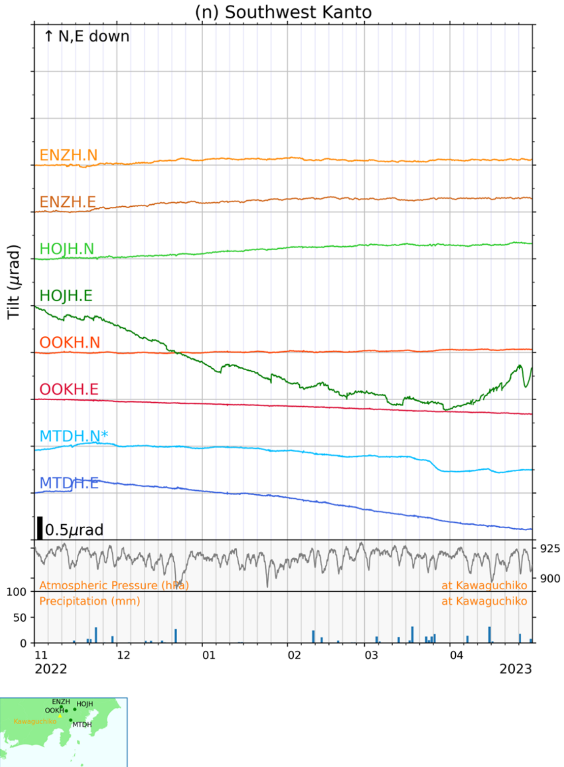
第 2 図 (n) 傾斜の時間値記録（関東南西部）及び気圧・日雨量（河口湖）。
