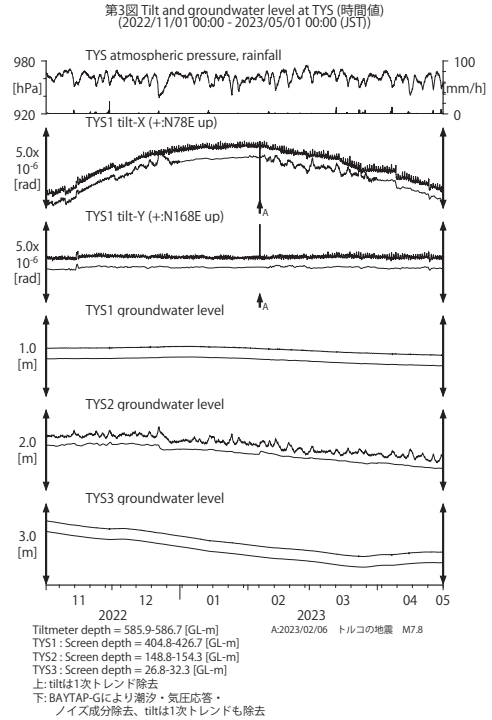
第 3 図 TYS における傾斜・地下水位観測結果 (2022 年 11 月 ~ 2023 年 4 月) Fig. 3 Observed tilts and groundwater levels at the TYS observation site from November 2022 to April 2023.
