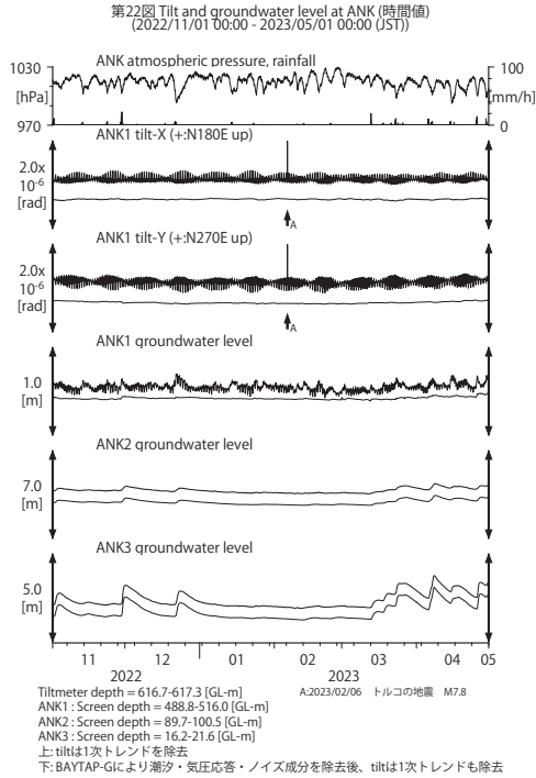
第 22 図 ANK における傾斜・地下水位観測結果 (2022 年 11 月～2023 年 4 月) Fig. 22 Observed tilts and groundwater levels at the ANK observation site from November 2022 to April 2023.
