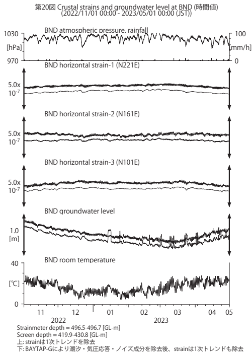
第 20 図 BND における歪・地下水位観測結果 (2022 年 11 月～2023 年 4 月) Fig. 20 Observed strains and groundwater level at the BND observation site from November 2022 to April 2023.
