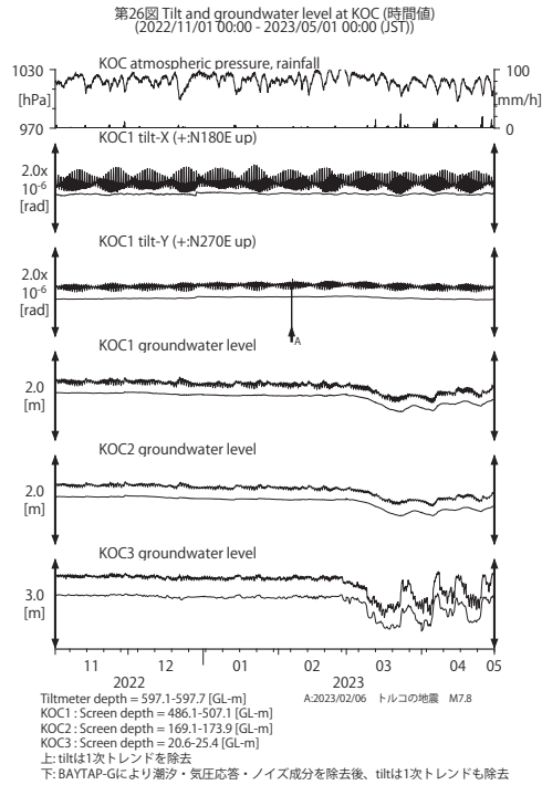
第 26 図 KOC における傾斜・地下水位観測結果 (2022 年 11 月～2023 年 4 月)
