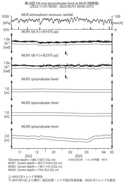
第 24 図 MUR における傾斜・地下水位観測結果 (2022 年 11 月～2023 年 4 月) Fig. 24 Observed tilts and groundwater levels at the MUR observation site from November 2022 to April 2023.
