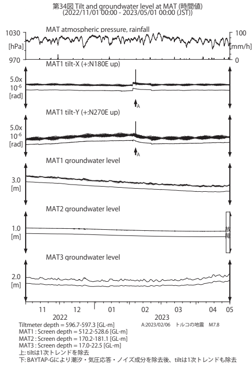
第 34 図 MAT における傾斜・地下水位観測結果 (2022 年 11 月～2023 年 4 月) Fig. 34. Observed tilts and groundwater levels at the MAT observation site from November 2022 to April 2023.
