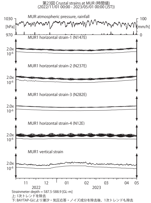
第 23 図 MUR における歪観測結果 (2022 年 11 月～2023 年 4 月) Fig. 23 Observed strains at the MUR observation site from November 2022 to April 2023.
