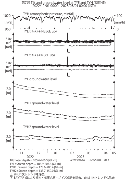
第 7 図 TYE および TYH における傾斜・地下水位観測結果 (2022 年 11 月 ~ 2023 年 4 月) Fig. 7 Observed tilts and groundwater levels at the TYE and the TYH observation site from November 2022 to April 2023.
