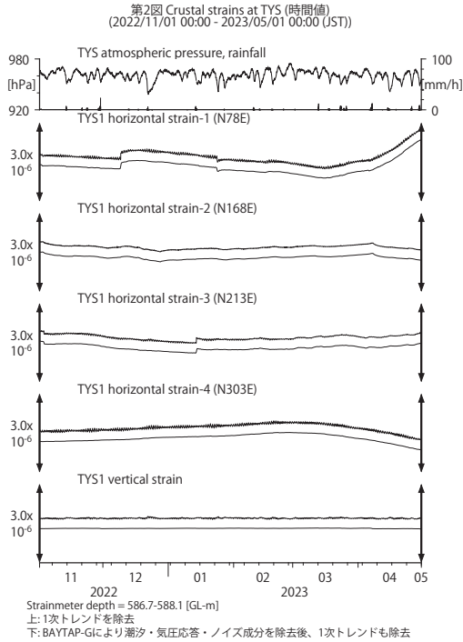
第 2 図 TYS における歪観測結果 (2022 年 11 月 ~ 2023 年 4 月) Fig. 2 Observed strains at the TYS observation site from November 2022 to April 2023.
