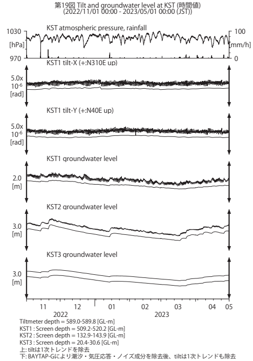
第 19 図 KST における傾斜・地下水位観測結果 (2022 年 11 月～2023 年 4 月) Fig. 19 Observed tilts and groundwater levels at the KST observation site from November 2022 to April 2023.
