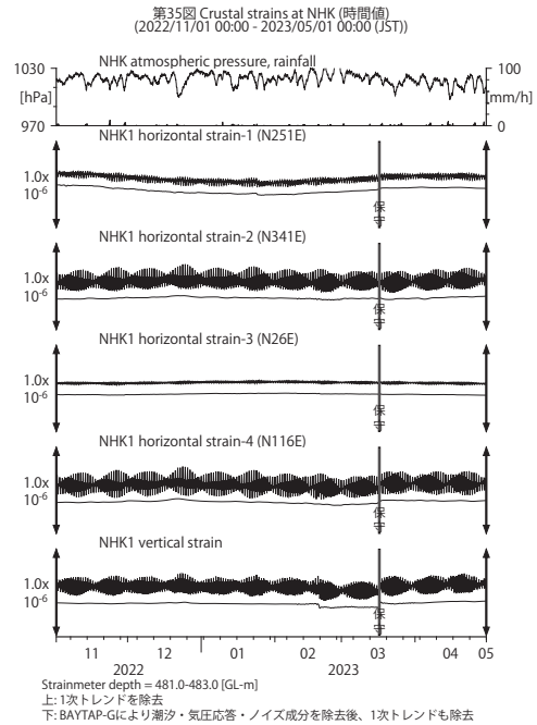
第 35 図 NHK における歪観測結果 (2022 年 11 月～2023 年 4 月) Fig. 35. Observed strains at the NHK observation site from November 2022 to April 2023.
