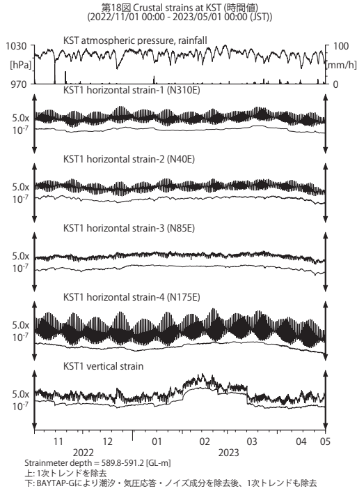
第 18 図 KST における歪観測結果 (2022 年 11 月～2023 年 4 月) Fig. 18 Observed strains at the KST observation site from November 2022 to April 2023.
