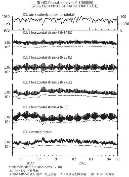
第 14 図 ICU における歪観測結果 (2022 年 11 月～2023 年 4 月) Fig. 14 Observed strains at the ICU observation site from November 2022 to April 2023.
