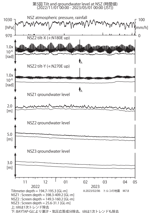
第 5 図 NSZ における傾斜・地下水位観測結果 (2022 年 11 月 ~ 2023 年 4 月) Fig. 5 Observed tilts and groundwater levels at the NSZ observation site from November 2022 to April 2023.
