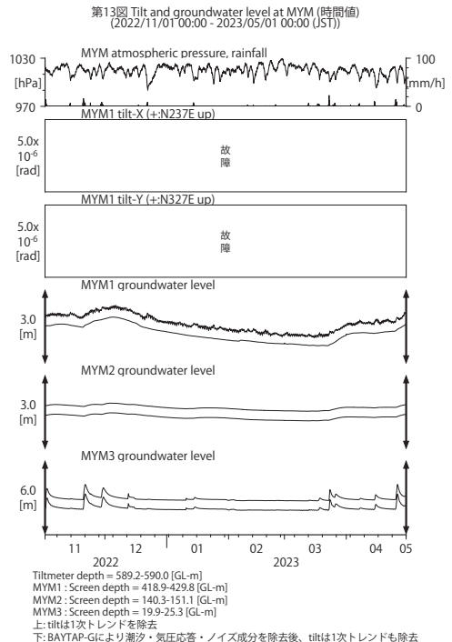
第 13 図 MYM における傾斜・地下水位観測結果 (2022 年 11 月～2023 年 4 月) Fig. 13 Observed tilts and groundwater levels at the MYM observation site from November 2022 to April 2023.
