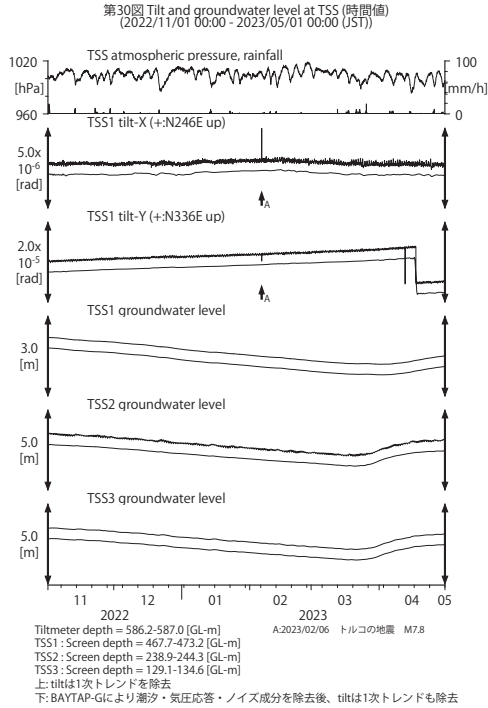
第 30 図 TSS における傾斜・地下水位観測結果 (2022 年 11 月～2023 年 4 月) Fig. 30. Observed tilts and groundwater levels at the TSS observation site from November 2022 to April 2023.
