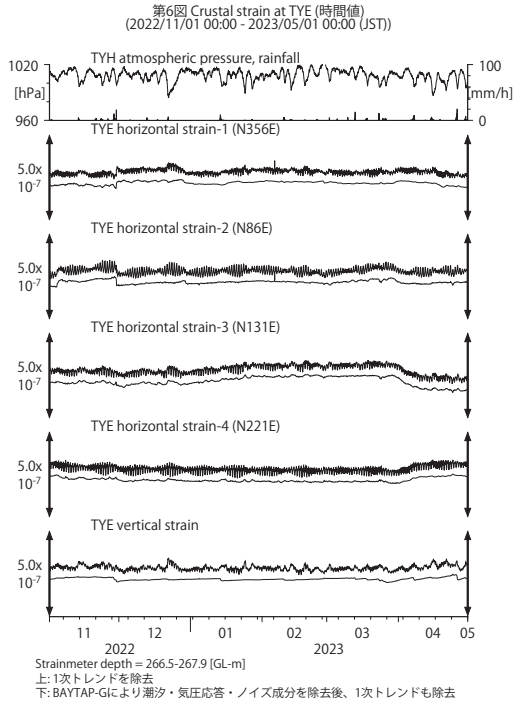
第 6 図 TYE における歪観測結果 (2022 年 11 月 ~ 2023 年 4 月) Fig. 6 Observed strains at the TYE observation site from November 2022 to April 2023.
