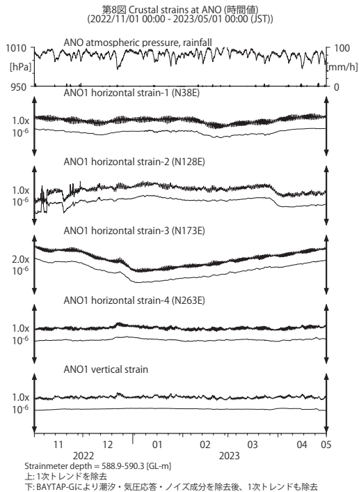
第 8 図 ANO における歪観測結果 (2022 年 11 月 ~ 2023 年 4 月) Fig. 8 Observed strains at the ANO observation site from November 2022 to April 2023.
