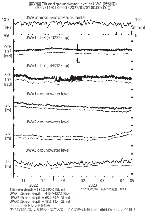
第 32 図 UWA における傾斜・地下水位観測結果 (2022 年 11 月～2023 年 4 月) Fig. 32. Observed tilts and groundwater levels at the UWA observation site from November 2022 to April 2023.
