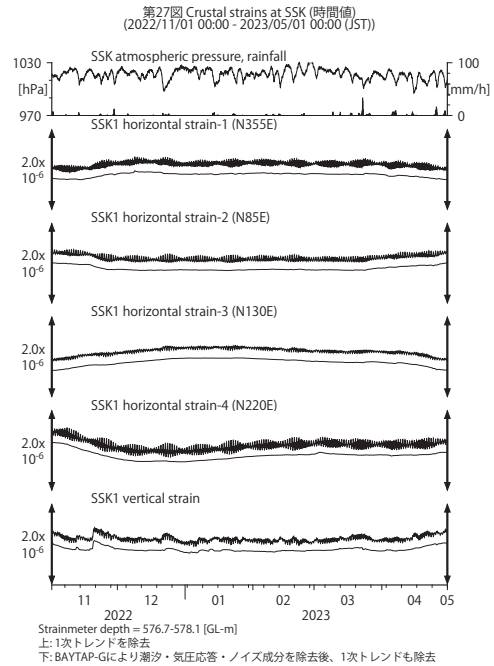
第 27 図 SSK における歪観測結果 (2022 年 11 月～2023 年 4 月)
