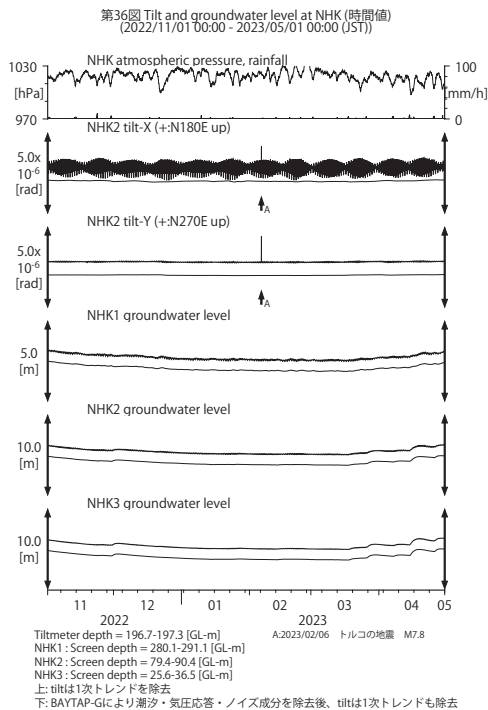
第 36 図 NHK における傾斜・地下水位観測結果 (2022 年 11 月～2023 年 4 月) Fig. 36. Observed tilts and groundwater levels at the NHK observation site from November 2022 to April 2023.
