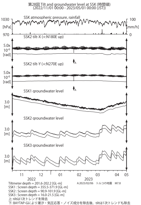
第 28 図 SSK における傾斜・地下水位観測結果 (2022 年 11 月～2023 年 4 月)
