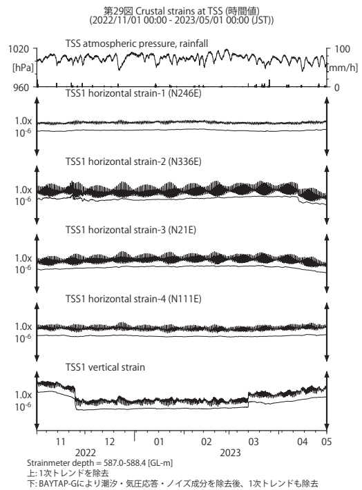
第 29 図 TSS における歪観測結果 (2022 年 11 月～2023 年 4 月)
