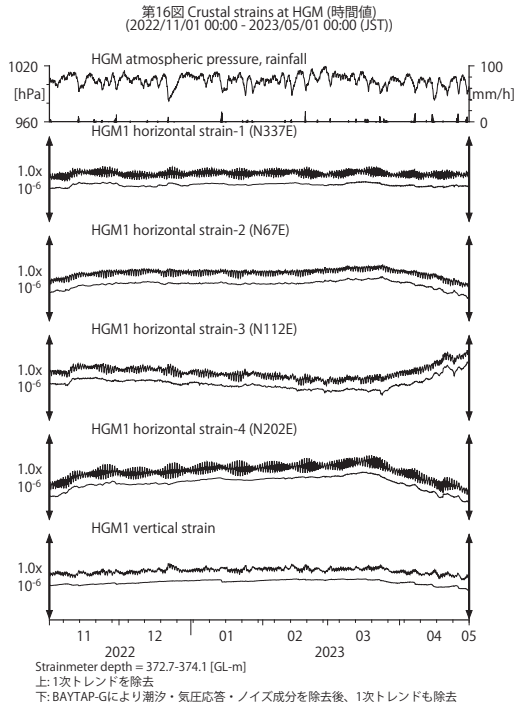
第 16 図 HGM における歪観測結果 (2022 年 11 月～2023 年 4 月) Fig. 16 Observed strains at the HGM observation site from November 2022 to April 2023.
