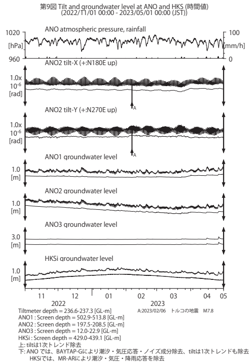
第 9 図 ANO および HKS における傾斜・地下水位観測結果 (2022 年 11 月 ~ 2023 年 4 月) Fig. 9 Observed tilts and groundwater levels at the ANO and the HKS observation site from November 2022 to April 2023.
