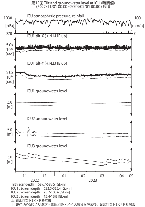
第 15 図 ICU における傾斜・地下水位観測結果 (2022 年 11 月～2023 年 4 月) Fig. 15 Observed tilts and groundwater levels at the ICU observation site from November 2022 to April 2023.
