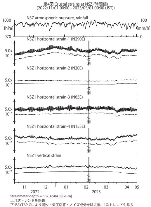
第 4 図 NSZ における歪観測結果 (2022 年 11 月 ~ 2023 年 4 月) Fig. 4 Observed strains at the NSZ observation site from November 2022 to April 2023.
