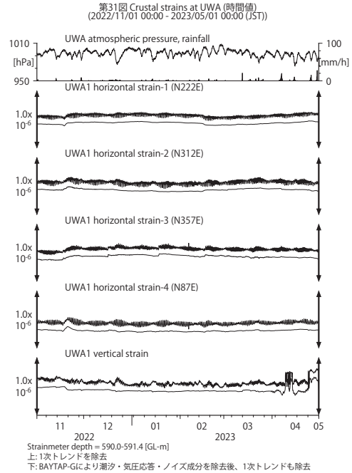
第 31 図 UWA における歪観測結果 (2022 年 11 月～2023 年 4 月) Fig. 31. Observed strains at the UWA observation site from November 2022 to April 2023.
