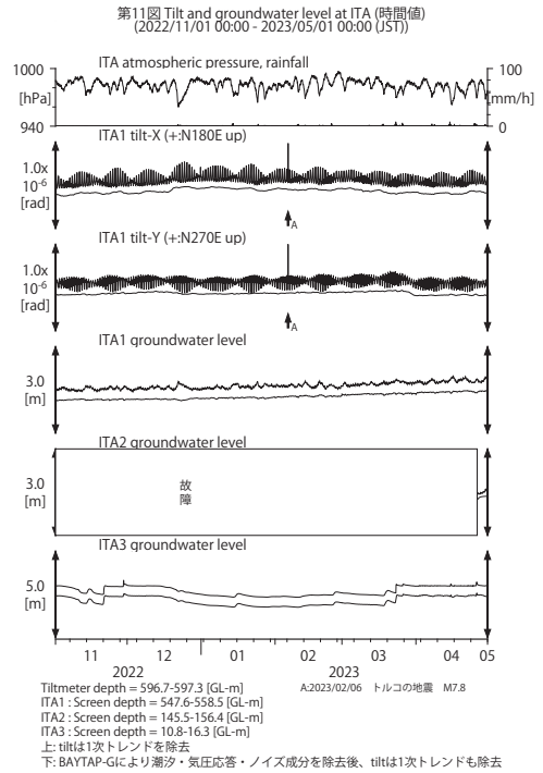
第 11 図 ITA における傾斜・地下水位観測結果 (2022 年 11 月～2023 年 4 月) Fig. 11 Observed tilts and groundwater levels at the ITA observation site from November 2022 to April 2023.
