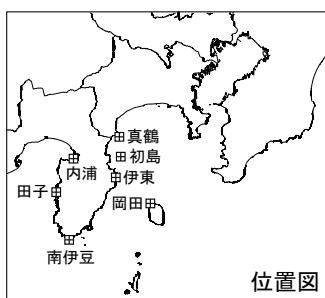
第 17 図 加藤・津村 (1979) の方法による験潮場の上下変動
