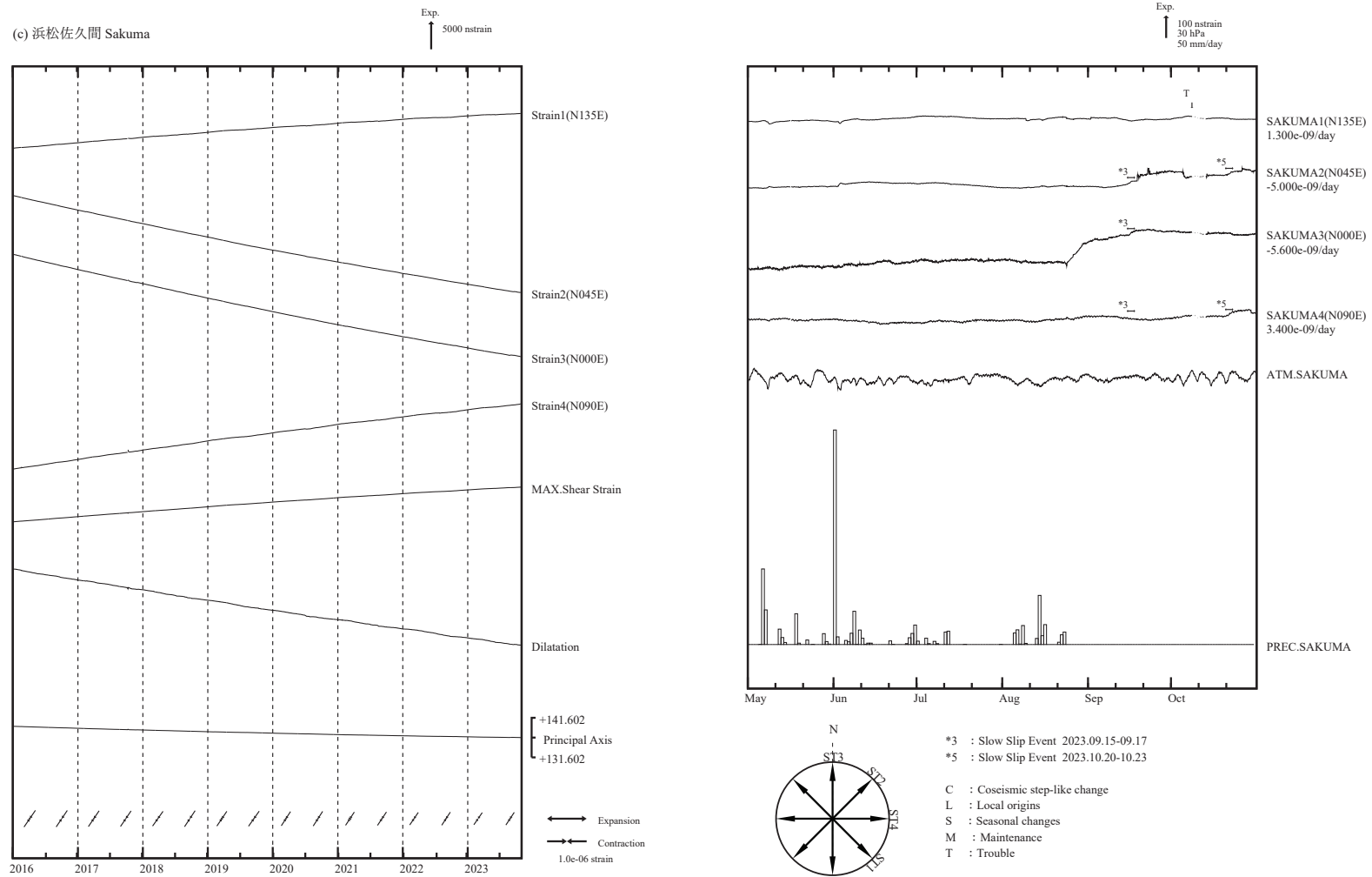
第 4 図 (c) 左 : 2016 年 1 月以後の多成分ひずみ計変化 (日平均値)。主ひずみ・最大せん断ひずみ・面積ひずみは各方向成分から計算されている。 右 : 2023 年 5 月～10 月の多成分ひずみ計変化 (時間値 : 気圧・潮汐・地磁気・降水補正した値)。各図下部に気圧変化と降水量を示す。
