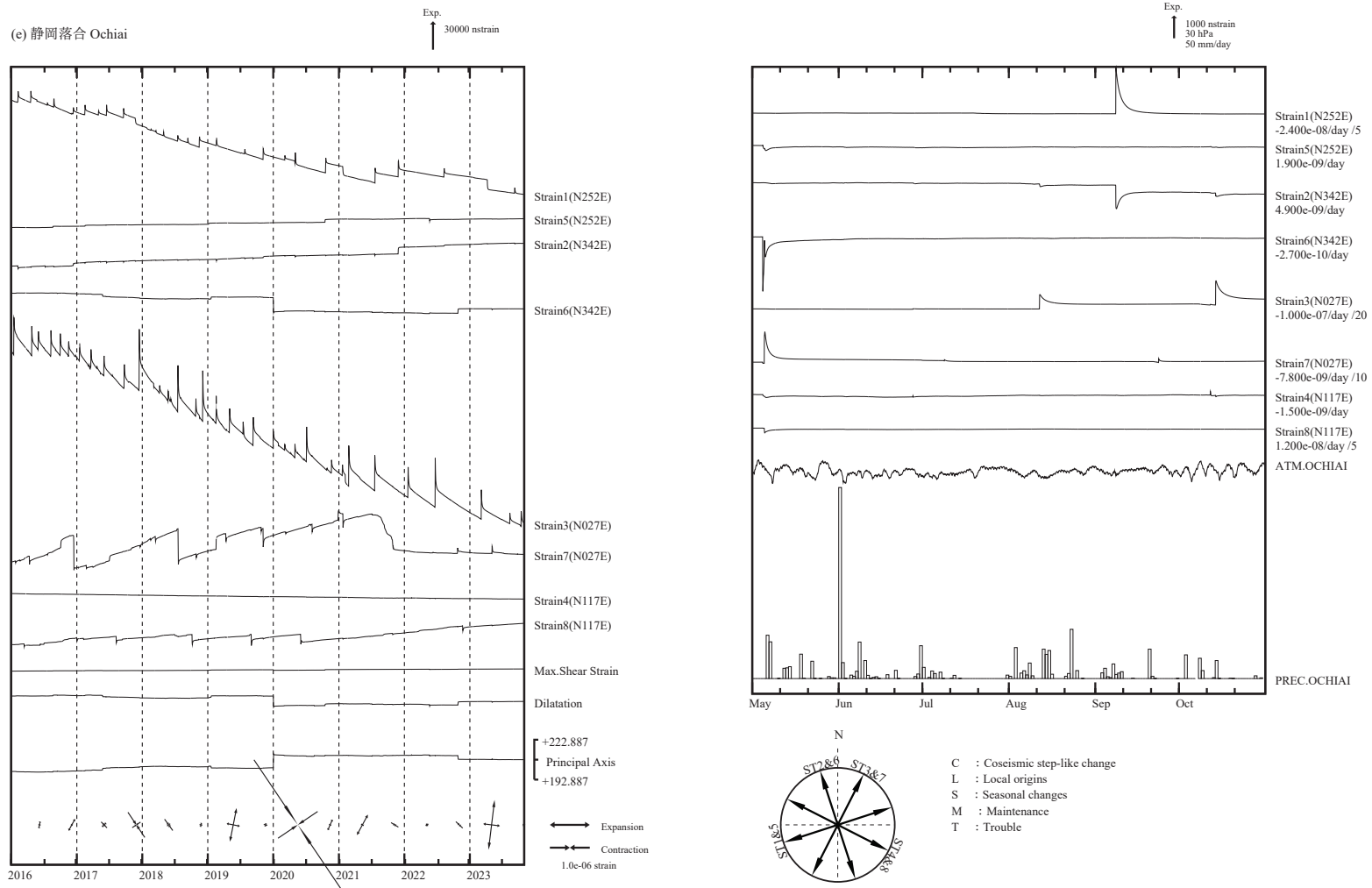
第 4 図 (e) 左：2016 年 1 月以後の多成分ひずみ計変化（日平均値）。主ひずみ・最大せん断ひずみ・面積ひずみは各方向成分から計算されている。 右：2023 年 5 月～10 月の多成分ひずみ計変化（時間値：気圧・潮汐・地磁気・降水補正した値）。各図下部に気圧変化と降水量を示す。
