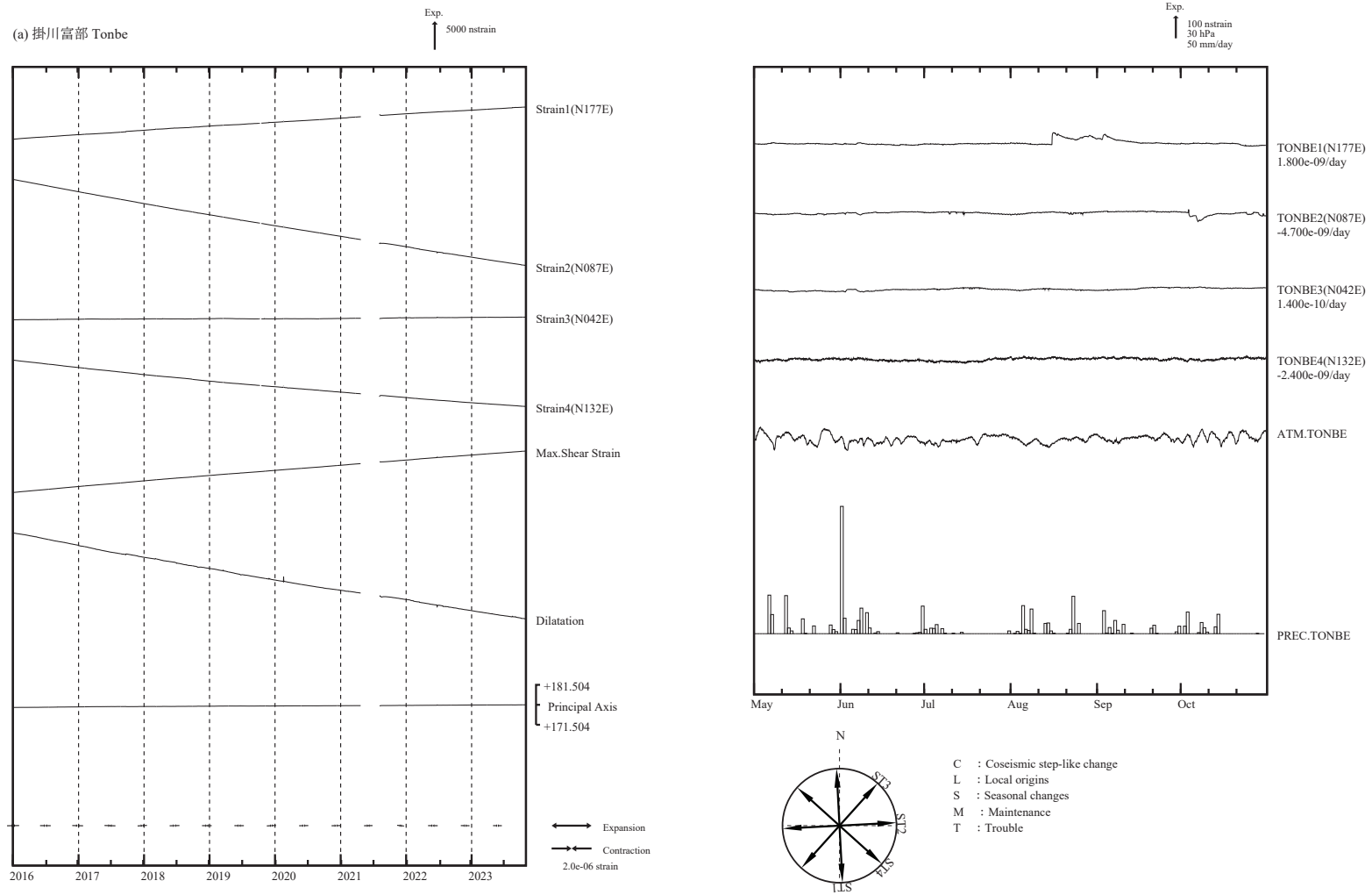
第 4 図 (a) 左：2016 年 1 月以後の多成分ひずみ計変化（日平均値）。主ひずみ・最大せん断ひずみ・面積ひずみは各方向成分から計算されている。 右：2023 年 5 月～10 月の多成分ひずみ計変化（時間値：気圧・潮汐・地磁気・降水補正した値）。各図下部に気圧変化と降水量を示す。
