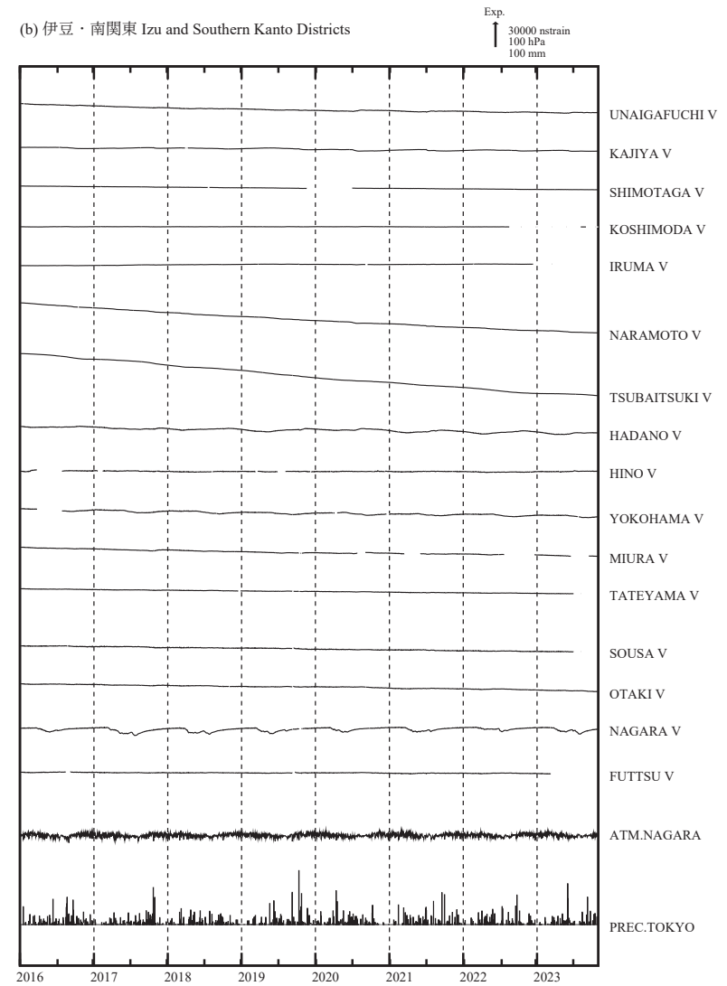
第 2 図 (a), (b) 2016 年 1 月以後の東海・伊豆・南関東地域における区域別体積ひずみ (V) 及び面積ひずみ (S) の変化 (日平均値). 各図下部に区域を代表する気圧変化と降水量を示す.
