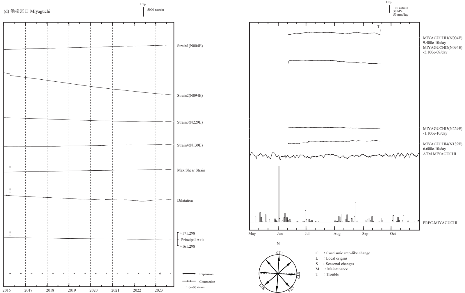
第 4 図 (d) 左 : 2016 年 1 月以後の多成分ひずみ計変化 (日平均値)。主ひずみ・最大せん断ひずみ・面積ひずみは各方向成分から計算されている。 右 : 2023 年 5 月～10 月の多成分ひずみ計変化 (時間値 : 気圧・潮汐・地磁気・降水補正した値)。各図下部に気圧変化と降水量を示す。
