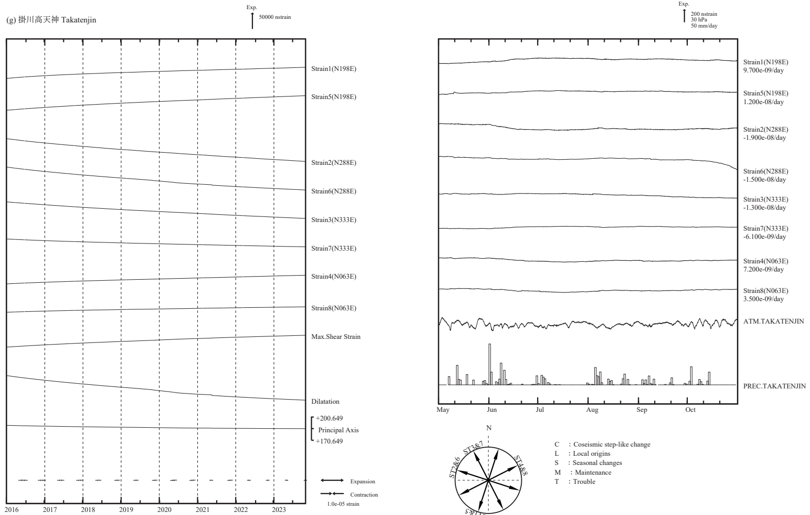
第 4 図 (g) 左：2016 年 1 月以後の多成分ひずみ計変化（日平均値）。主ひずみ・最大せん断ひずみ・面積ひずみは各方向成分から計算されている。 右：2023 年 5 月～10 月の多成分ひずみ計変化（時間値：気圧・潮汐・地磁気・降水補正した値）。各図下部に気圧変化と降水量を示す。
