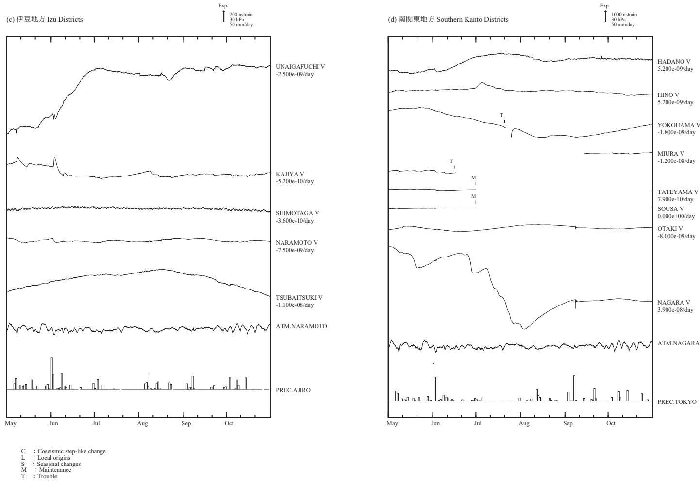
第 3 図 (c), (d) 2023 年 5 月～10 月の東海・伊豆・南関東地域における区域別体積ひずみ (V) 及び面積ひずみ (S) の変化 (時間値: 気圧・潮汐・降水補正した値). 各図下部に区域を代表する気圧変化と降水量を示す. 地点名の下の D strain/day 及び /M はそれぞれ 1 日あたりのトレンド変化量を D として補正していること及び縮尺を 1/M 倍にして表示していることを示している.
