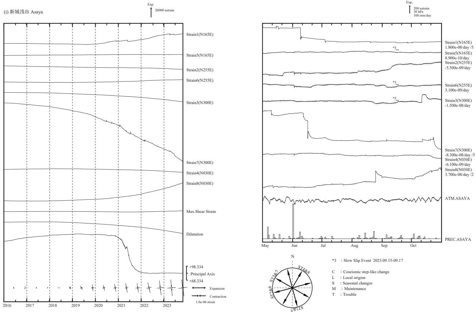
第 4 図 (i) 左 : 2016 年 1 月以後の多成分ひずみ計変化 (日平均値)。主ひずみ・最大せん断ひずみ・面積ひずみは各方向成分から計算されている。 右 : 2023 年 5 月 ~ 10 月の多成分ひずみ計変化 (時間値 : 気圧・潮汐・地磁気・降水補正した値)。各図下部に気圧変化と降水量を示す。
