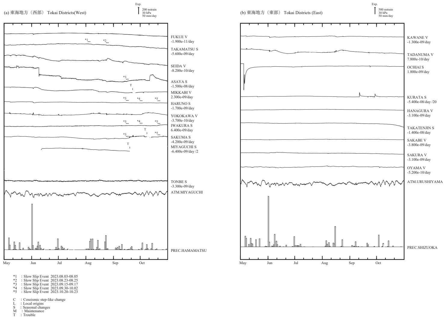
第 3 図 (a), (b) 2023 年 5 月～ 10 月の東海・伊豆・南関東地域における区域別体積ひずみ (V) 及び面積ひずみ (S) の変化 (時間値: 気圧・潮汐・降水補正した値). 各図下部に区域を代表する気圧変化と降水量を示す. 地点名の下に D strain/day 及び /M はそれぞれ 1 日あたりのトレンド変化量を D として補正していること及び縮尺を 1/M 倍にして表示していることを示している.
