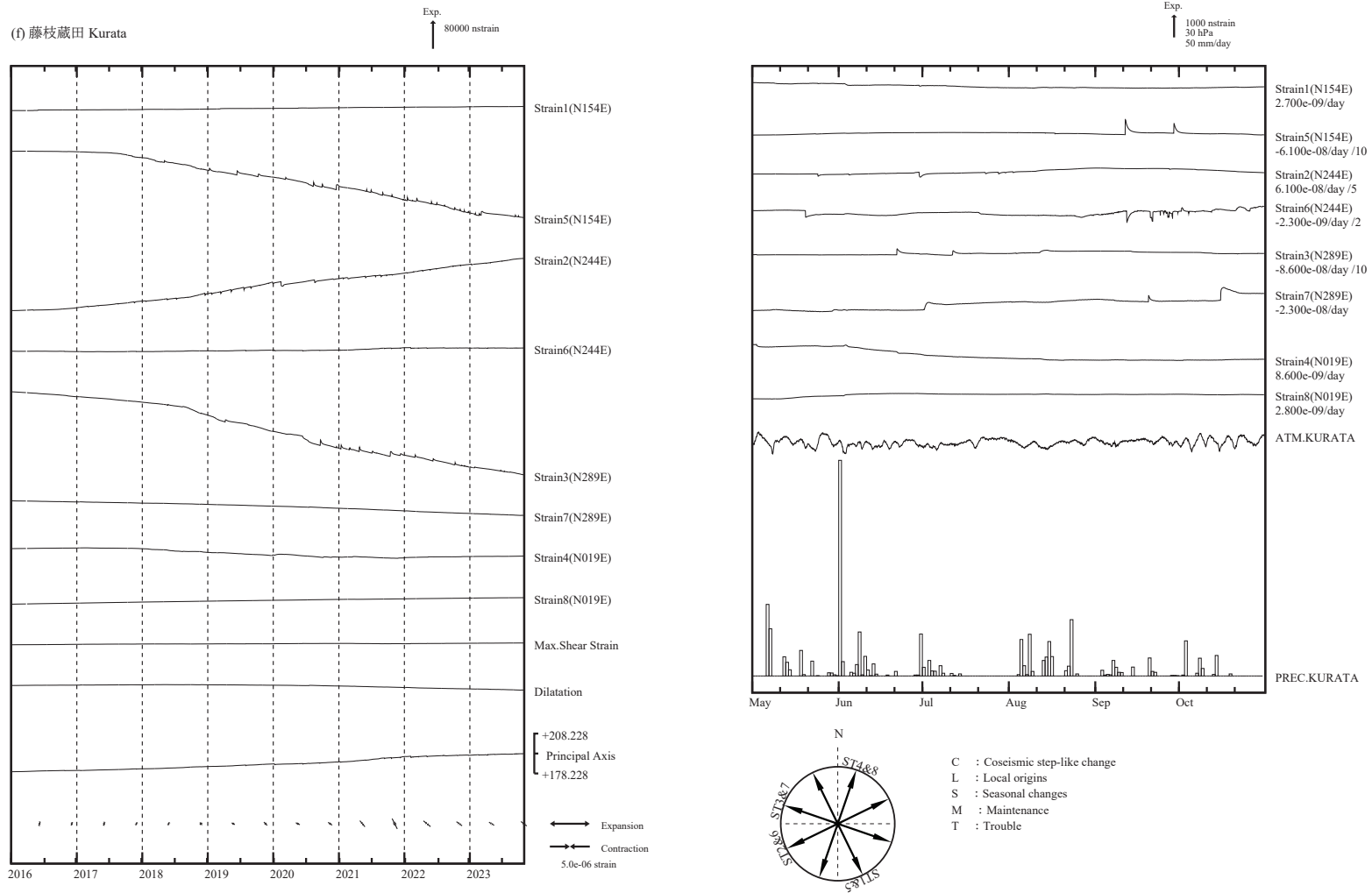
第 4 図 (f) 左 : 2016 年 1 月以後の多成分ひずみ計変化 (日平均値)。主ひずみ・最大せん断ひずみ・面積ひずみは各方向成分から計算されている。 右 : 2023 年 5 月～10 月の多成分ひずみ計変化 (時間値 : 気圧・潮汐・地磁気・降水補正した値)。各図下部に気圧変化と降水量を示す。
