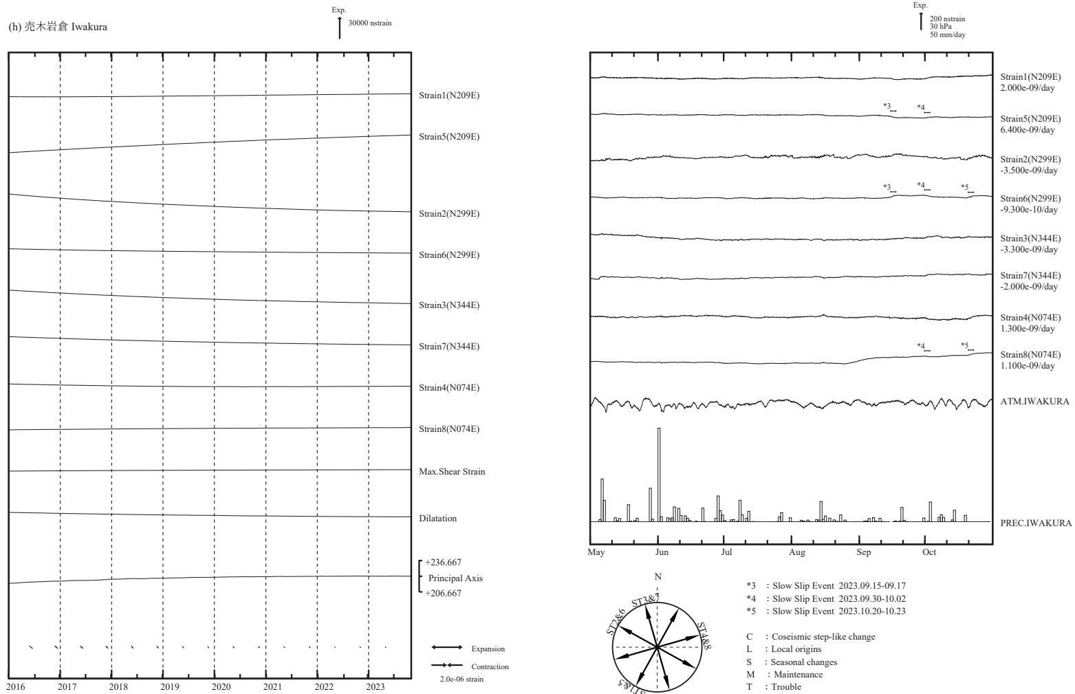
第 4 図 (h) 左：2016 年 1 月以後の多成分ひずみ計変化（日平均値）。主ひずみ・最大せん断ひずみ・面積ひずみは各方向成分から計算されている。 右：2023 年 5 月～10 月の多成分ひずみ計変化（時間値：気圧・潮汐・地磁気・降水補正した値）。各図下部に気圧変化と降水量を示す。
