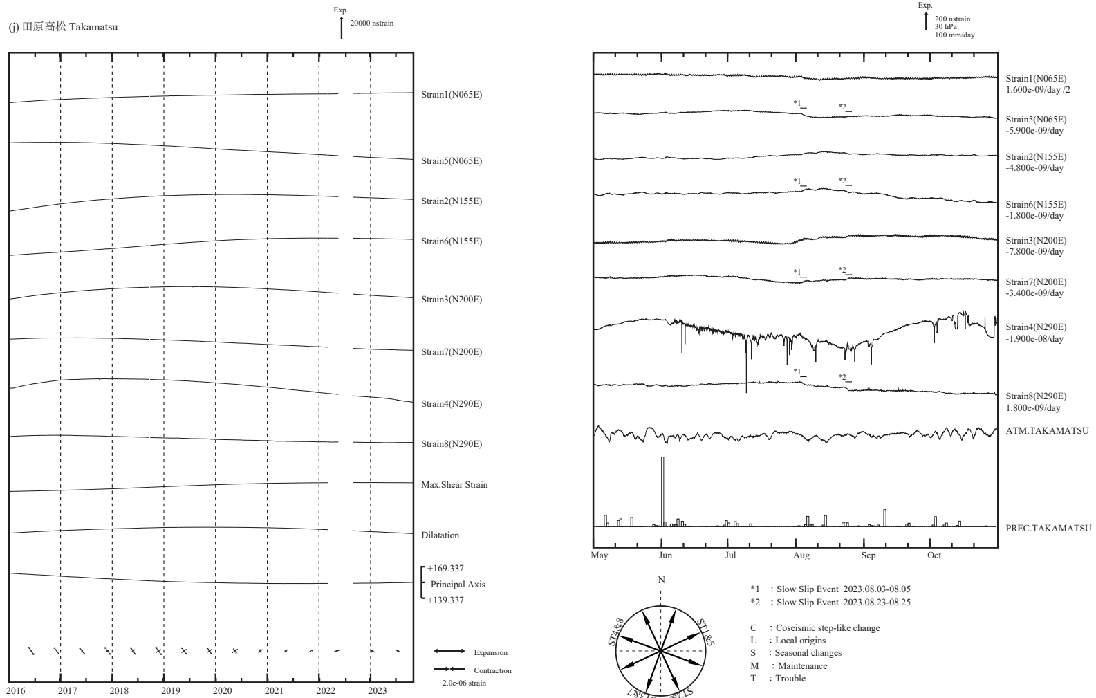
第 4 図 (j) 左 : 2016 年 1 月以後の多成分ひずみ計変化 (日平均値)。主ひずみ・最大せん断ひずみ・面積ひずみは各方向成分から計算されている。 右 : 2023 年 5 月～10 月の多成分ひずみ計変化 (時間値 : 気圧・潮汐・地磁気・降水補正した値)。各図下部に気圧変化と降水量を示す。
