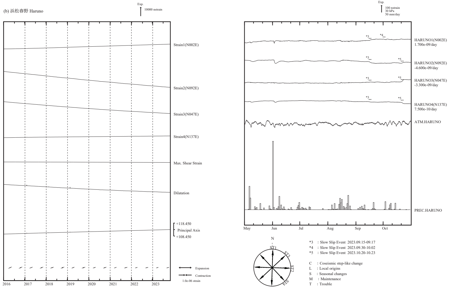
第 4 図 (b) 左：2016 年 1 月以後の多成分ひずみ計変化（日平均値）。主ひずみ・最大せん断ひずみ・面積ひずみは各方向成分から計算されている。 右：2023 年 5 月～10 月の多成分ひずみ計変化（時間値：気圧・潮汐・地磁気・降水補正した値）。各図下部に気圧変化と降水量を示す。
