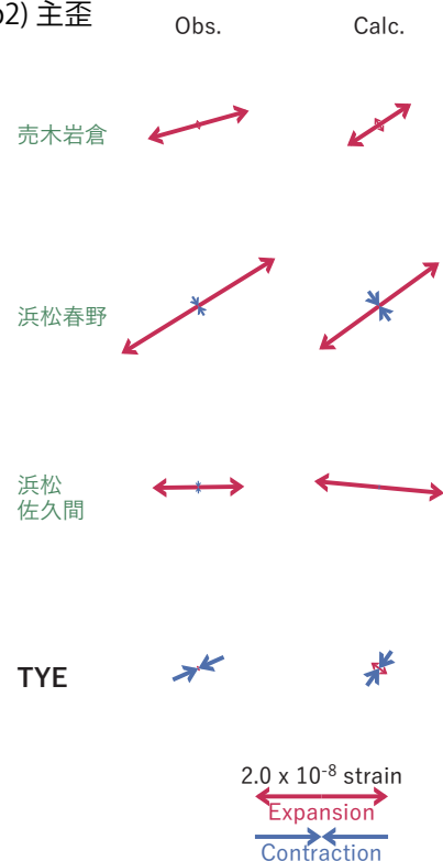
(b2) 主歪
