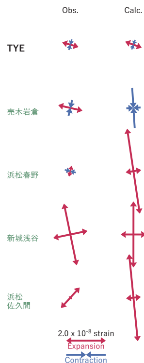
(b2) 主歪
