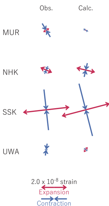
(b2) 主歪
