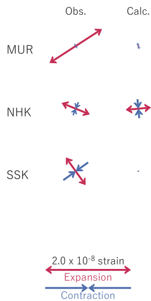
(b2) 主歪
