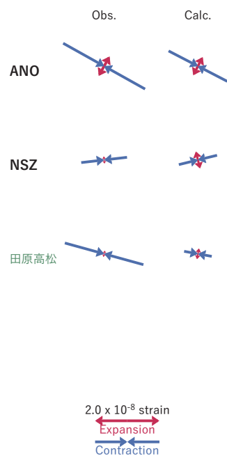
(b2) 主歪
