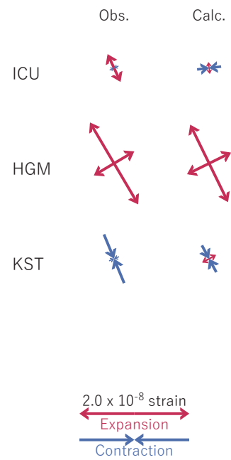
(b2) 主歪
