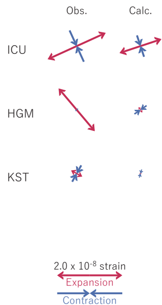
(b2) 主歪
