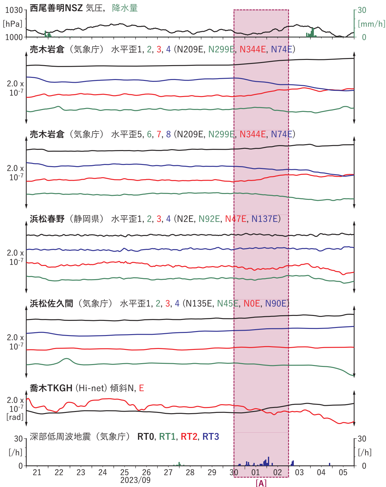
第 45 図 東海地方における歪・傾斜の観測結果と低周波地震の検出数 (2023/09/21 ~ 2023/10/05).
