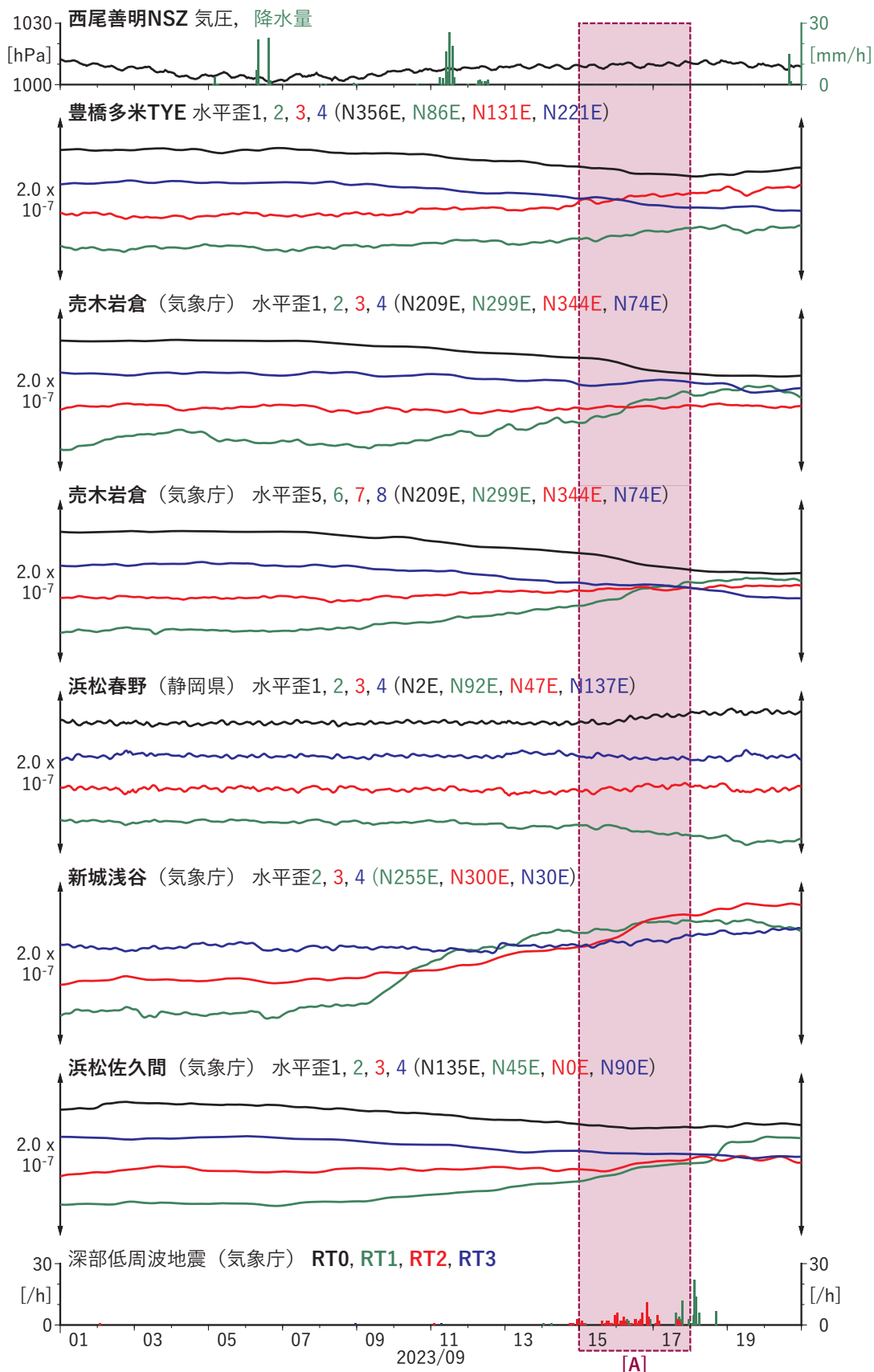
第 42 図 東海地方における歪・傾斜の観測結果と低周波地震の検出数 (2023/09/01 ~ 2023/09/20)。
