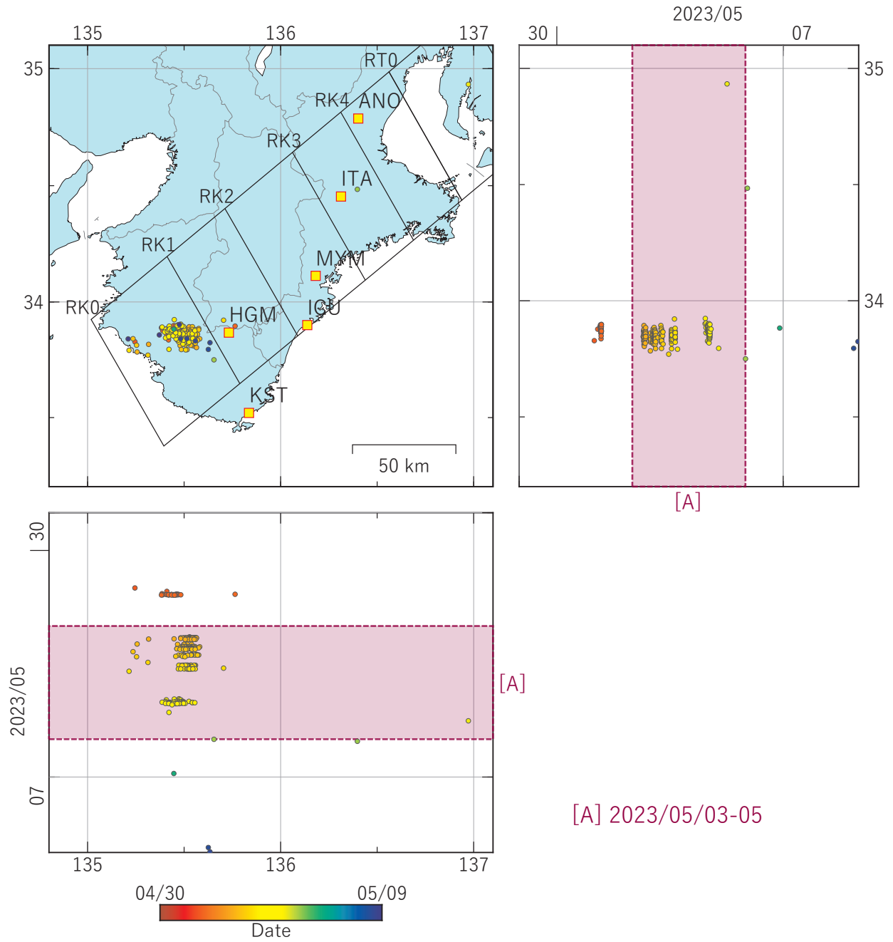
第 1 図 紀伊半島における低周波地震（気象庁一元化カタログによる）の時空間分布（2023/04/30 ～ 2023/05/08）. Fig. 1 Space-time distribution of low-frequency earthquakes by JMA unified hypocenter catalog in the Kii Peninsula from April 30 to May 8, 2023.
