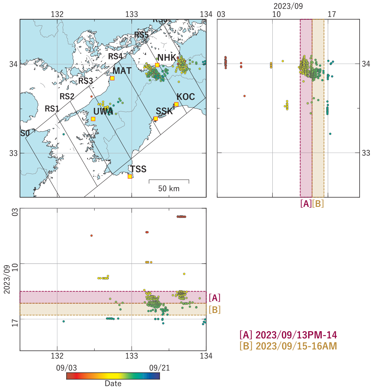
第 37 図 四国地方における低周波地震（気象庁一元化カタログによる）の時空間分布（2023/09/03 ～ 2023/09/20）. Fig. 37 Space-time distribution of low-frequency earthquakes by JMA unified hypocenter catalog in the Shikoku region from September 3 to 20, 2023.
