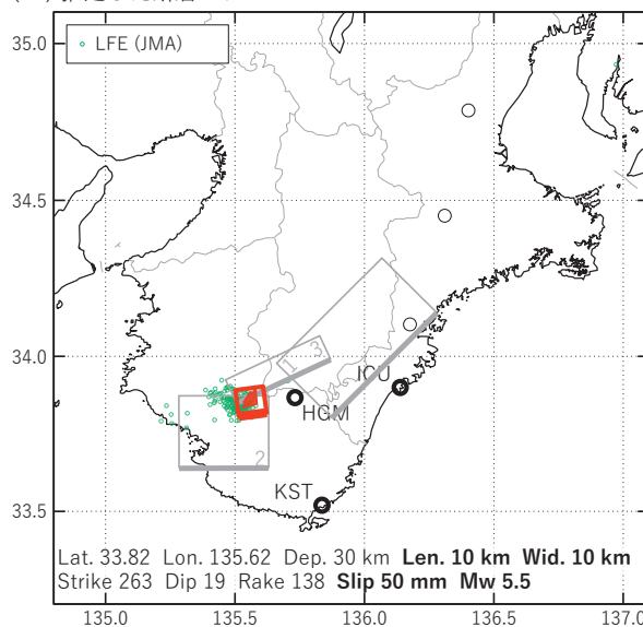
第 3 図 第 2 図 [A] を説明する断層モデル。以下の凡例の説明は以降の同様の図に共通。(図によっては気象庁・静岡県の観測点や (b3) 体積歪の結果はない場合がある。) 黒・緑・青の丸印はそれぞれ産総研・気象庁および静岡県・防災科研 Hi-net の観測点、緑の小さな丸印は気象庁の推定した低周波地震。(a) 1 段階目の結果。灰色の濃淡は残差の総和で、赤色矩形が残差の総和が最小となる断層面の位置 (大きさは 20x20 km で固定)。(b1) 2 段階目の結果。赤色矩形が残差の総和が最小となる断層面。矢印は傾斜の観測値と計算値の比較。灰色矩形は最近周辺で発生した短期的 SSE の推定断層面 (番号との対応は本文参照)。(b2) 主歪の観測値と (b1) に示した断層モデルから求めた計算値との比較。(b3) 体積歪の観測値と (b1) に示した断層モデルから求めた計算値との比較。
