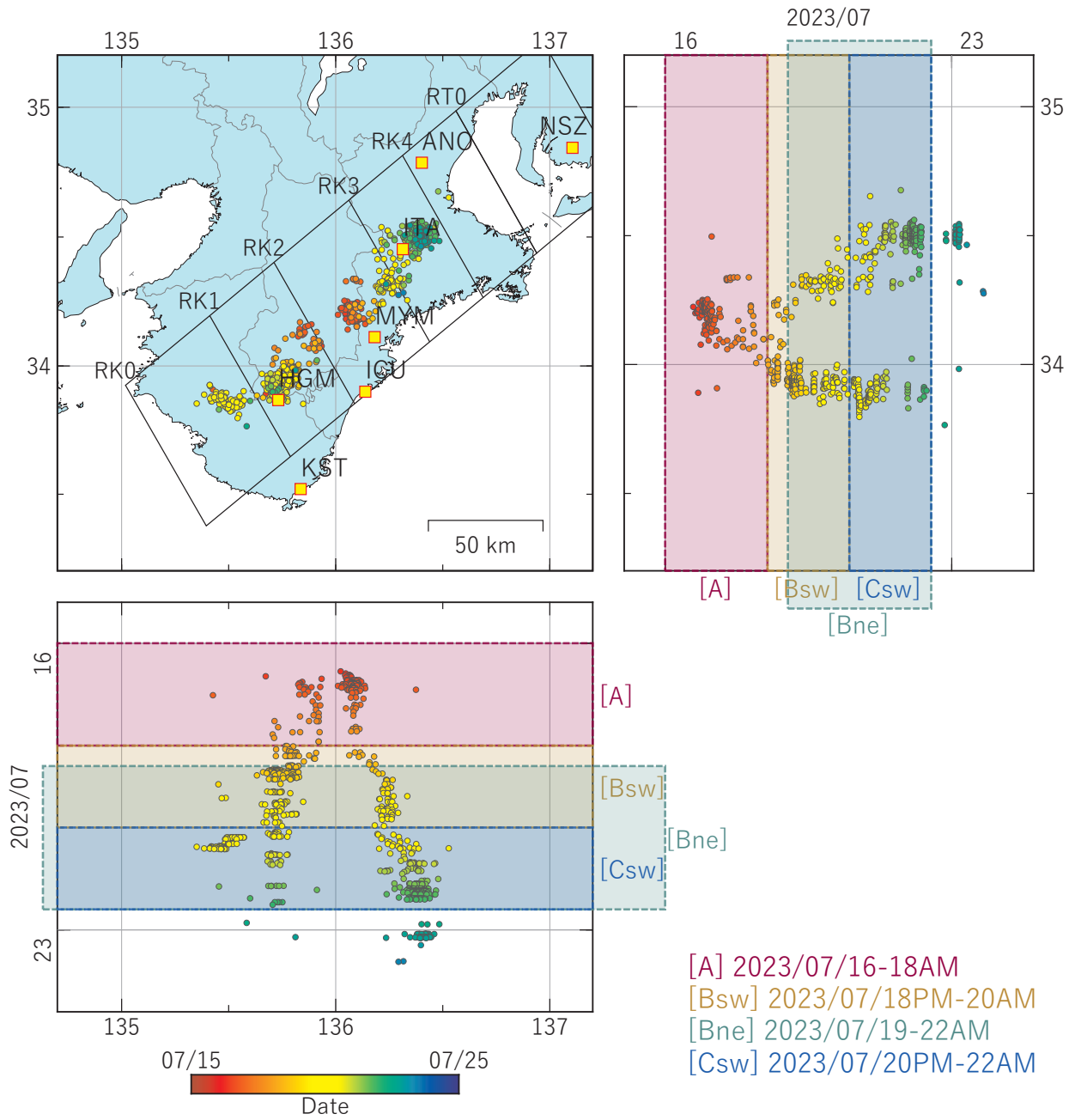
第 20 図 紀伊半島における低周波地震（気象庁一元化カタログによる）の時空間分布（2023/07/15～2023/07/24）. Fig. 20 Space-time distribution of low-frequency earthquakes by JMA unified hypocenter catalog in the Kii Peninsula from July 15 to 24, 2023.
