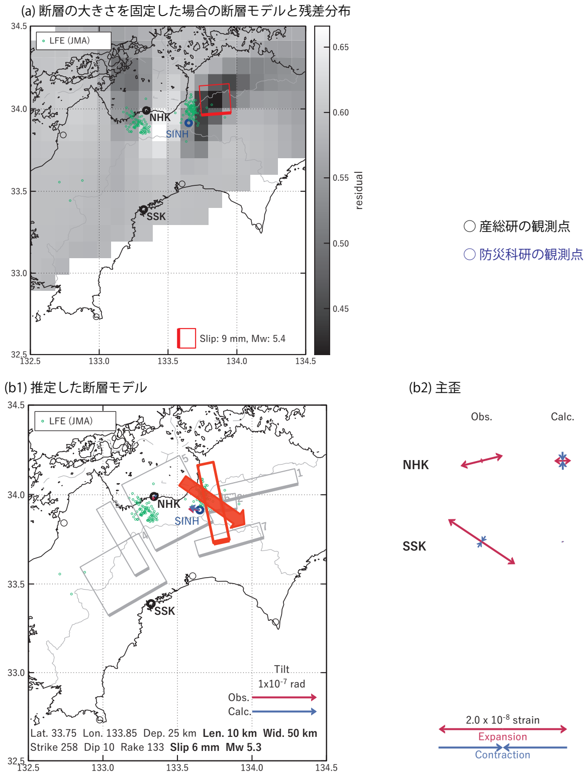
第 39 図 第 38 図 [A] を説明する断層モデル. 各図の説明は第 3 図を参照. Fig. 39 Inferred fault models for Fig. 38[A]. See also the caption of Fig. 3.
