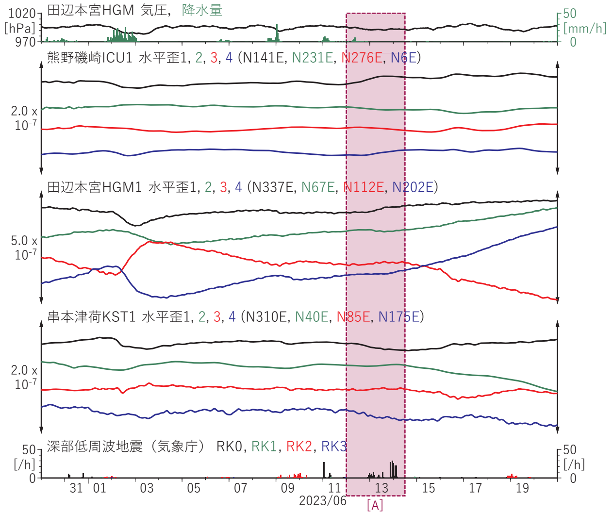
第 9 図 紀伊半島における歪の観測結果と低周波地震の検出数 (2023/05/30 ~ 2023/06/21)。
