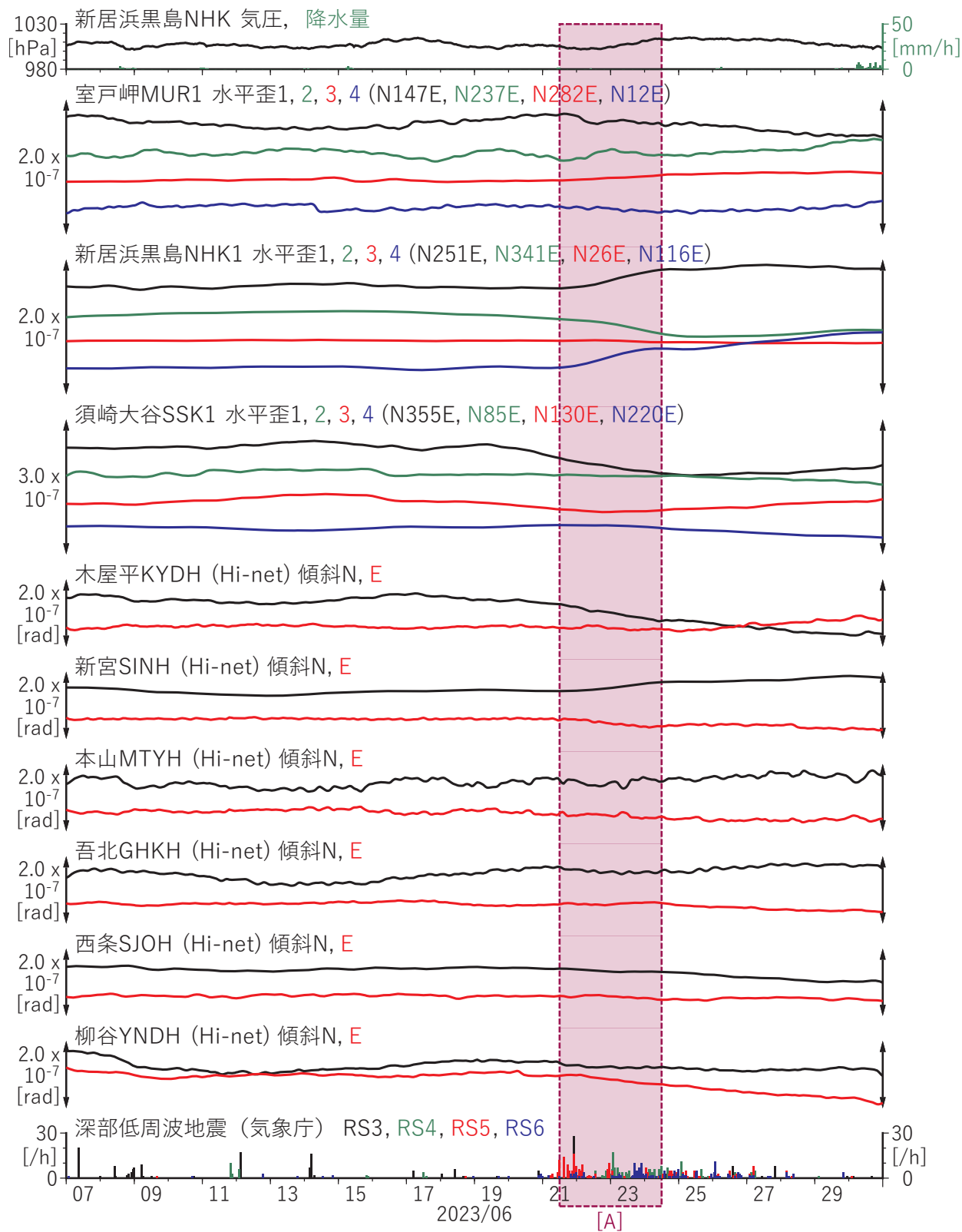
第 12 図 四国地方における歪・傾斜の観測結果と低周波地震の検出数 (2023/06/07 ~ 2023/06/30).
