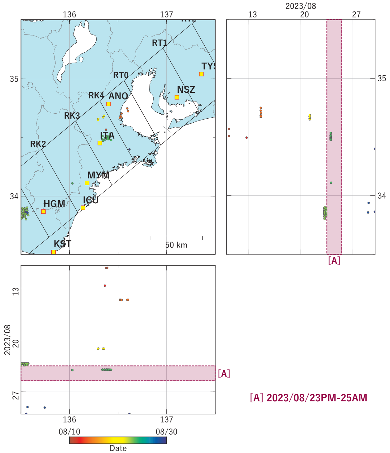
第 33 図 紀伊半島から東海地方における低周波地震（気象庁一元化カタログによる）の時空間分布（2023/08/10 ～ 2023/08/29）。
