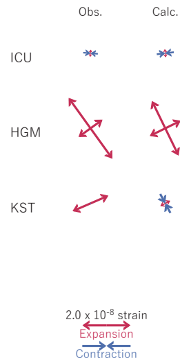
第 3 図 第 2 図 [A] を説明する断層モデル。以下の凡例の説明は以降の同様の図に共通。(図によっては気象庁・静岡県の観測点や (b3) 体積歪の結果はない場合がある。) 黒・緑・青の丸印はそれぞれ産総研・気象庁および静岡県・防災科研 Hi-net の観測点、緑の小さな丸印は気象庁の推定した低周波地震。(a) 1 段階目の結果。灰色の濃淡は残差の総和で、赤色矩形が残差の総和が最小となる断層面の位置 (大きさは 20x20 km で固定)。(b1) 2 段階目の結果。赤色矩形が残差の総和が最小となる断層面。矢印は傾斜の観測値と計算値の比較。灰色矩形は最近周辺で発生した短期的 SSE の推定断層面 (番号との対応は本文参照)。(b2) 主歪の観測値と (b1) に示した断層モデルから求めた計算値との比較。(b3) 体積歪の観測値と (b1) に示した断層モデルから求めた計算値との比較。
