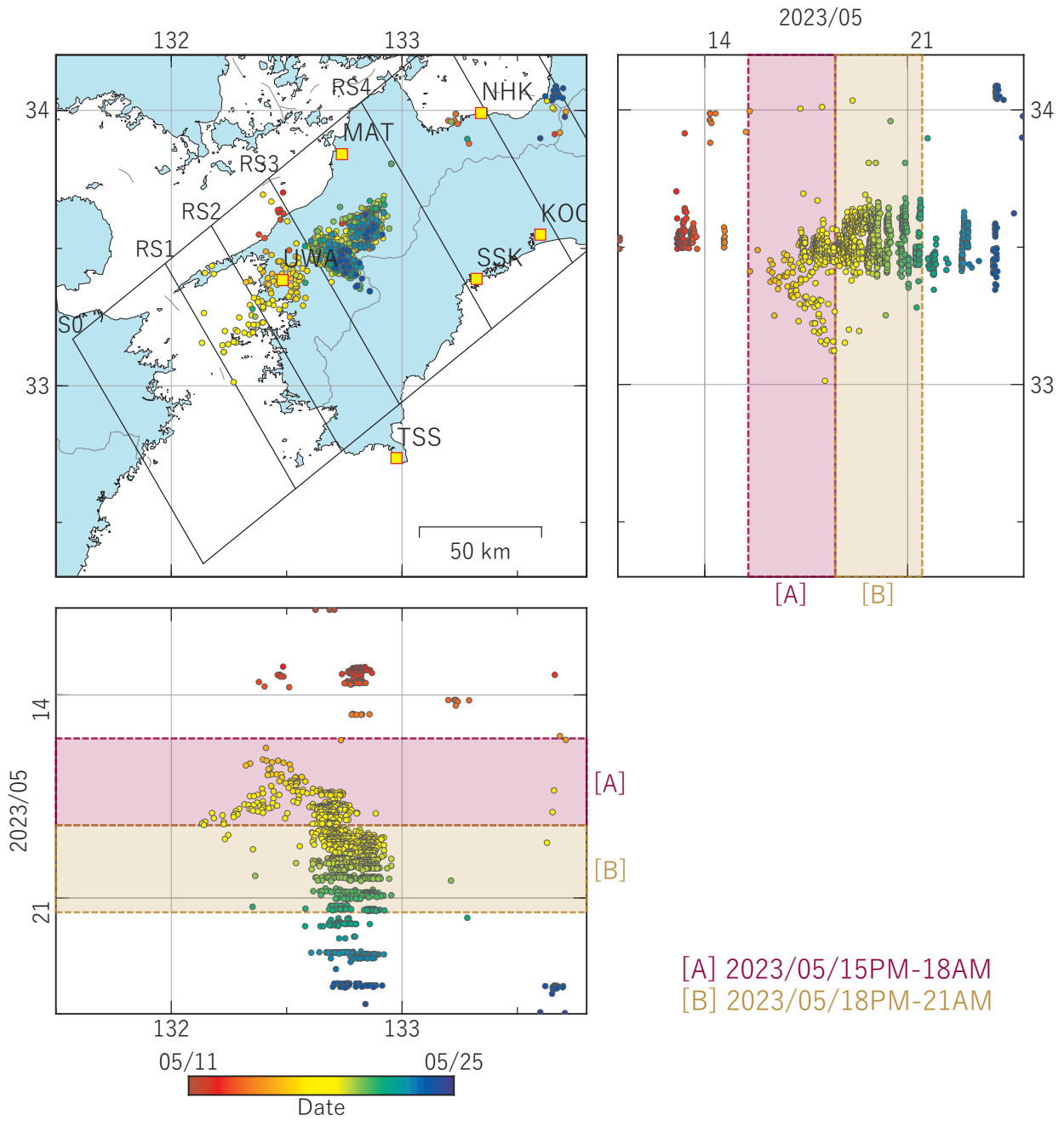
第 4 図 四国地方における低周波地震（気象庁一元化カタログによる）の時空間分布（2023/05/11 ～ 2023/05/24）.
