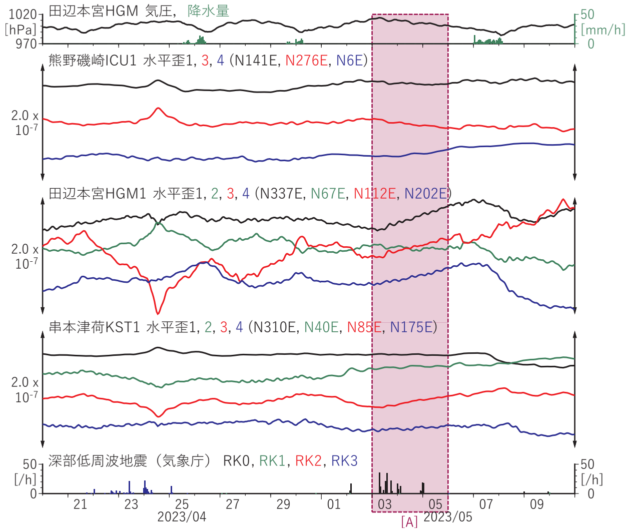
第 2 図 紀伊半島における歪の観測結果と低周波地震の検出数 (2023/04/20 ~ 2023/05/11).
