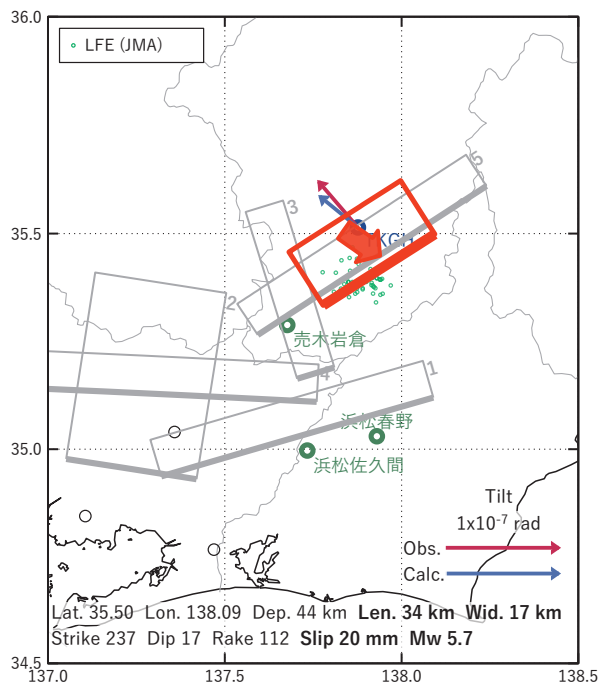
第 46 図 第 45 図 [A] を説明する断層モデル. 各図の説明は第 3 図を参照. Fig. 46 Inferred fault models for Fig. 45[A]. See also the caption of Fig. 3.
