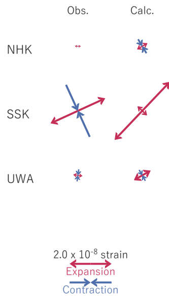
(b2) 主歪
