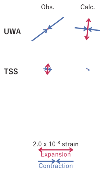
(b2) 主歪
