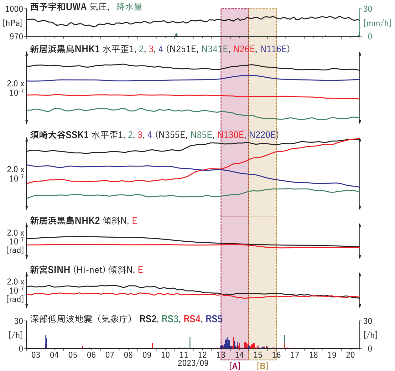
第 38 図 四国地方における歪・傾斜の観測結果と低周波地震の検出数 (2023/09/03 ~ 2023/09/20).
