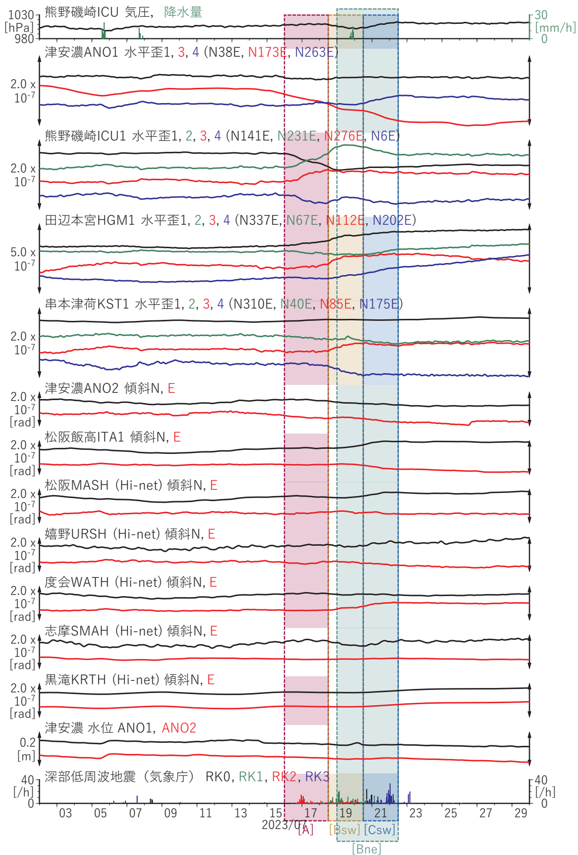
第 21 図 紀伊半島における歪・傾斜・地下水の観測結果と低周波地震の検出数 (2023/07/02 ~ 2023/07/29).
