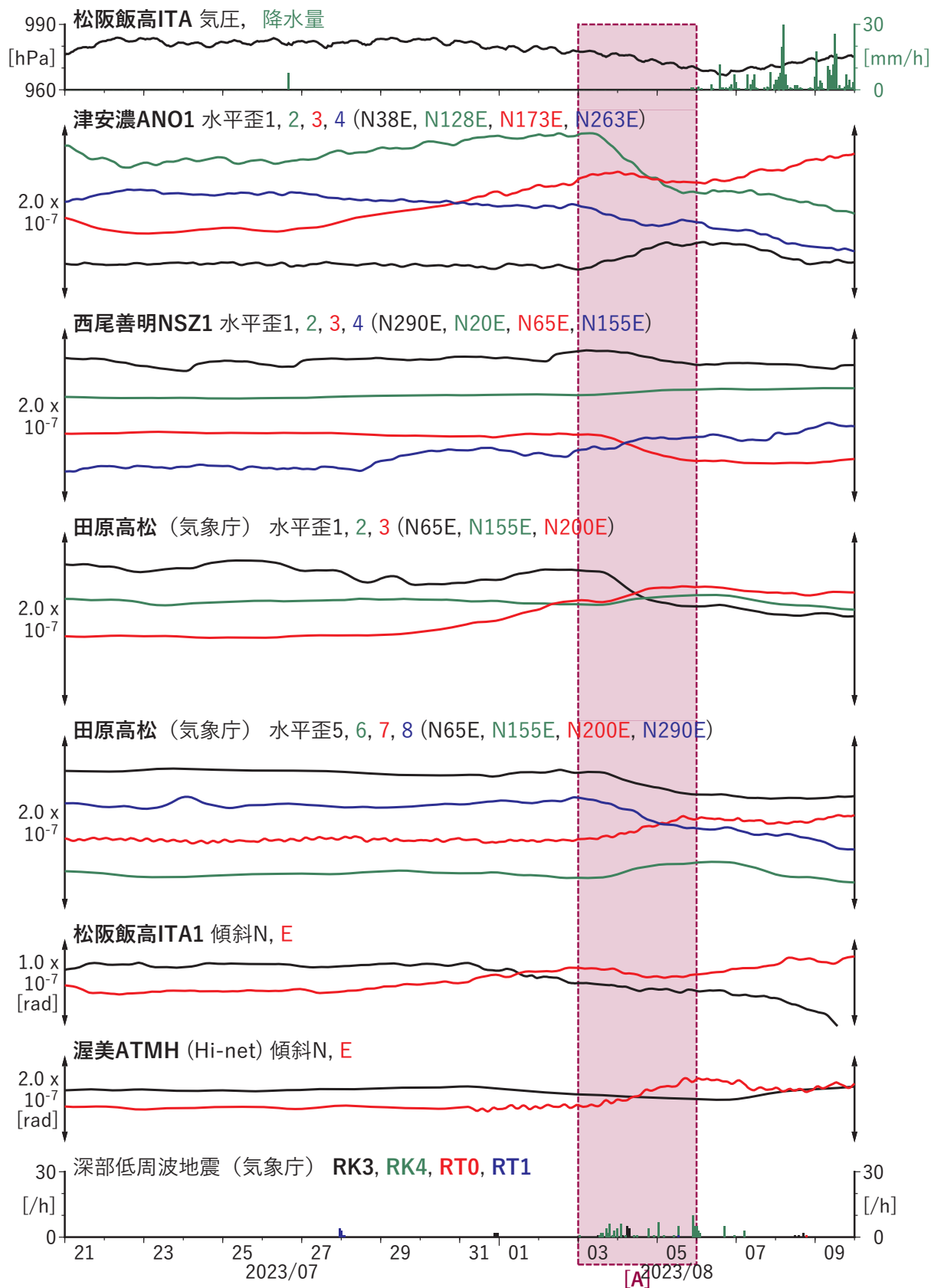
第 27 図 紀伊半島から東海地方における歪・傾斜の観測結果と低周波地震の検出数 (2023/07/21 ~ 2023/08/09)。
