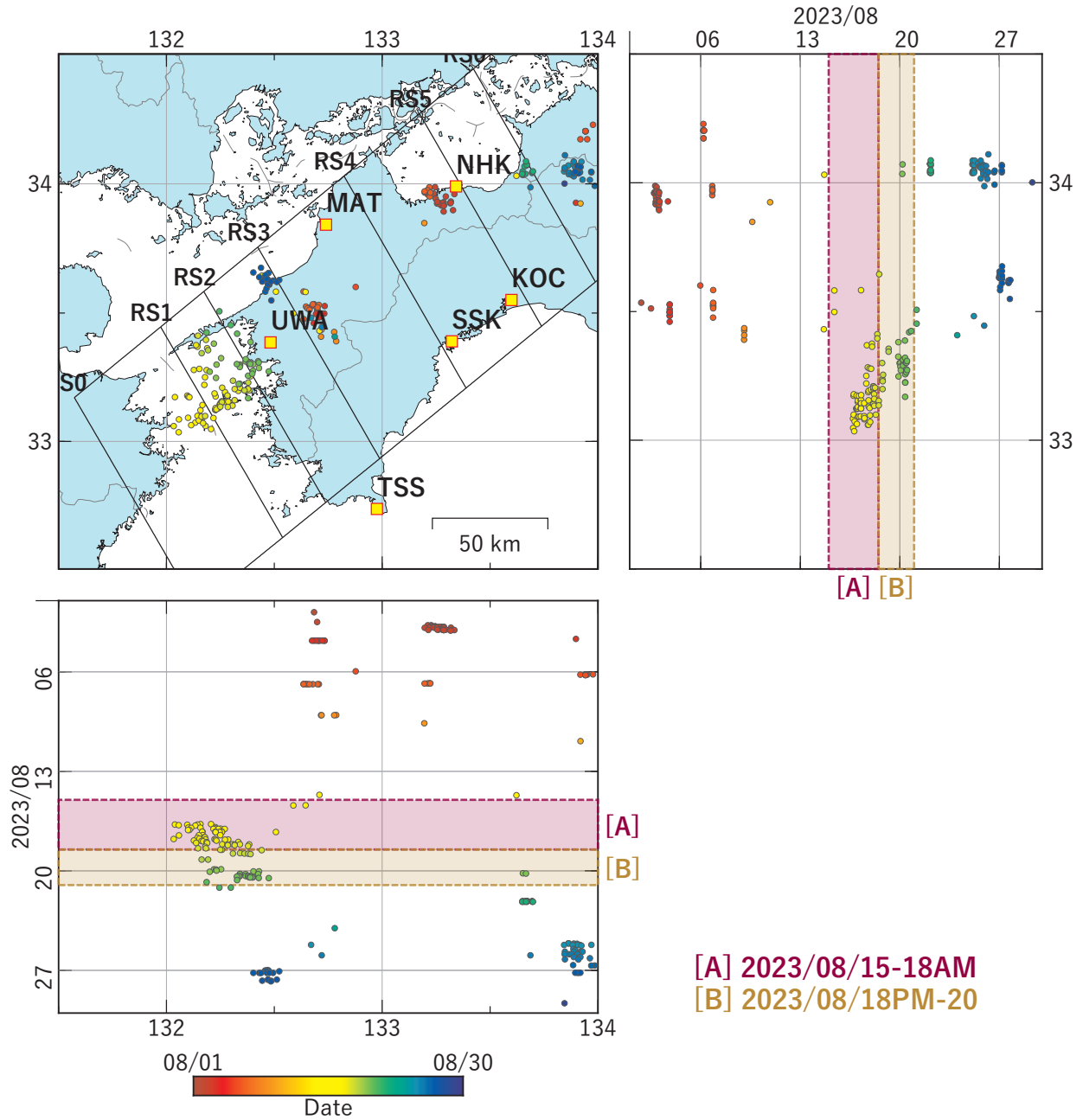
第 29 図 四国地域における低周波地震（気象庁一元化カタログによる）の時空間分布（2023/08/01 ～ 2023/08/29）. Fig. 29 Space-time distribution of low-frequency earthquakes by JMA unified hypocenter catalog in the Shikoku region from August 01 to 29, 2023.
