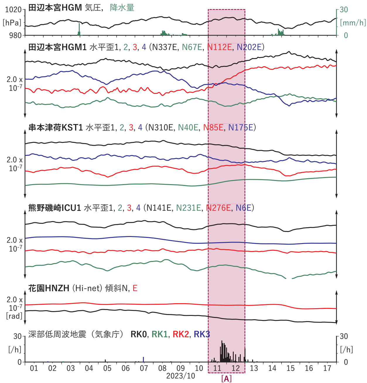
第 48 図 紀伊半島における歪・傾斜の観測結果と低周波地震の検出数 (2023/10/01 ~ 2023/10/17).
