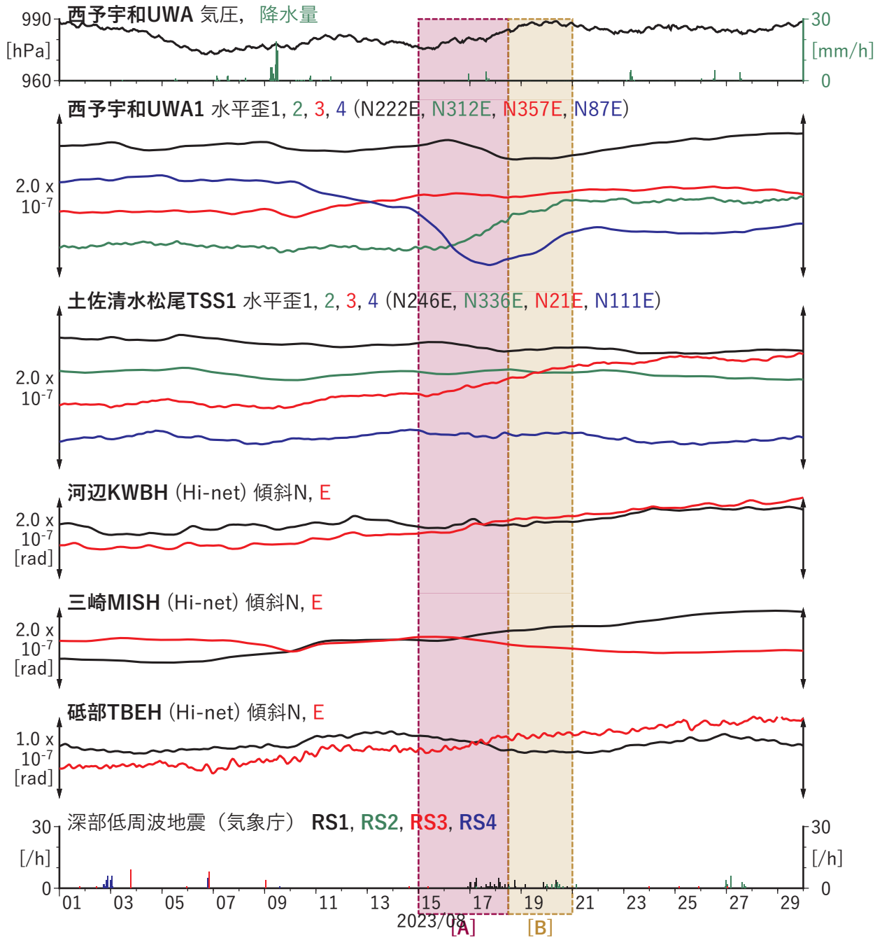
第 30 図 四国地方における歪・傾斜の観測結果と低周波地震の検出数 (2023/08/01 ~ 2023/08/29).
