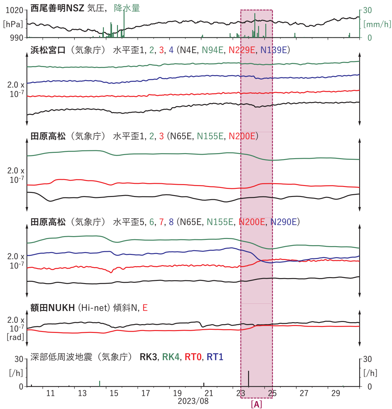
第 35 図 紀伊半島から東海地方における歪・傾斜の観測結果と低周波地震の検出数 (2) (2023/08/10 ~ 2023/08/30).
