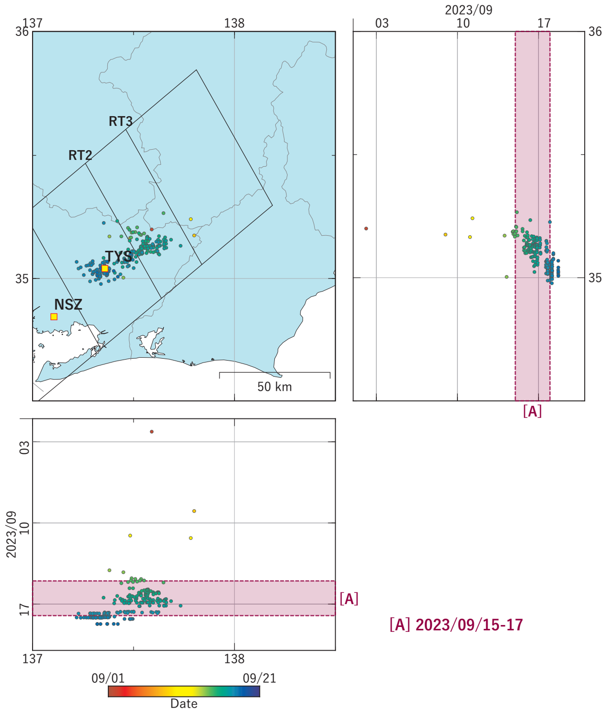
第 41 図 東海地方における低周波地震（気象庁一元化カタログによる）の時空間分布（2023/09/01 ～ 2023/09/20）. Fig. 41 Space-time distribution of low-frequency earthquakes by JMA unified hypocenter catalog in the Tokai region from September 1 to 20, 2023.
