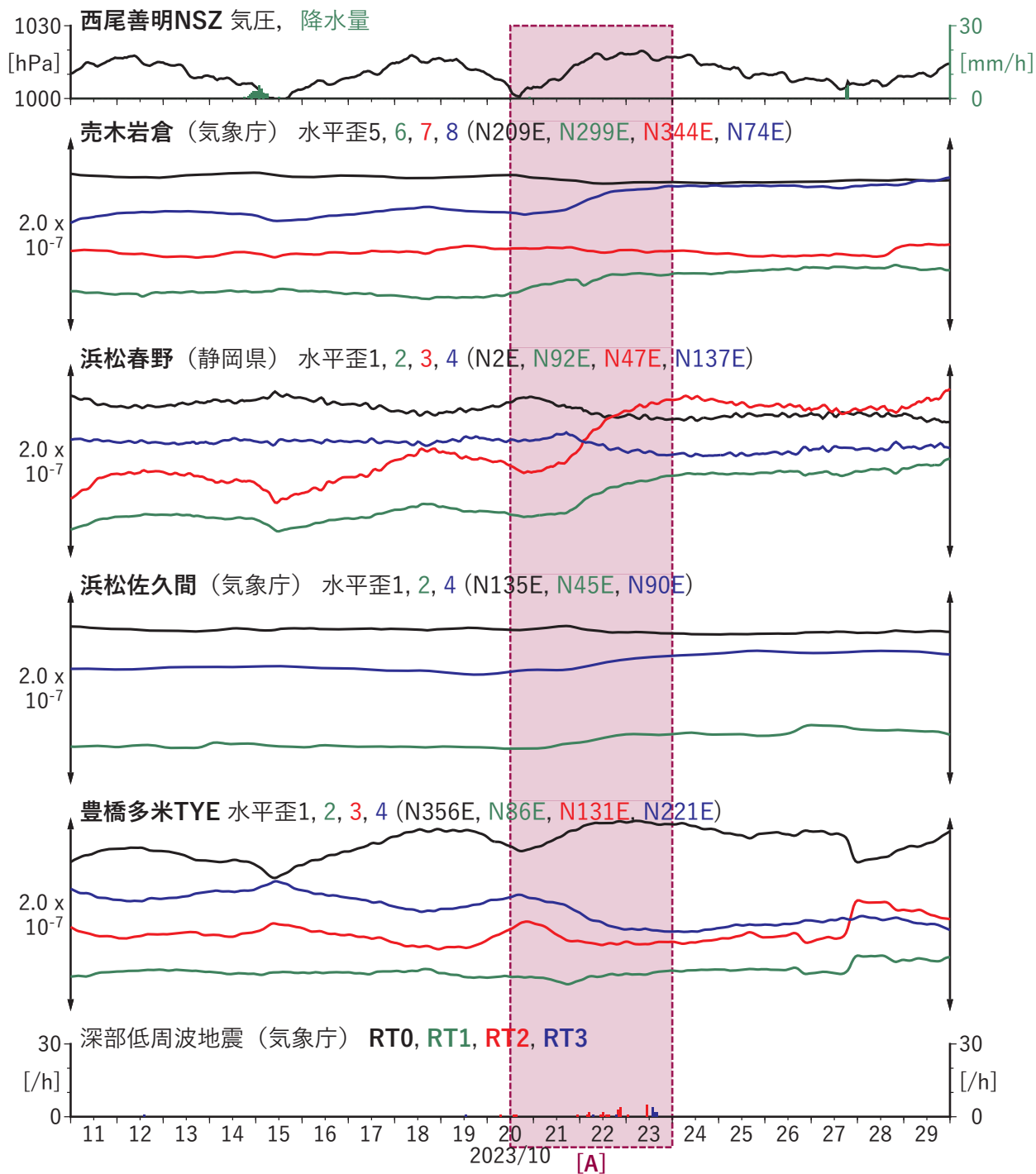
第 51 図 東海地方における歪の観測結果と低周波地震の検出数 (2023/10/11 ~ 2023/10/29).
