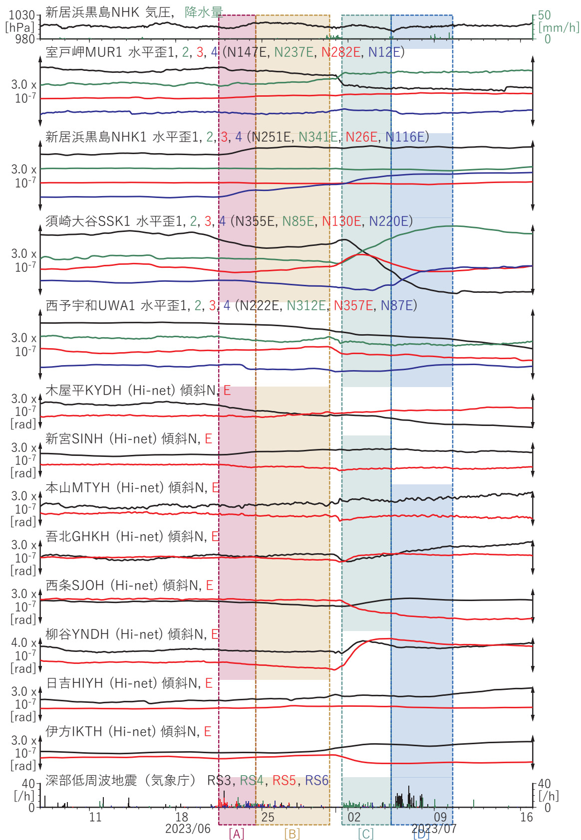
第 15 図 四国地域における歪・傾斜の観測結果と低周波地震の検出数 (2023/06/07 ~ 2023/07/16)。
