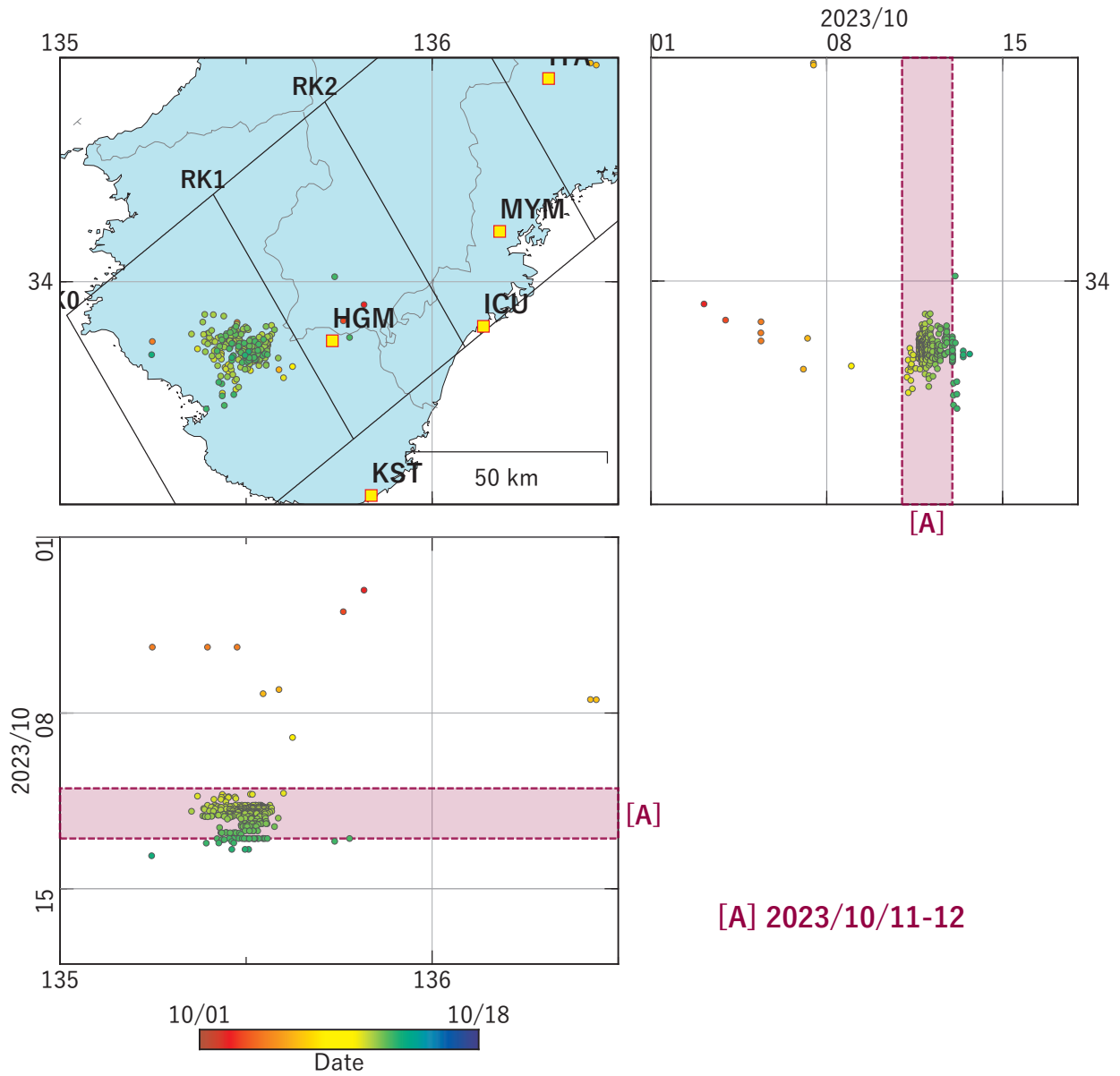
第 47 図 紀伊半島における低周波地震（気象庁一元化カタログによる）の時空間分布（2023/10/01 ～ 2023/10/17）. Fig. 47 Space-time distribution of low-frequency earthquakes by JMA unified hypocenter catalog in the Kii Peninsula from October 1 to 17, 2023.
