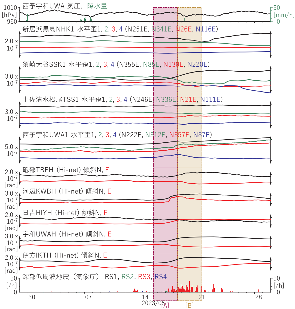
第 5 図 四国地方における歪・傾斜の観測結果と低周波地震の検出数 (2023/04/29 ~ 2023/05/29).
