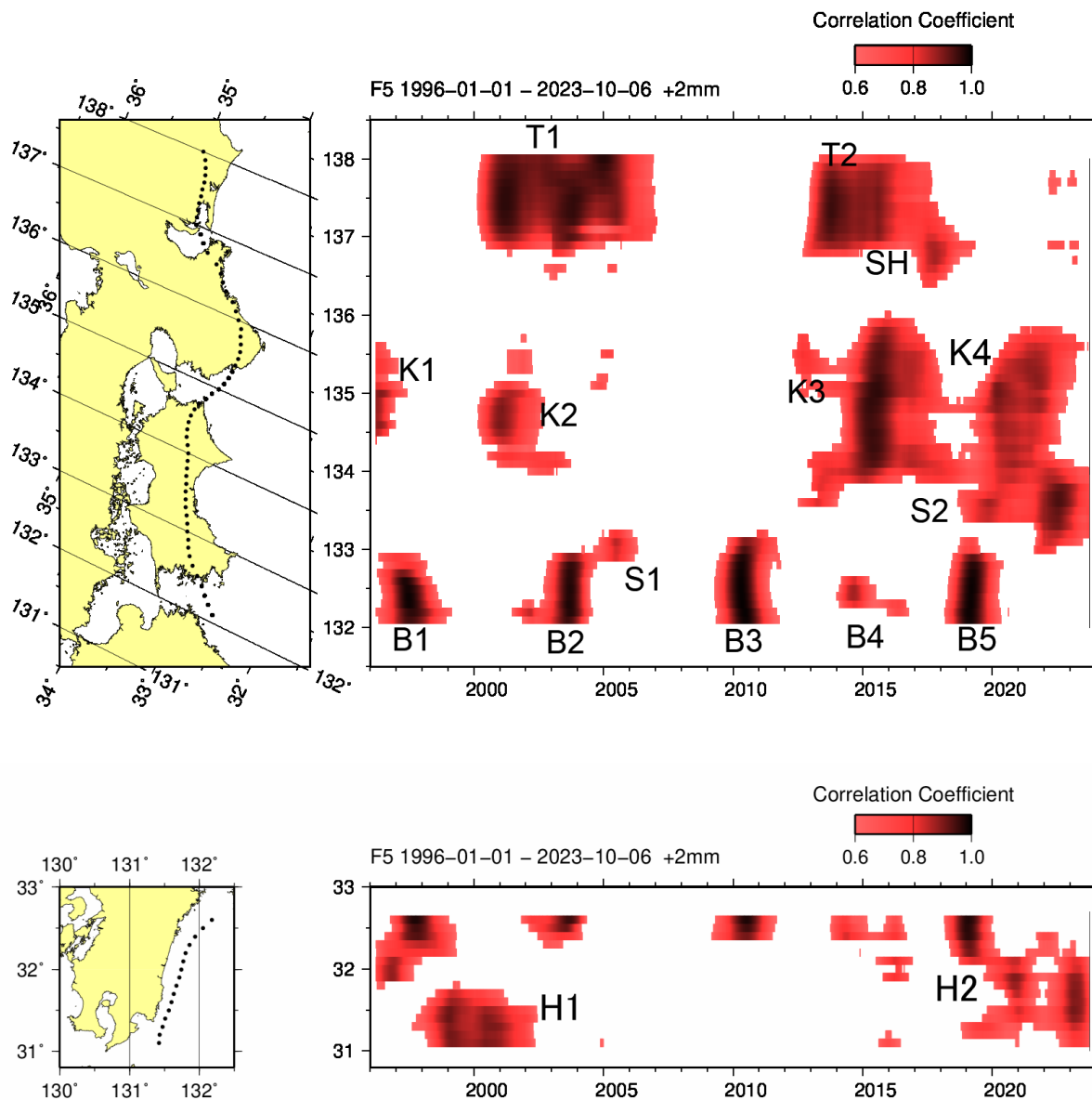
第 1 図 長期的スロースリップ客観検知図（1996 年から 2023 年 10 月）
