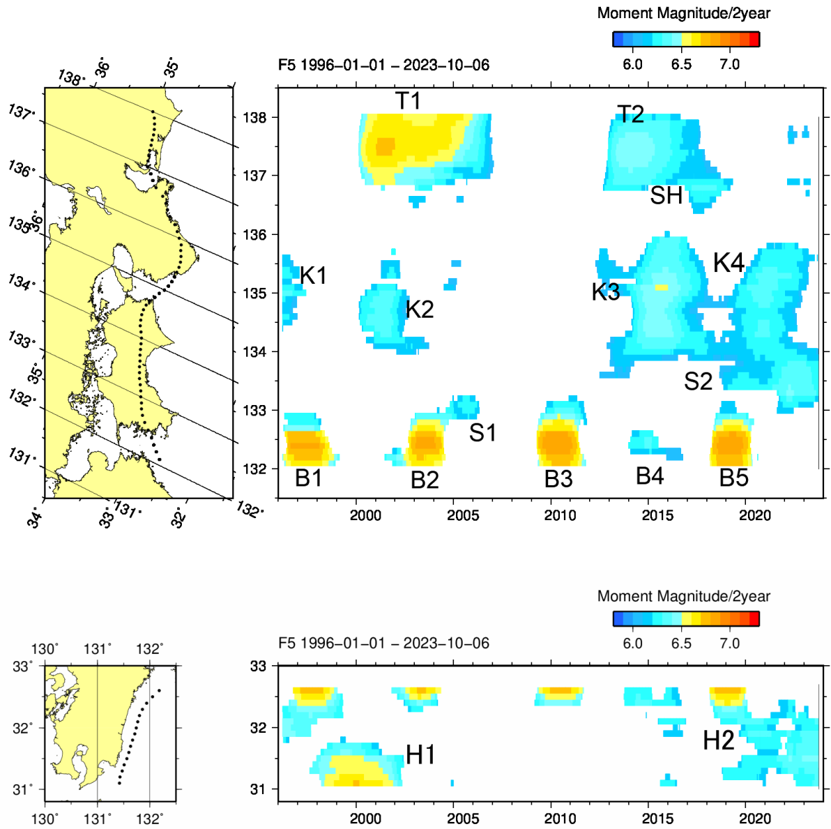
第 2 図 長期的スロースリップの規模分布（1996 年から 2023 年 10 月） 2 年間あたりの変化量から推定したモーメントマグニチュード。イベントの略号は第 1 図と同じ。 Fig. 2 Moment magnitude distribution of long-term slow slip events. The event abbreviations are the same as in Fig. 1.
