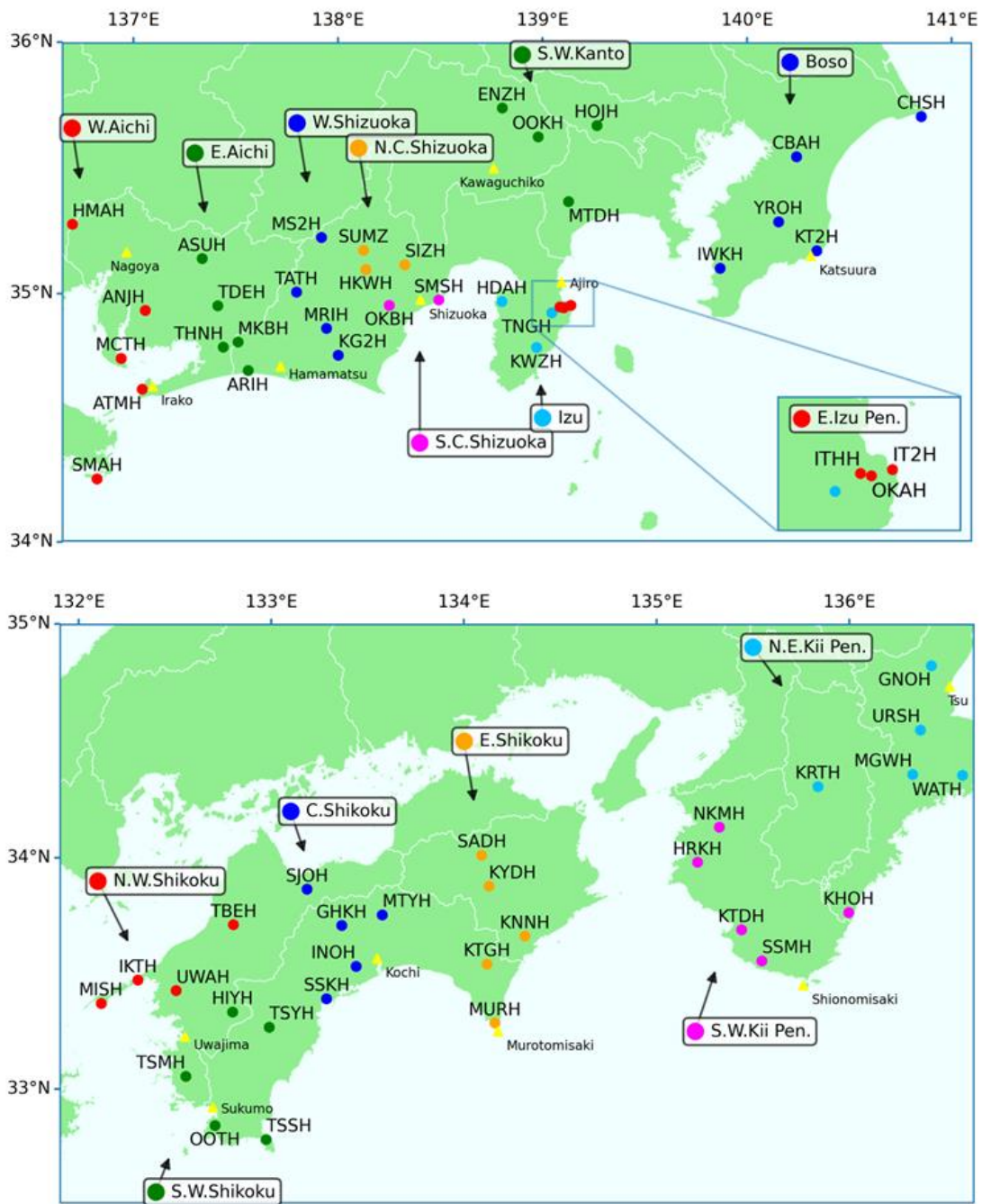
第 1 図 傾斜観測点 (丸印) の配置. シンボルの色で分けた観測点グループ毎に図 2 で傾斜記録を表示している. 使用した気象庁気象観測点を三角形 (黄色) であわせて示す. Fig. 1 Tilt observation stations (colored solid circles). Tilt data of stations grouped by the symbol color are depicted in Fig 2 (a) - (o). Meteorological stations operated by the Japan Meteorological Agency are also shown by yellow triangles.
