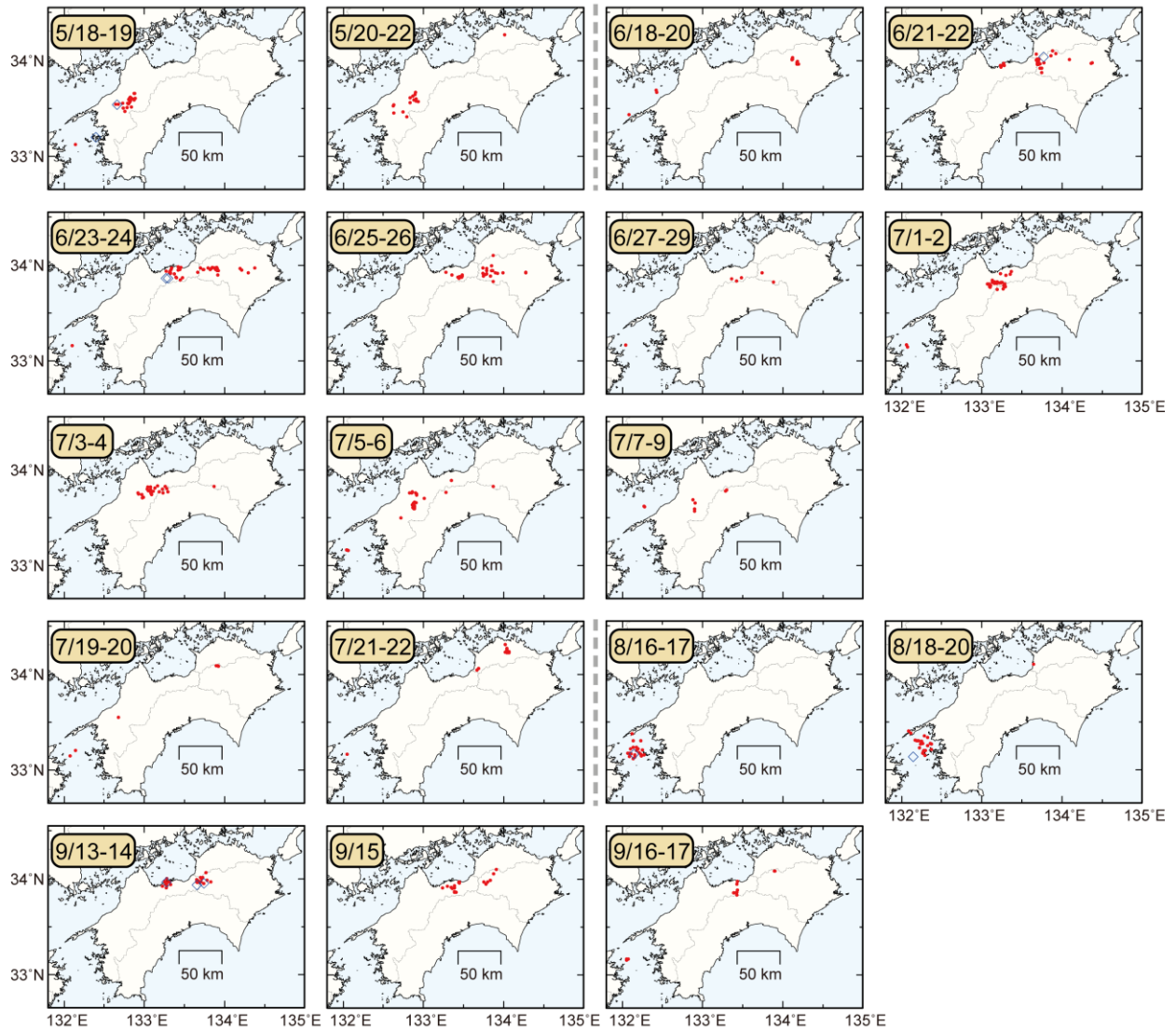
第 5 図 2023 年 5 月から 2023 年 10 月までの期間に四国地域で発生した、主な深部低周波微動及び超低周波地震の活動における震央分布スナップショット。赤丸が当該期間の微動、青菱形が超低周波地震を表す。
