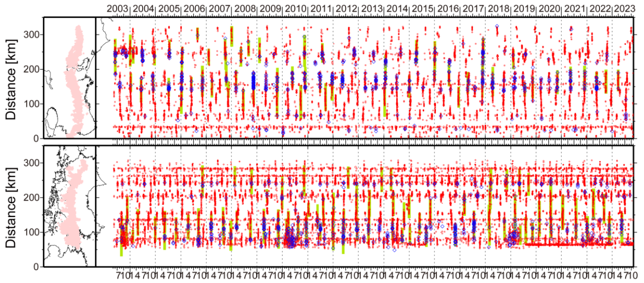
第 3 図 西南日本で発生した深部低周波微動（赤丸）及び深部超低周波地震（青菱形）の 2003 年 5 月から約 20 年間の時空間分布。黄緑色太線は、傾斜変動から検出された短期的スロースリップイベントを示す。
