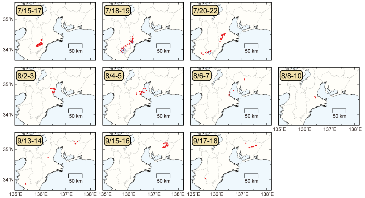
第 4 図 2023 年 5 月から 2023 年 10 月までの期間に東海・紀伊半島地域で発生した、主な深部低周波微動及び深部超低周波地震の活動における震央分布スナップショット。赤丸が当該期間の微動、青菱形が超低周波地震を表す。
