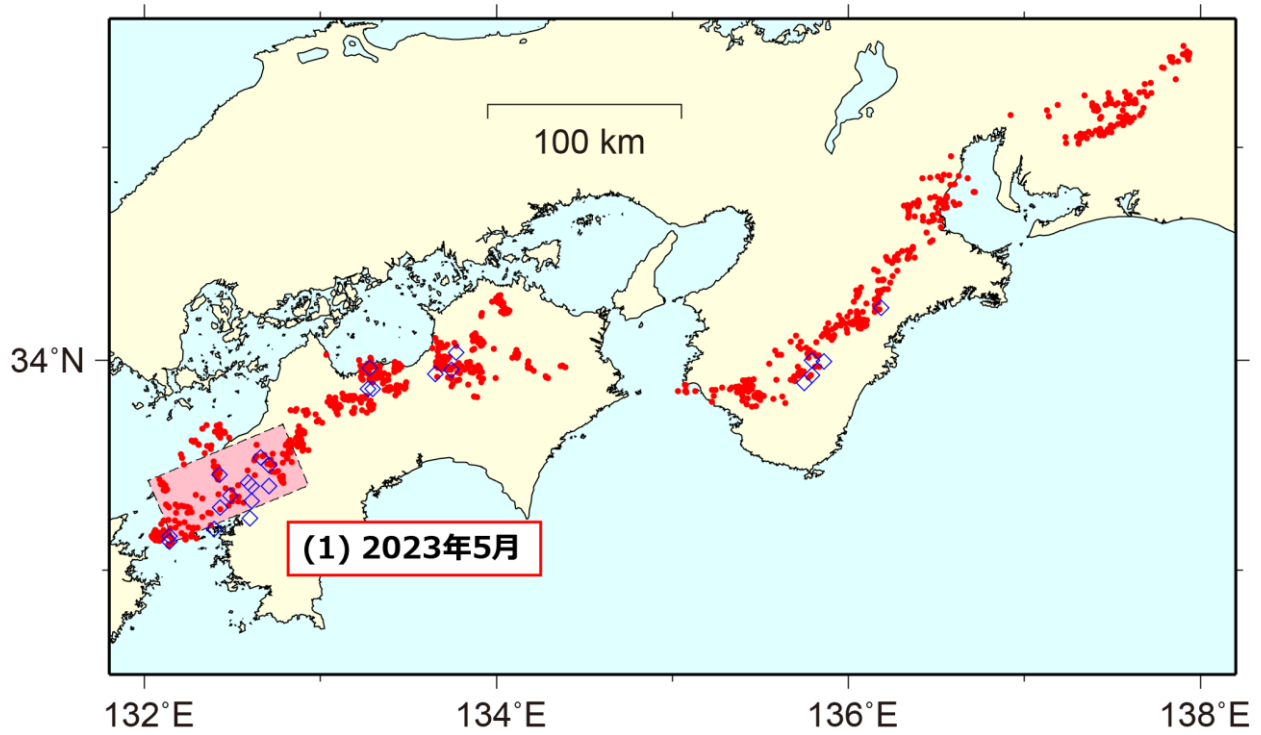
第 1 図 2023 年 5 月 1 日～10 月 31 日の期間に検知された短期的 SSE (ピンク矩形). 同期間に発生した深部低周波微動 (赤点) 及び VLFE の震央 (青菱形) を重ねて表示した.
