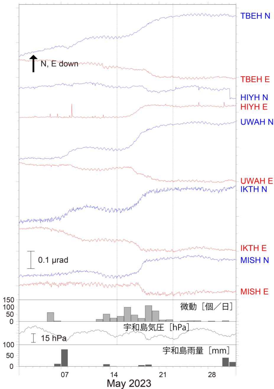
第 2 図 2023 年 5 月 1 日から 5 月 31 日までの傾斜時系列。観測点位置は第 3 図に示した。記録は上方向への変化が北・東下がり傾斜変動を表す。気圧応答・潮汐成分を BAYTAP-G 4) により除去し、直線トレンドを補正した後の記録を示した。5 月 15 日～5 月 22 日の傾斜変化量を SSE によるものと仮定した。四国西部～中部での微動活動度・気象庁宇和島観測点での気圧変化および雨量をあわせて表示した。
