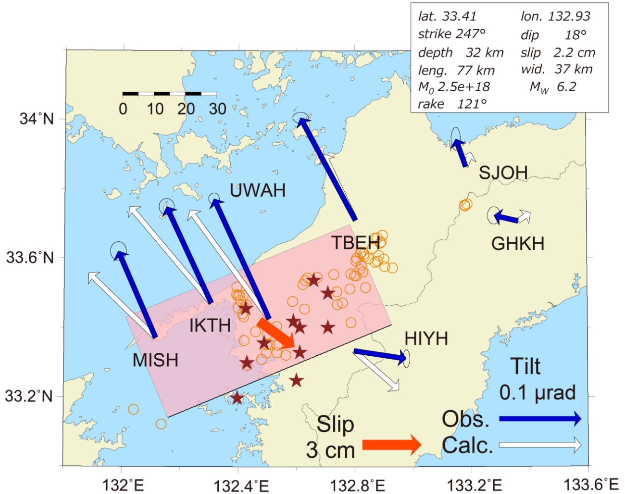
第 3 図 2023 年 5 月四国西部の短期的 SSE の断層モデル。第 2 図の破線で示された期間に観測された傾斜変化ベクトル (青矢印)・このデータから推定された SSE の断層モデル (赤矩形・矢印)・モデルから計算される傾斜変化ベクトル (白抜き矢印) を示す。同じ期間の微動と VLFE の震央を橙円と茶星印で示した。
