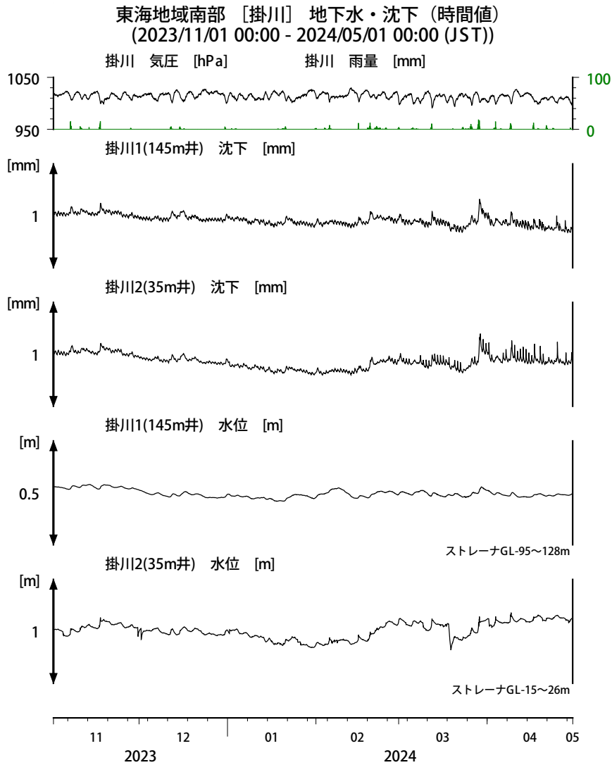
第 5 図 掛川における沈下等の観測結果 (2023 年 11 月～2024 年 4 月) Fig. 5 Observed subsidence data and others at the Kakegawa observation well from Nov. 2023 to Apr. 2024.
