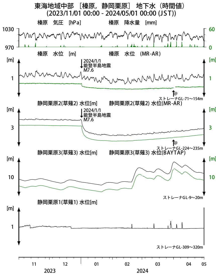
第3図 東海地域中部の地下水等の観測結果 (2023年11月～2024年4月) Fig. 3 Observed groundwater levels and others in the central Tokai district from Nov. 2023 to Apr. 2024.
