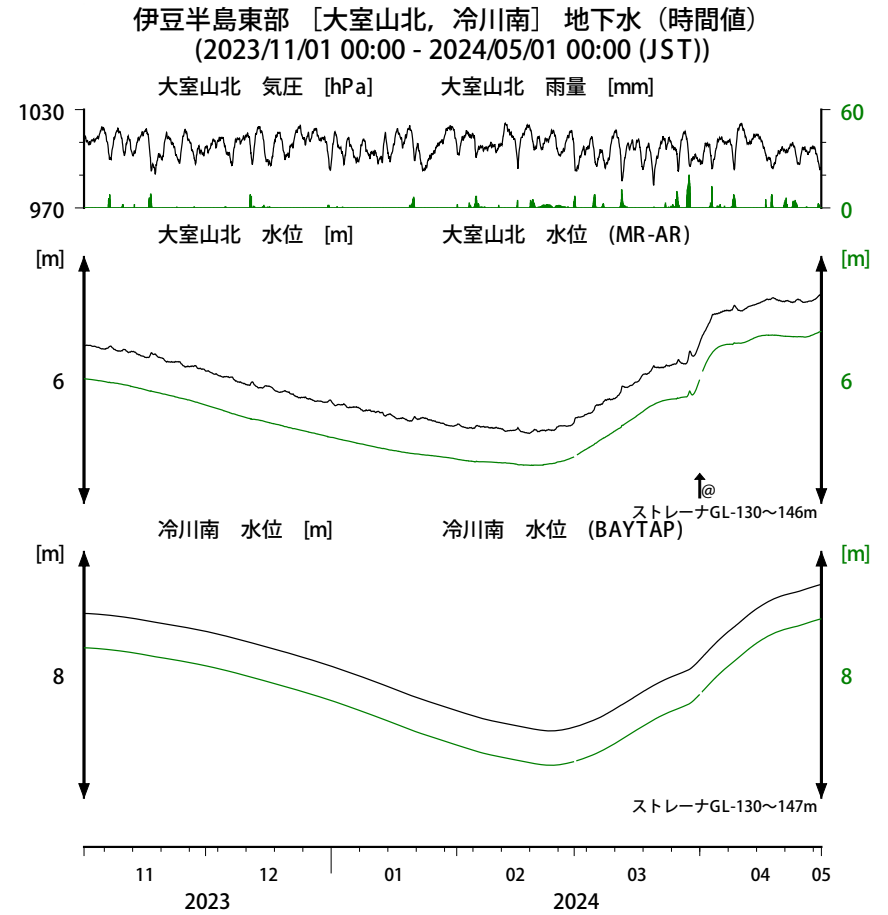
第 6 図 伊豆半島東部の地下水等の観測結果 (2023 年 11 月～2024 年 4 月) Fig. 6 Observed groundwater levels and others in the eastern Izu peninsula district from Nov. 2023 to Apr. 2024.
