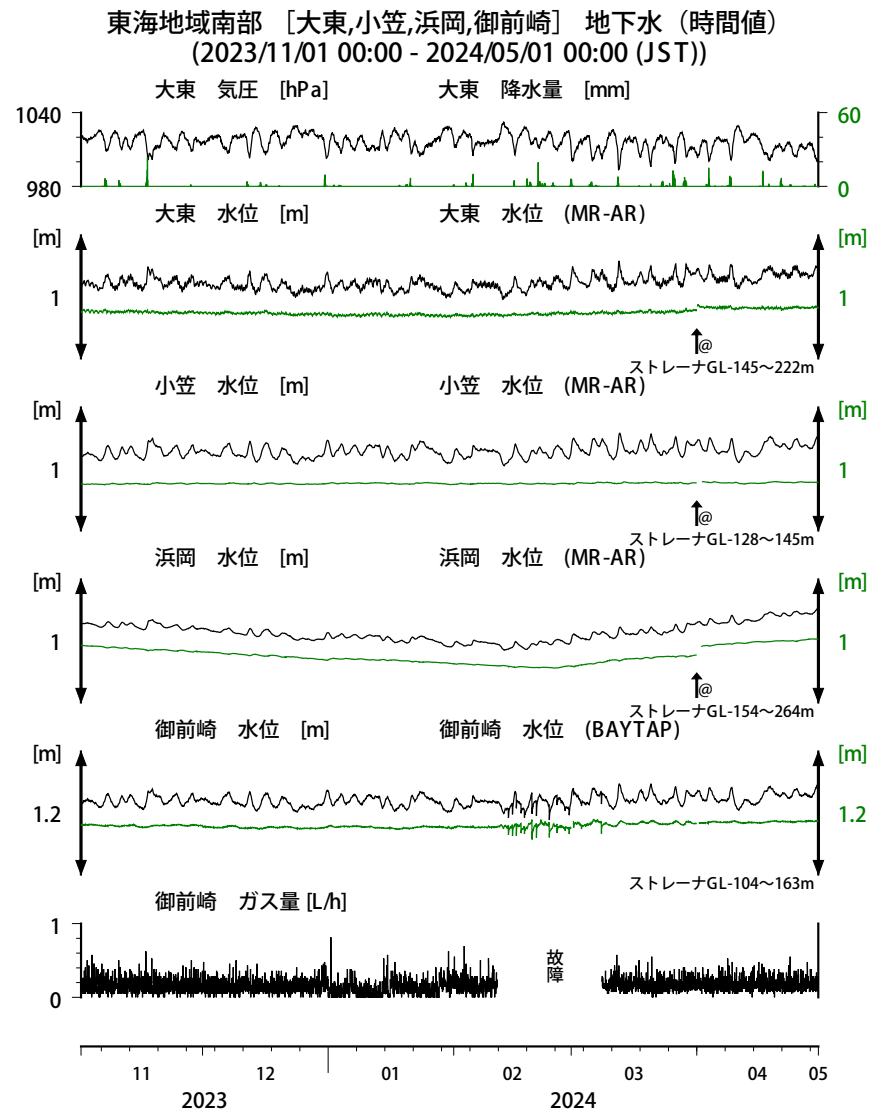
第4図 東海地域南部の地下水等の観測結果 (2023年11月～2024年4月) Fig. 4 Observed groundwater levels and others in the southern Tokai district from Nov. 2023 to Apr. 2024.
