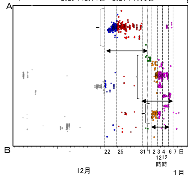
第 6 図 (a) 東海から紀伊半島中部の深部低周波地震活動とひずみ変化, 及び推定されるゆっくりすべり領域
