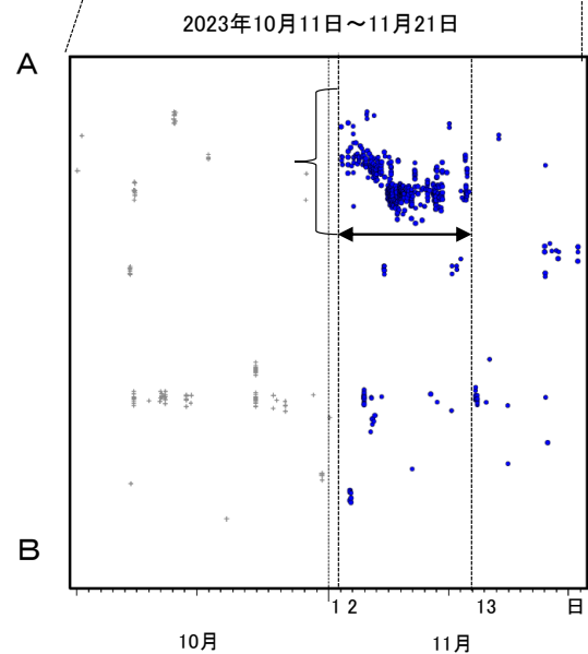
第 4 図 (a) 四国東部の深部低周波地震活動とひずみ変化, 及び推定されるゆっくりすべり領域
