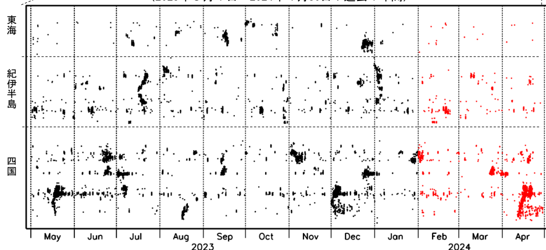
(2023年 5 月 1 日～2024年 4 月 30 日：過去 1 年間)
