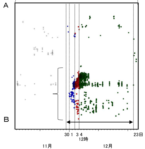
第 5 図 (a) 四国西部の深部低周波地震活動とひずみ変化, 及び推定されるゆっくりすべり領域
