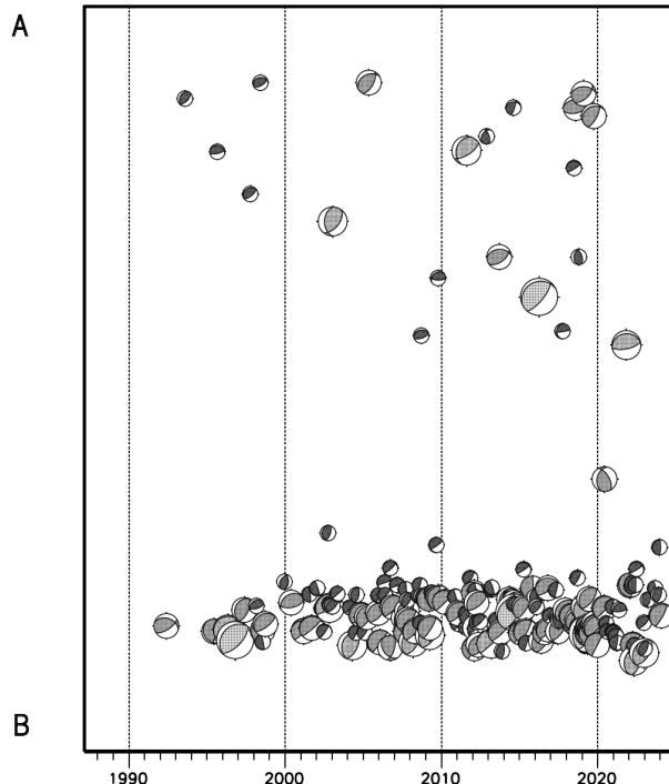
第 13 図 想定南海トラフ地震の発震機構解と類似の型の地震
