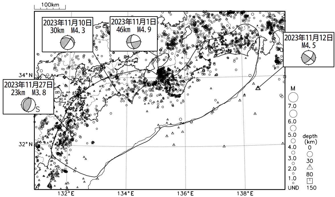
第 1 図 (a) 南海トラフ周辺の月別震央分布 (2023 年 11 月)
