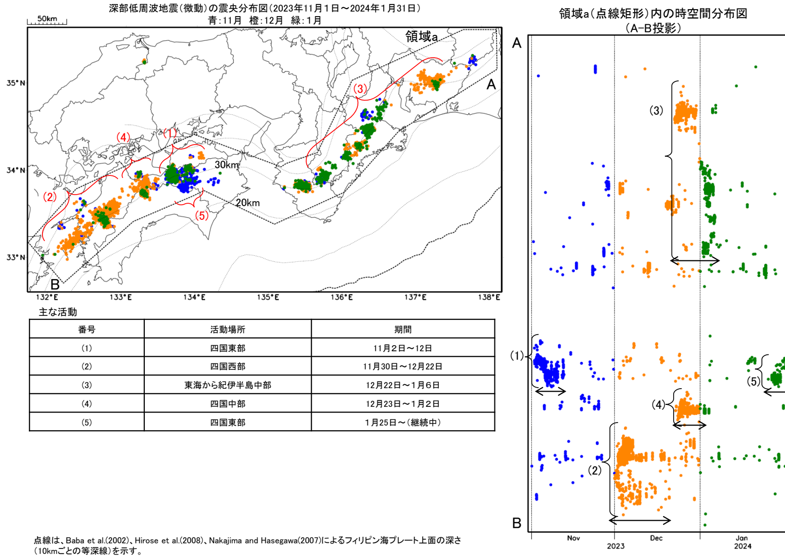
第2図(a) 東海地域から豊後水道にかけての深部低周波地震活動(2023年11月~2024年1月)
