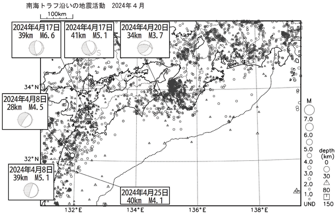
第 1 図 (f) つづき (2024 年 4 月)
