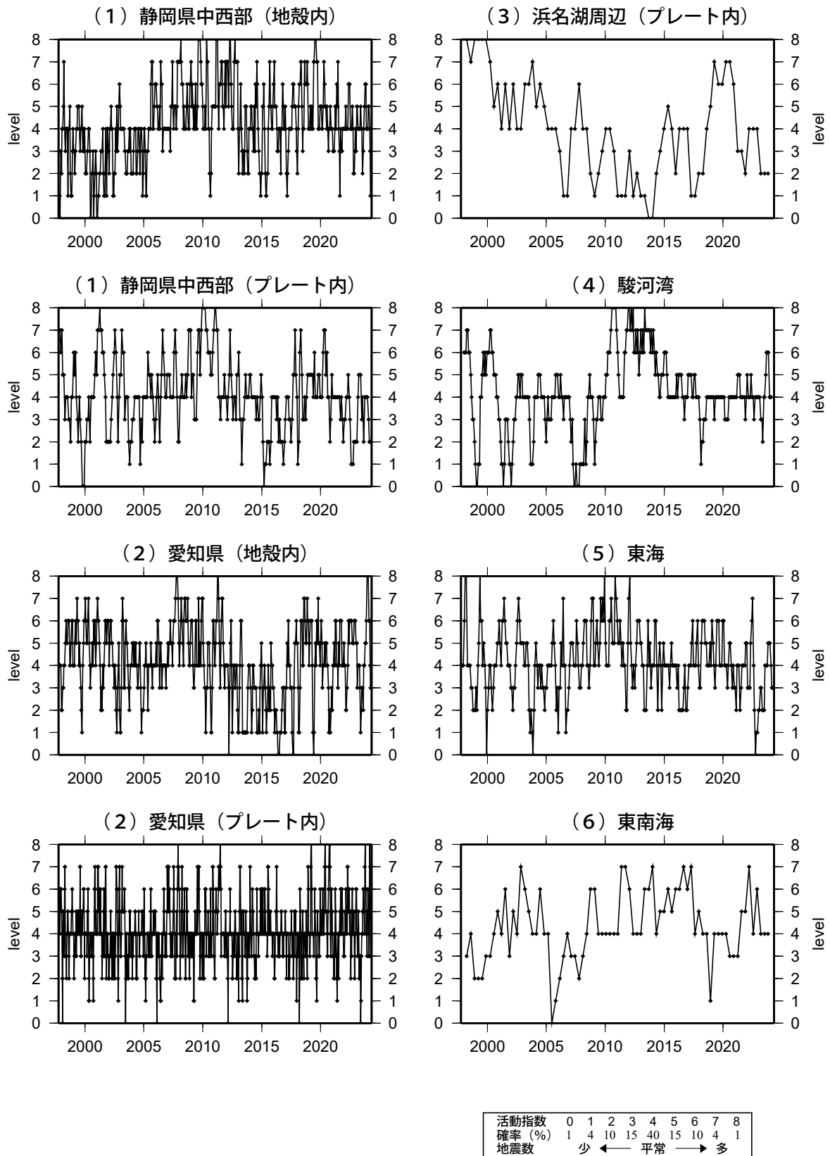
第 15 図 (a) 南海トラフ周辺の地震活動指数の推移
