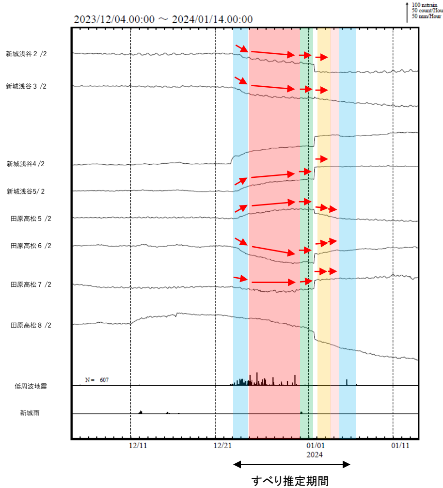
第 6 図 (b) つづき Fig. 6(b) Continued.
