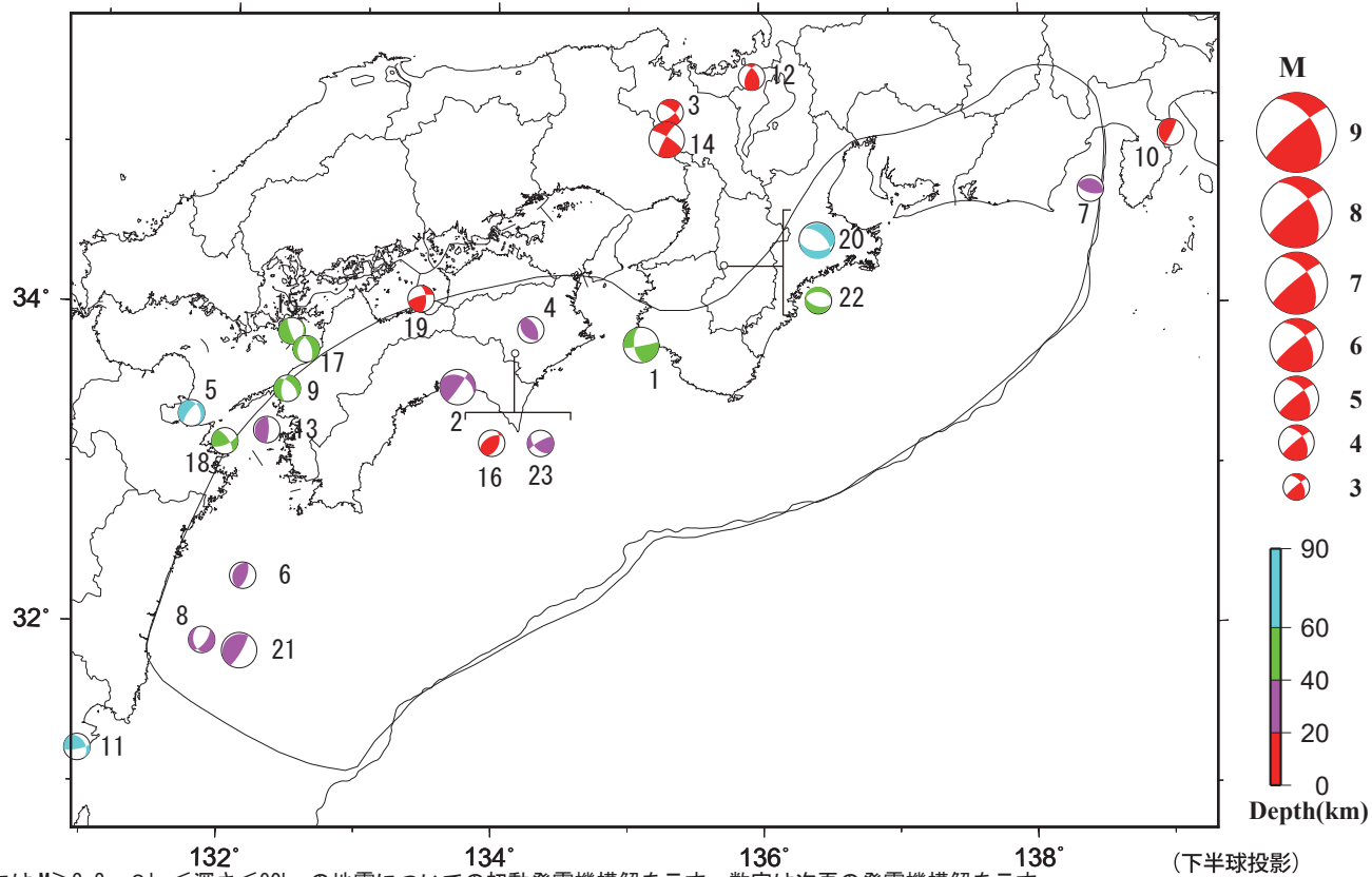
第3図(a) 南海トラフ周辺で発生した主な地震の発震機構解 (2023年11月～2024年1月)
