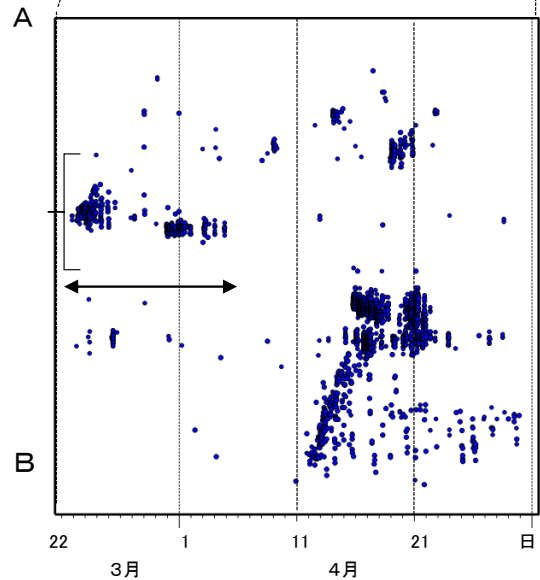
第 10 図 (a) 四国中部の深部低周波地震活動とひずみ変化, 及び推定されるゆっくりすべり領域
