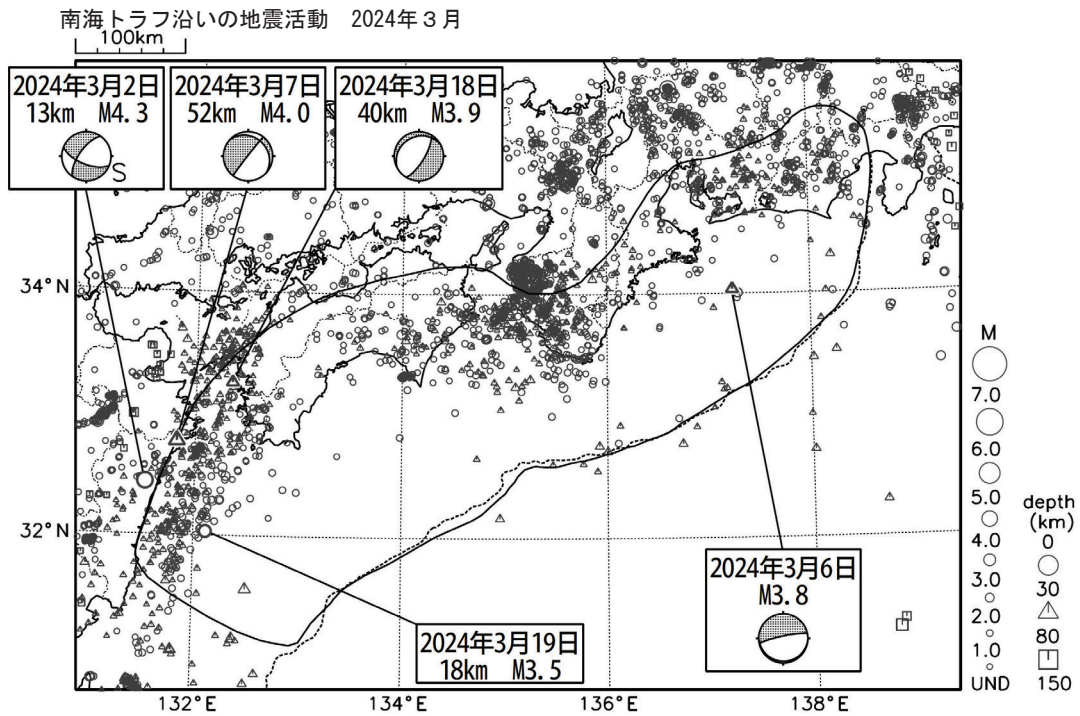
第 1 図 (e) つづき (2024 年 3 月)
