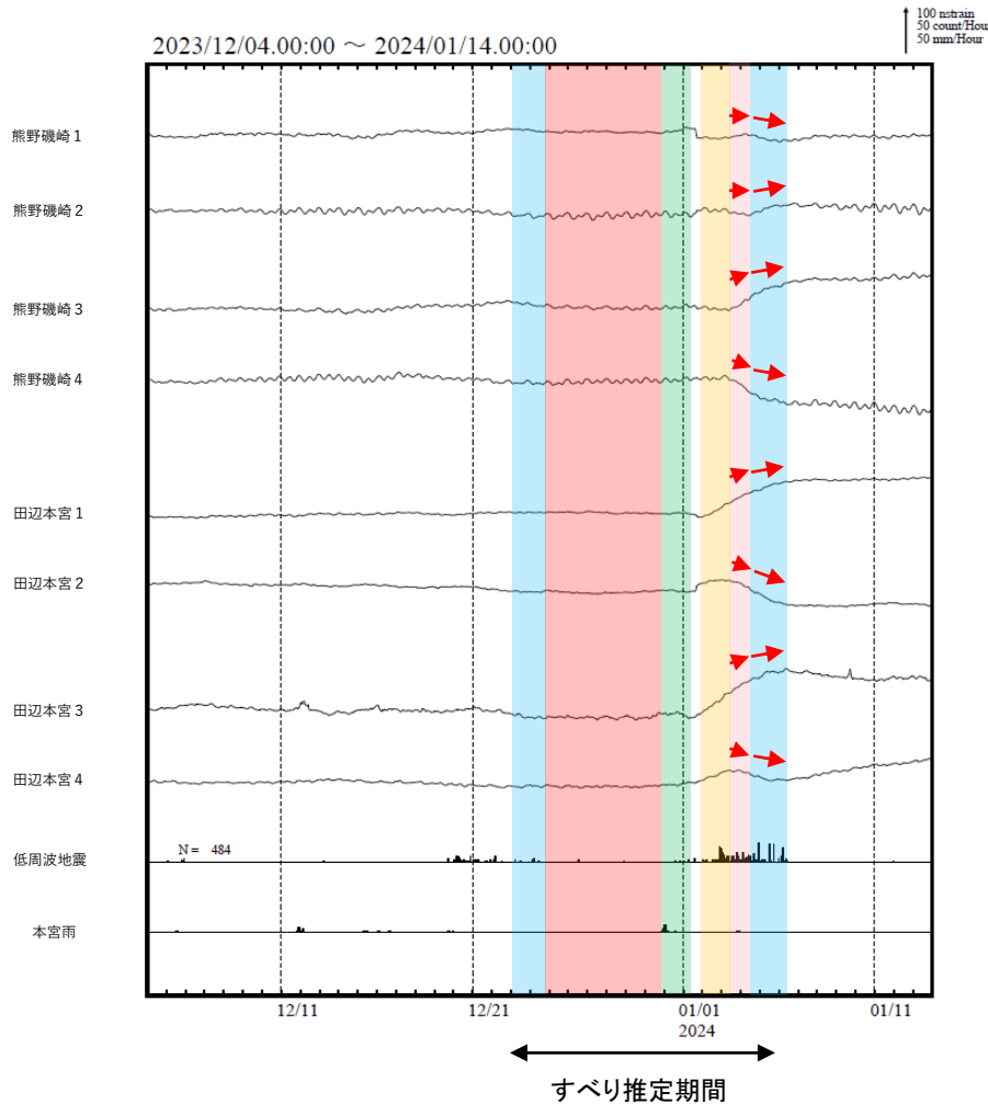
第 6 図 (b) つづき Fig. 6(b) Continued.
