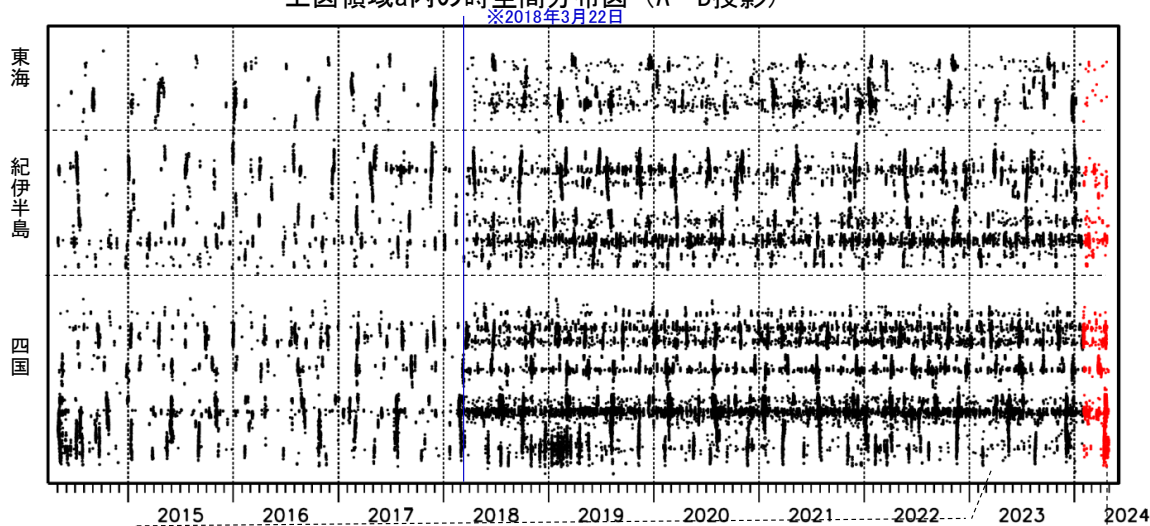
(2023年 5 月 1 日～2024年 4 月 30 日：過去 1 年間)
