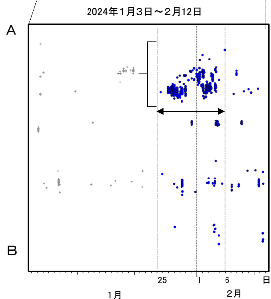
第 8 図 (a) 四国東部の深部低周波地震活動とひずみ変化, 及び推定されるゆっくりすべり領域
