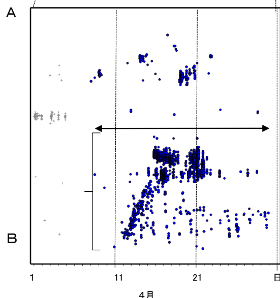
第 11 図 (a) 四国西部の深部低周波地震活動とひずみ変化, 及び推定されるゆっくりすべり領域
