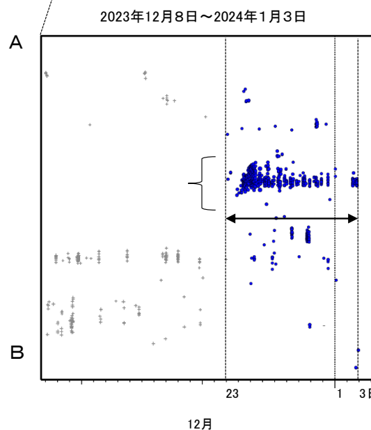
第 7 図 (a) 四国中部の深部低周波地震活動とひずみ変化, 及び推定されるゆっくりすべり領域
