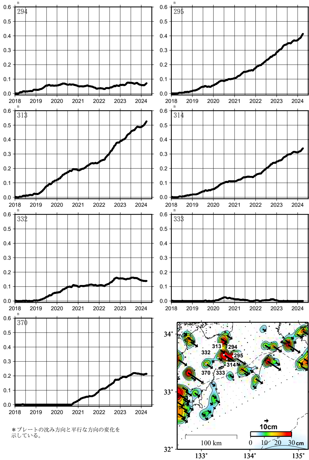
第 5 図 四国中部において推定される長期的ゆっくりすべり (暫定) (つづき)
