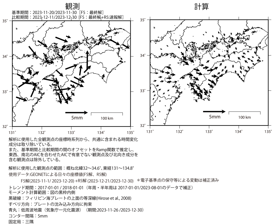
第 1 図 四国西部の深部低周波微動と同期したスロースリップ(暫定)
