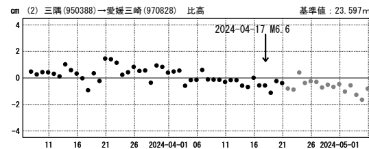
第 2 図 豊後水道の地震 (2024 年 4 月 17 日, M6.6) 前後の観測データ: (上図) 水平変動, (下図) 3 成分時系列グラフ
