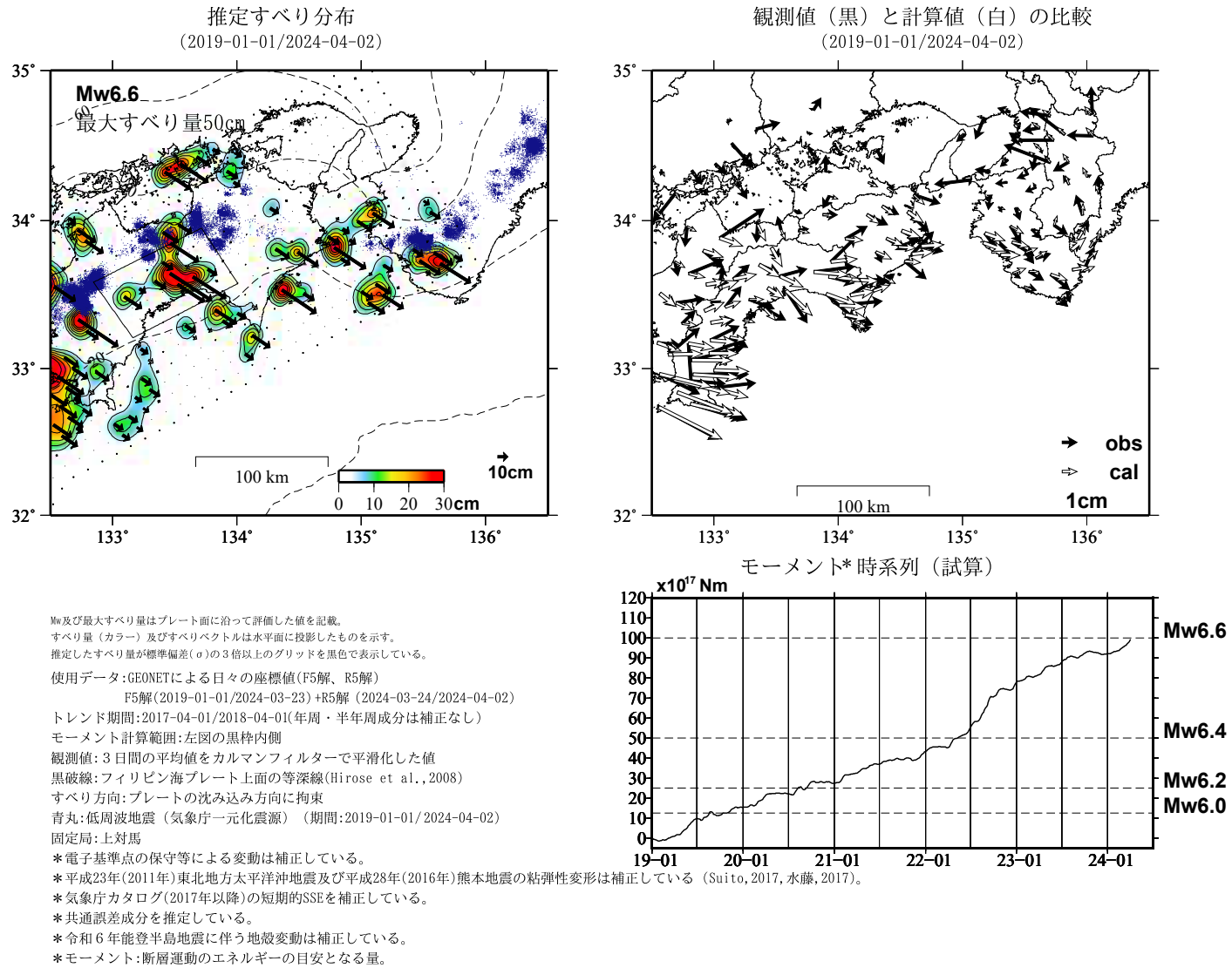
第4図 四国中部において推定される長期的ゆっくりすべり（暫定）
