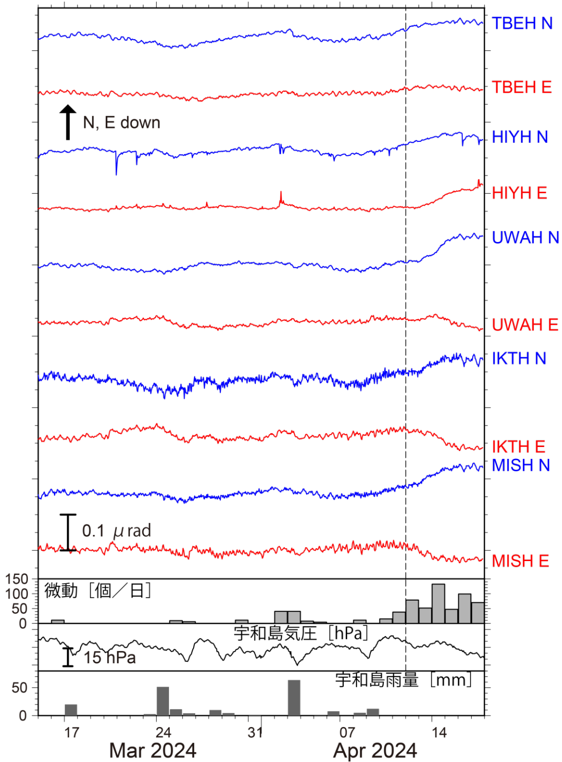
第 6 図 2024 年 3 月 15 日～4 月 17 日までの傾斜時系列. 図の見方は第 2 図と同様. 観測点位置は第 5 図に示した. 4 月 12 日～4 月 17 日 21 時の傾斜変化量を SSE によるものと仮定した. 四国西武での微動活動度・気象庁宇和島観測点での気圧変化および雨量をあわせて表示した.
