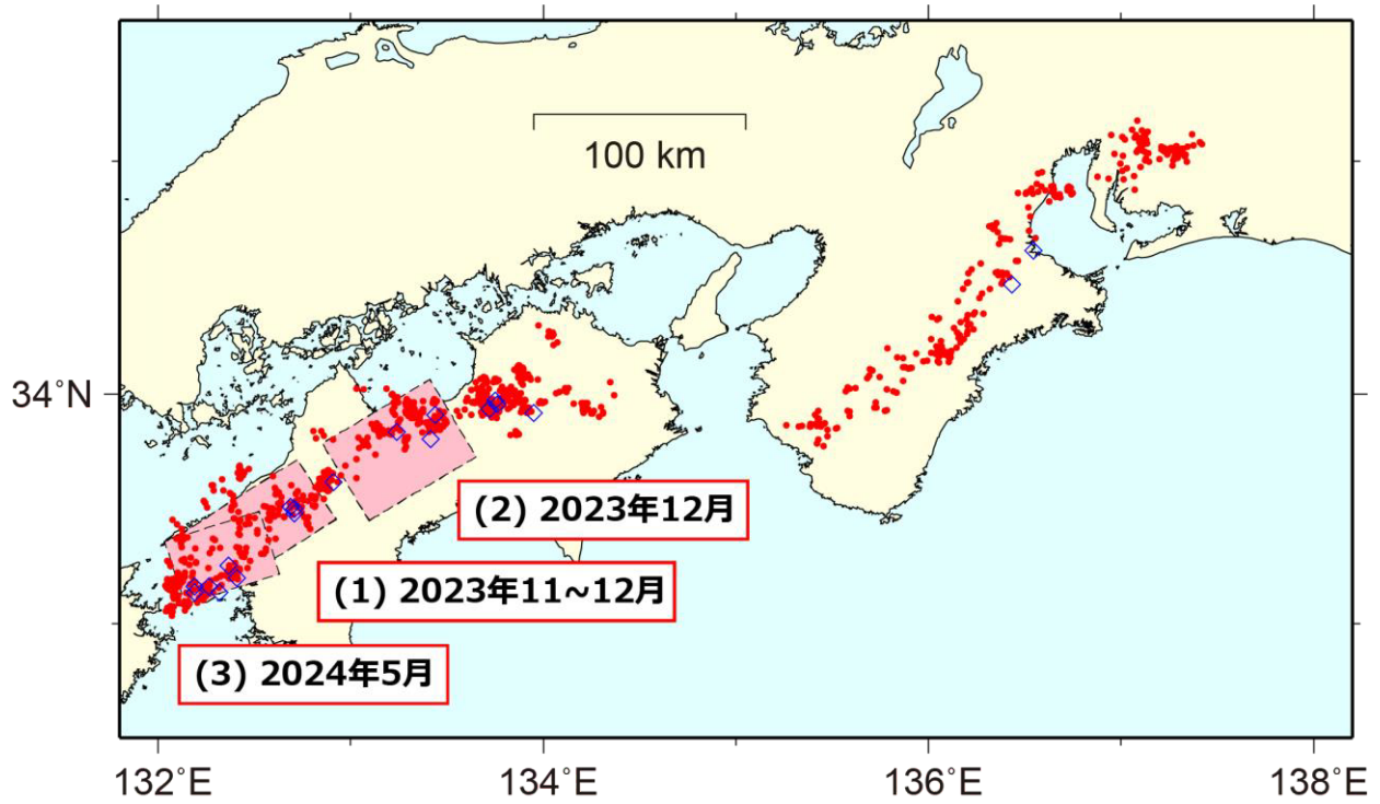
第 1 図 2023 年 11 月 1 日～2024 年 4 月 30 日の期間に検知された短期的 SSE (ピンク矩形). 同期間に発生した深部低周波微動 (赤点) 及び VLFE の震央 (青菱形) を重ねて表示した.
