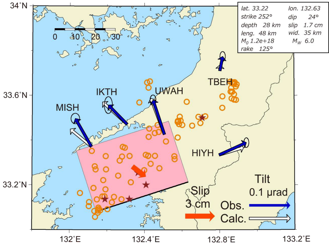
第 7 図 2024 年 4 月豊後水道の短期的 SSE の断層モデル. 図の見方は第 3 図と同じ.
