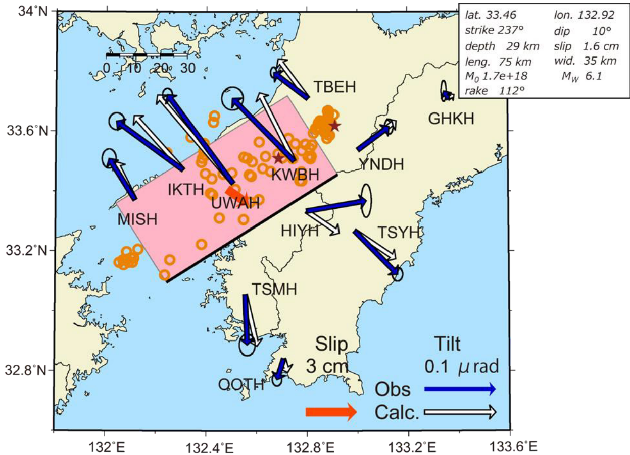
第 3 図 2023 年 11~12 月四国西部の短期的 SSE の断層モデル。第 2 図の破線で示された期間に観測された傾斜変化ベクトル (青矢印)・このデータから推定された SSE の断層モデル (赤矩形・矢印)・モデルから計算される傾斜変化ベクトル (白抜き矢印) を示す。同じ期間の微動と VLFE の震央を橙円と茶星印で示した。
