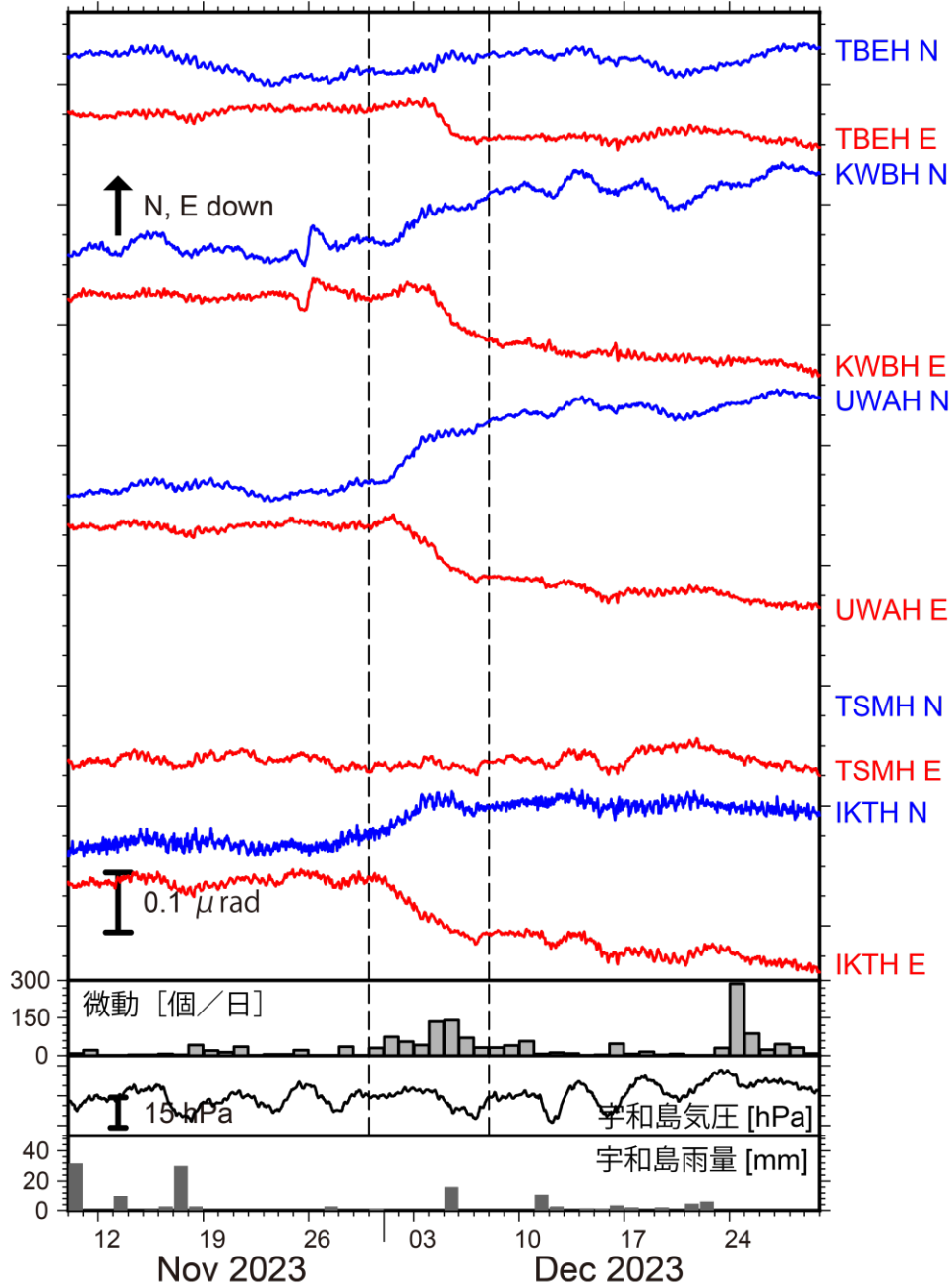
第 2 図 2023 年 11 月 10 日から 12 月 29 日までの傾斜時系列。観測点位置は第 3 図に示した。記録は上方向への変化が北・東下がり傾斜変動を表す。気圧応答・潮汐成分を BAYTAP-G 4) により除去し、直線トレンドを補正した後の記録を示した。11 月 30 日～12 月 7 日の傾斜変化量を SSE によるものと仮定した。四国西部～中部での微動活動度・気象庁宇和島観測点での気圧変化および雨量をあわせて表示した。
