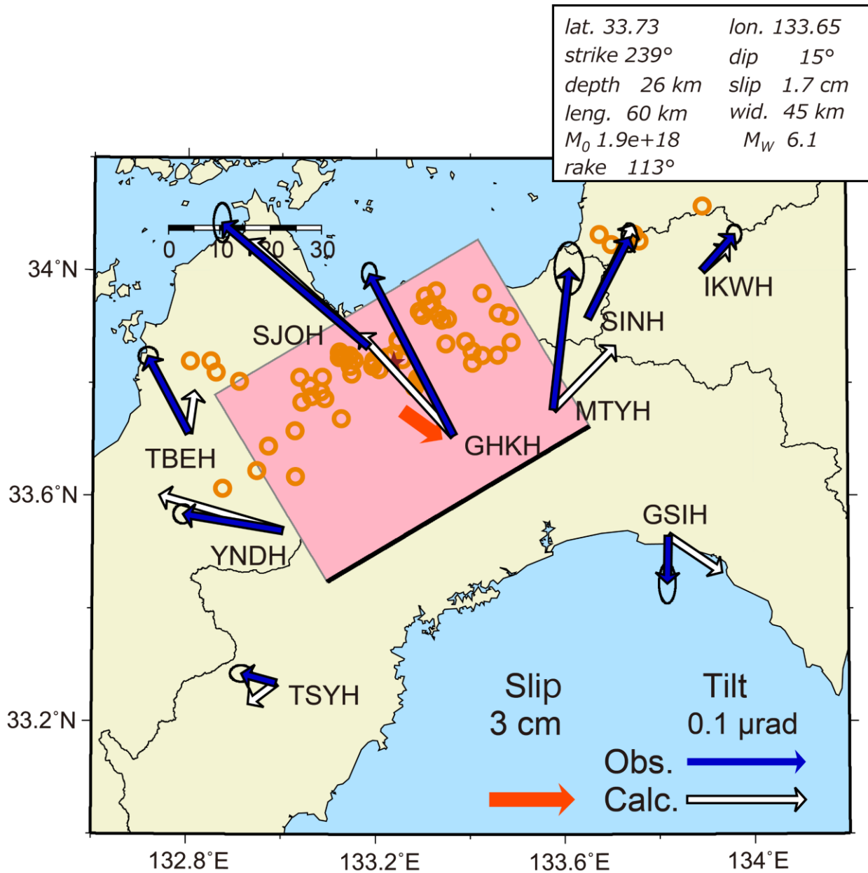
第 5 図 2023 年 12 月四国中部の短期的 SSE の断層モデル。図の見方は第 3 図と同じ。
