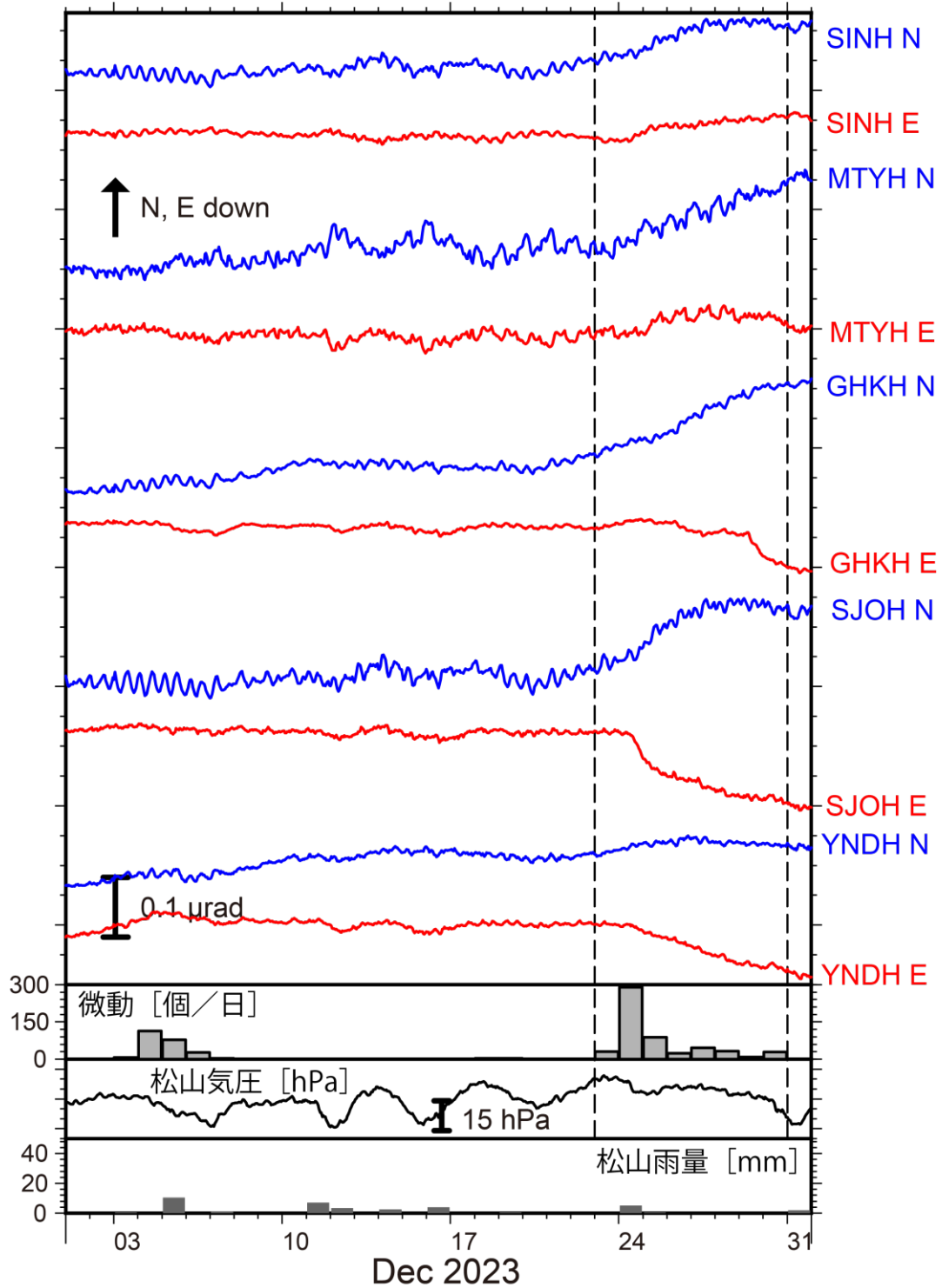
第 4 図 2023 年 12 月 1 日～12 月 31 日までの傾斜時系列。図の見方は第 2 図と同様。観測点位置は第 5 図に示した。12 月 23 日～12 月 30 日の傾斜変化量を SSE によるものと仮定した。四国中部での微動活動度・気象庁松山観測点での気圧変化および雨量をあわせて表示した。
