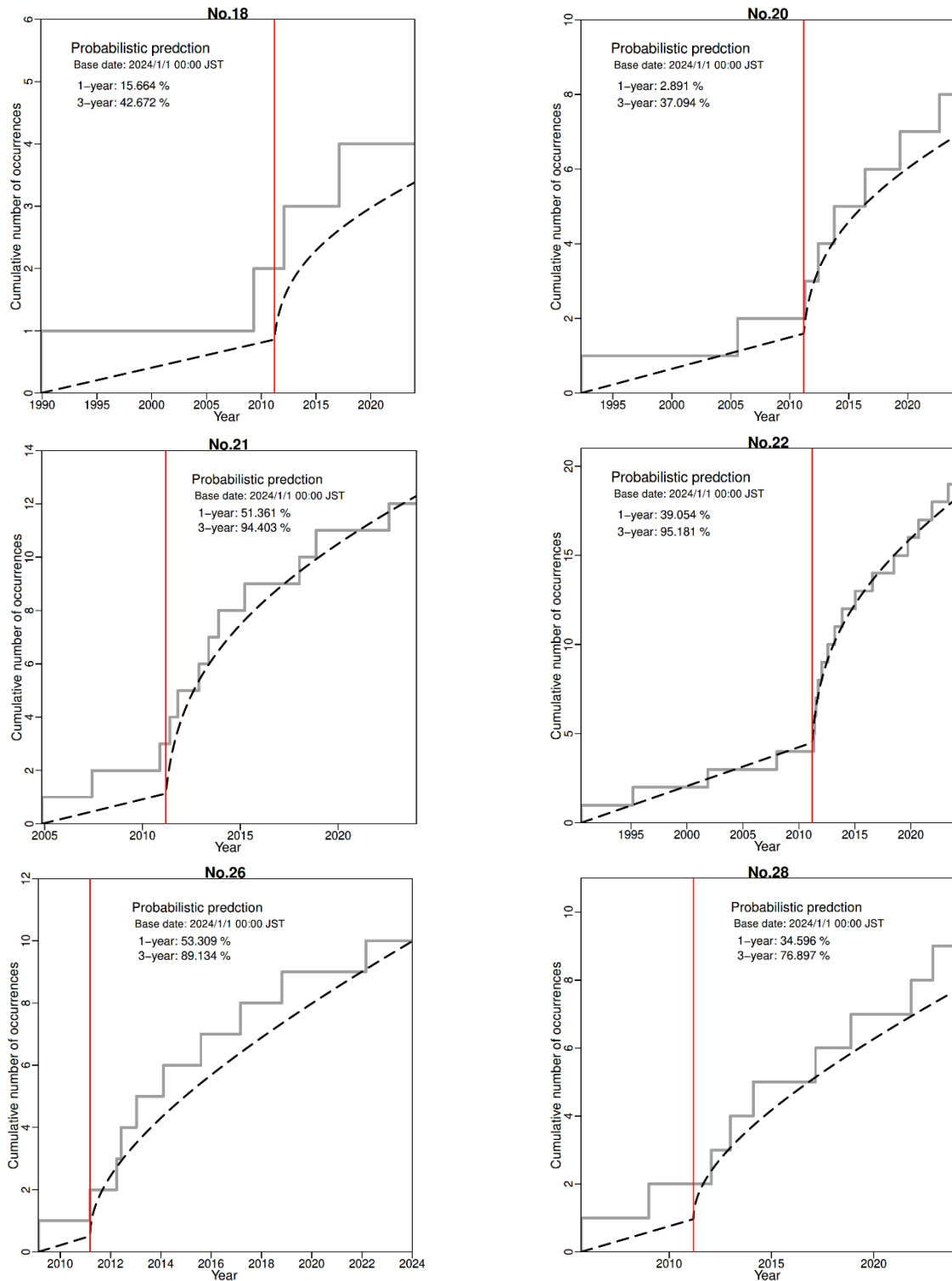
第 3 図 非定常更新過程モデルによる 2024 年 1 月から 1 年以内の発生確率
