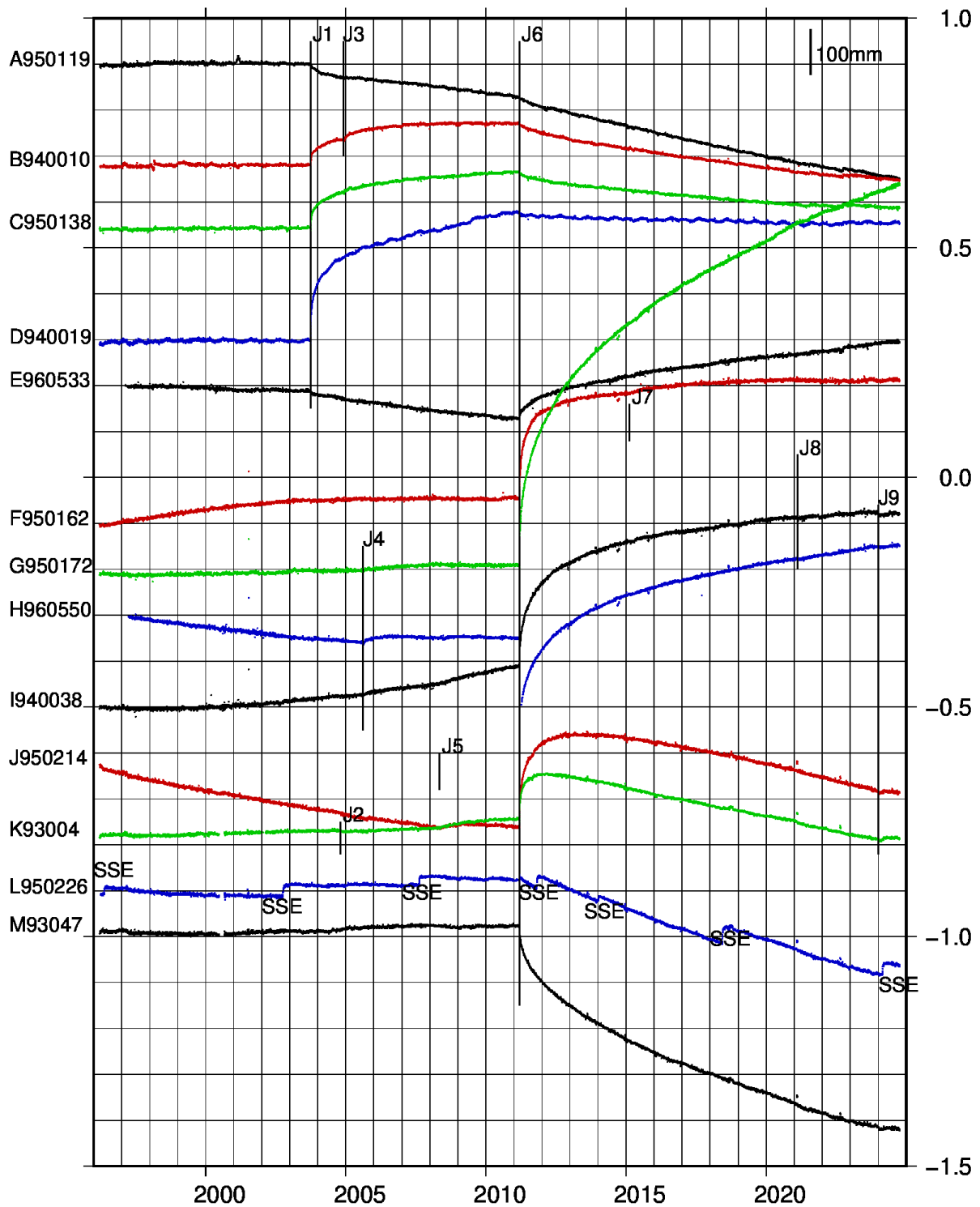
第 2a 図 プレート沈み込み方向の位置変化 (東日本 ; 1996 年から 2024 年 10 月) 沈み込みと逆方向が上向き。地点番号は、第 1 図の観測点記号に GEONET 観測点番号を付加したもの。 J1:2003 年十勝沖地震 (M8.0), J2:2004 年新潟県中越地震 (M6.8), J3:2004 年 11 月 29 日釧路沖の地震 (M7.1), J4:2005 年 8 月 16 日宮城県沖の地震 (M7.2), J5:2008 年 5 月 8 日茨城県沖の地震 (M7.0), J6:2011 年東北地方太平洋沖地震 (M9.0), J7:2015 年 2 月 17 日三陸沖の地震 (M6.9), J8:2021 年 2 月 13 日福島県沖の地震 (M7.3), J9: 2024 年能登半島地震 (M7.6).
