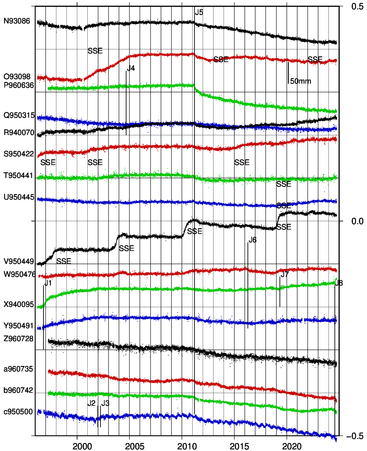
第 2b 図 プレート沈み込み方向の位置変化（西日本；1996 年から 2024 年 10 月） 沈み込みと逆方向が上向き。地点番号は、第 1 図の観測点記号に GEONET 観測点番号を付加したもの。 J1:1996 年 10 月 19 日日向灘の地震 (M6.9), J2:2001 年 12 月 18 日与那国島近海 (M7.3), J3:2002 年 3 月 31 日台湾付近の地震 (M7.2), J4:2004 年 9 月 5 日三重県南東沖の地震 (M7.4), J5:2011 年東北地方太平洋沖地震 (M9.0), J6:2016 年熊本地震 (M7.3), J7:2019 年 5 月 10 日日向灘の地震 (M6.3), J8:2024 年 8 月 8 日日向灘の地震 (M7.1).
