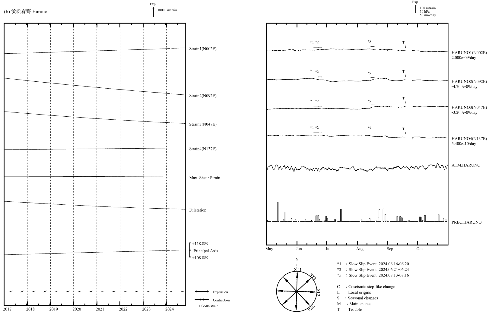
第 4 図 (b) 左 : 2017 年 1 月以後の多成分ひずみ計変化 (日平均値)。主ひずみ・最大せん断ひずみ・面積ひずみは各方向成分から計算されている。 右 : 2024 年 5 月～10 月の多成分ひずみ計変化 (時間値 : 気圧・潮汐・地磁気・降水補正した値)。各図下部に気圧変化と降水量を示す。
