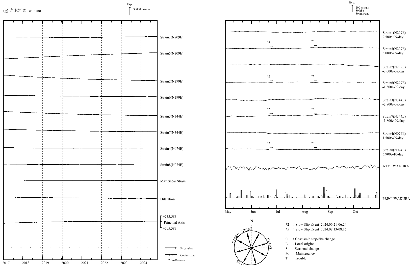
第 4 図 (g) 左 : 2017 年 1 月以後の多成分ひずみ計変化 (日平均値)。主ひずみ・最大せん断ひずみ・面積ひずみは各方向成分から計算されている。 右 : 2024 年 5 月～10 月の多成分ひずみ計変化 (時間値 : 気圧・潮汐・地磁気・降水補正した値)。各図下部に気圧変化と降水量を示す。
