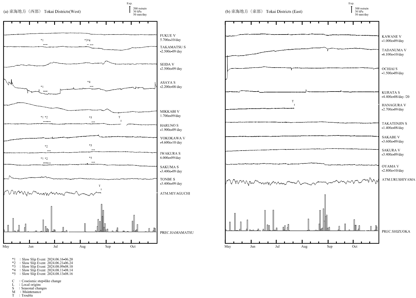
第 3 図 (a),(b) 2024 年 5 月～10 月の東海・伊豆・南関東地域における区域別体積ひずみ (V) 及び面積ひずみ (S) の変化 (時間値: 気圧・潮汐・降水補正した値). 各図下部に区域を代表する気圧変化と降水量を示す. 地点名の下に D strain/day 及び /M はそれぞれ 1 日あたりのトレンド変化量を D として補正していること及び縮尺を 1/M 倍にして表示していることを示している.
