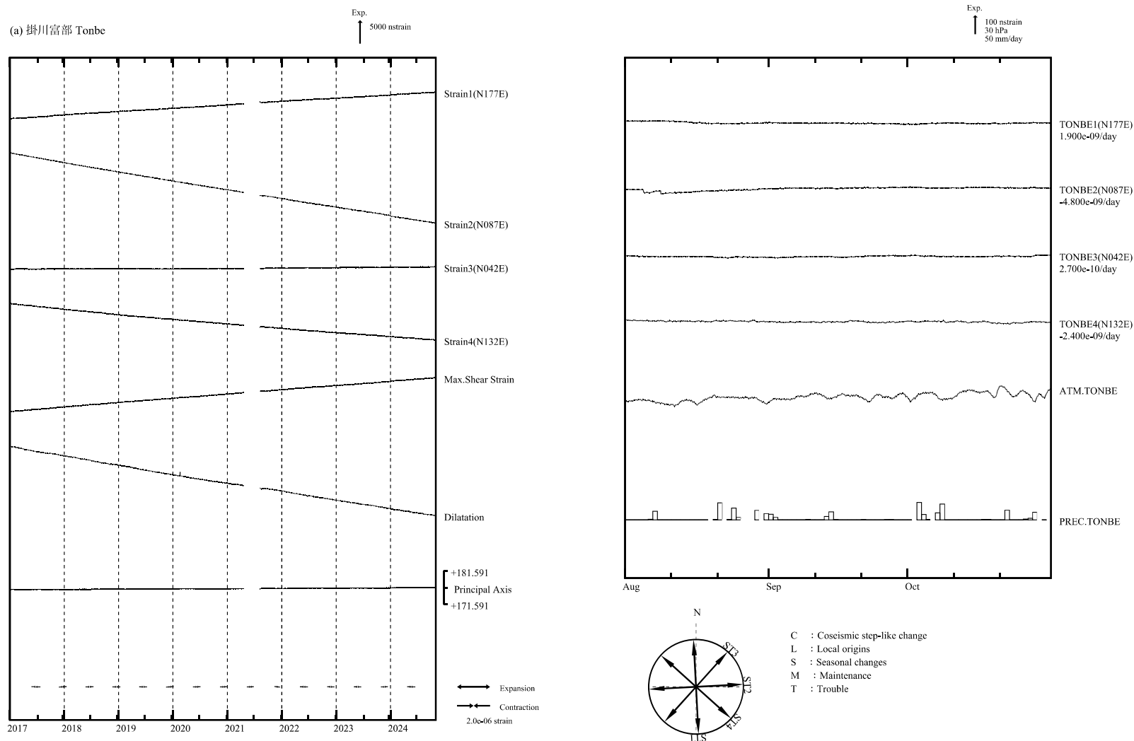
第 4 図 (a) 左 : 2017 年 1 月以後の多成分ひずみ計変化 (日平均値)。主ひずみ・最大せん断ひずみ・面積ひずみは各方向成分から計算されている。 右 : 2024 年 5 月～10 月の多成分ひずみ計変化 (時間値 : 気圧・潮汐・地磁気・降水補正した値)。各図下部に気圧変化と降水量を示す。
