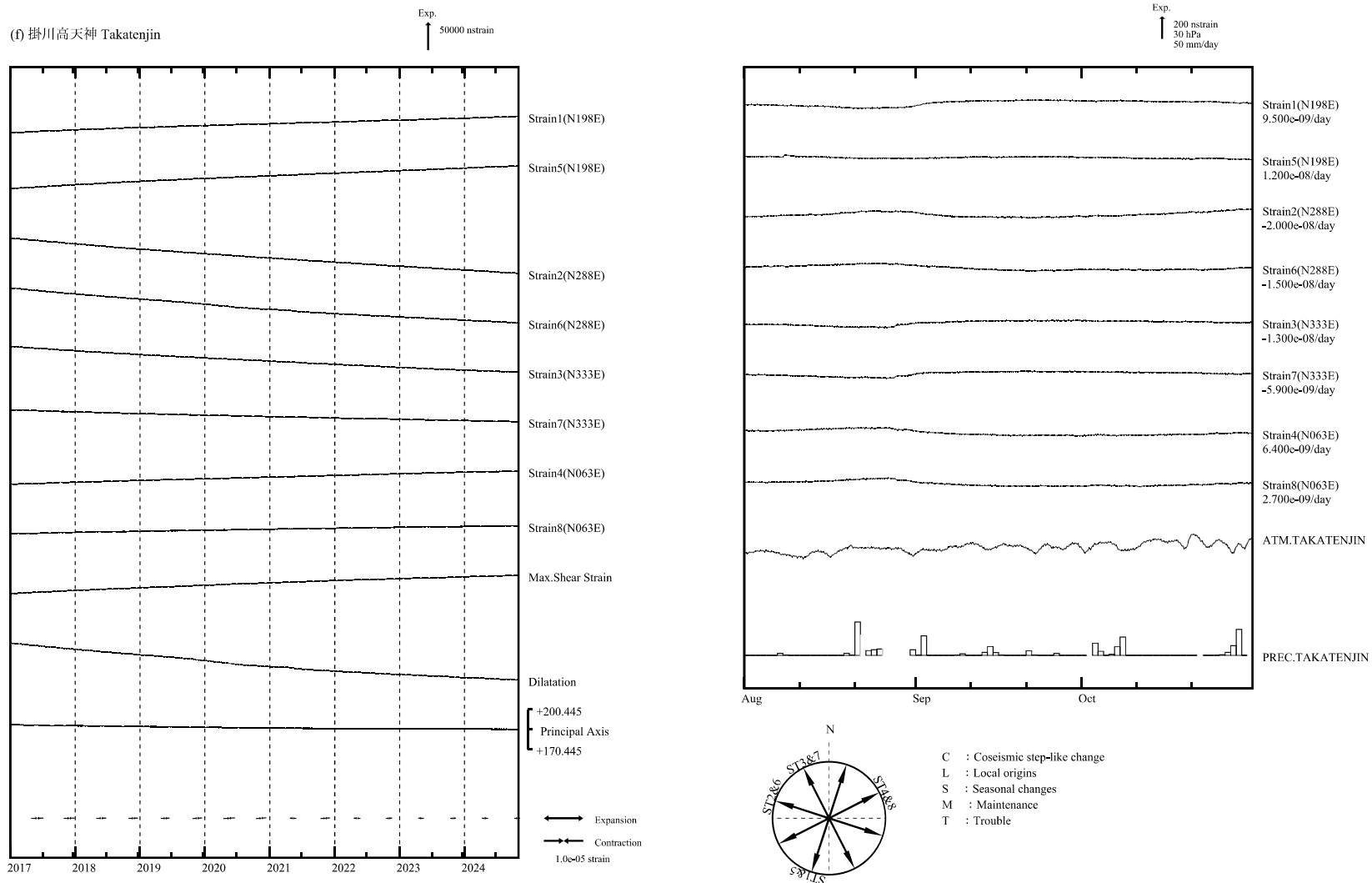
第4図(f) 左：2017年1月以後の多成分ひずみ計変化（日平均値）。主ひずみ・最大せん断ひずみ・面積ひずみは各方向成分から計算されている。 右：2024年5月～10月の多成分ひずみ計変化（時間値：気圧・潮汐・地磁気・降水補正した値）。各図下部に気圧変化と降水量を示す。
