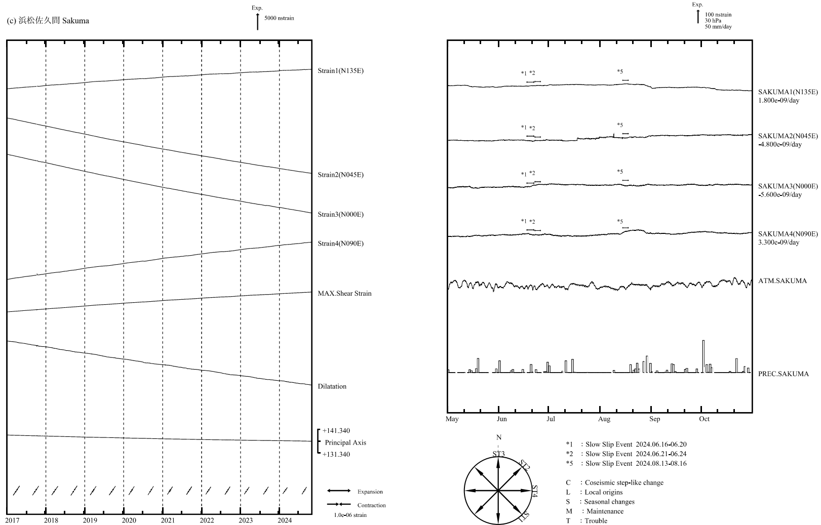
第 4 図 (c) 左 : 2017 年 1 月以後の多成分ひずみ計変化 (日平均値)。主ひずみ・最大せん断ひずみ・面積ひずみは各方向成分から計算されている。 右 : 2024 年 5 月～10 月の多成分ひずみ計変化 (時間値 : 気圧・潮汐・地磁気・降水補正した値)。各図下部に気圧変化と降水量を示す。
