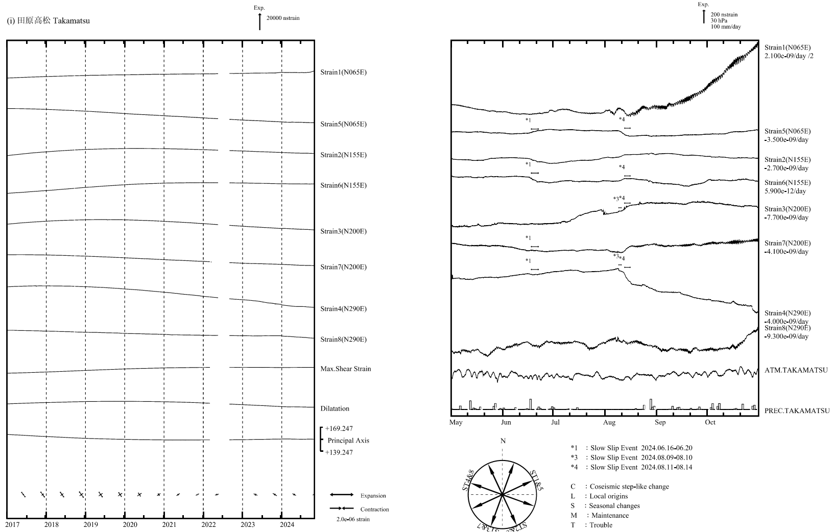
第 4 図 (i) 左 : 2017 年 1 月以後の多成分ひずみ計変化 (日平均値)。主ひずみ・最大せん断ひずみ・面積ひずみは各方向成分から計算されている。 右 : 2024 年 5 月～10 月の多成分ひずみ計変化 (時間値 : 気圧・潮汐・地磁気・降水補正した値)。各図下部に気圧変化と降水量を示す。
