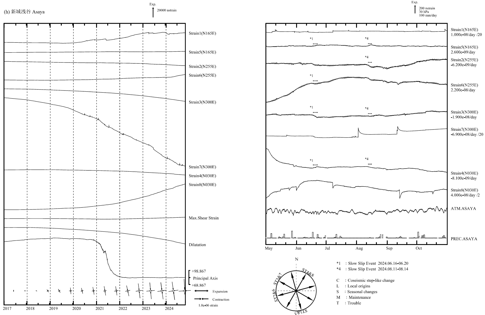
第 4 図 (h) 左 : 2017 年 1 月以後の多成分ひずみ計変化 (日平均値)。主ひずみ・最大せん断ひずみ・面積ひずみは各方向成分から計算されている。 右 : 2024 年 5 月～10 月の多成分ひずみ計変化 (時間値 : 気圧・潮汐・地磁気・降水補正した値)。各図下部に気圧変化と降水量を示す。
