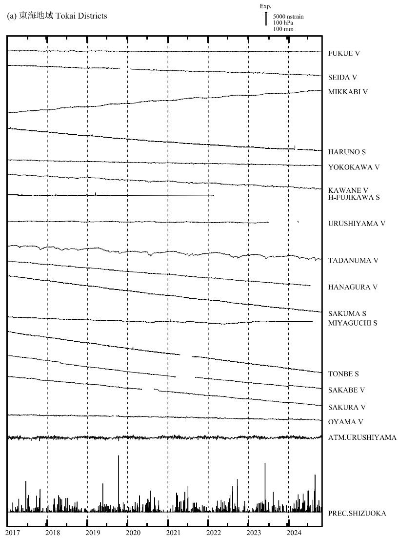
第 2 図 (a),(b) 2017 年 1 月以後の東海・伊豆・南関東地域における区域別体積ひずみ (V) 及び面積ひずみ (S) の変化 (日平均値). 各図下部に区域を代表する気圧変化と降水量を示す.
