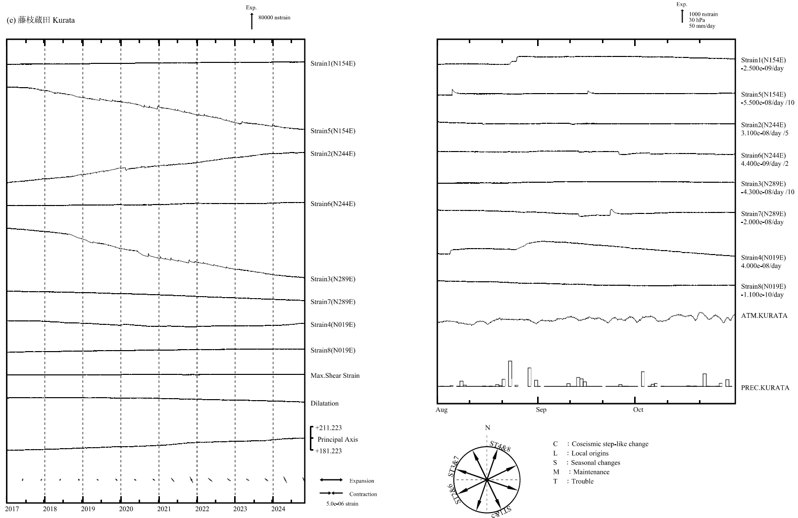
第 4 図 (e) 左 : 2017 年 1 月以後の多成分ひずみ計変化 (日平均値)。主ひずみ・最大せん断ひずみ・面積ひずみは各方向成分から計算されている。 右 : 2024 年 5 月～10 月の多成分ひずみ計変化 (時間値 : 気圧・潮汐・地磁気・降水補正した値)。各図下部に気圧変化と降水量を示す。
