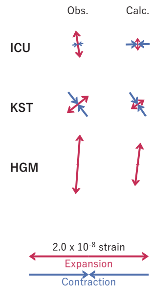
(b2) 主歪
