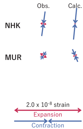
(b2) 主歪
