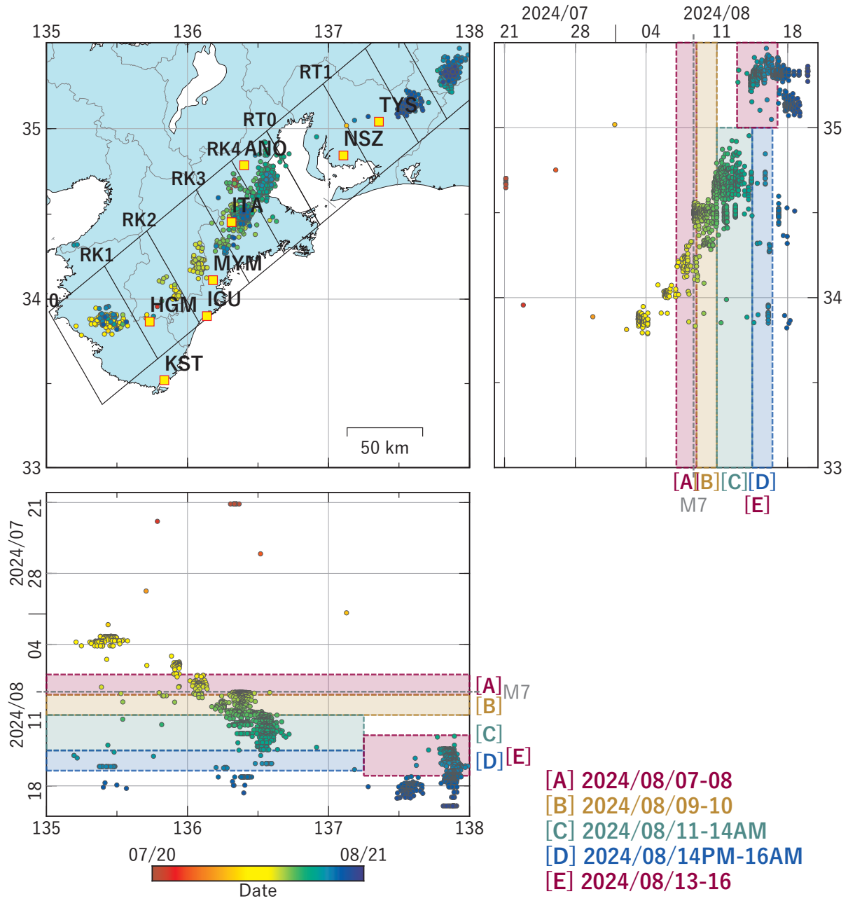
第 17 図 紀伊半島から東海地方における低周波地震（気象庁一元化カタログによる）の時空間分布（2024/07/20～2024/08/20）. [M7] は日向灘における Mj7.1 の地震の発生時刻.
