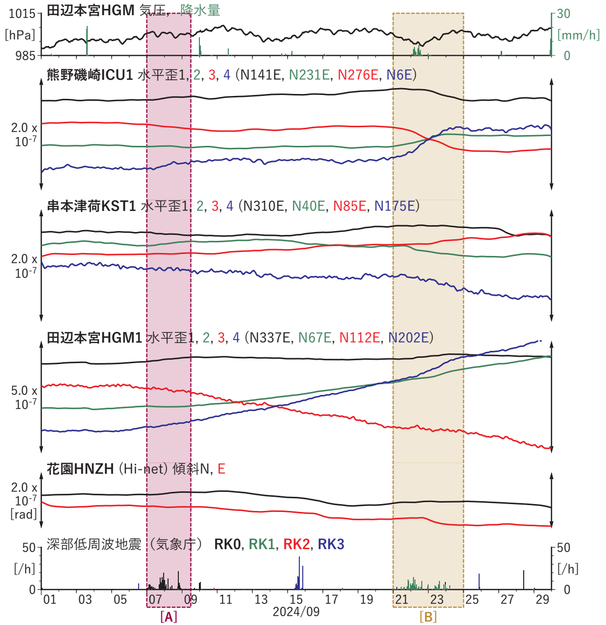
第 34 図 紀伊半島における歪・傾斜の観測結果と低周波地震の検出数 (2024/09/01 ~ 2024/09/29)。
