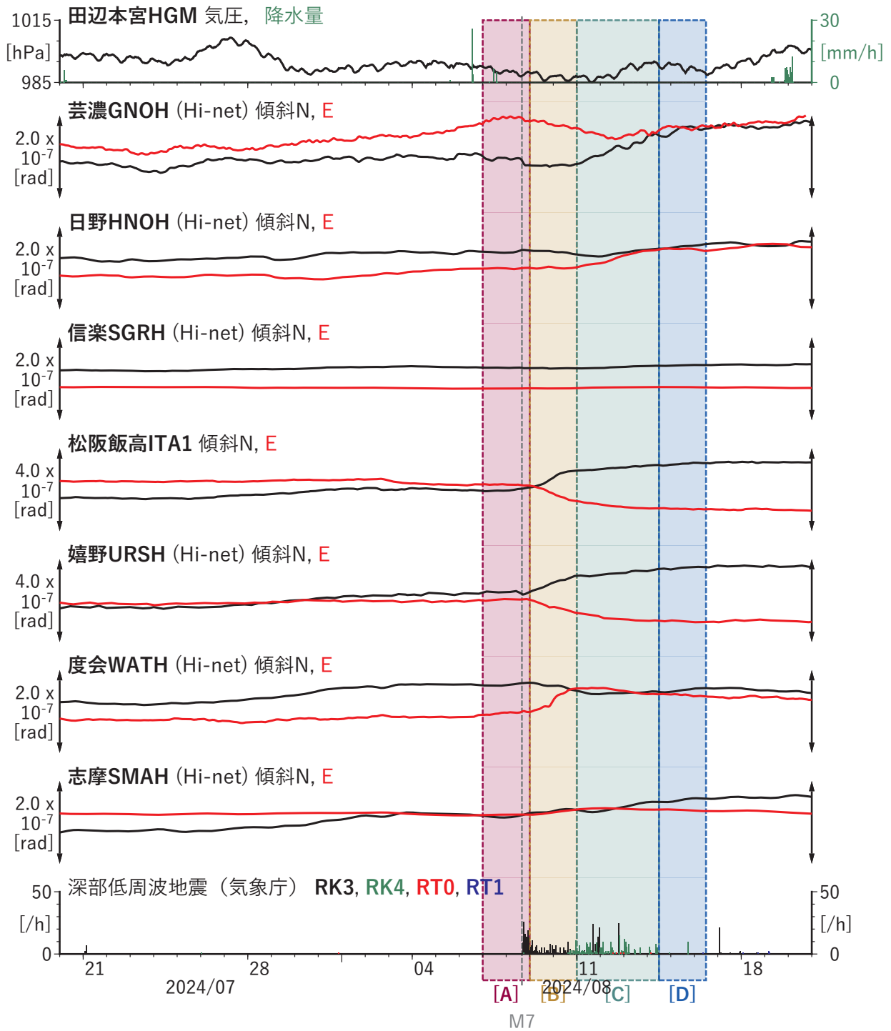
第 22 図 紀伊半島における傾斜の観測結果と低周波地震の検出数 (2024/07/20 ~ 2024/08/20). [M7] は日向灘における Mj7.1 の地震の発生時刻.
