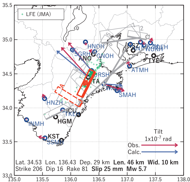
第 25 図 第 18-23 図 [B] を説明する断層モデル。各図の説明は第 3 図を参照。
