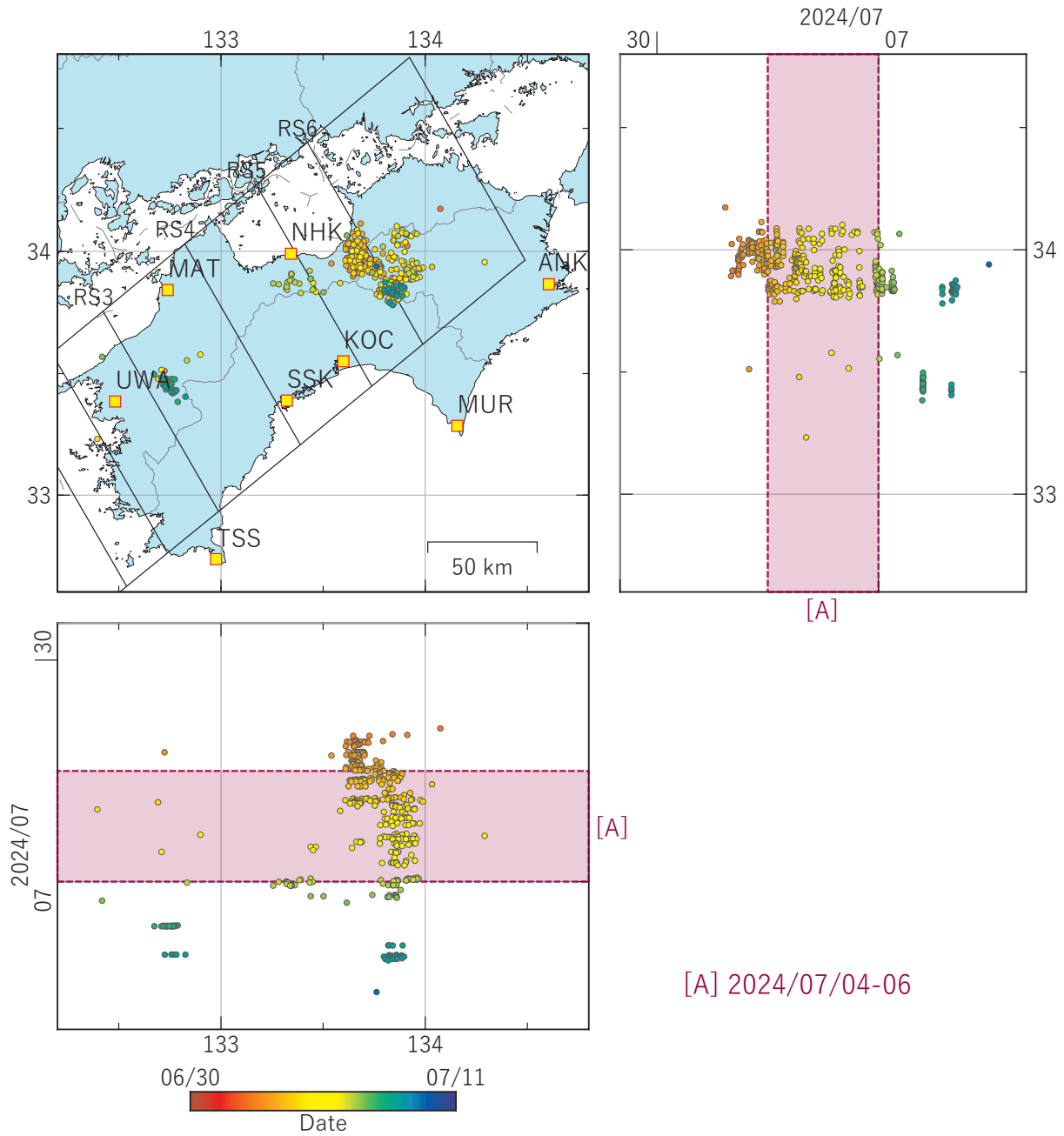
第 14 図 四国地域における低周波地震（気象庁一元化カタログによる）の時空間分布（2024/06/30 ～ 2024/07/10）。
