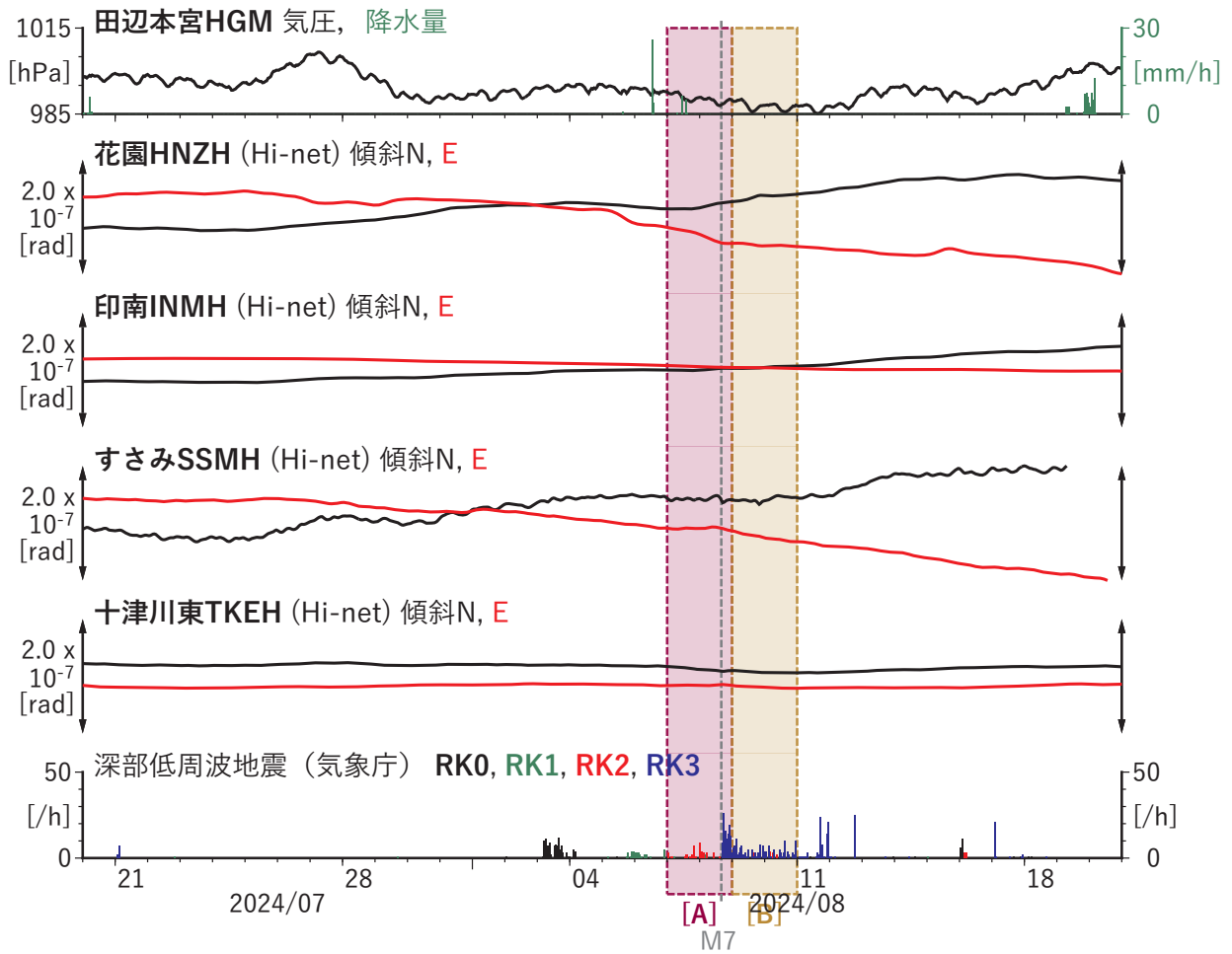
第 21 図 紀伊半島における傾斜の観測結果と低周波地震の検出数 (2024/07/20 ~ 2024/08/20)． [M7] は日向灘における M_j7.1 の地震の発生時刻．
