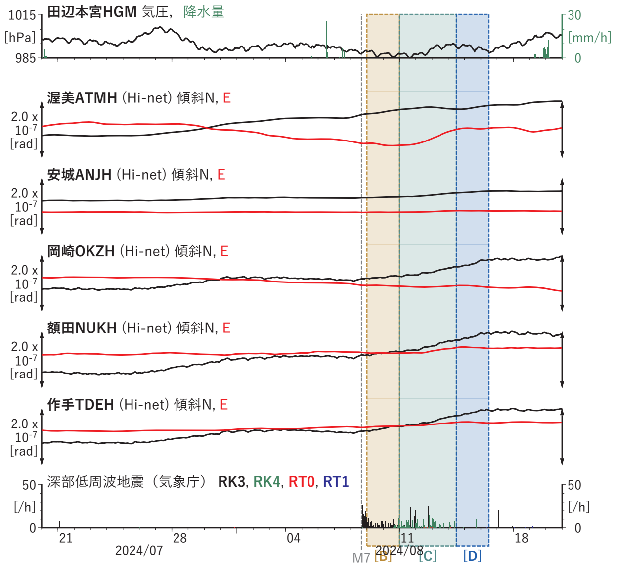
第 23 図 東海地方における傾斜の観測結果と低周波地震の検出数 (2024/07/20 ~ 2024/08/20). [M7] は日向灘における Mj7.1 の地震の発生時刻.
