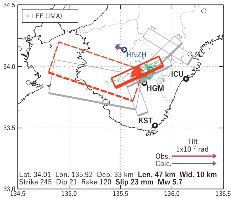
第 36 図 第 34 図 [B] を説明する断層モデル。各図の説明は第 3 図を参照。
