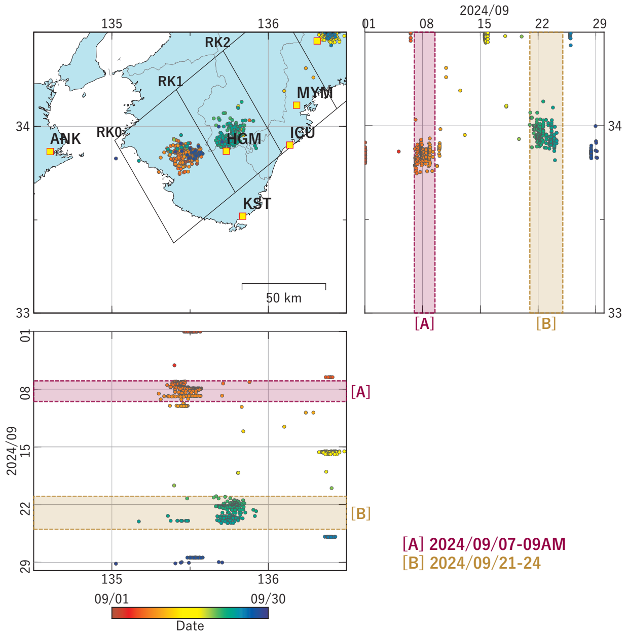
第 33 図 紀伊半島における低周波地震（気象庁一元化カタログによる）の時空間分布（2024/09/01 ～ 2024/09/29）。
