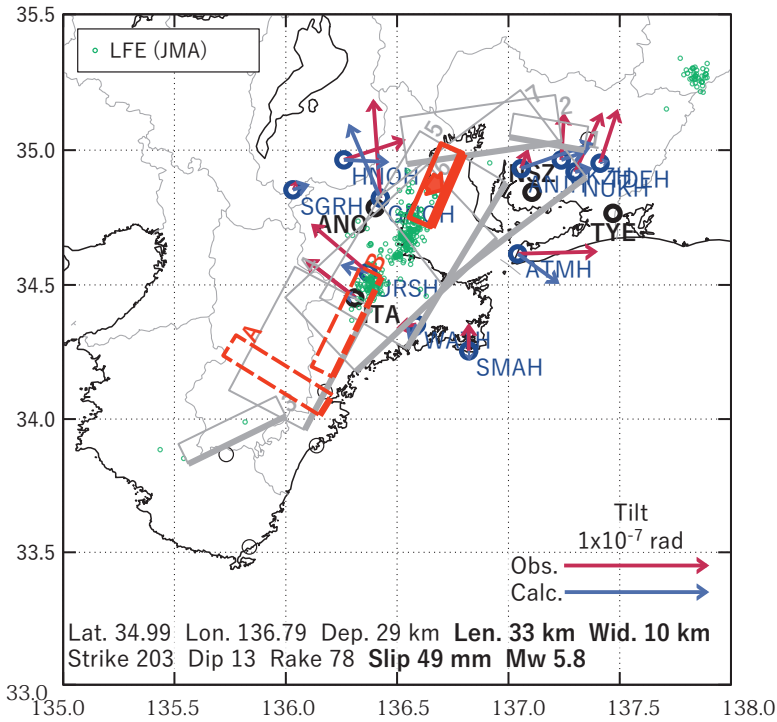
第 26 図 第 18-23 図 [C] を説明する断層モデル. 各図の説明は第 3 図を参照.
