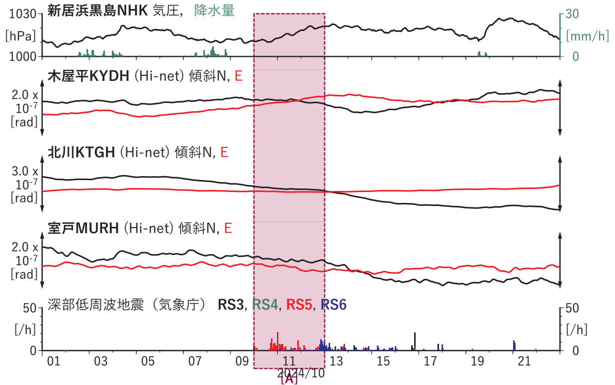
第 39 図 四国地方における傾斜の観測結果と低周波地震の検出数 (2024/10/01 ~ 2024/10/22).
