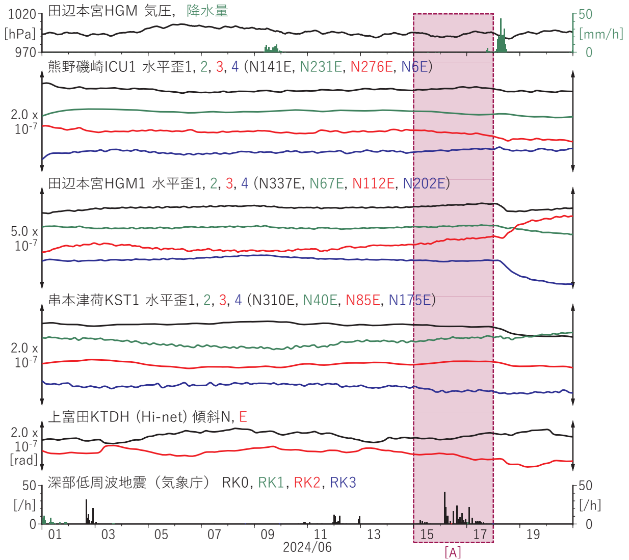
第 5 図 紀伊半島における歪・傾斜の観測結果と低周波地震の検出数 (2024/06/01 ~ 2024/06/20).
