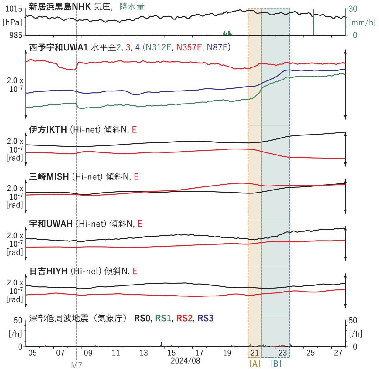
第 30 図 四国地域における歪・傾斜の観測結果と低周波地震の検出数 (2024/08/05 ~ 2024/08/27).
