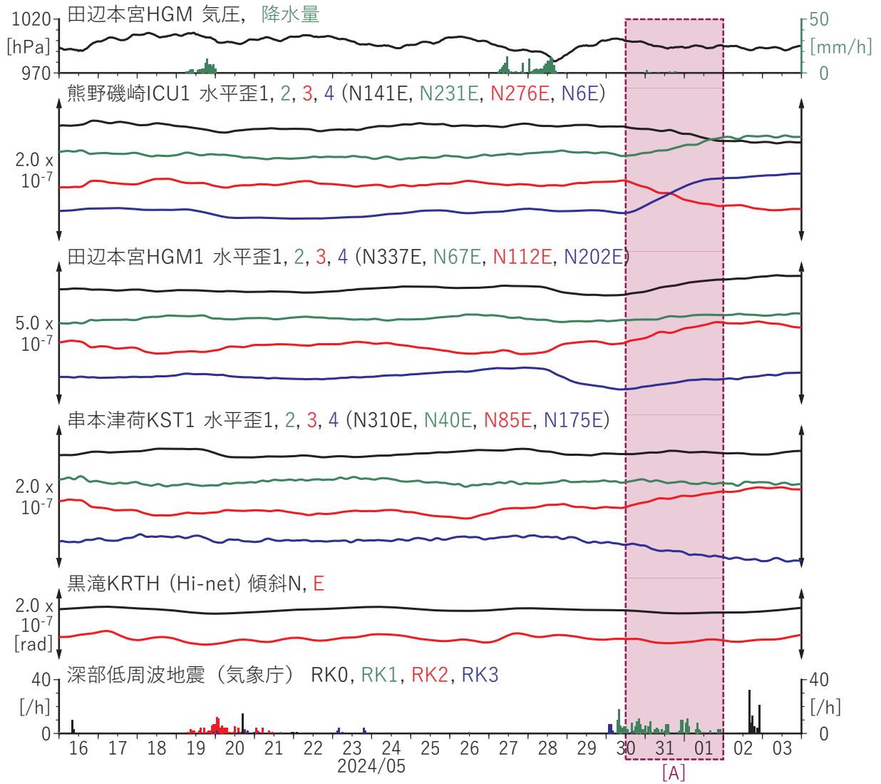
第 2 図 紀伊半島における歪・傾斜の観測結果と低周波地震の検出数 (2024/05/16 ~ 2024/06/03)。
