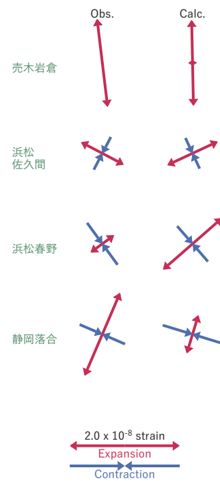
(b2) 主歪
