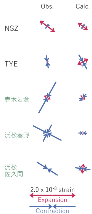
(b2) 主歪
