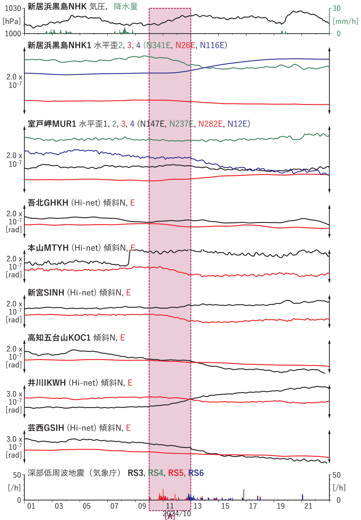
第 38 図 四国地方における歪・傾斜の観測結果と低周波地震の検出数 (2024/10/01 ~ 2024/10/22).
