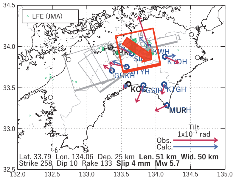
第 40 図 第 38-39 図 [A] を説明する断層モデル. 各図の説明は第 3 図を参照.
