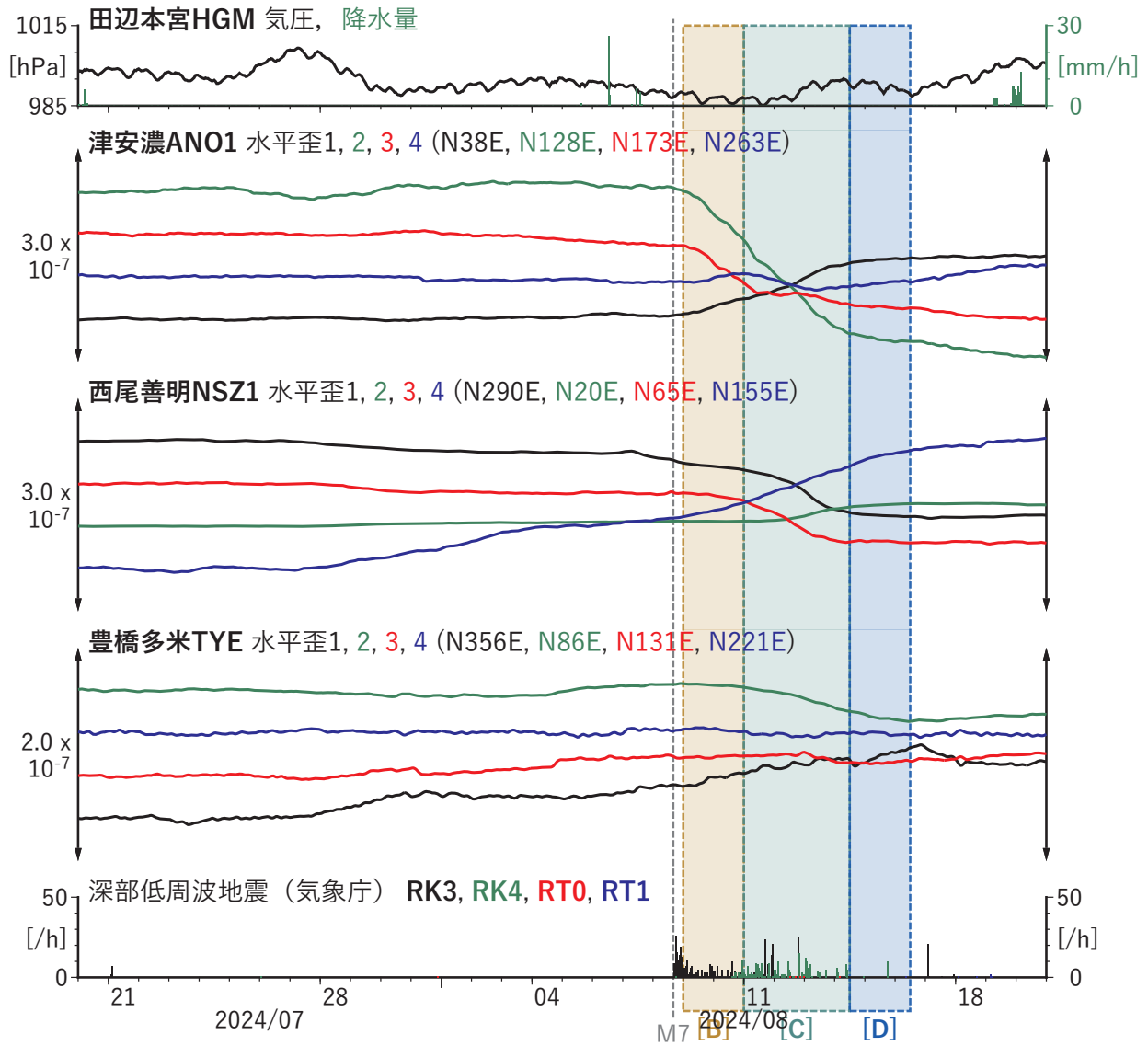
第 19 図 紀伊半島～東海地方における歪の観測結果と低周波地震の検出数（2024/07/20～2024/08/20）． [M7] は日向灘における Mj7.1 の地震の発生時刻．
