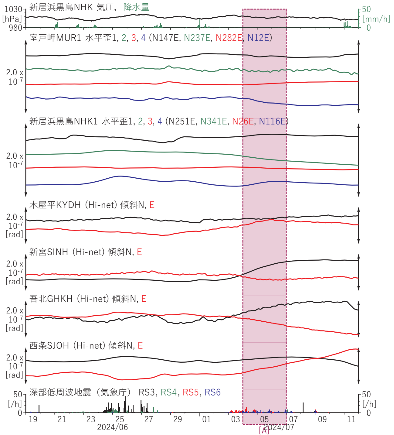
第 15 図 四国地域における歪・傾斜の観測結果と低周波地震の検出数 (2024/06/19 ~ 2024/07/11).
