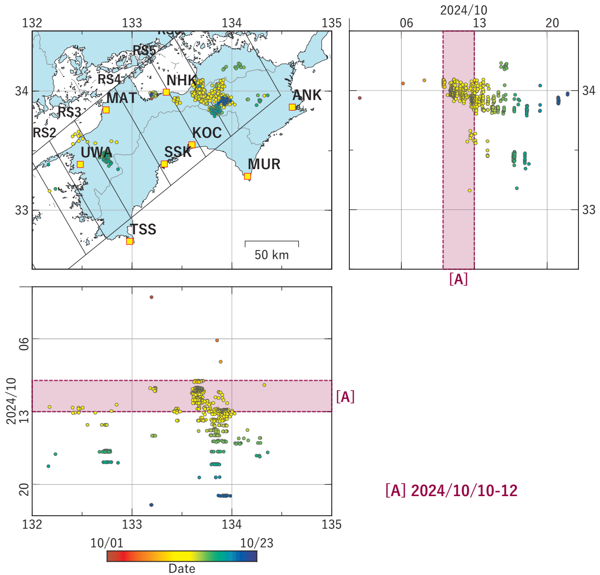
第 37 図 四国地方における低周波地震（気象庁一元化カタログによる）の時空間分布（2024/10/01 ～ 2024/10/22）。
