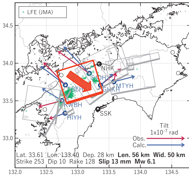
第 13 図 第 12 図 [A] を説明する断層モデル。各図の説明は第 3 図を参照。
