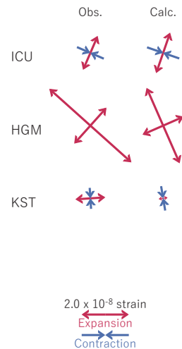
第 3 図 第 2 図 [A] を説明する断層モデル. 以下の凡例の説明は以降の同様の図に共通. (図によっては気象庁・静岡県の観測点や (b3) 体積歪の結果はない場合がある.) 黒・緑・青の丸印はそれぞれ産総研・気象庁および静岡県・防災科研 Hi-net の観測点, 緑の小さな丸印は気象庁の推定した低周波地震. (a) 1 段階目の結果. 灰色の濃淡は残差の総和で, 赤色矩形が残差の総和が最小となる断層面の位置 (大きさは 20x20 km で固定). (b1) 2 段階目の結果. 赤色矩形が残差の総和が最小となる断層面. 矢印は傾斜の観測値と計算値の比較. 灰色矩形は最近周辺で発生した短期的 SSE の推定断層面 (番号との対応は本文参照). (b2) 主歪の観測値と (b1) に示した断層モデルから求めた計算値との比較. (b3) 体積歪の観測値と (b1) に示した断層モデルから求めた計算値との比較.
