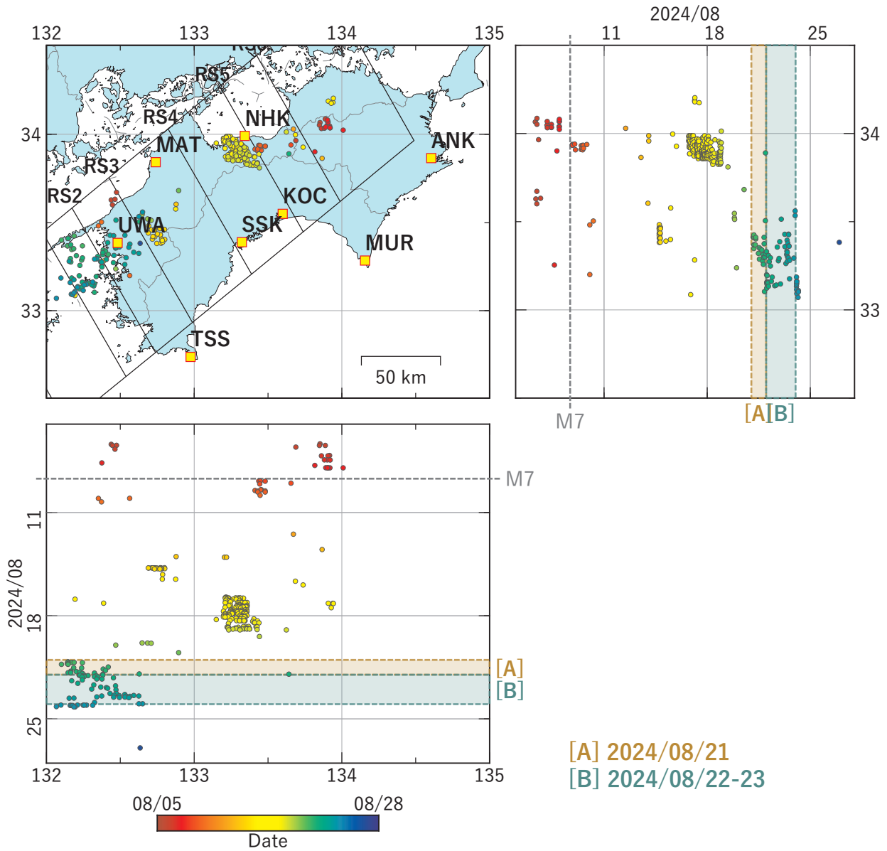
第 29 図 四国地域における低周波地震（気象庁一元化カタログによる）の時空間分布（2024/08/05 ～ 2024/08/27）。
