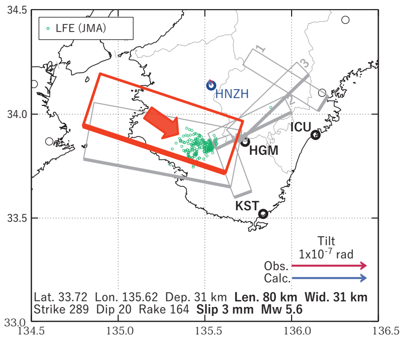
第 35 図 第 34 図 [A] を説明する断層モデル. 各図の説明は第 3 図を参照.
