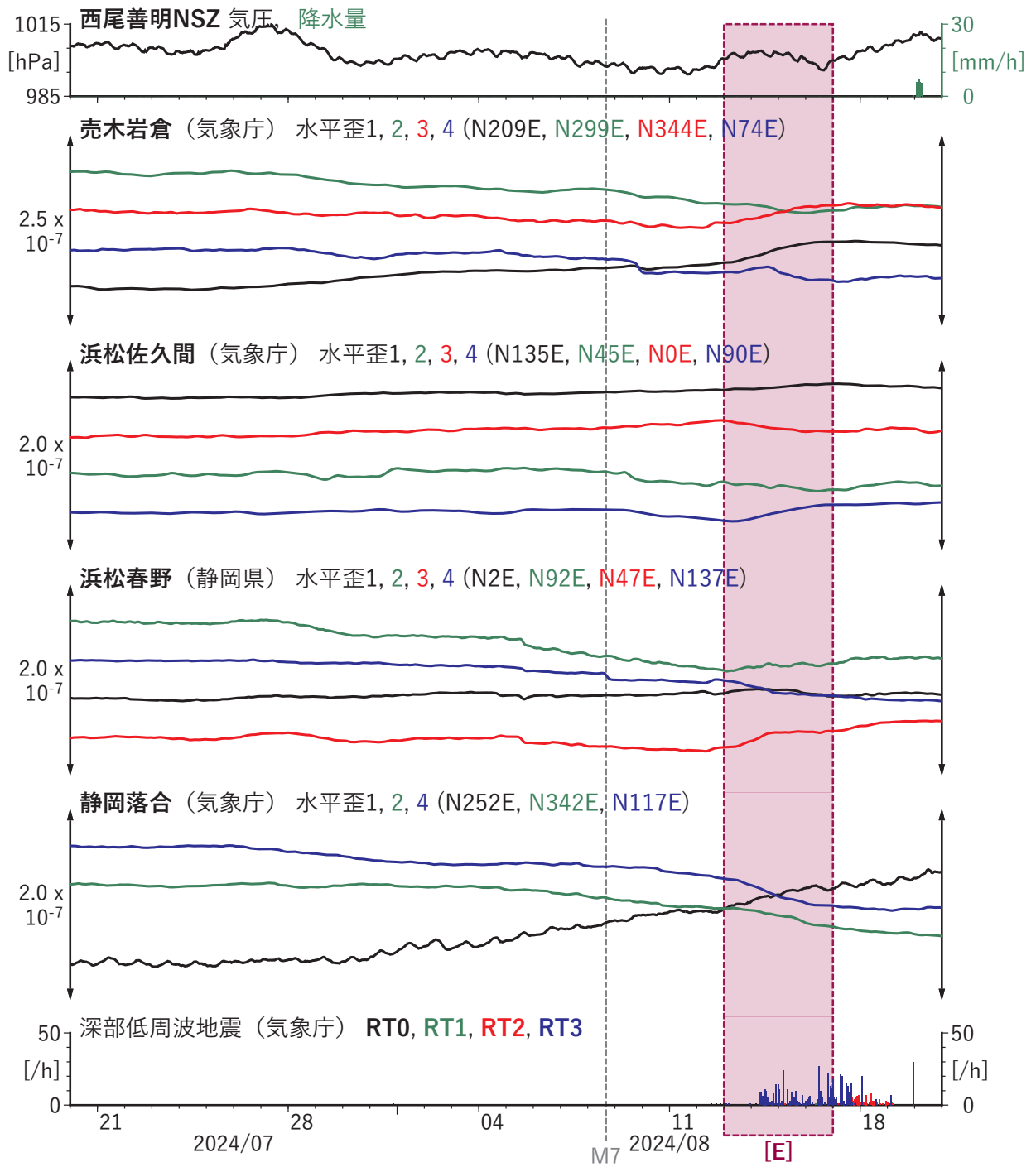
第 20 図 東海地方における歪の観測結果と低周波地震の検出数 (2024/07/20 ~ 2024/08/20). [M7] は日向灘における Mj7.1 の地震の発生時刻.
