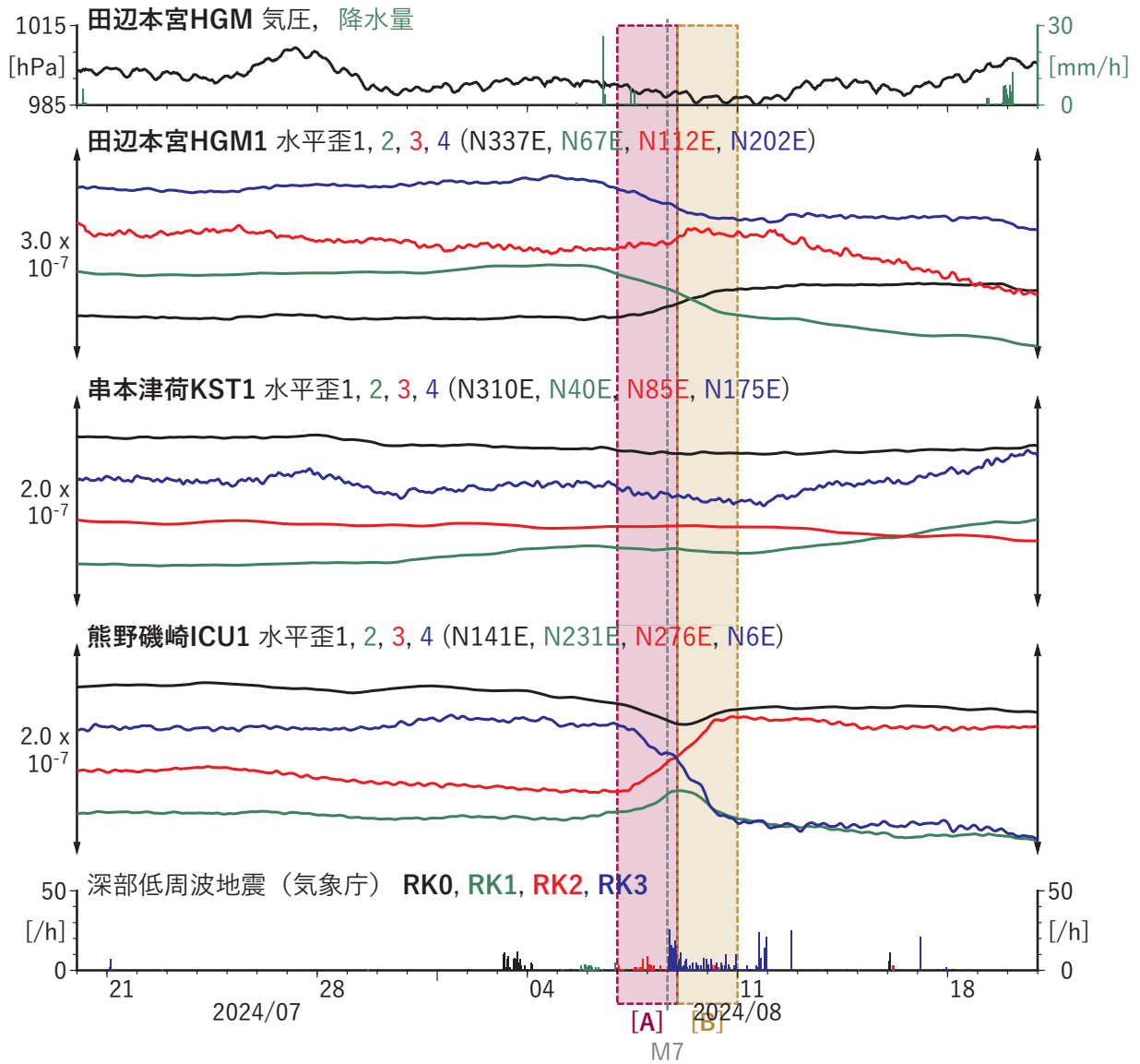
第 18 図 紀伊半島における歪の観測結果と低周波地震の検出数 (2024/07/20 ~ 2024/08/20). [M7] は日向灘における Mj7.1 の地震の発生時刻.
