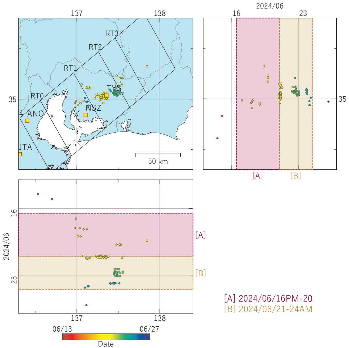
第 7 図 東海地方における低周波地震（気象庁一元化カタログによる）の時空間分布（2024/06/13 ～ 2024/06/26）。
