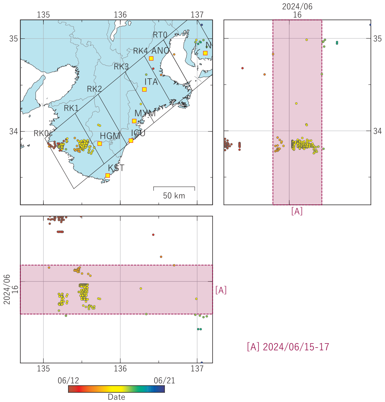
第 4 図 紀伊半島における低周波地震（気象庁一元化カタログによる）の時空間分布（2024/06/12 ～ 2024/06/20）。
