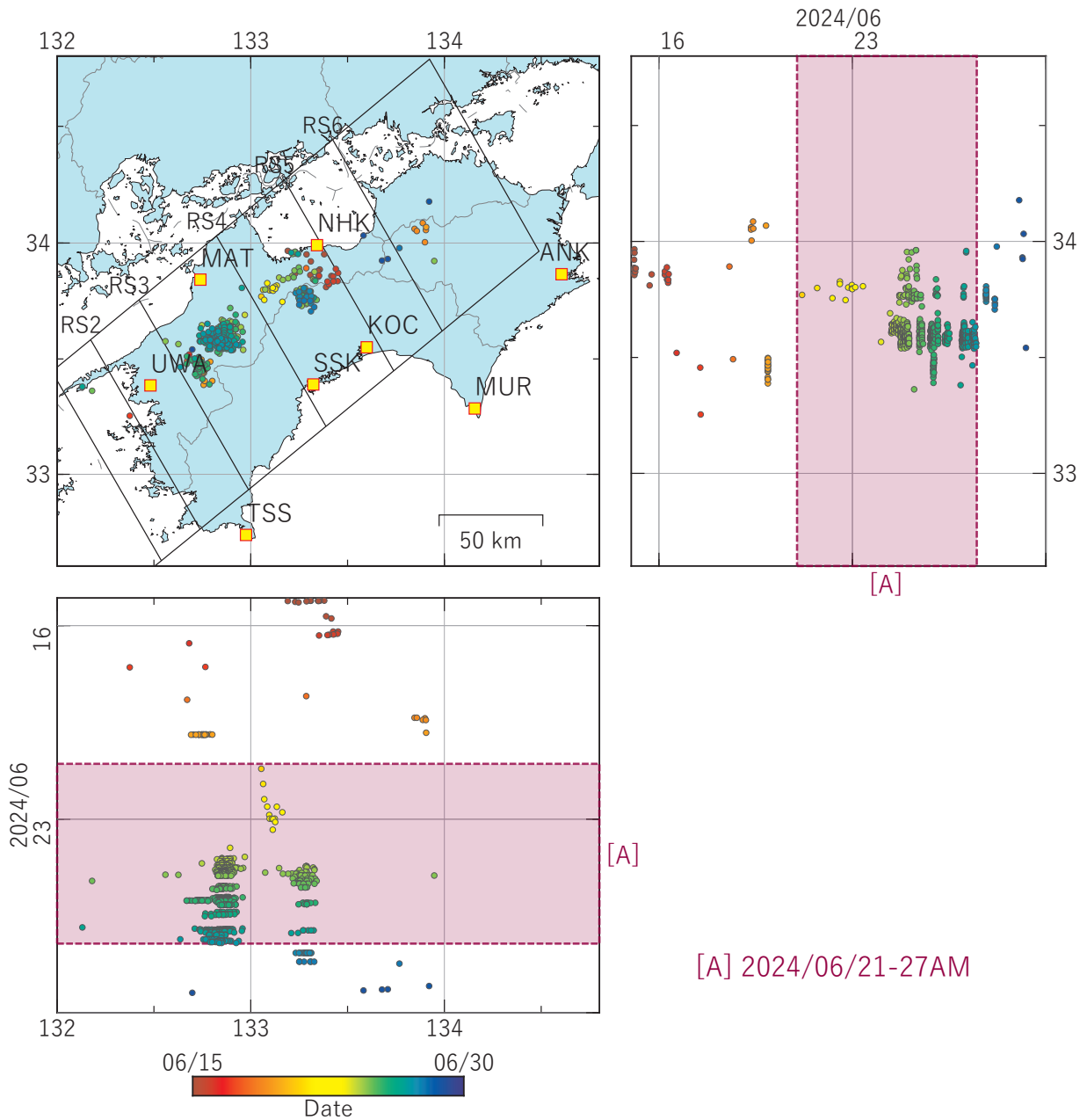
第 11 図 四国地方における低周波地震（気象庁一元化カタログによる）の時空間分布（2024/06/15 ～ 2024/06/29）。
