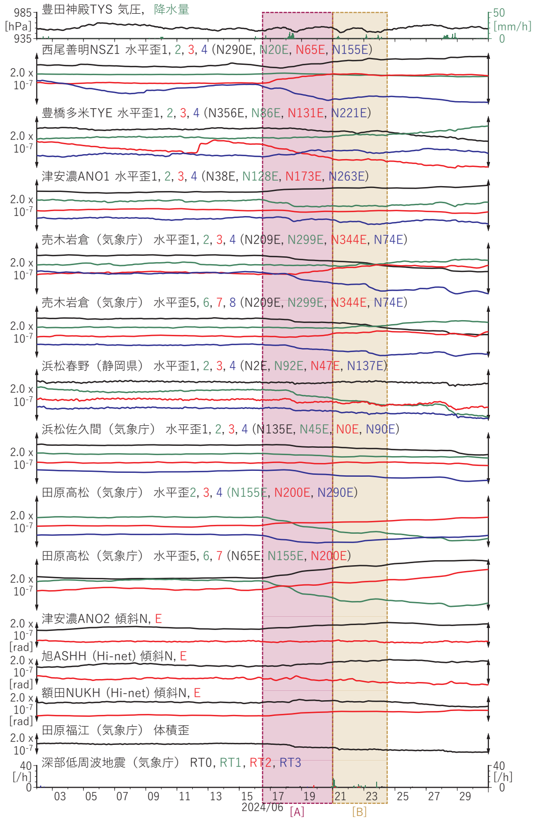
第 8 図 紀伊半島～東海地方における歪・傾斜の観測結果と低周波地震の検出数（2024/06/02～2024/06/30）。
