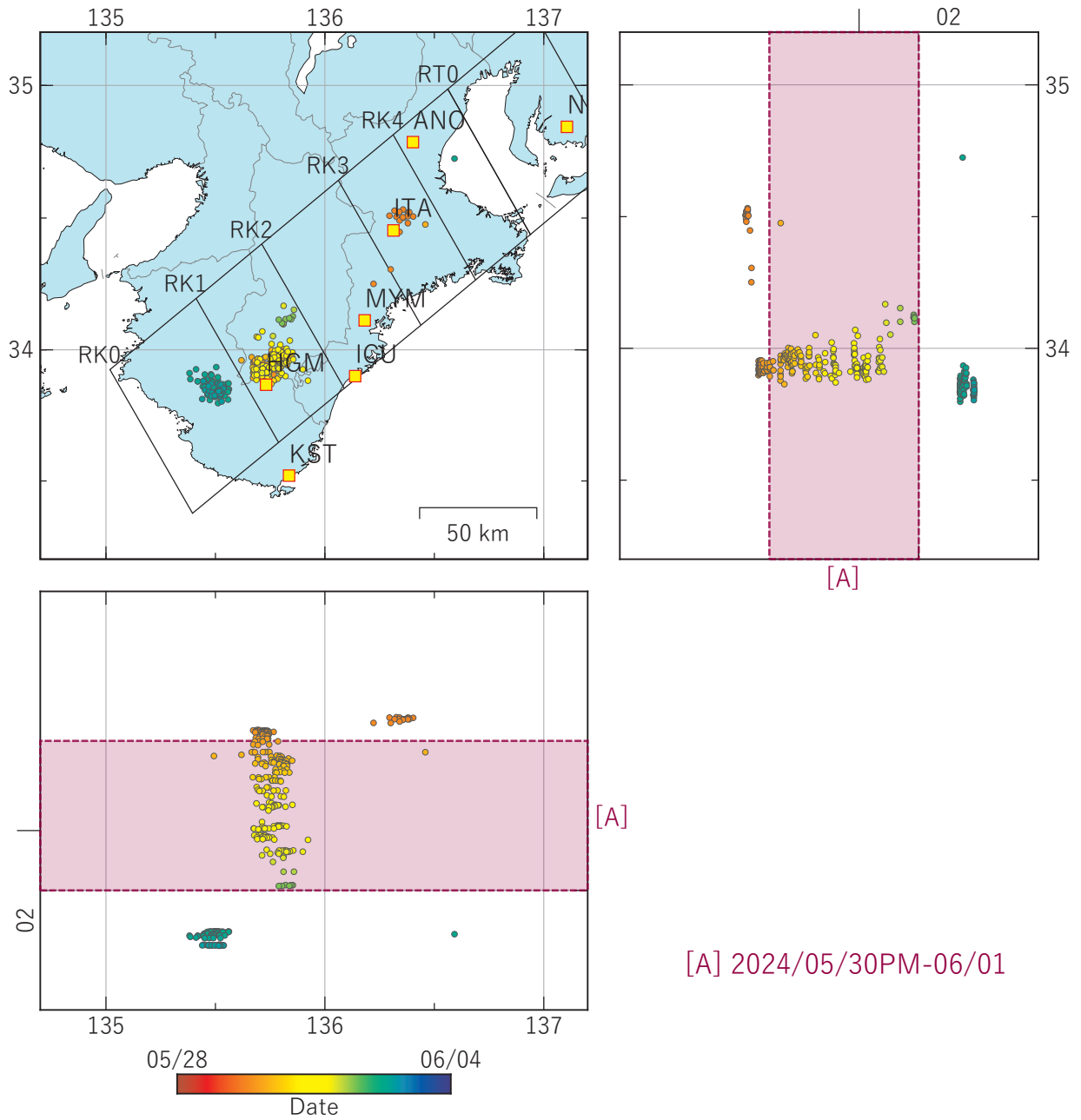
第 1 図 紀伊半島における低周波地震（気象庁一元化カタログによる）の時空間分布（2024/05/28 ～ 2024/06/03）。
