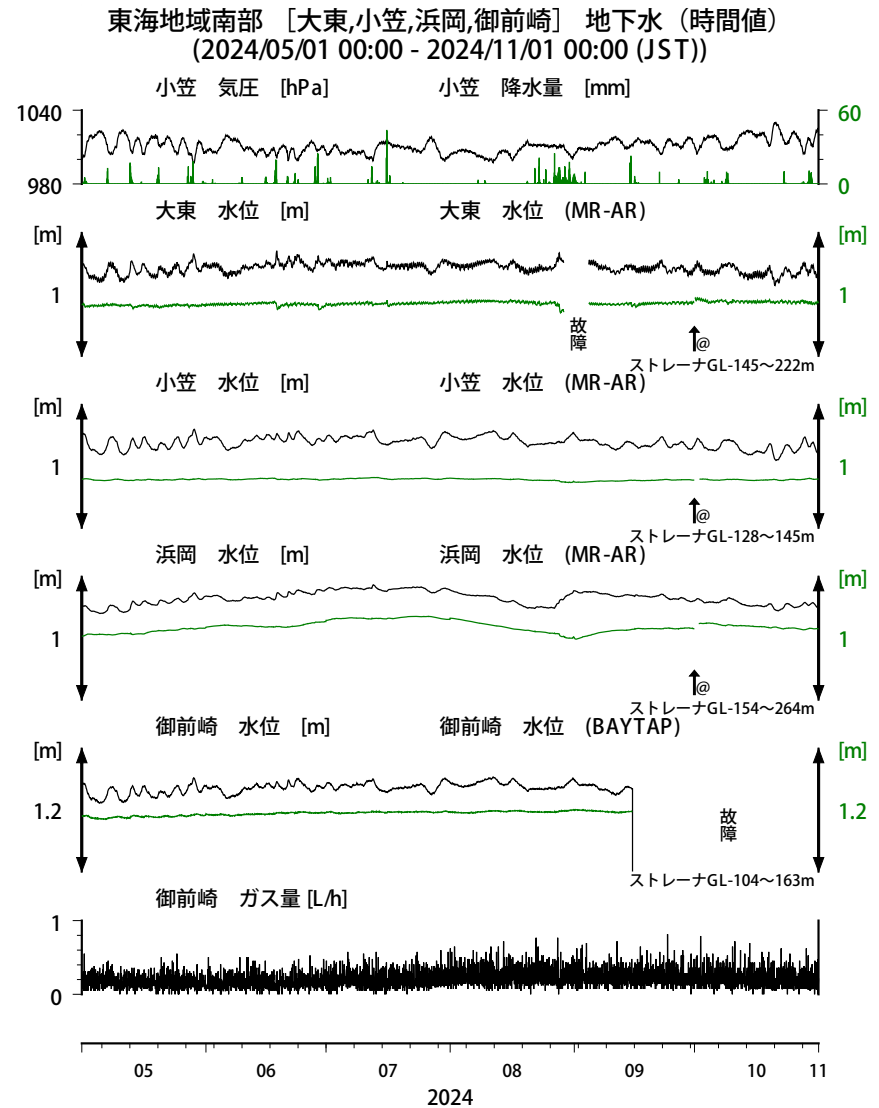
第4図 東海地域南部の地下水等の観測結果 (2024年5月～2024年10月) Fig. 4 Observed groundwater levels and others in the southern Tokai district from May 2024 to Oct. 2024.
