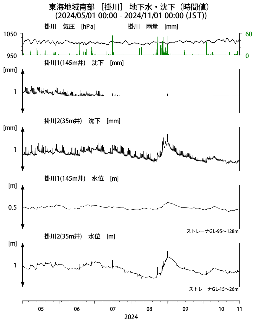
第5図 掛川における沈下等の観測結果 (2024年5月～2024年10月)
