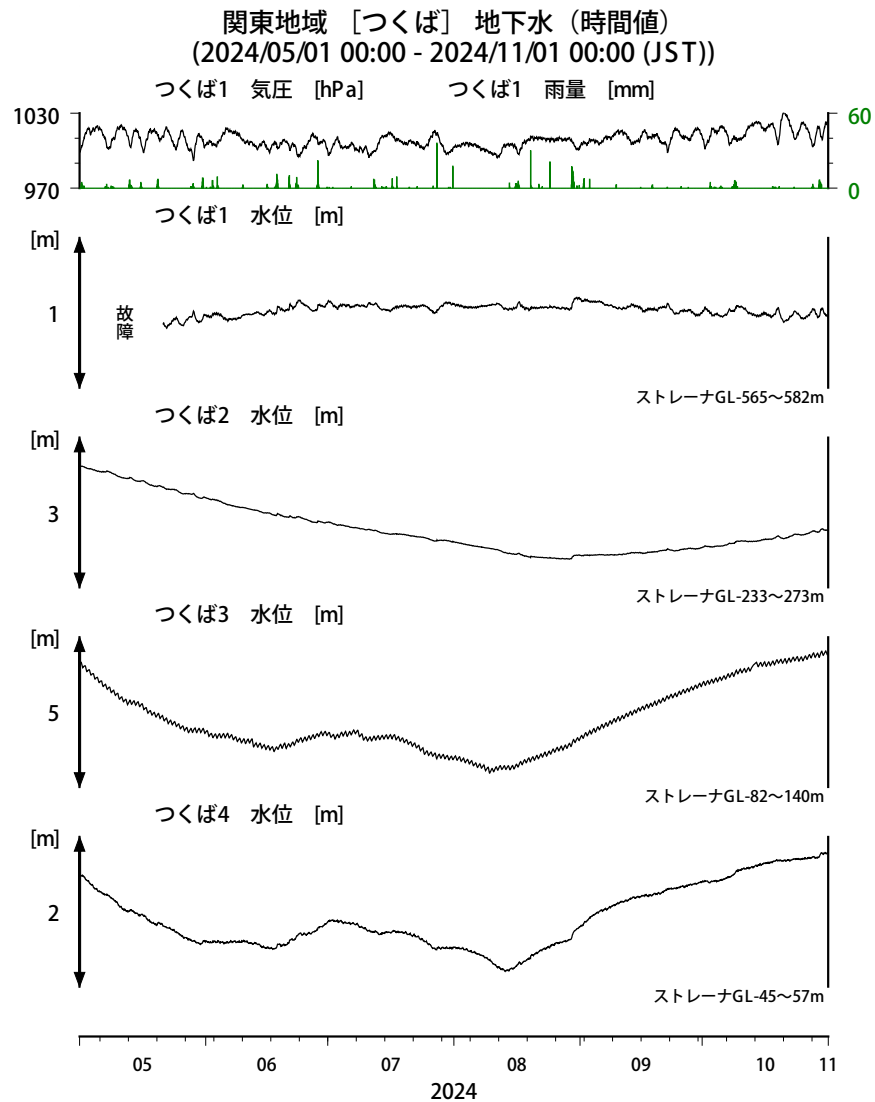
第7図 関東地域の地下水等の観測結果(2024年5月~2024年10月)
