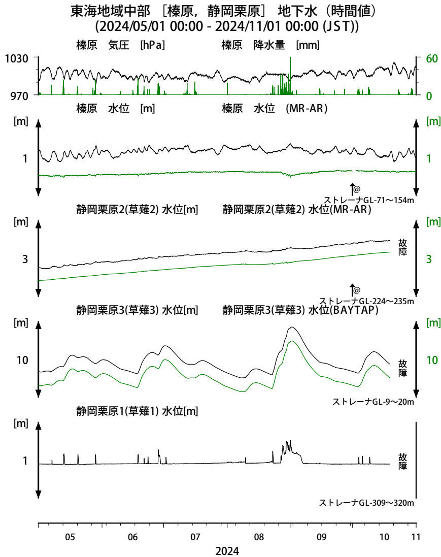
第3図 東海地域中部の地下水等の観測結果 (2024年5月～2024年10月) Fig. 3 Observed groundwater levels and others in the central Tokai district from May 2024 to Oct. 2024.
