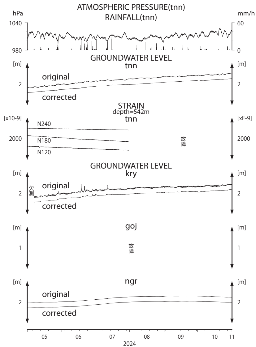
第 4 図 tnn, kry, goj, ngr の 2024 年 5 月～ 2024 年 10 月の観測結果。 Fig. 4 Observation results at tnn, kry, goj and ngr from May 2024 to October 2024.
