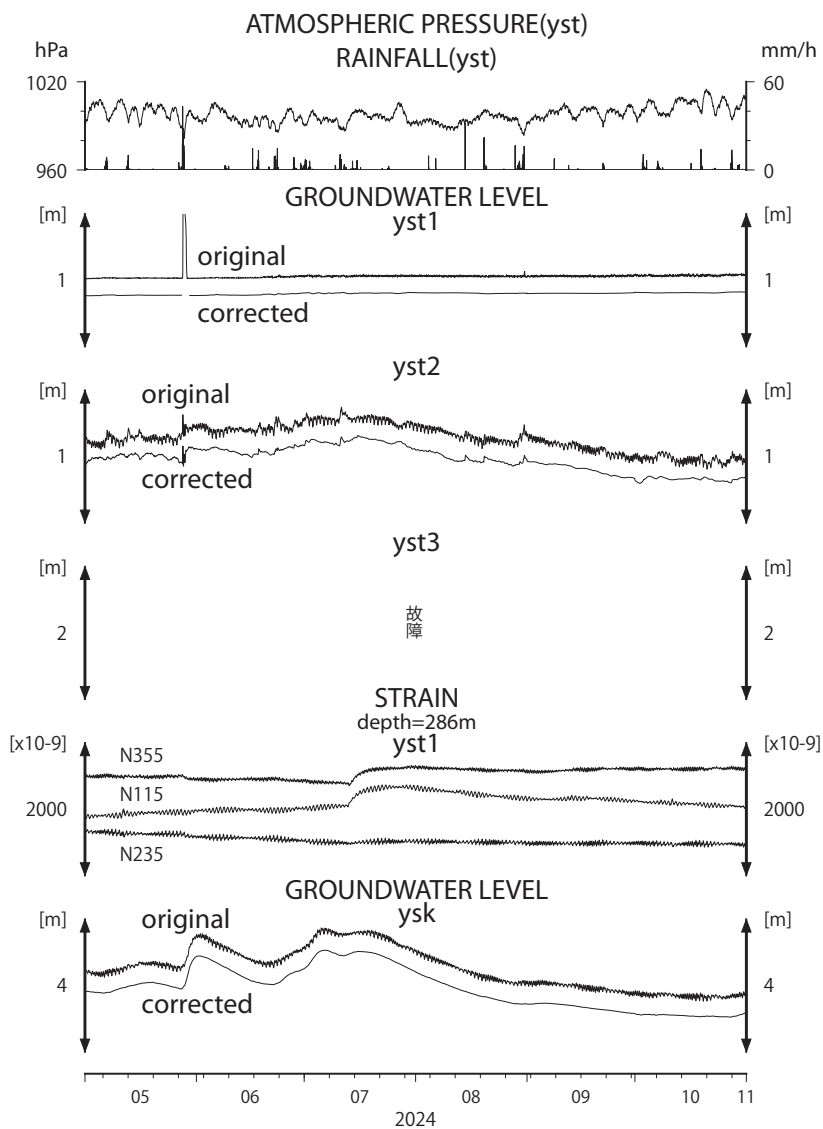
第2図 yst1, yst2, yst3, ysk の2024年5月～2024年10月の観測結果。 Fig. 2 Observation results at yst1, yst2, yst3 and ysk from May 2024 to October 2024.
